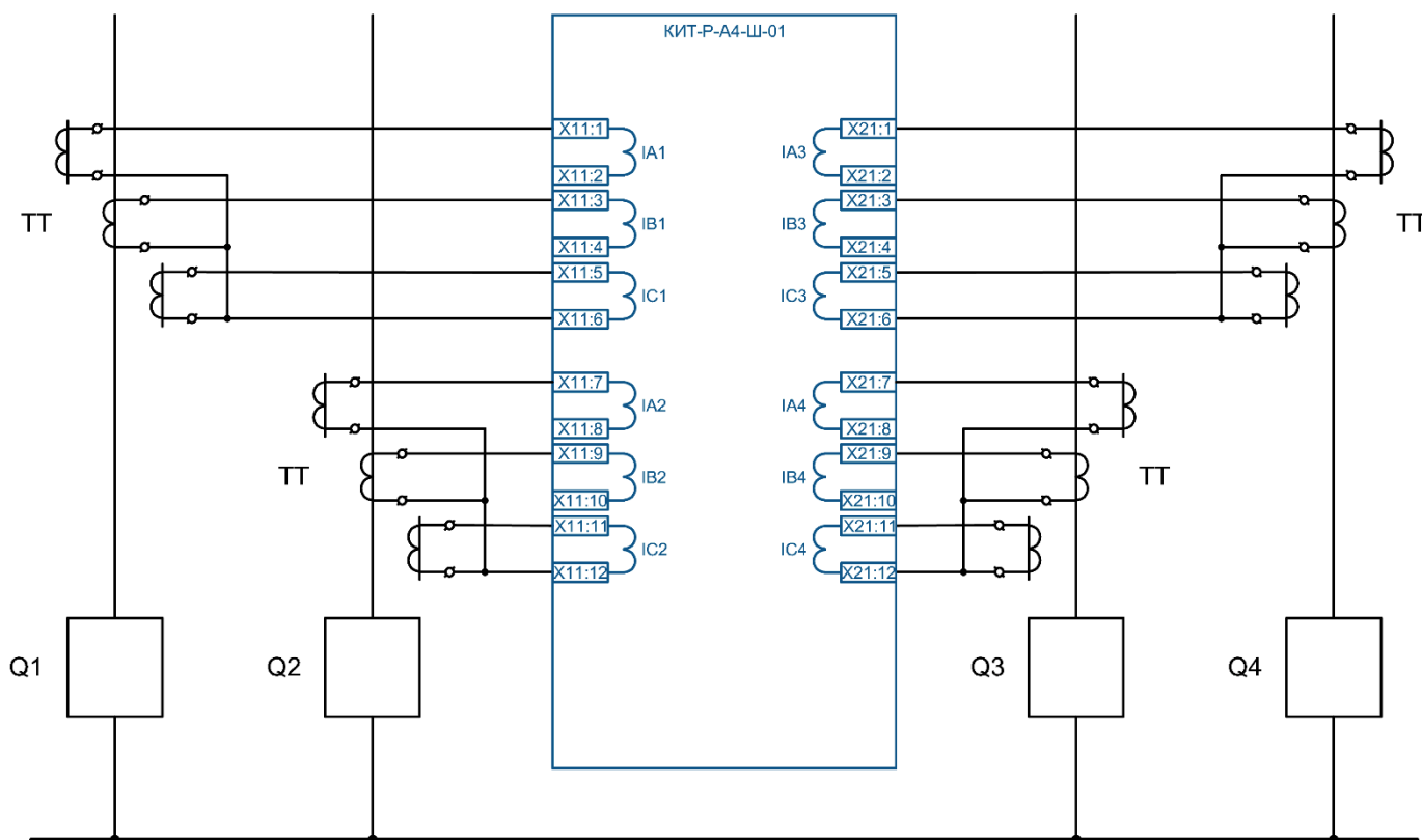
Рисунок 1.1 – Упрощенная схема подключения устройства
