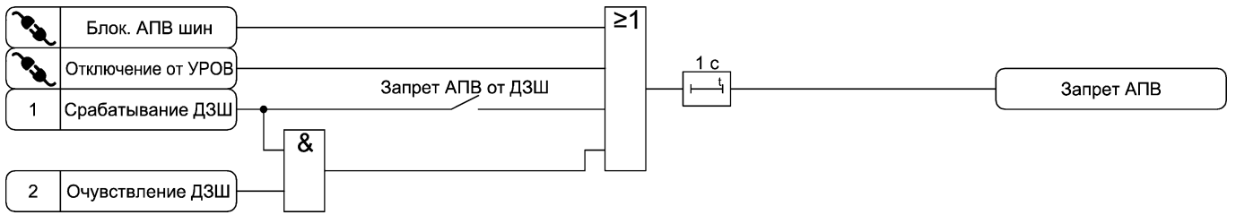
Рисунок А.6 – Функциональная схема алгоритма блокировки АПВ шин
