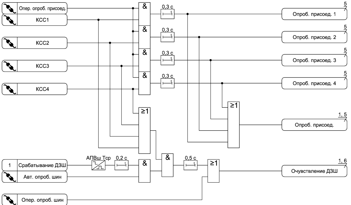
Рисунок А.2 – Функциональная схема алгоритма опробования присоединений / шин
