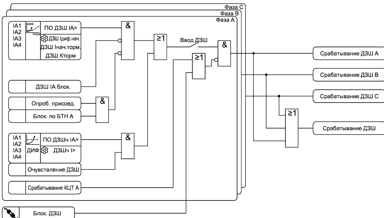
Рисунок 3.1 – Функциональная схема алгоритма ДЗШ
