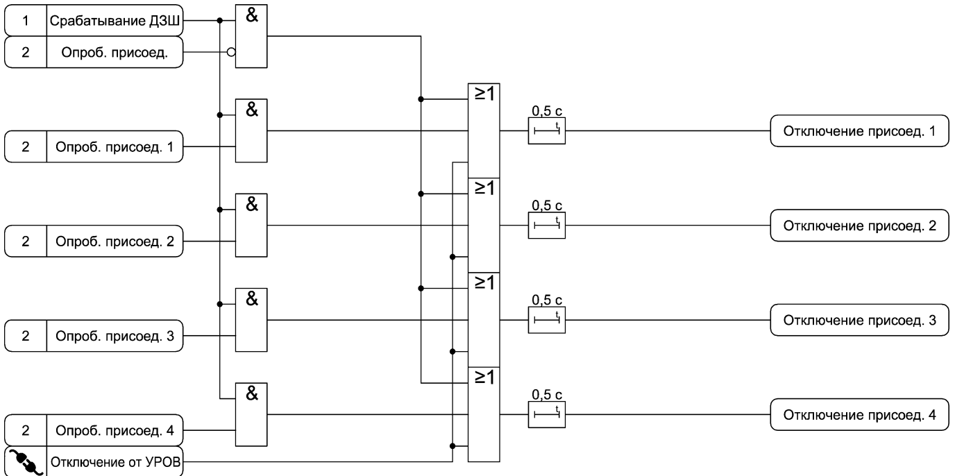
Рисунок А.5 – Функциональная схема алгоритма отключения выключателей присоединений
