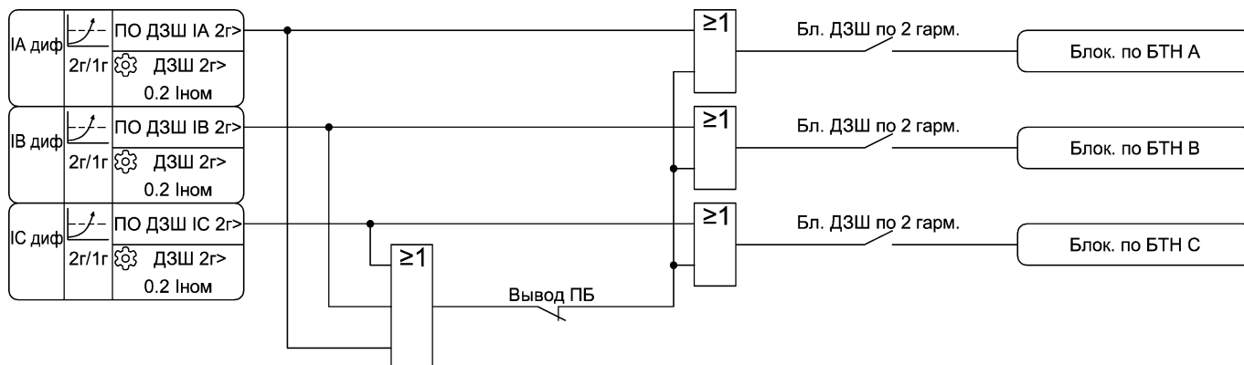
Рисунок 3.4 – Функциональная схема алгоритма блокировки ДЗШ при БТН
