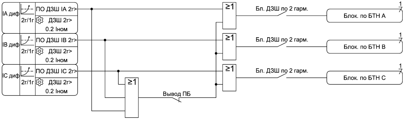
Рисунок А.3 – Функциональная схема блокировки ДЗШ от БТН трансформатора
