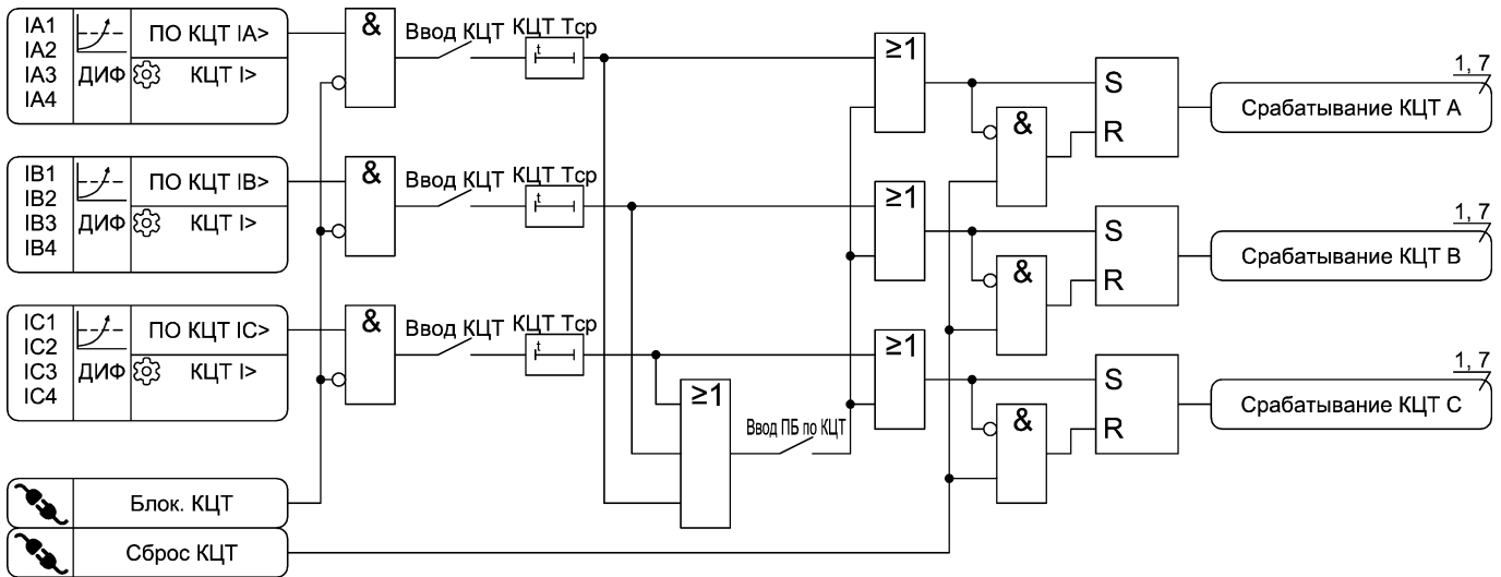
Рисунок А.4 – Функциональная схема алгоритма контроля исправности токовых цепей
