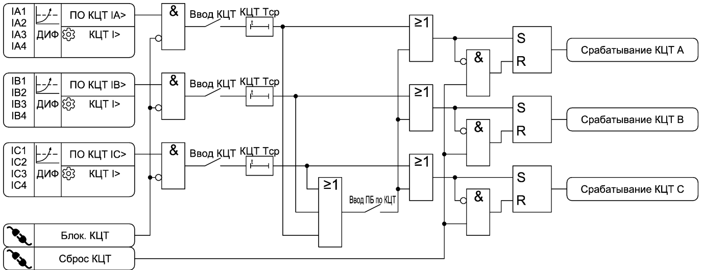
Рисунок 3.5 – Функциональная схема алгоритма КЦТ
