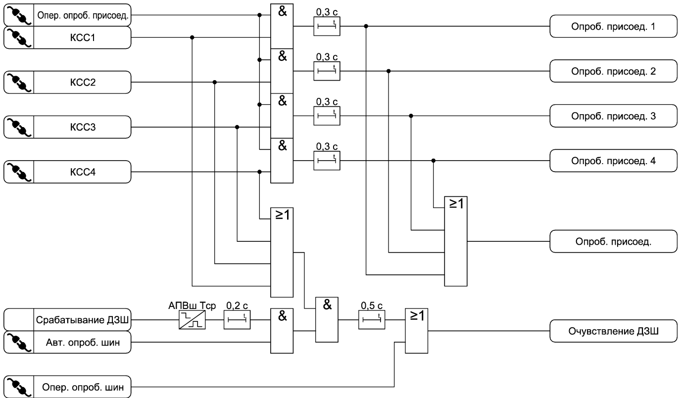
Рисунок 3.3 – Функциональная схема алгоритма опробования присоединений и шин
