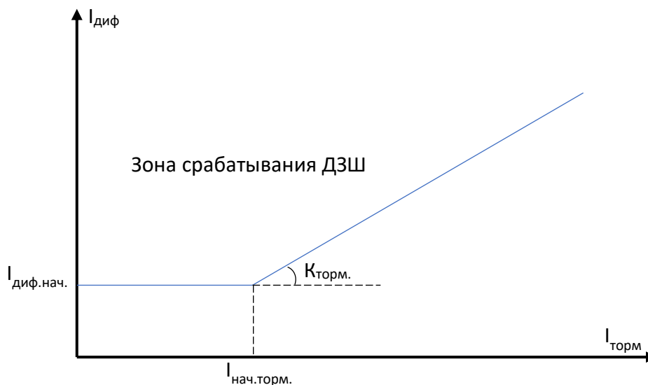
Рисунок 3.2 – Характеристика срабатывания ДЗШ
