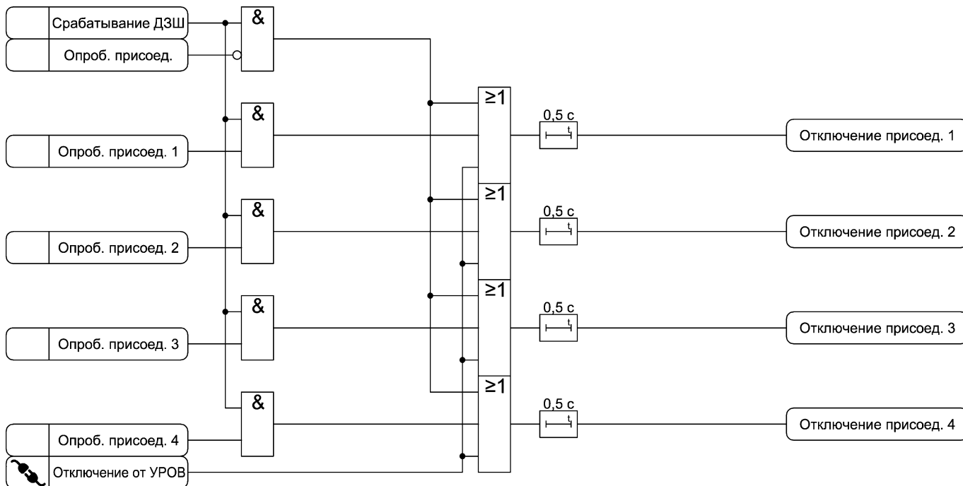
Рисунок 3.6 – Функциональная схема алгоритма отключения выключателей присоединений
