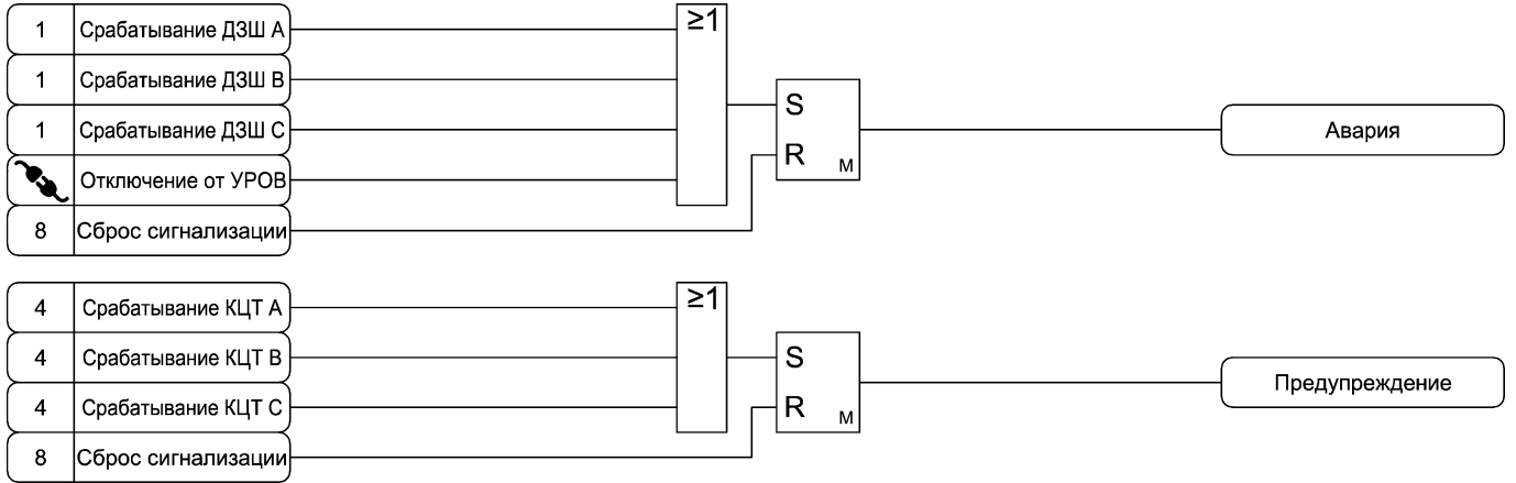
Рисунок А.7 – Функциональная схема сигнализации
