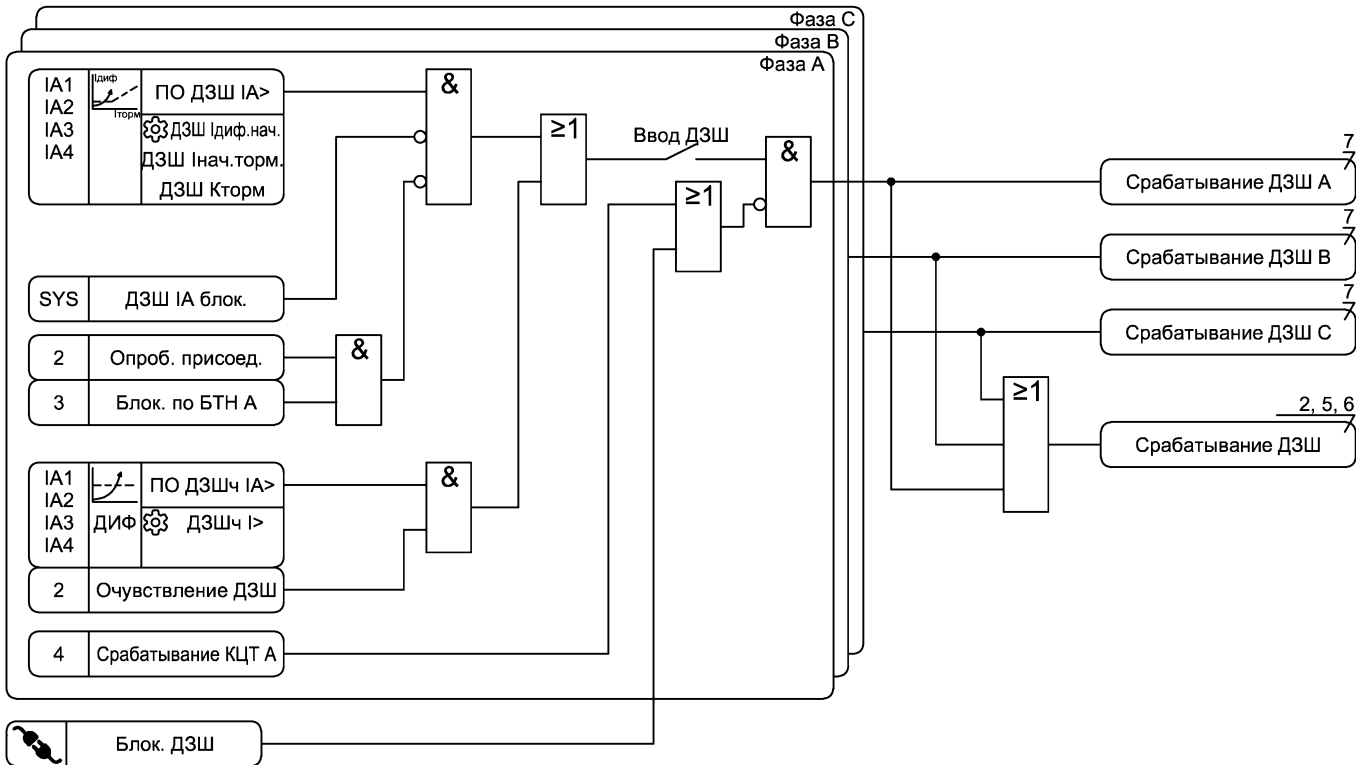
Рисунок А.1 – Функциональная схема алгоритма ДЗШ
