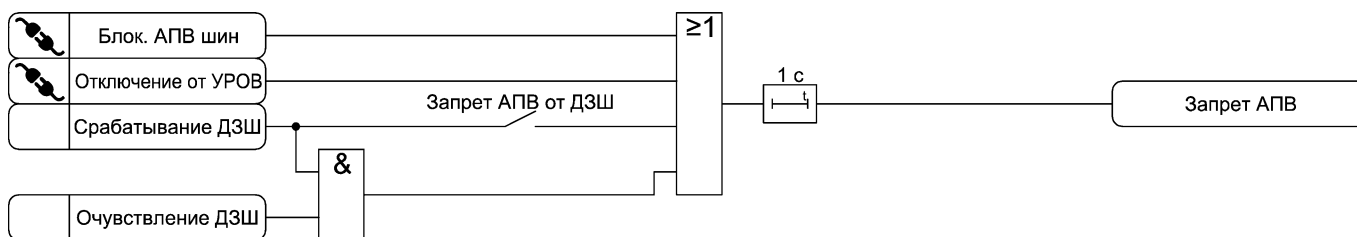
Рисунок 3.7 – Функциональная схема алгоритма запрета АПВ
