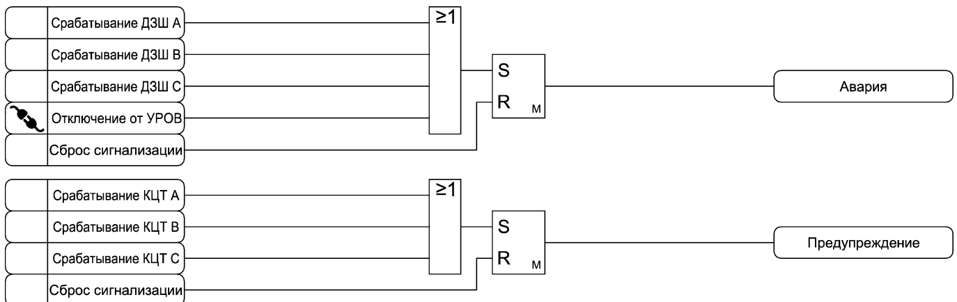
Рисунок 3.8 – Функциональная схема алгоритма сигнализации
