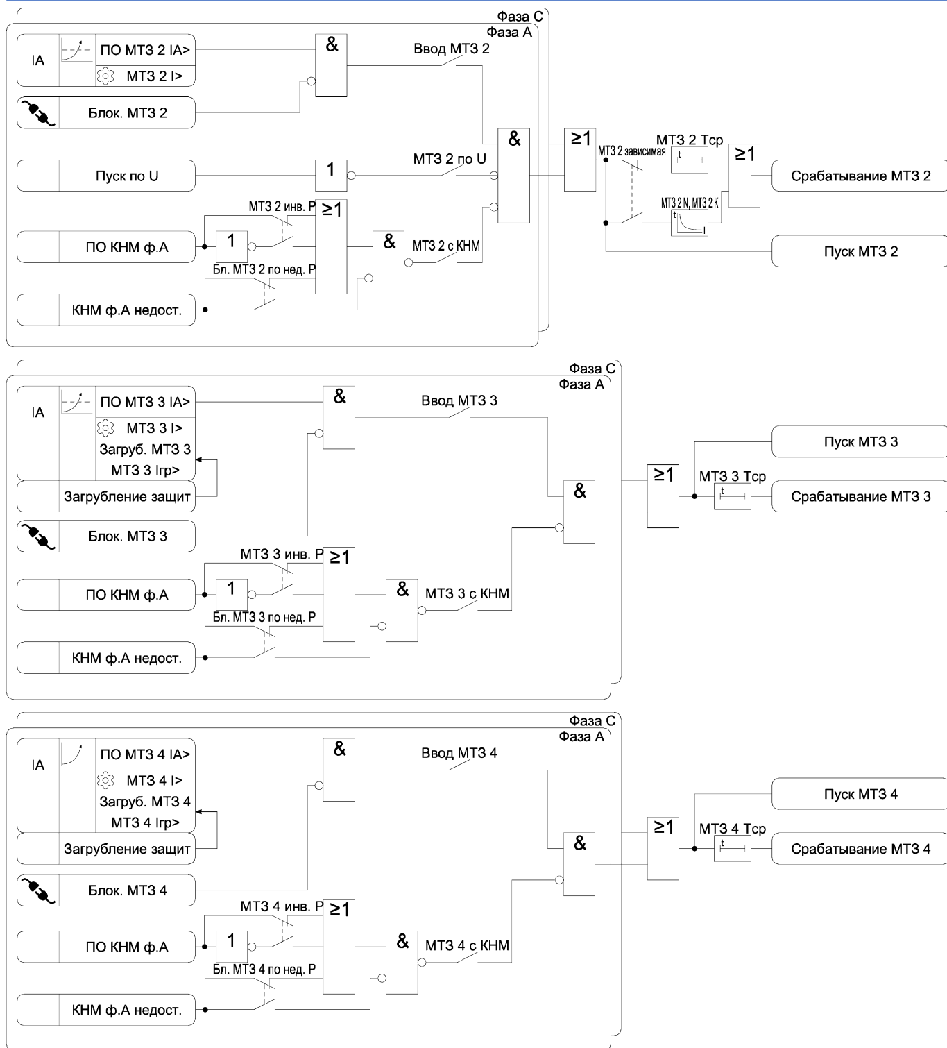
Рисунок 3.2 б) – Функциональная схема алгоритма MT3
