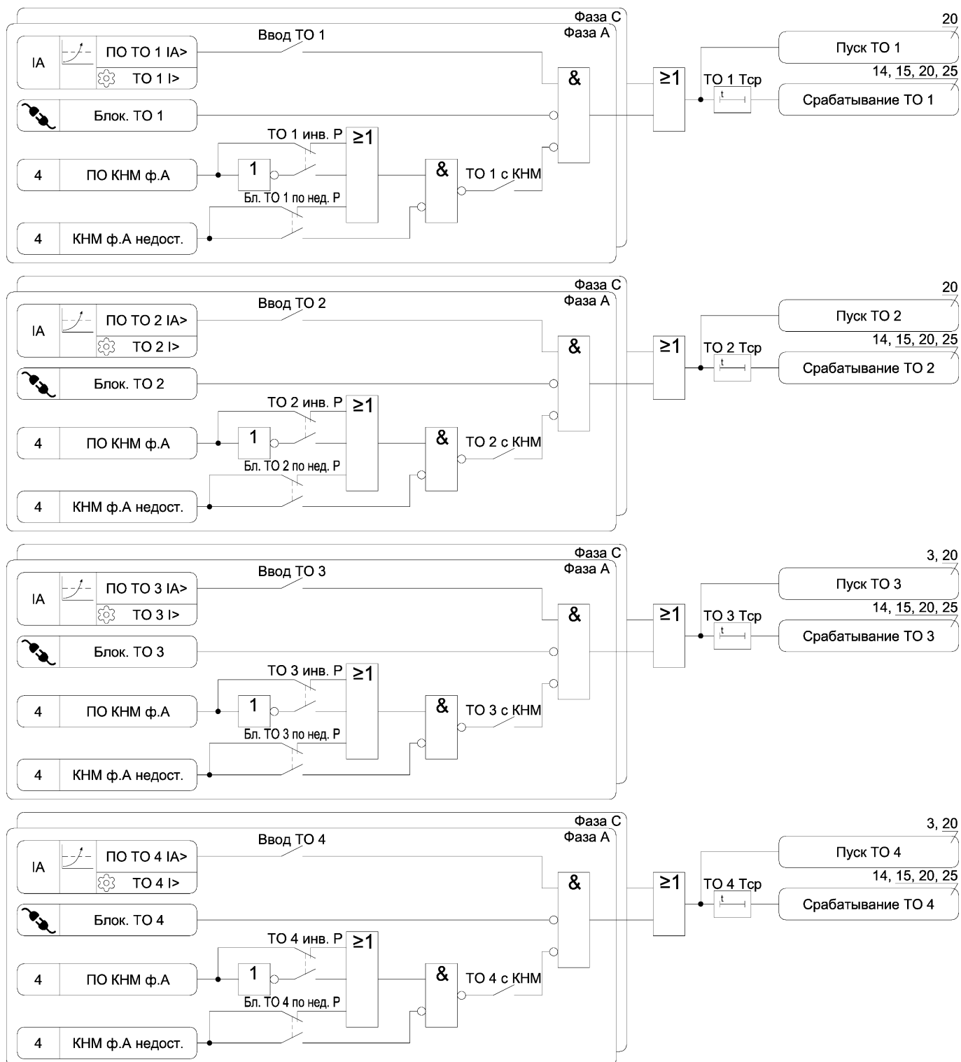
Рисунок А.1 – Функциональная схема алгоритма TO
