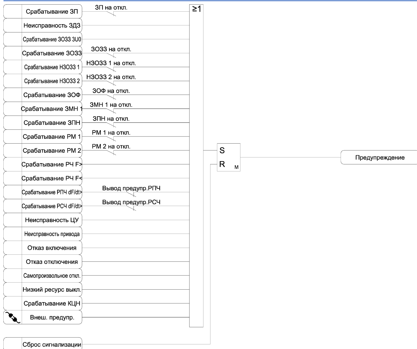
Рисунок 3.27 в) – Функциональная схема алгоритма сигнализации
