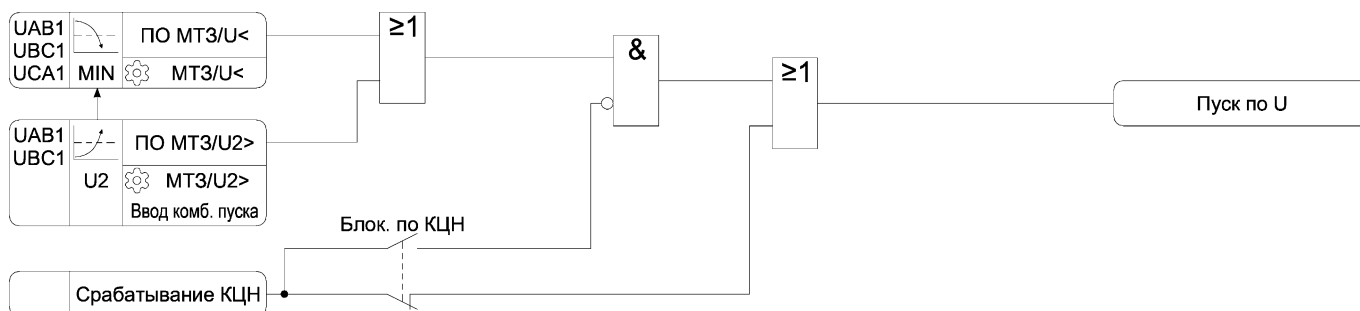
Рисунок 3.5 – Функциональная схема алгоритма МТЗ/У
