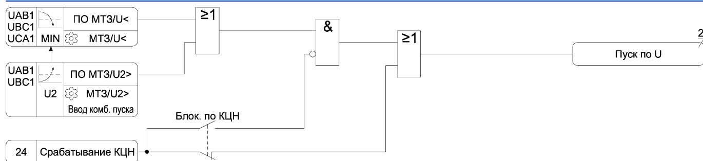
Рисунок А.5 – Функциональная схема алгоритма пуска по напряжению МТЗ
