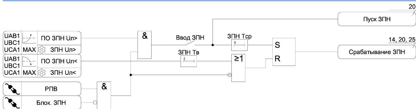
Рисунок А.11 – Функциональная схема алгоритма ЗПН
