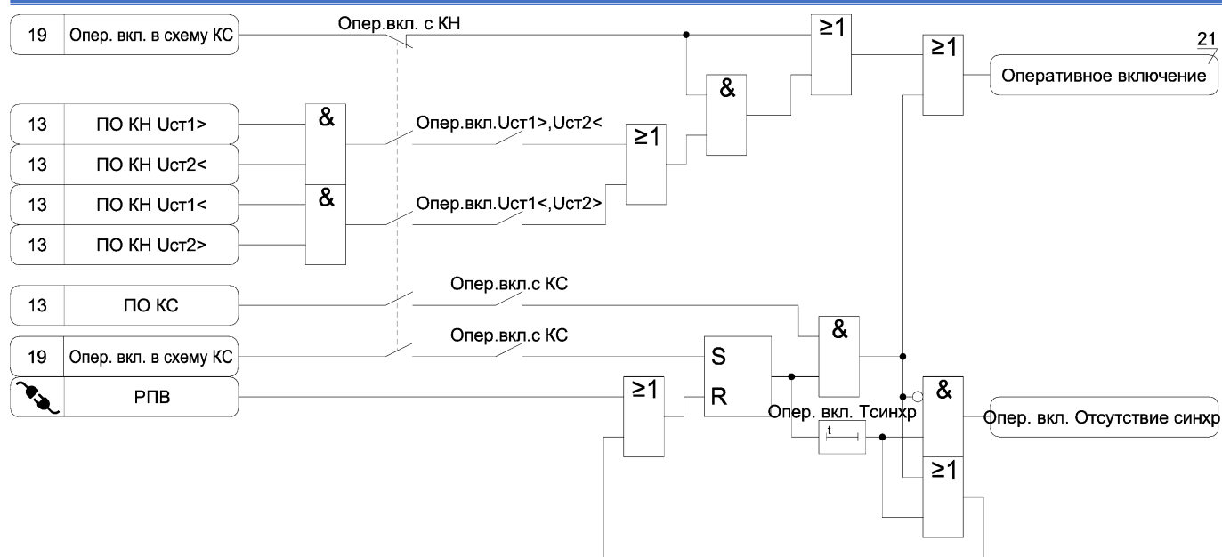
Рисунки А.19 б) – Функциональная схема алгоритма оперативного управления выключателем
