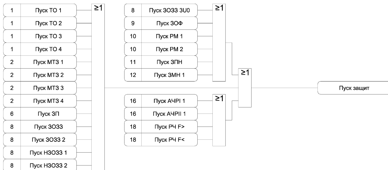
Рисунки А.20 а) – Функциональная схема алгоритма состояния защит
