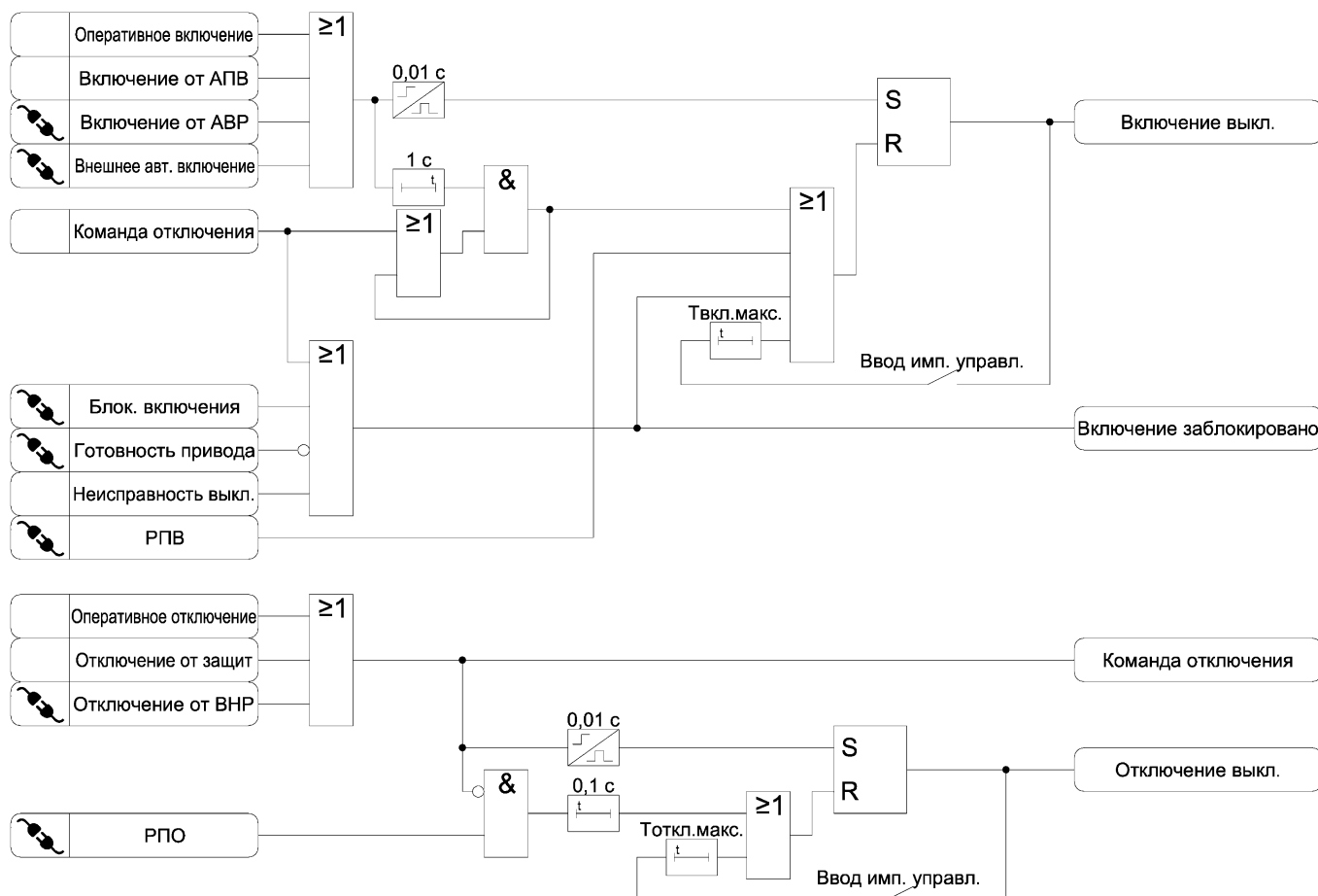
Рисунок 3.13 – Функциональная схема алгоритма управления выключателем
