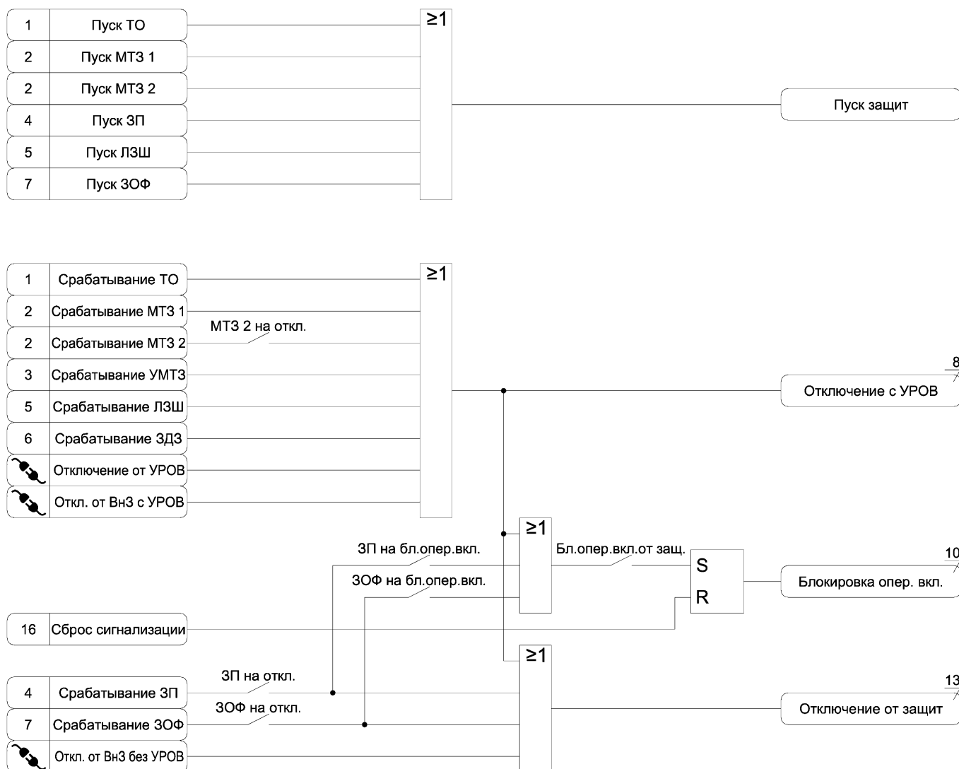
Рисунок А.11 – Функциональная схема алгоритма состояния защит
