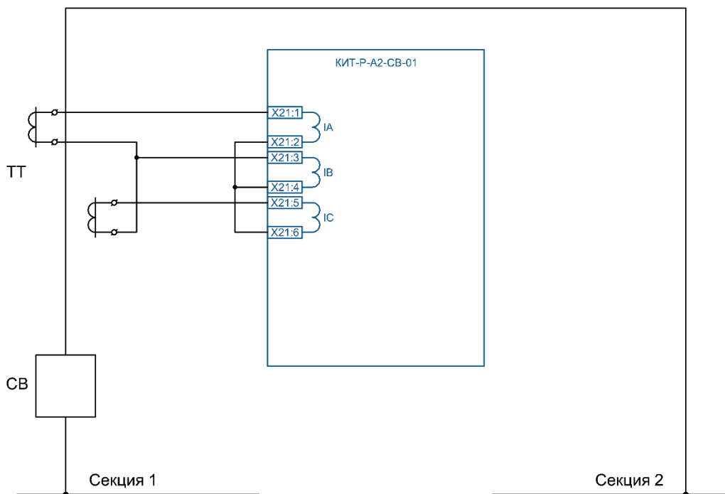
б) схема с двумя ТТ
