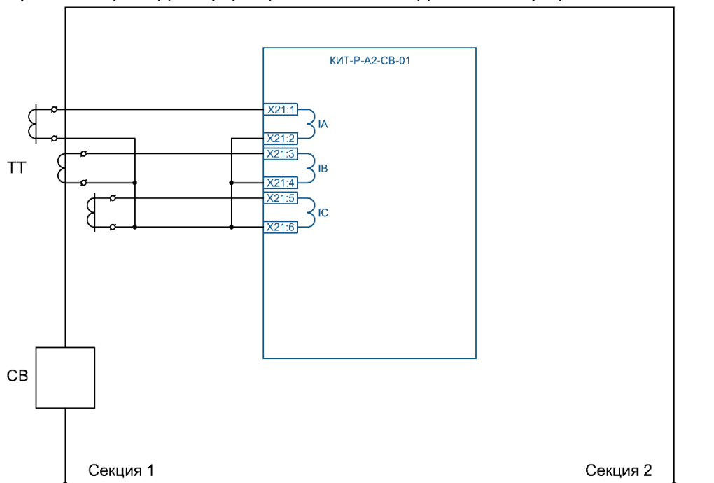
а) схема с тремя ТТ
