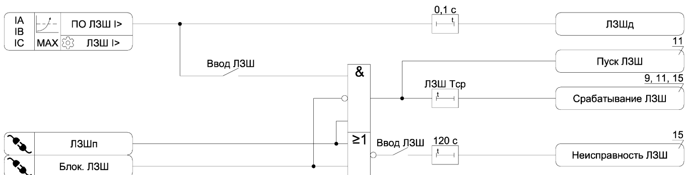
Рисунок А.5 – Функциональная схема алгоритма ЛЗШ
