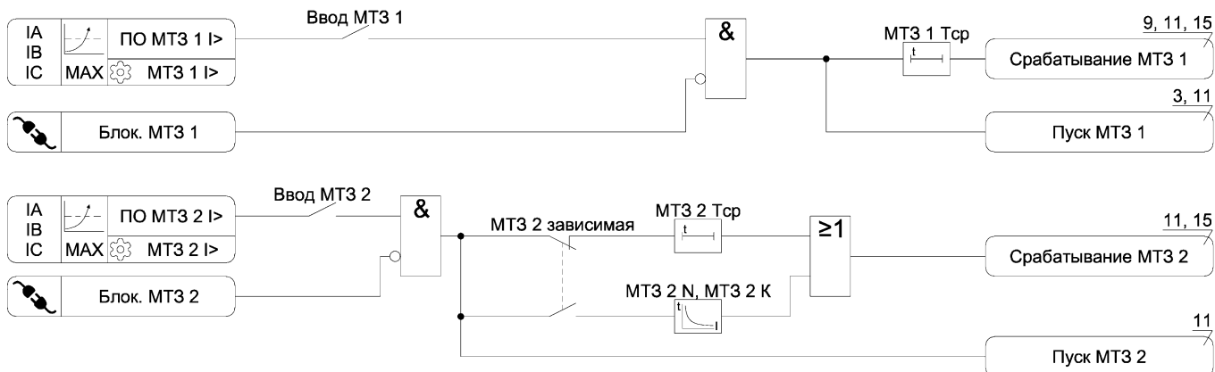
Рисунок А.2 – Функциональная схема алгоритма МТЗ
