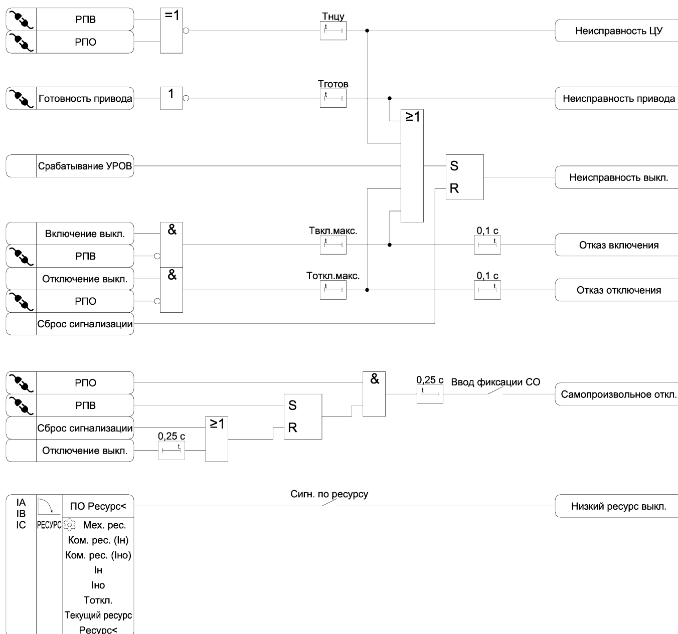
Рисунок 3.14 – Функциональная схема алгоритма диагностики выключателя
