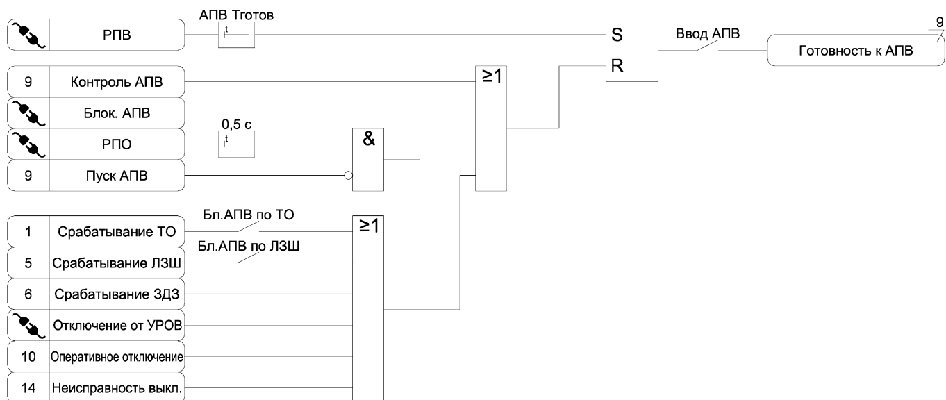
Рисунок А.9 – Функциональная схема алгоритма АПВ
