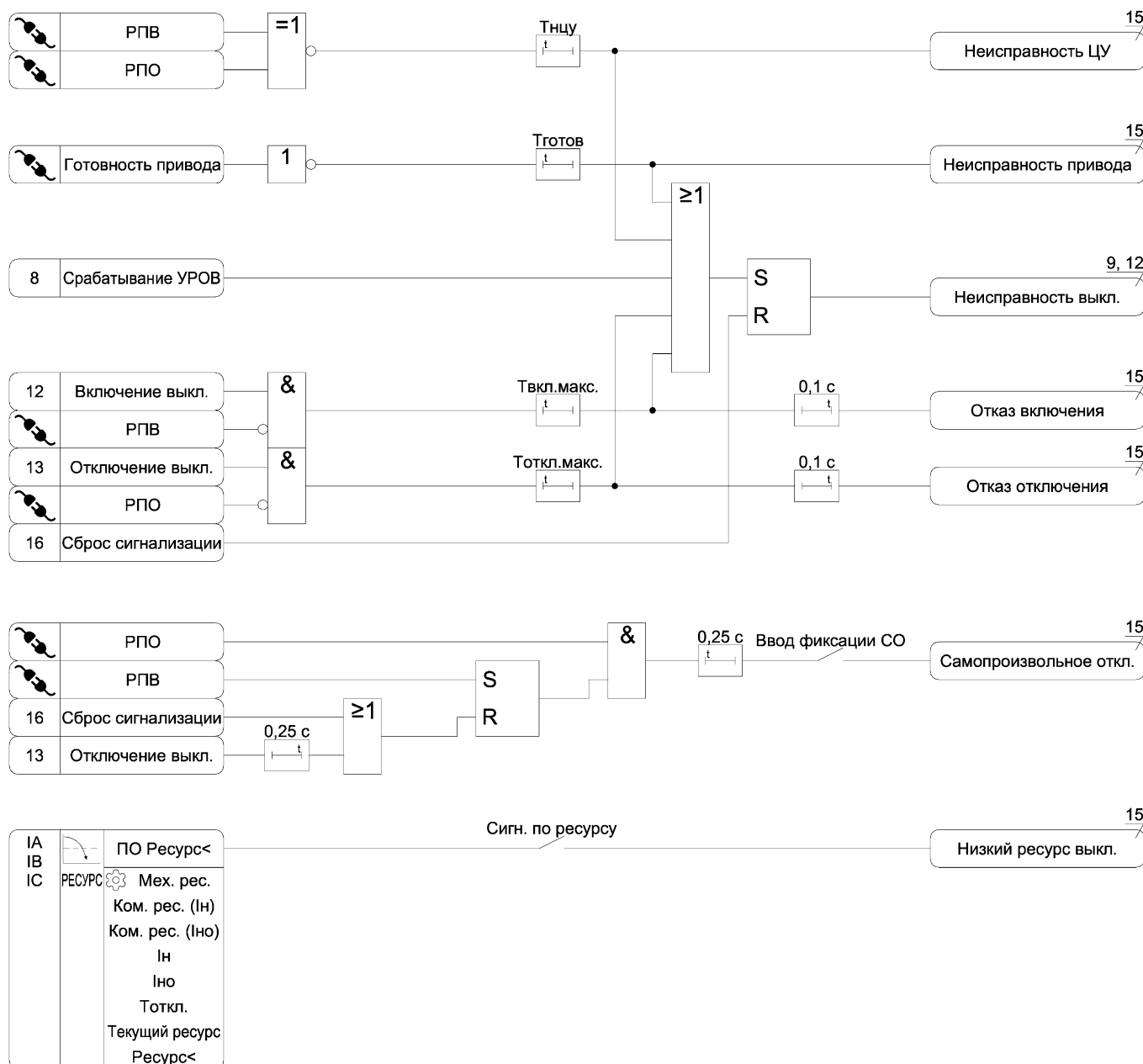
Рисунок А.14 – Функциональная схема алгоритма диагностики выключателя
