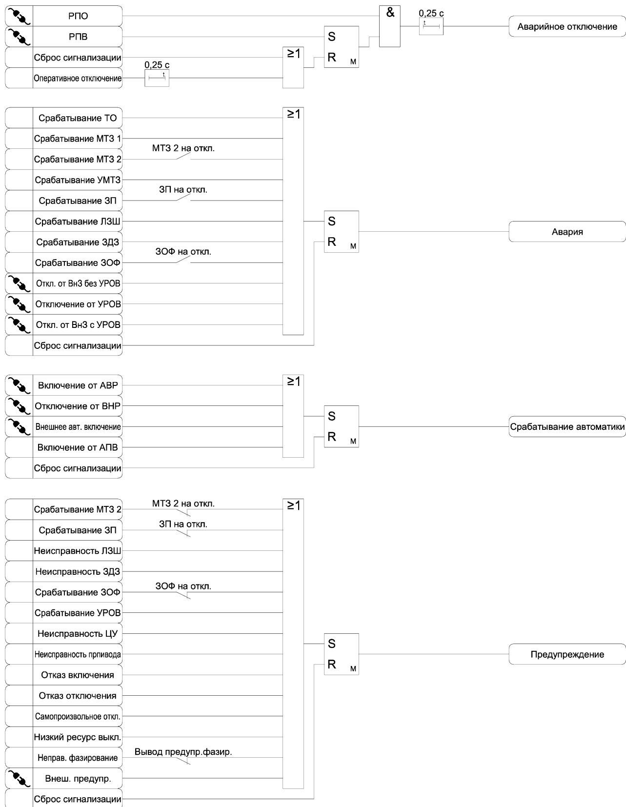
Рисунок 3.15 – Функциональная схема алгоритма сигнализации
