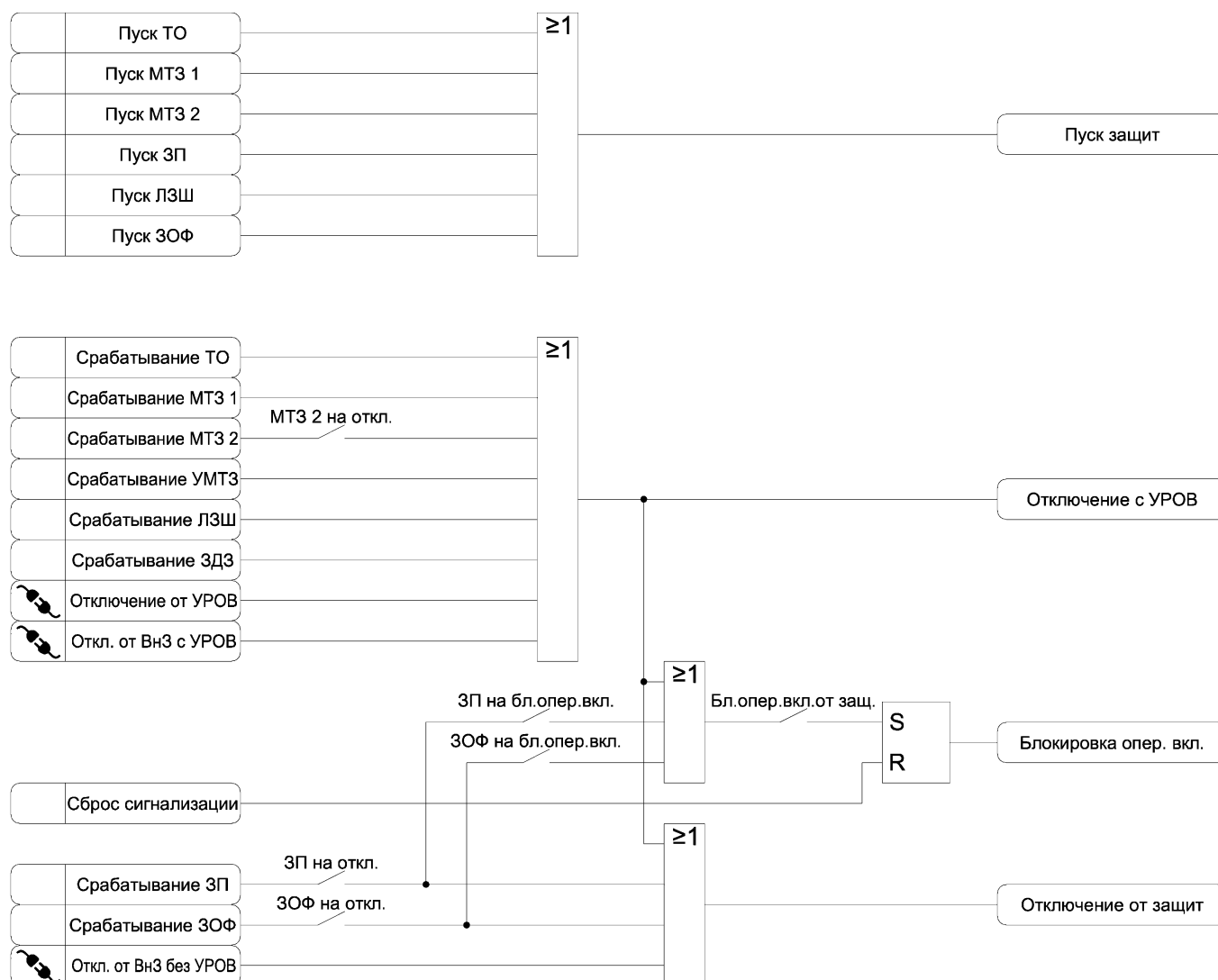
Рисунок 3.12 – Функциональная схема алгоритма формирования сигналов состояния защит
