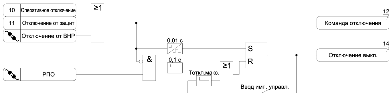
Рисунок А.13 – Функциональная схема алгоритма отключения выключателя
