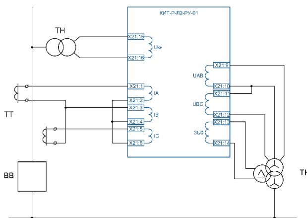
б) схема на ВВ с двумя ТТ
