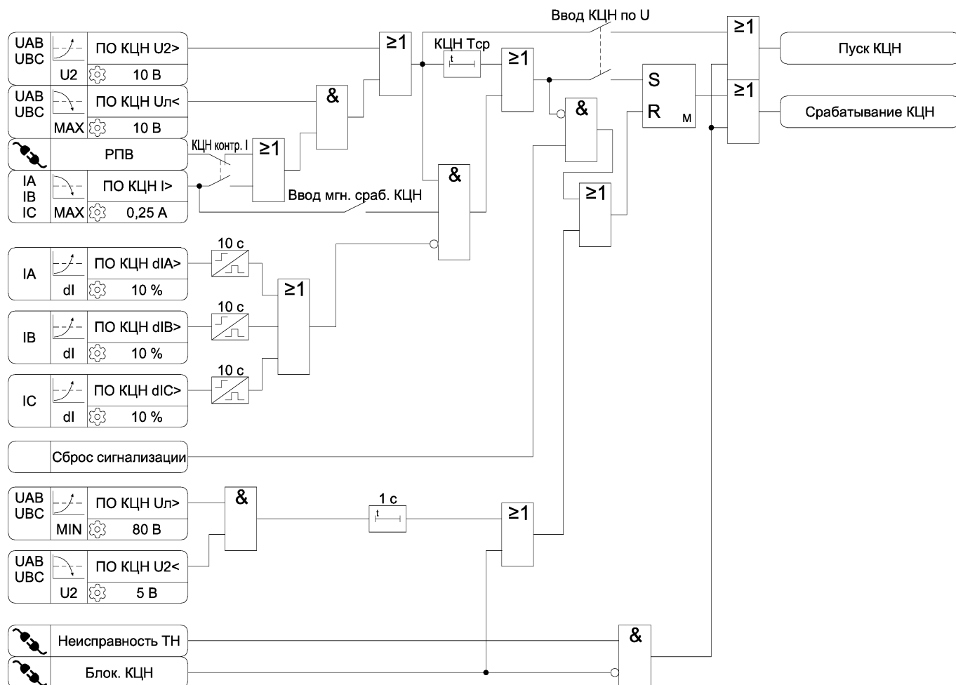
Рисунок 3.45 – Функциональная схема алгоритма КЦН
