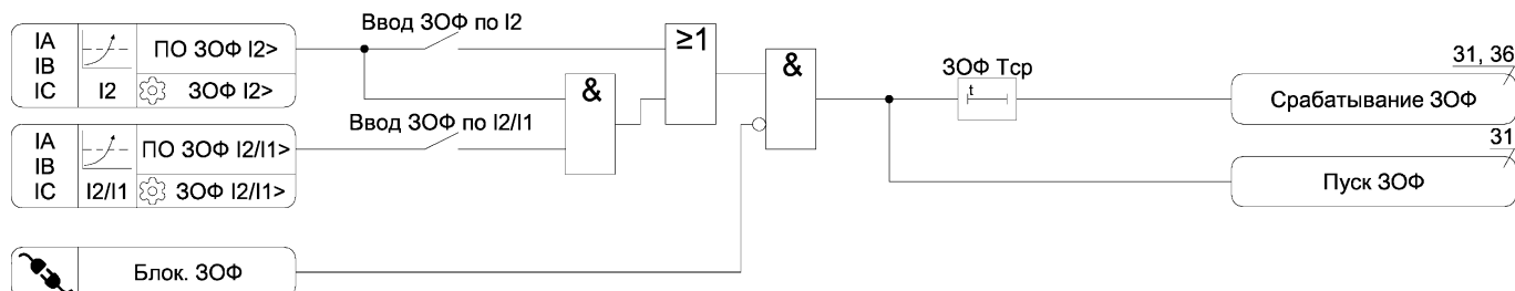
Рисунок А.15 – Функциональная схема алгоритма 30Ф
