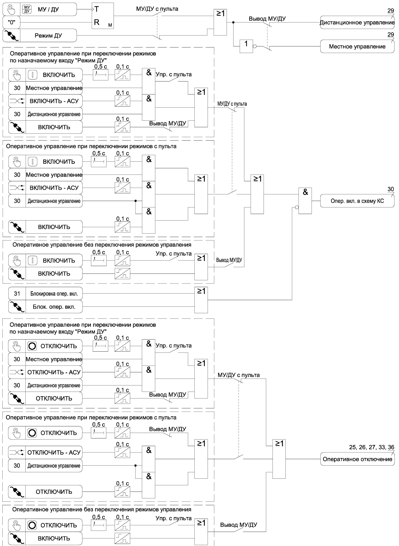
Рисунок А.29 а) – Функциональная схема алгоритма оперативного управления выключателем
