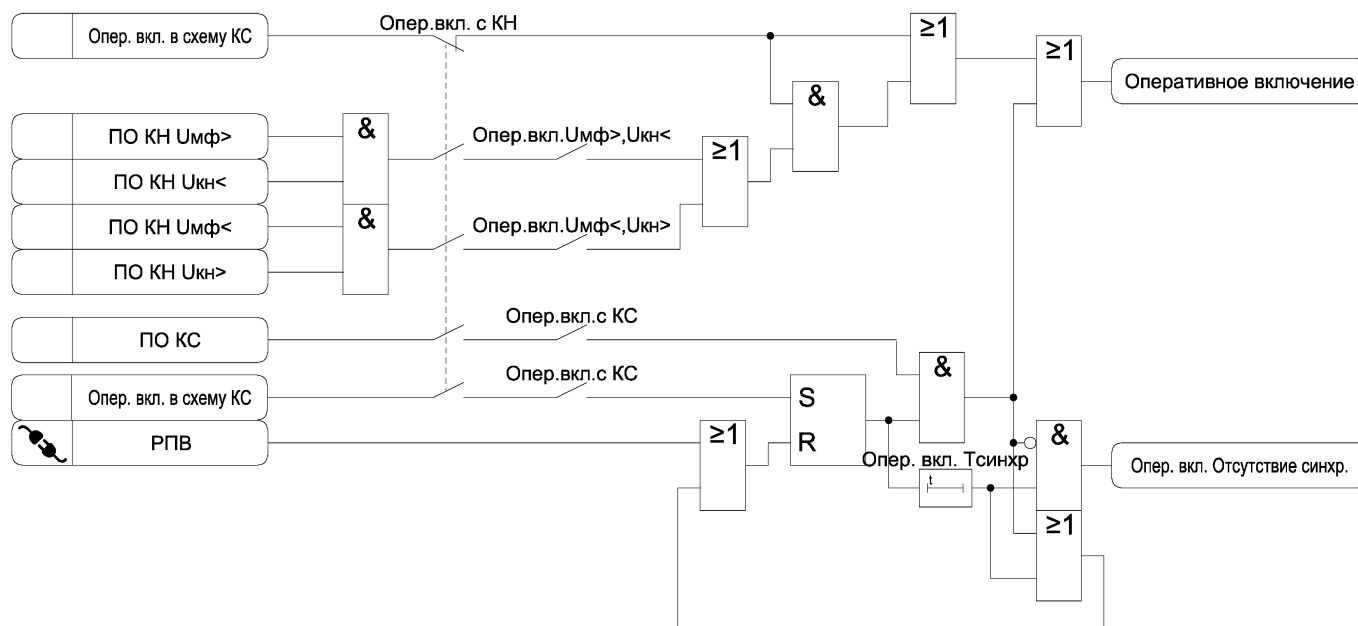
Рисунок 3.39 б) – Функциональная схема алгоритма оперативного управления выключателем
