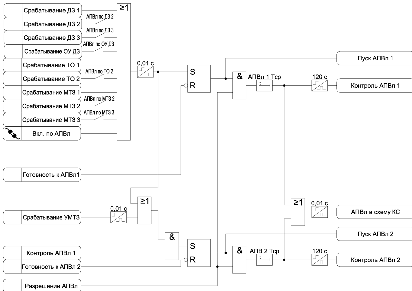
Рисунок 3.34 а) – Функциональная схема алгоритма АПВ
