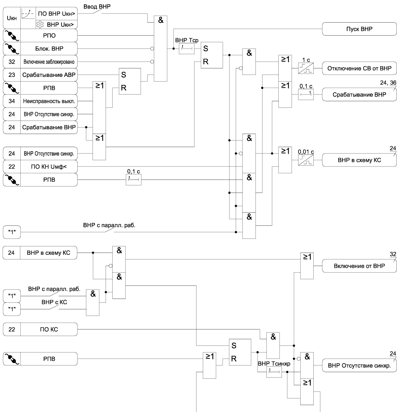
Рисунок А.24 – Функциональная схема алгоритма ВНР
