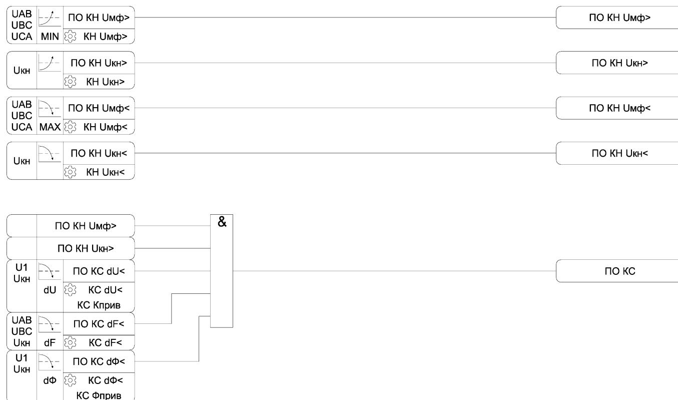
Рисунок 3.29 – Функциональная схема алгоритма КН
