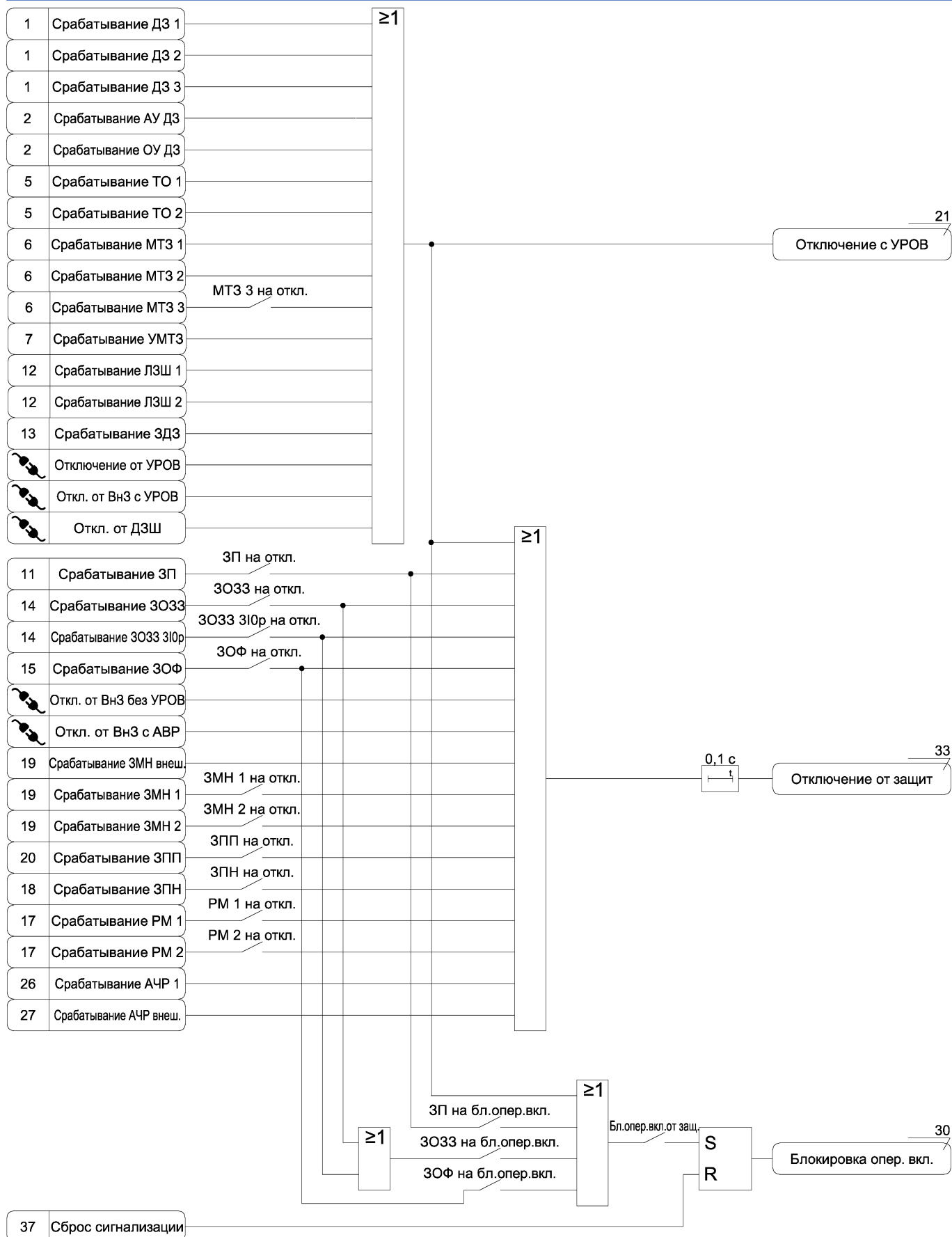
Рисунок А.31 б) – Функциональная схема алгоритма состояния защит
