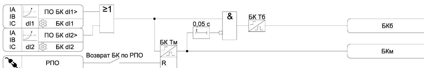
Рисунок 3.6 – Функциональная схема алгоритма БК
