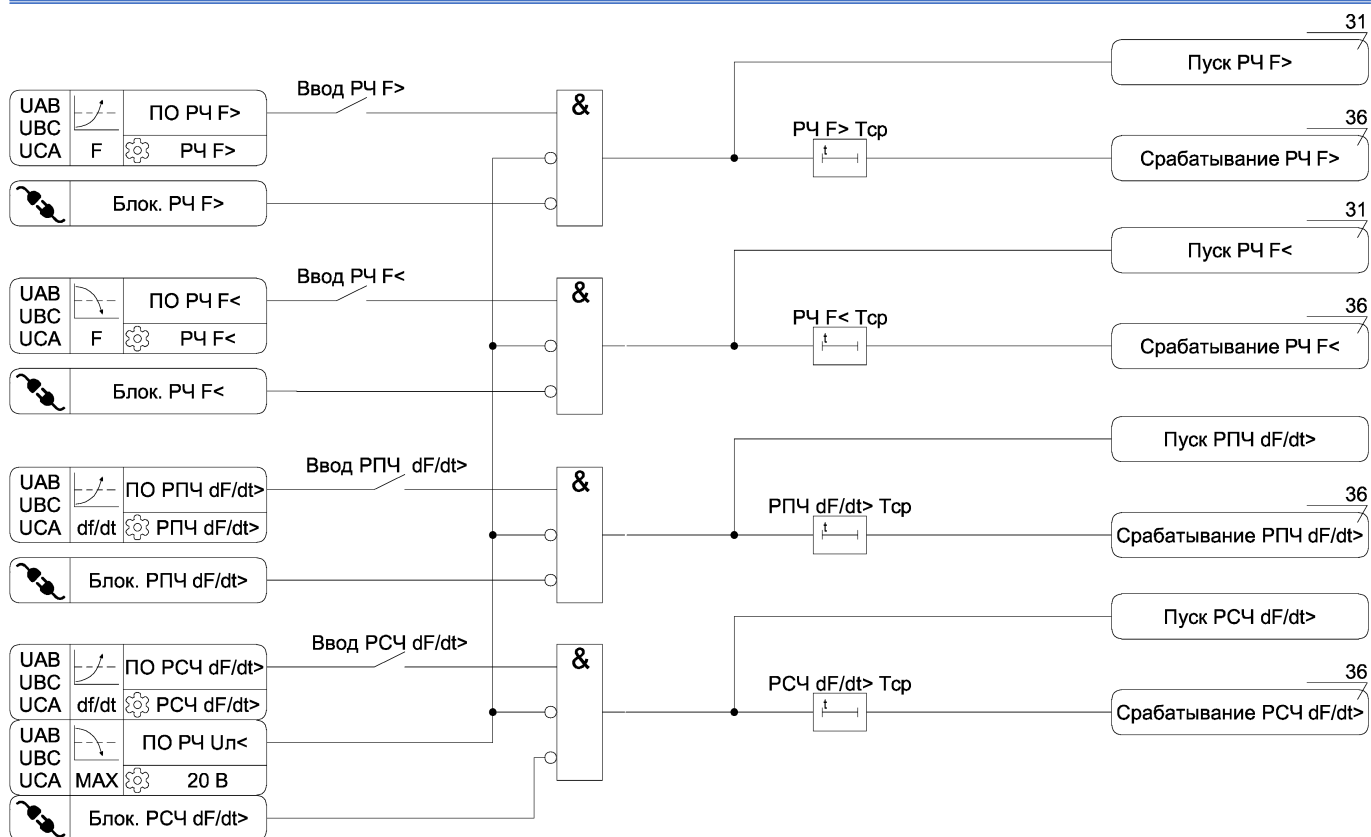
Рисунок А.28 – Функциональная схема алгоритма защиты от повышения и снижения частоты
