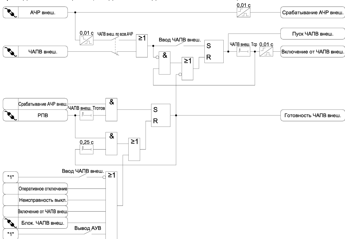
Рисунок 3.36 – Функциональные схемы алгоритмов АЧР и ЧАПВ от внешнего устройства
