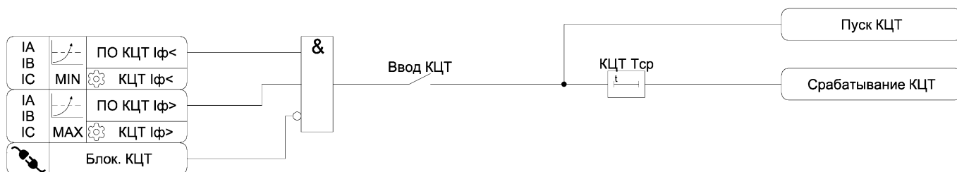
Рисунок 3.22 – Функциональная схема алгоритма КЦТ
