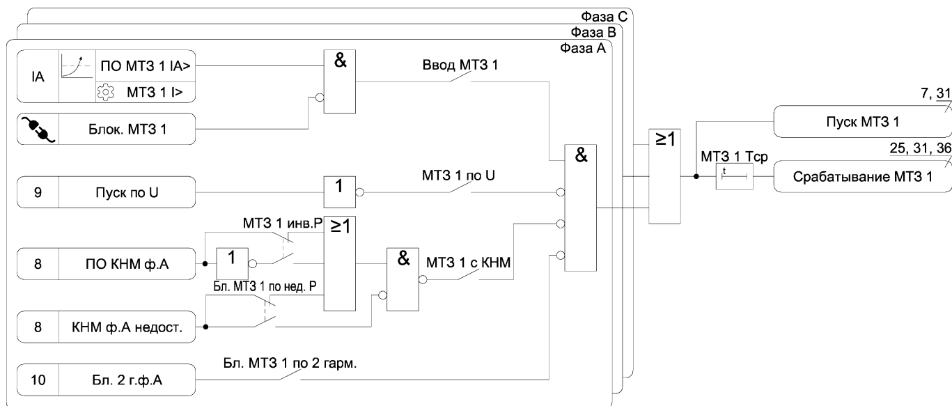
Рисунок А.6 а) – Функциональная схема алгоритма MT3
