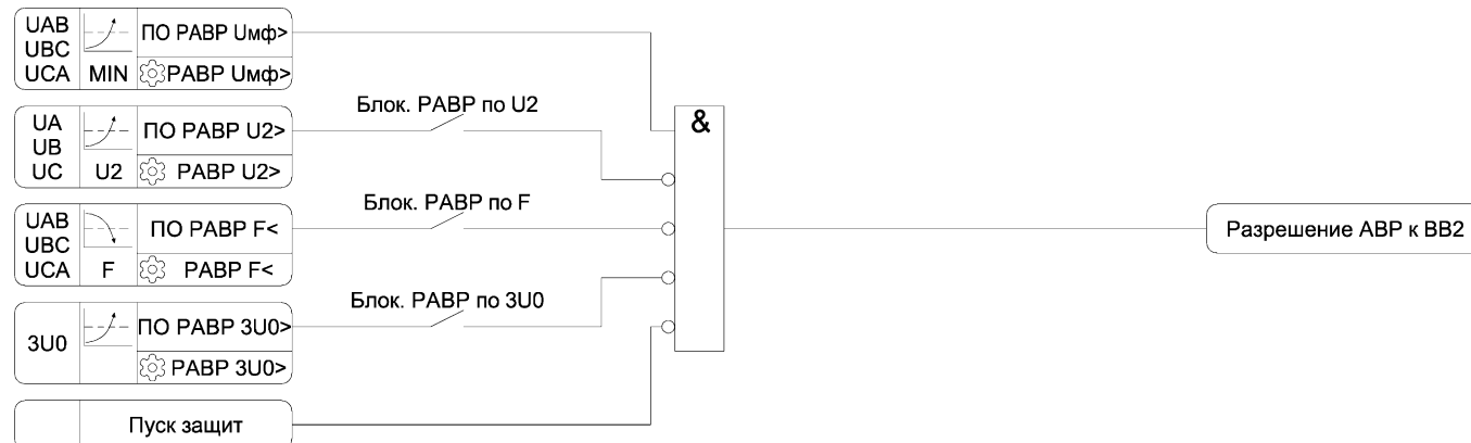
Рисунок 3.32 – Функциональная схема алгоритма РАВР
