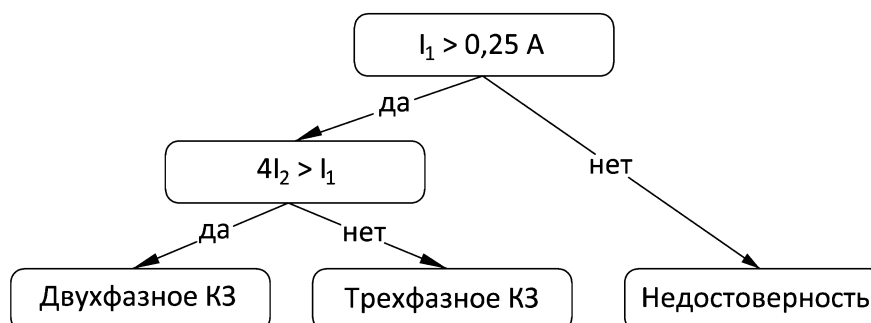
Рисунок 3.48 – Блок-схема определения вида короткого замыкания
