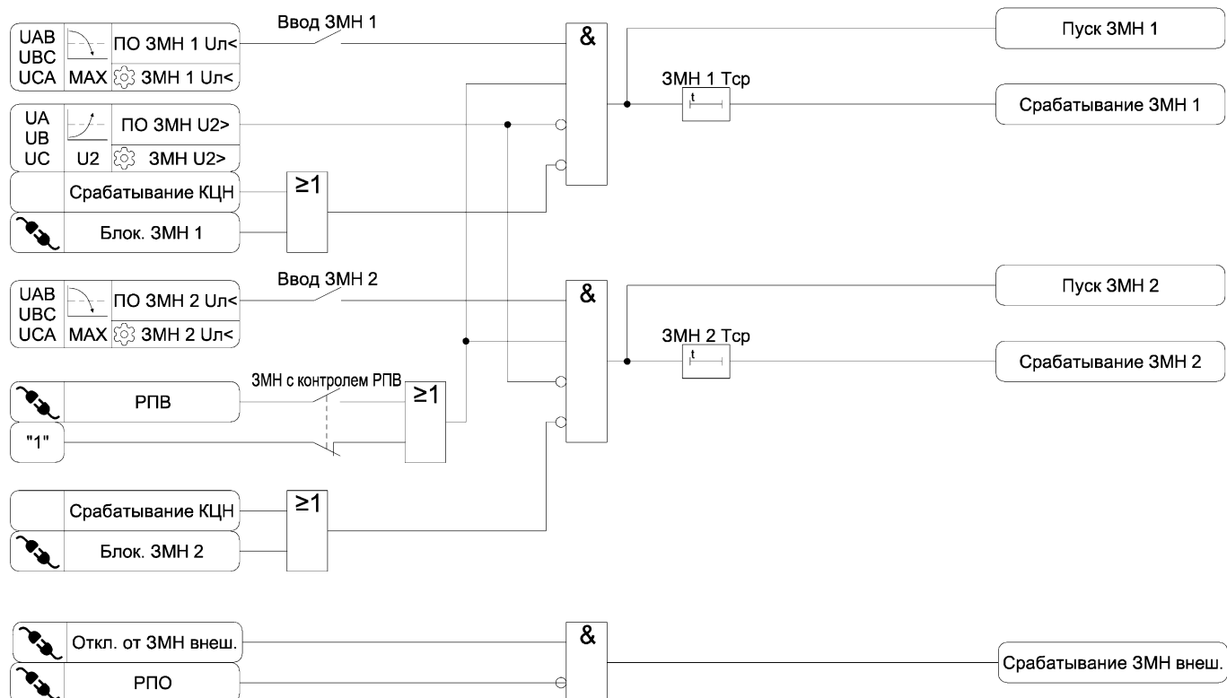
Рисунок 3.26 – Функциональная схема алгоритма ЗМН
