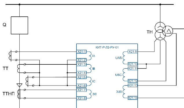
д) схема на отходящей линии с тремя ТТ
