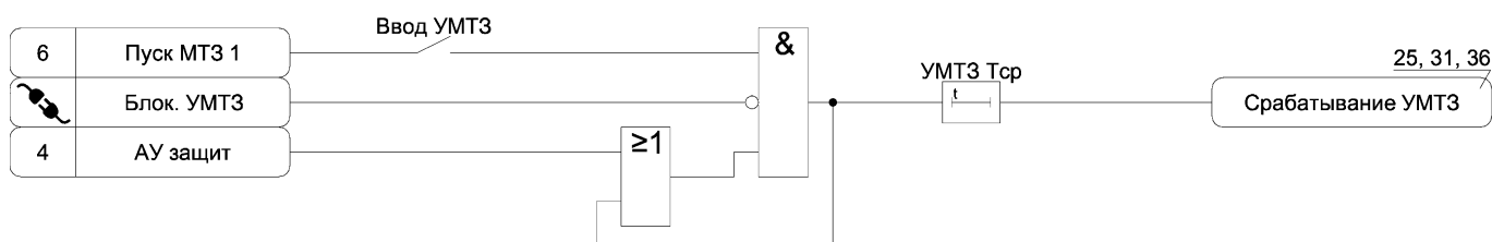
Рисунок А.7 – Функциональная схема алгоритма УМТЗ
