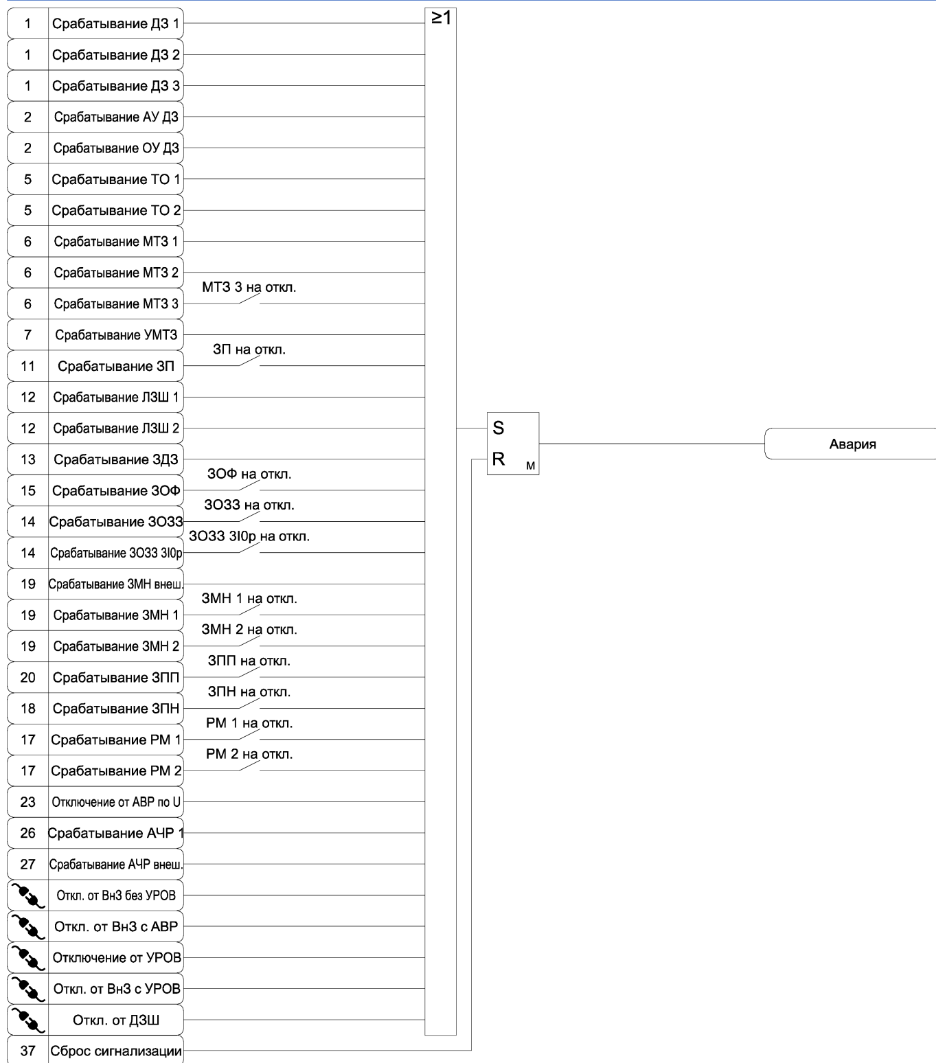
Рисунок А.36 б) – Функциональная схема алгоритма сигнализации
