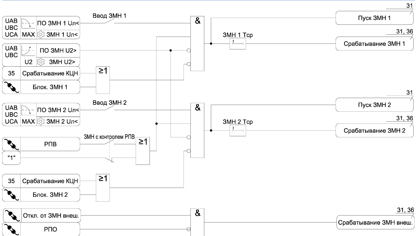
Рисунок А.19 – Функциональная схема алгоритма ЗМН
