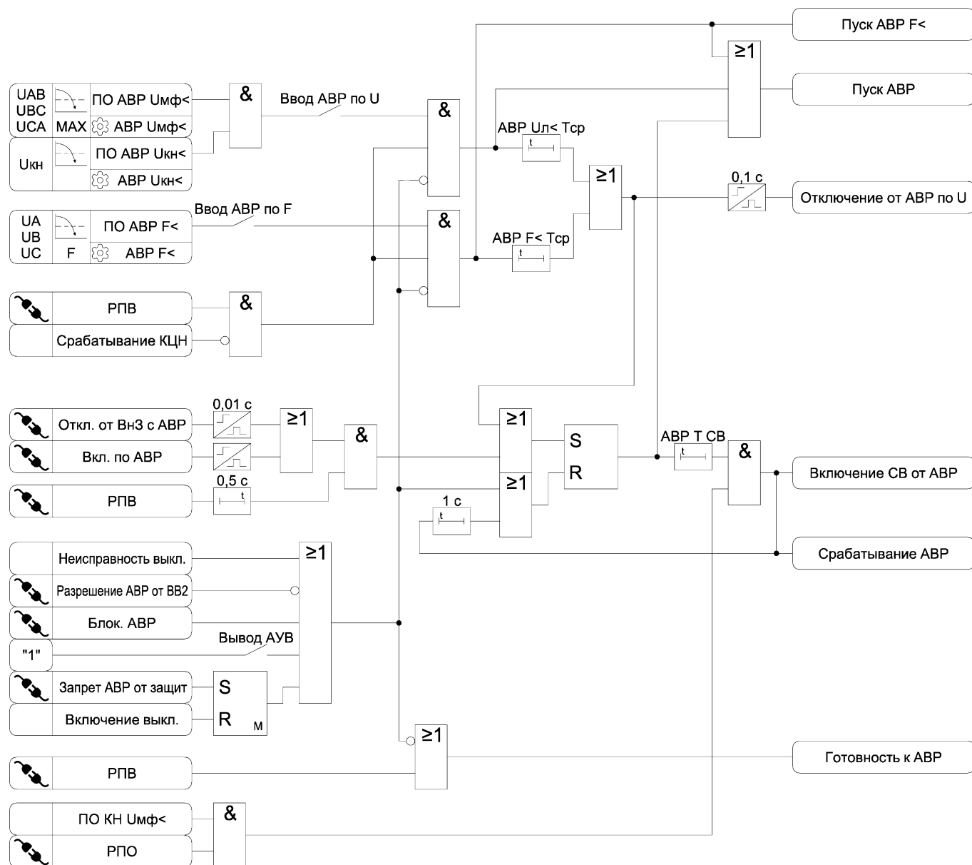
Рисунок 3.30 – Функциональная схема алгоритма АВР
