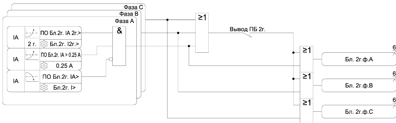
Рисунок А.10 – Функциональная схема алгоритма блокировки по второй гармонике
