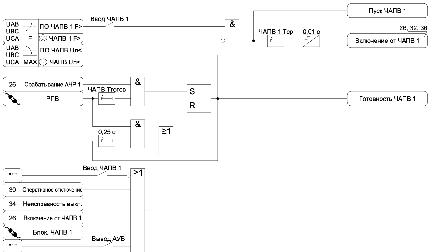
Рисунок А.26 б) – Функциональная схема алгоритма АЧР и ЧАПВ
