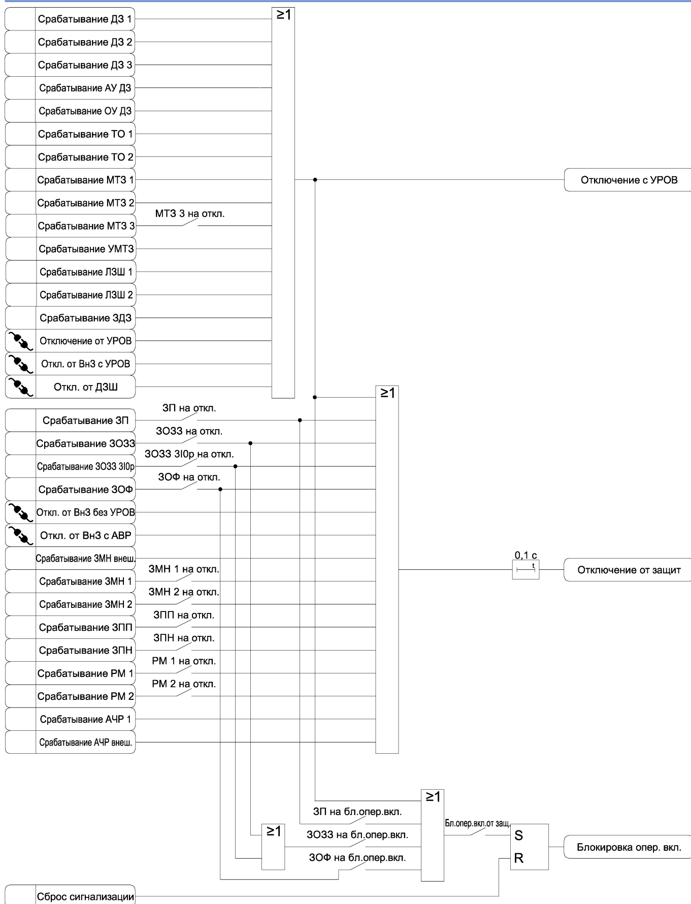
Рисунок 3.41 б) – Функциональная схема алгоритма формирования сигналов состояния защит
