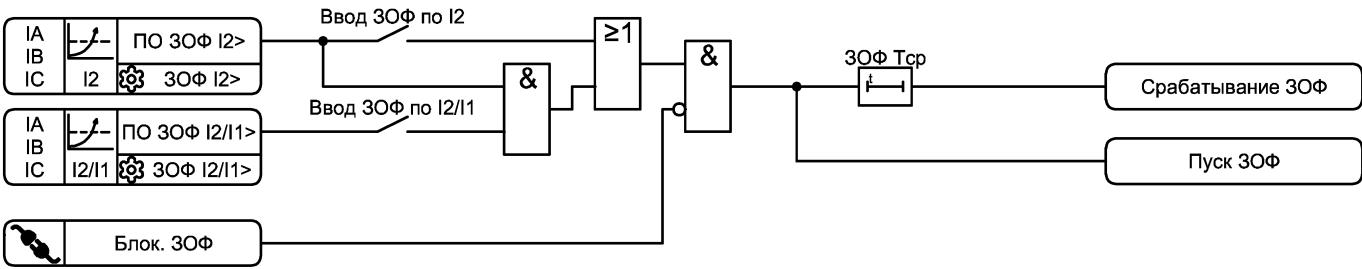
Рисунок 3.21 – Функциональная схема алгоритма ЗОФ
