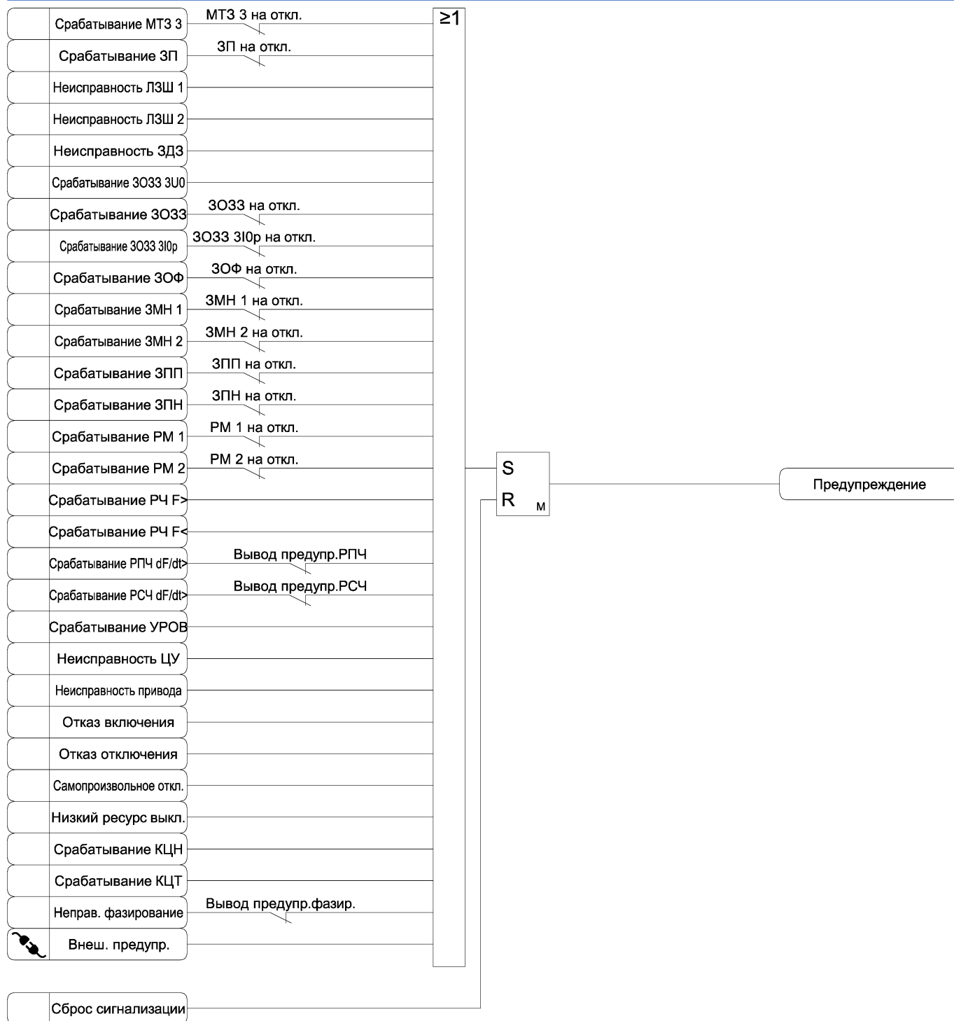
Рисунок 3.46 в) – Функциональная схема алгоритма сигнализации
