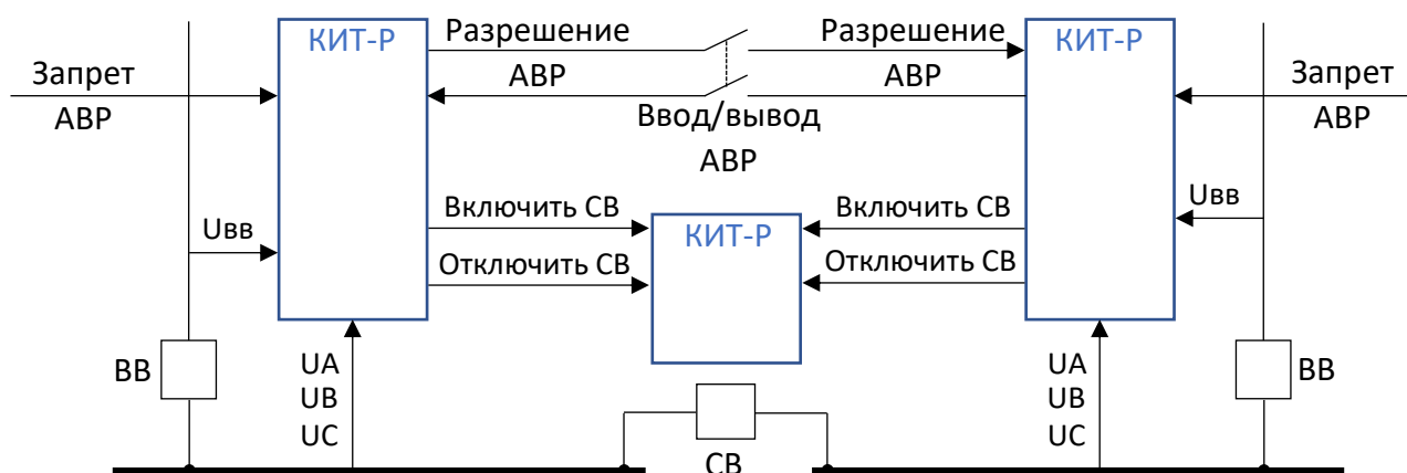
Рисунок 3.31 – Структурная схема АВР
