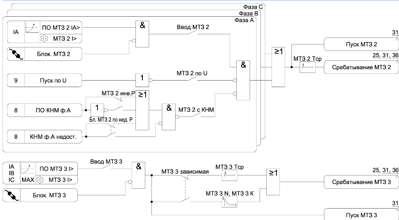
Рисунок А.6 б) – Функциональная схема алгоритма МТЗ
