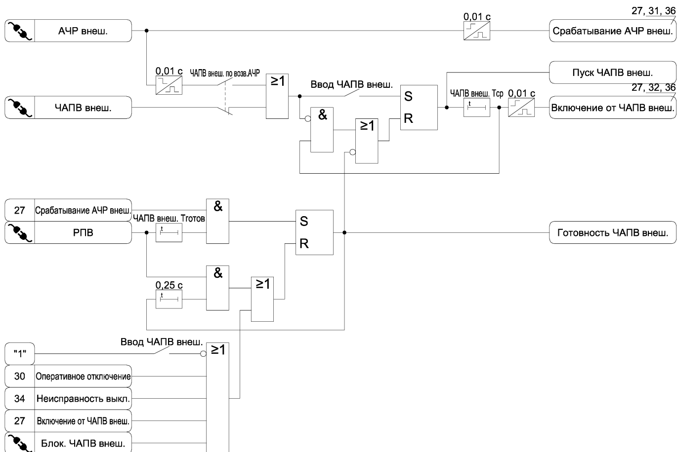
Рисунок А.27 – Функциональная схема алгоритма АЧР и ЧАПВ от внешнего устройства
