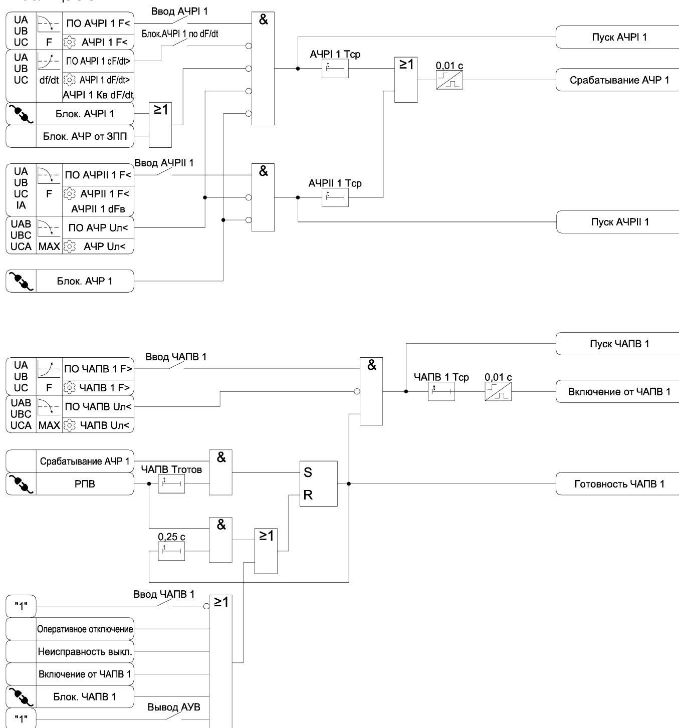
Рисунок 3.35 – Функциональные схемы алгоритмов АЧР и ЧАПВ
