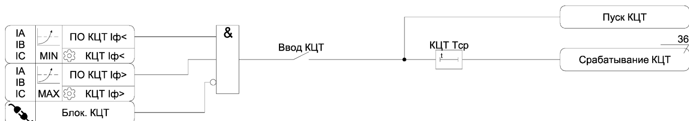
Рисунок А.16 – Функциональная схема алгоритма КЦТ
