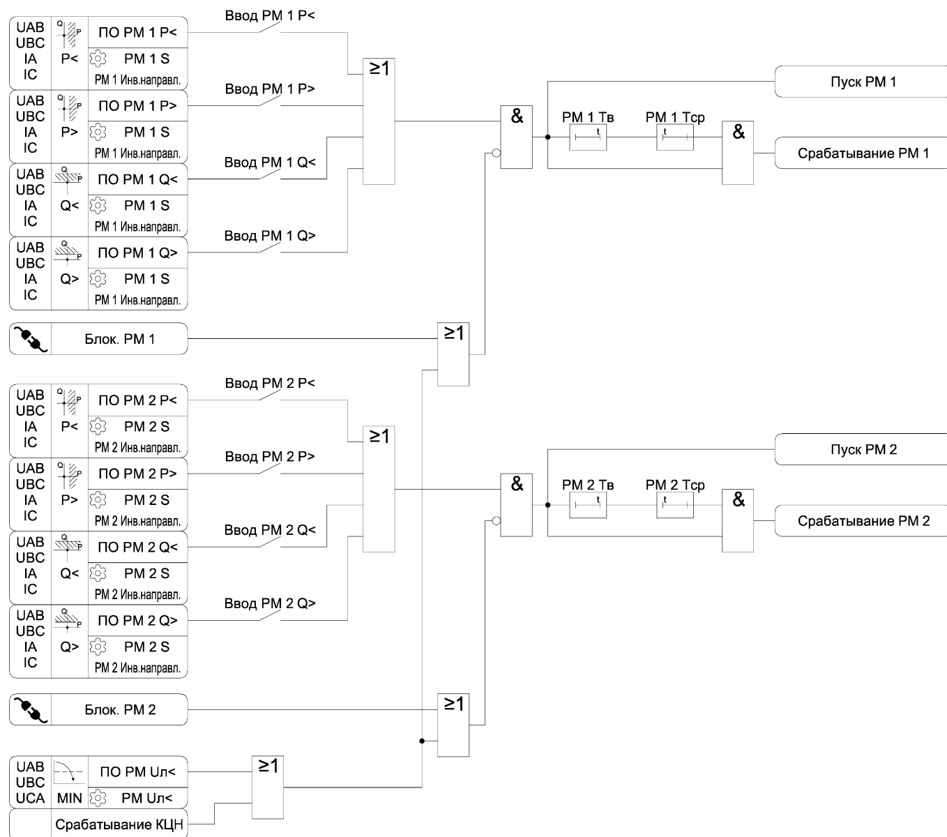
Рисунок 3.23 – Функциональная схема алгоритма защиты по направлению мощности
