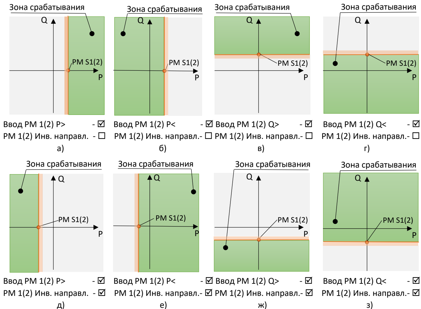
Рисунок 3.24 – Диаграмма срабатывания реле активного тока нулевой последовательности
