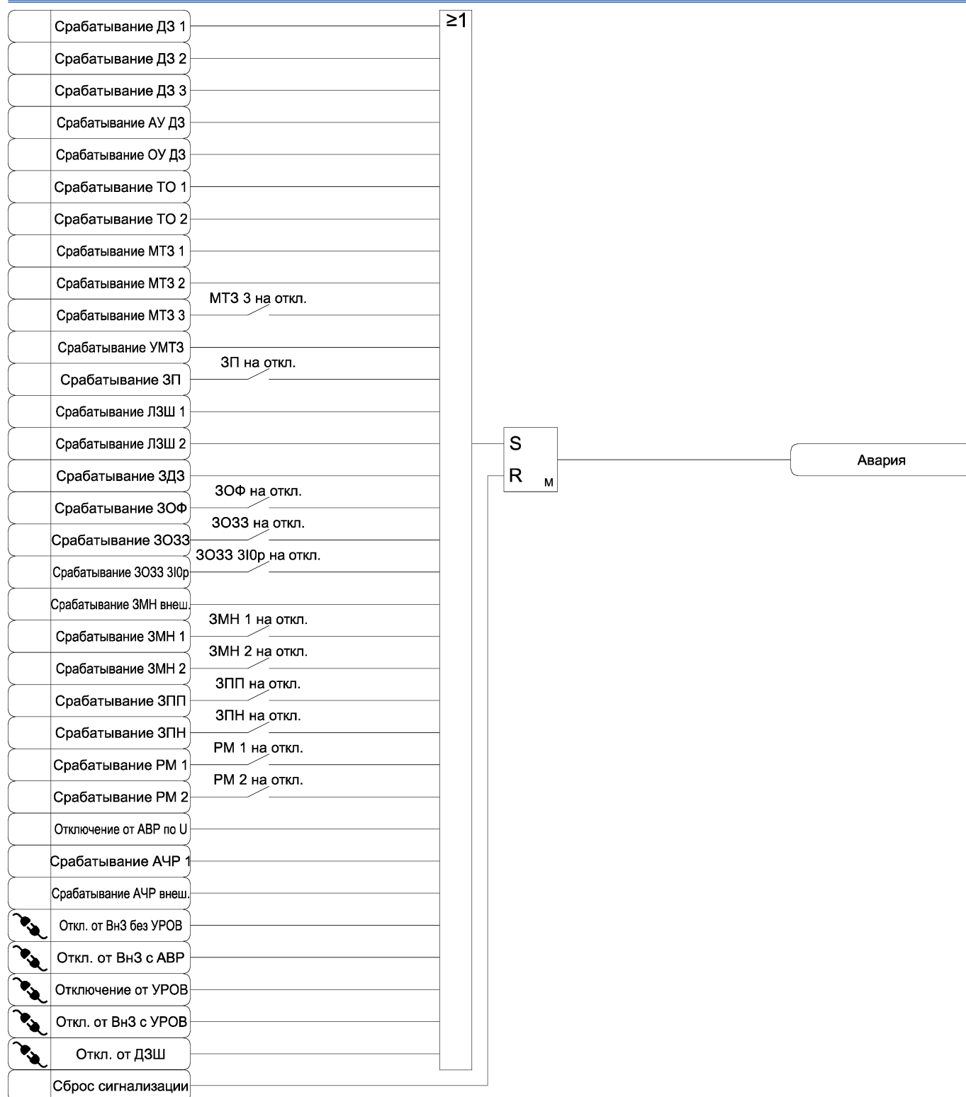
Рисунок 3.46 б) – Функциональная схема алгоритма сигнализации
