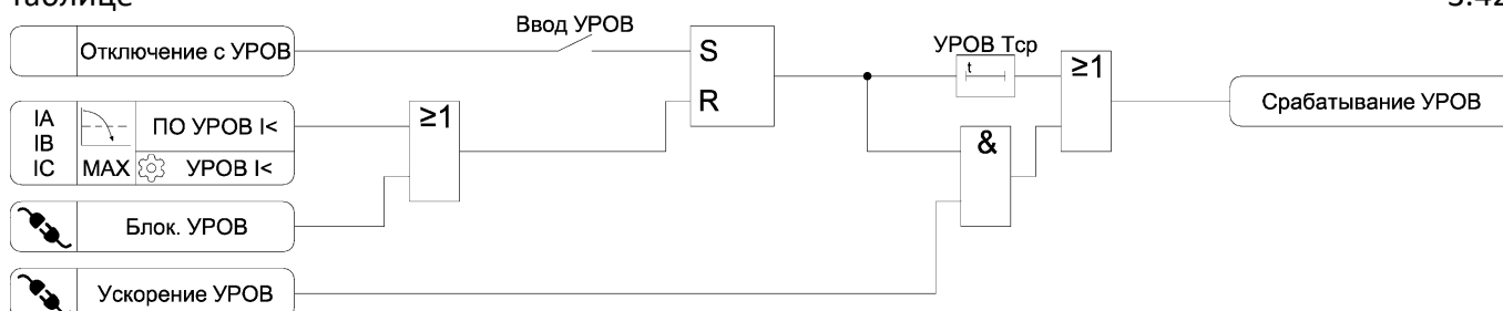
Рисунок 3.28 – Функциональная схема алгоритма УРОВ
