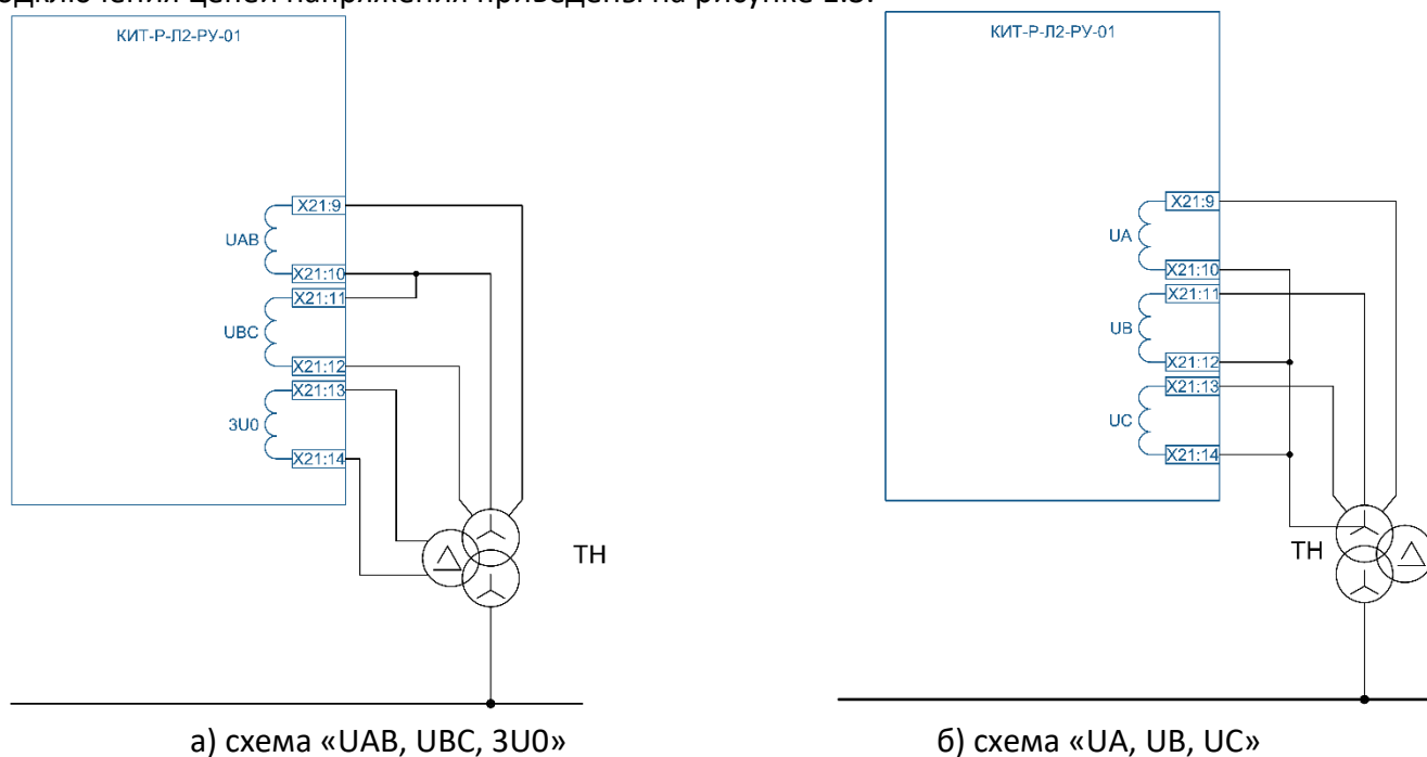
Рисунок 1.3 – Варианты подключения цепей напряжения
