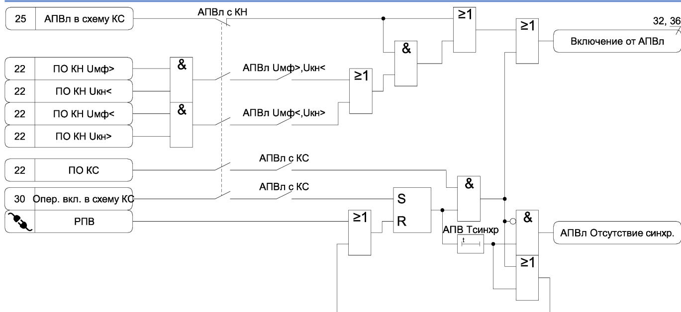
Рисунок А.25 б) – Функциональная схема алгоритма АПВ
