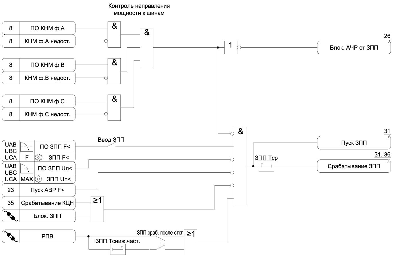
Рисунок А.20 – Функциональная схема алгоритма ЗПП
