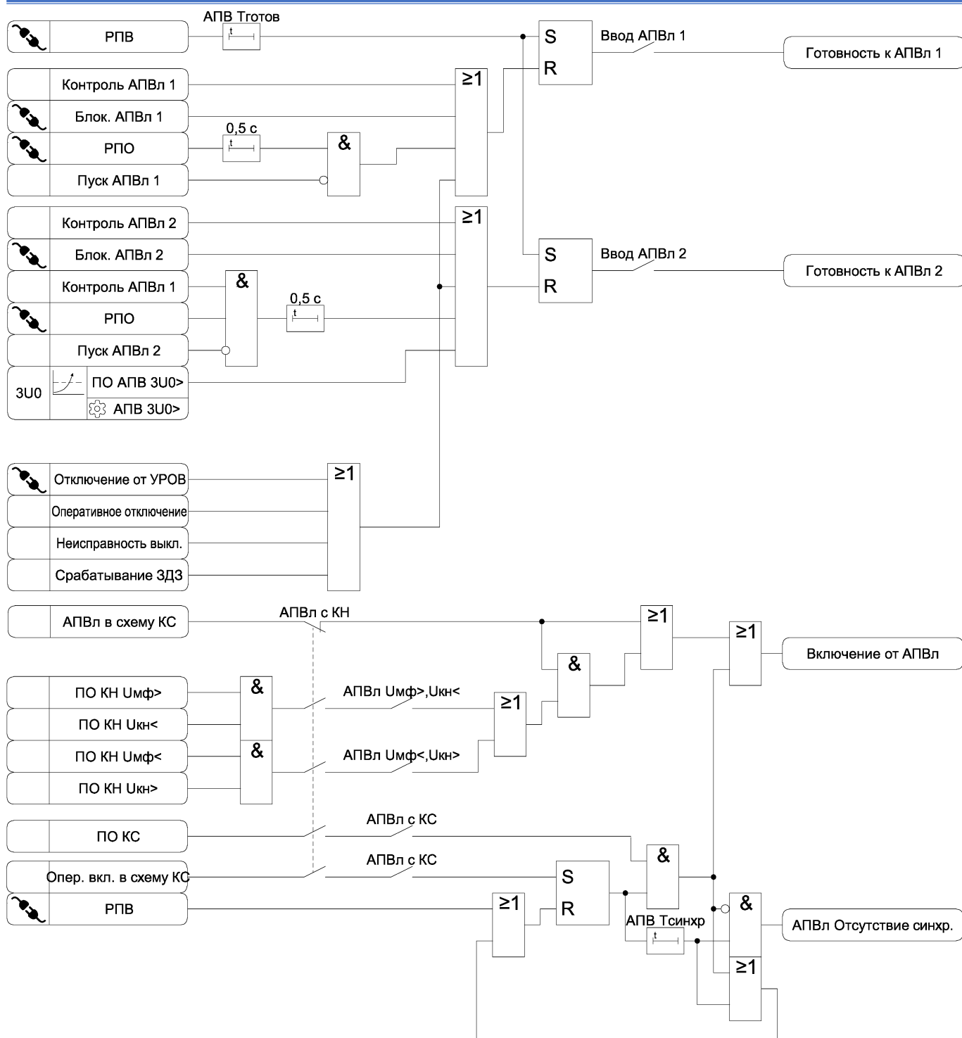
Рисунок 3.34 б) – Функциональная схема алгоритма АПВ
