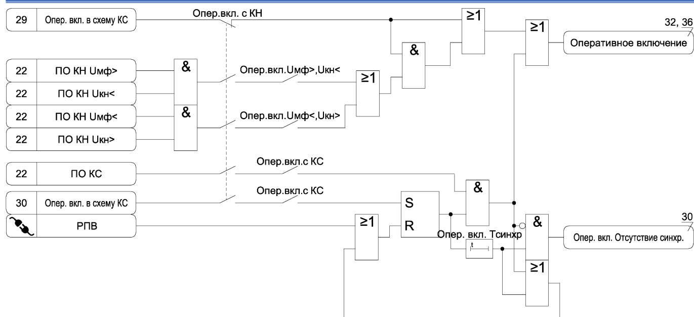
Рисунок А.30 б) – Функциональная схема алгоритма контроля синхронизма при оперативном включении
