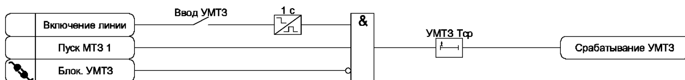
Рисунок 3.10 – Функциональная схема алгоритма УМТЗ
