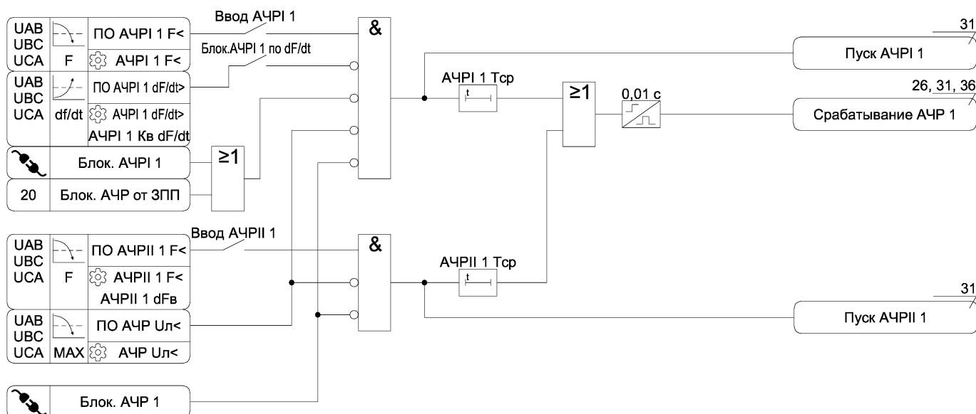
Рисунок А.26 а) – Функциональная схема алгоритма АЧР и ЧАПВ
