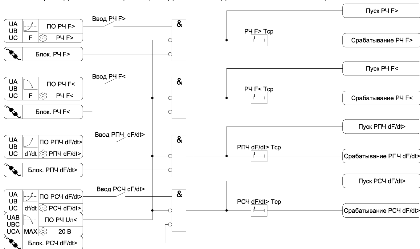
Рисунок 3.37 – Функциональные схемы алгоритмов защиты повышения и снижения частоты
