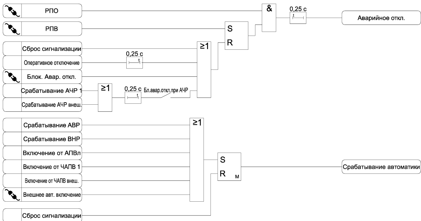
Рисунок 3.46 а) – Функциональная схема алгоритма сигнализации
