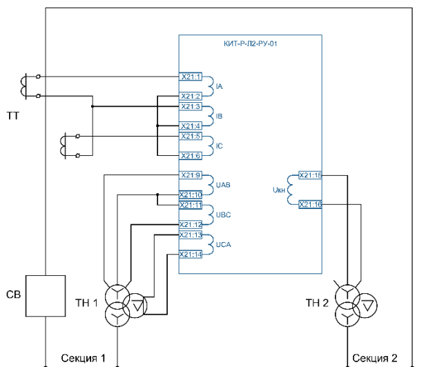
г) схема на СВ с двумя ТТ
