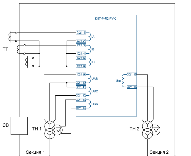
в) схема на СВ с тремя ТТ
