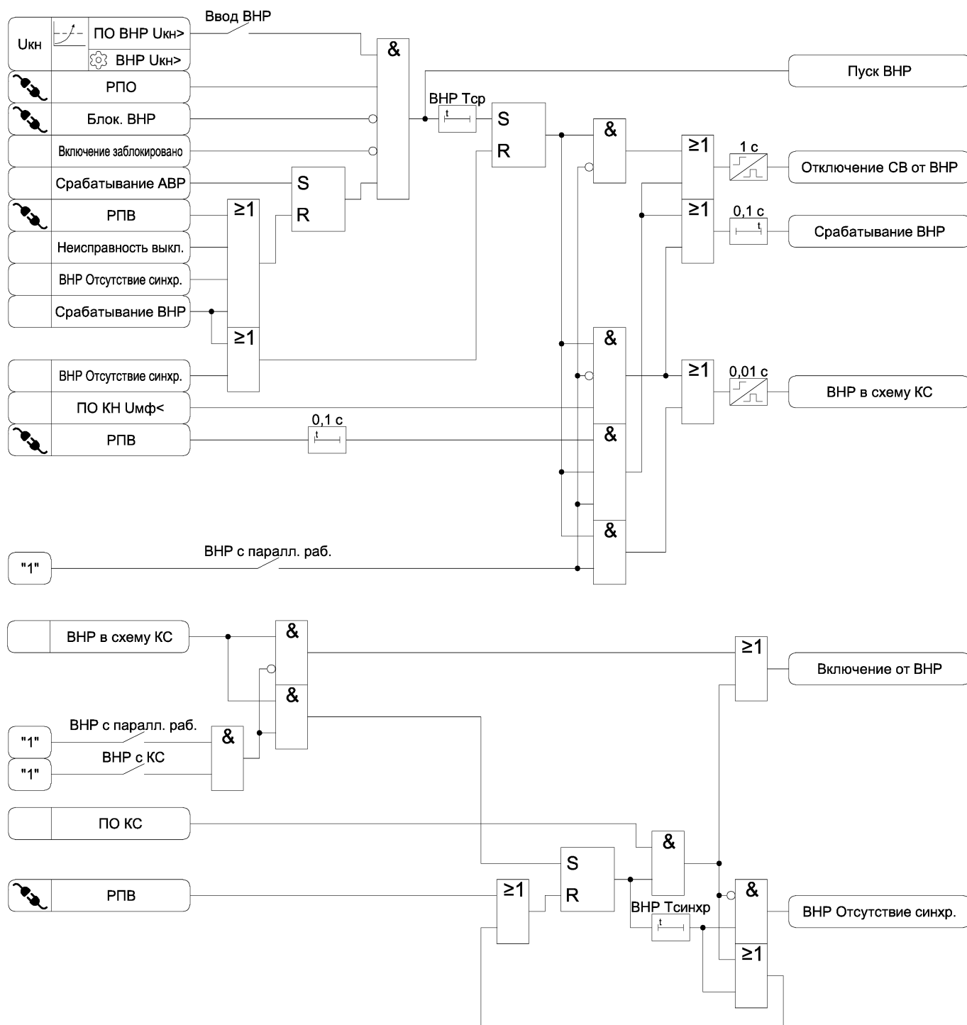
Рисунок 3.33 – Функциональная схема алгоритма ВНР
