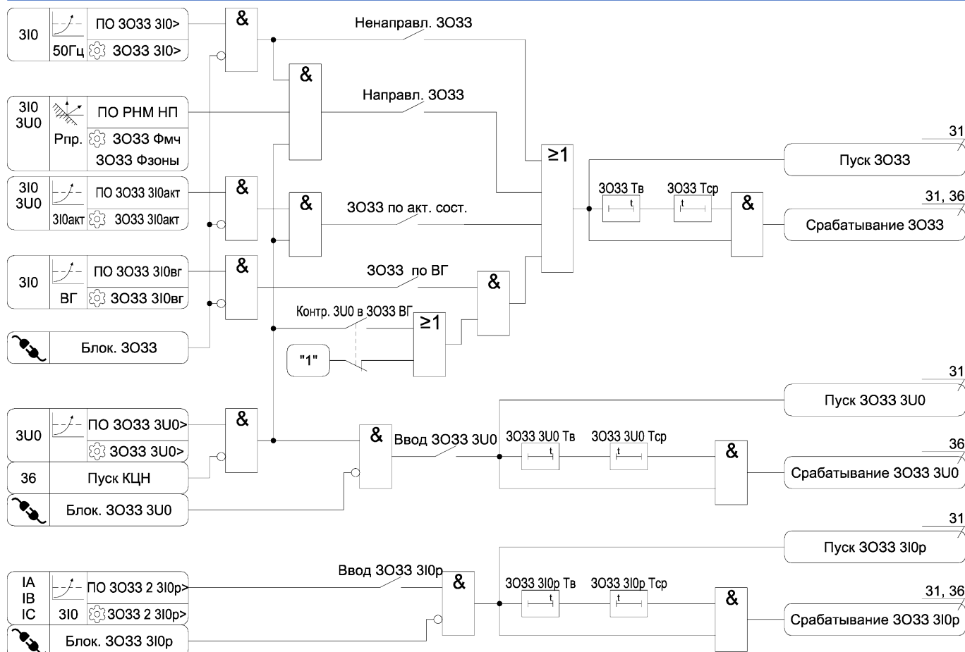
Рисунок А.14 – Функциональная схема алгоритма 3033
