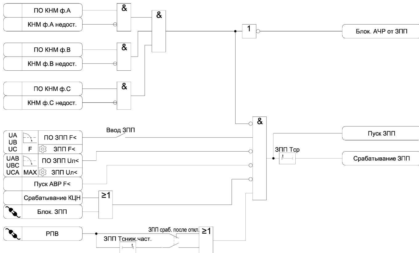
Рисунок 3.27 – Функциональная схема алгоритма ЗПП
