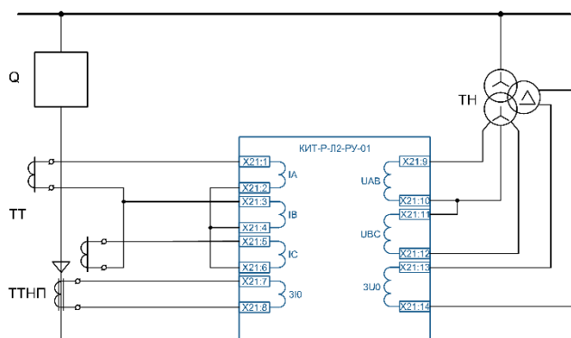
е) схема на отходящей линии с двумя ТТ
