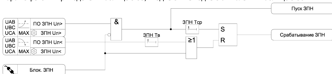
Рисунок 3.25 – Функциональная схема алгоритма ЗПН
