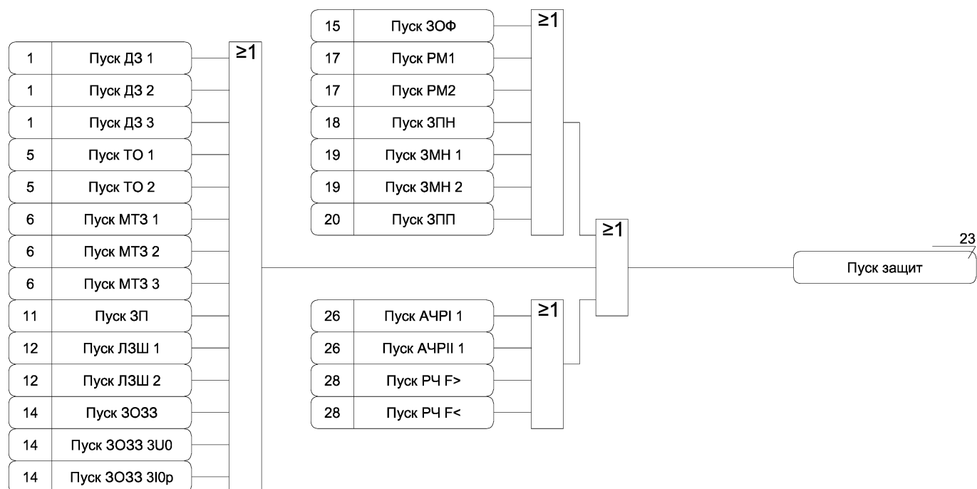
Рисунок А.31 а) – Функциональная схема алгоритма состояния защит
