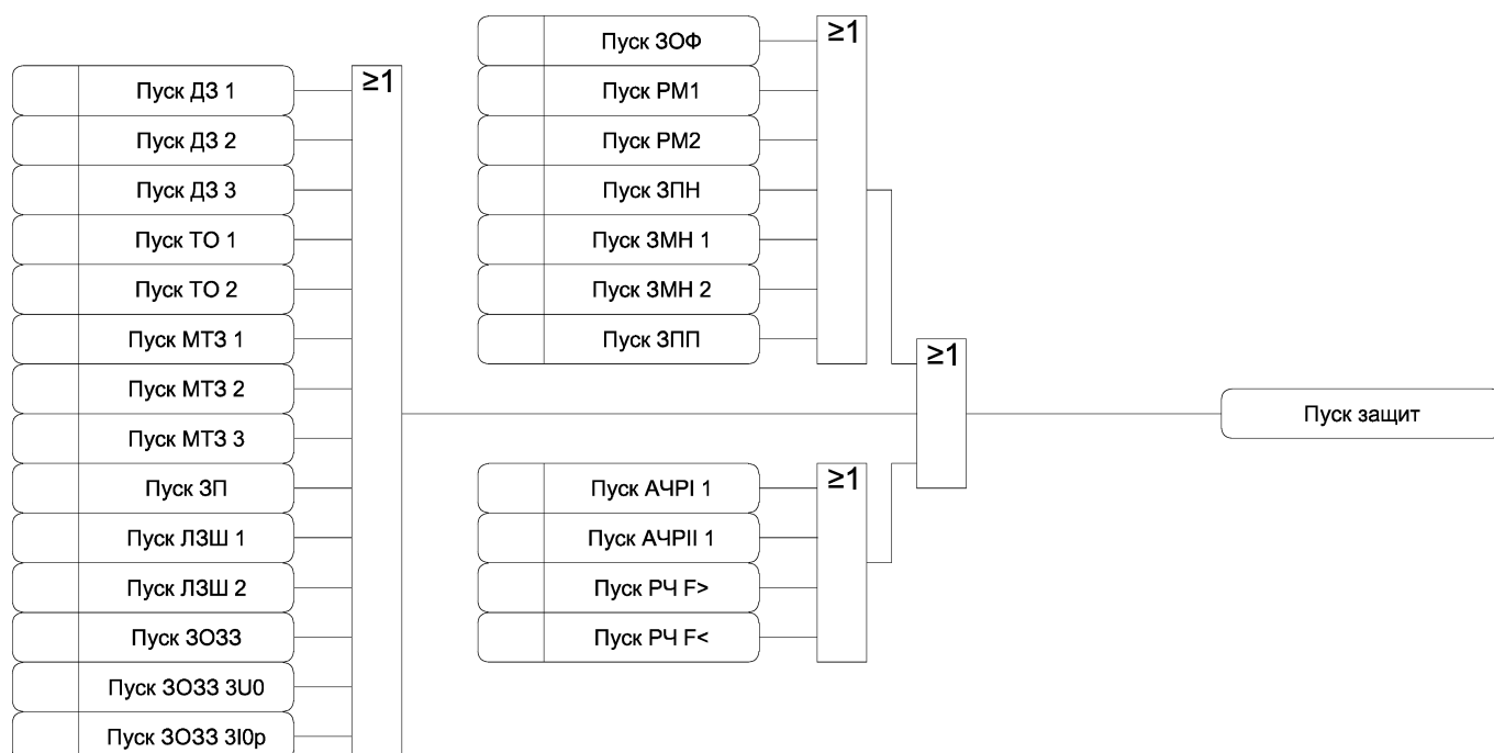
Рисунок 3.41 а) – Функциональная схема алгоритма формирования сигналов состояния защит
