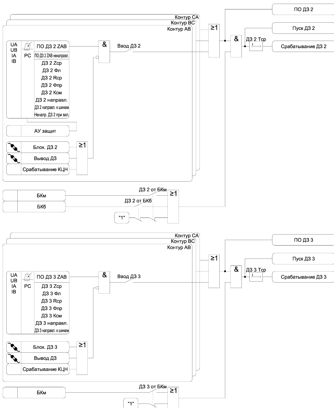
Рисунок 3.1 б) – Функциональная схема алгоритма ДЗ
