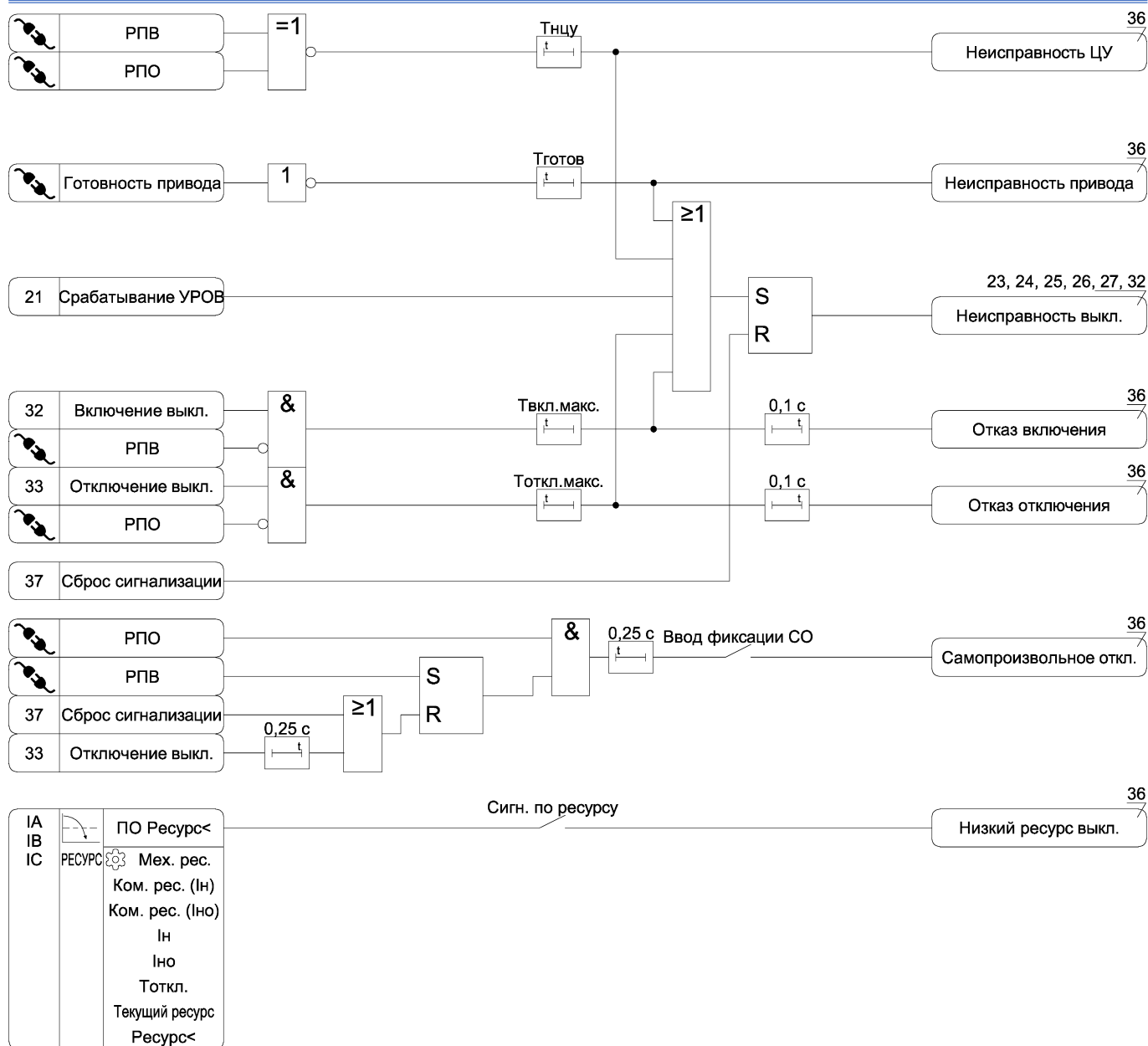
Рисунок А.34 – Функциональная схема алгоритма диагностики выключателя
