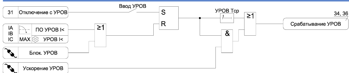
Рисунок А.21 – Функциональная схема алгоритма УРОВ
