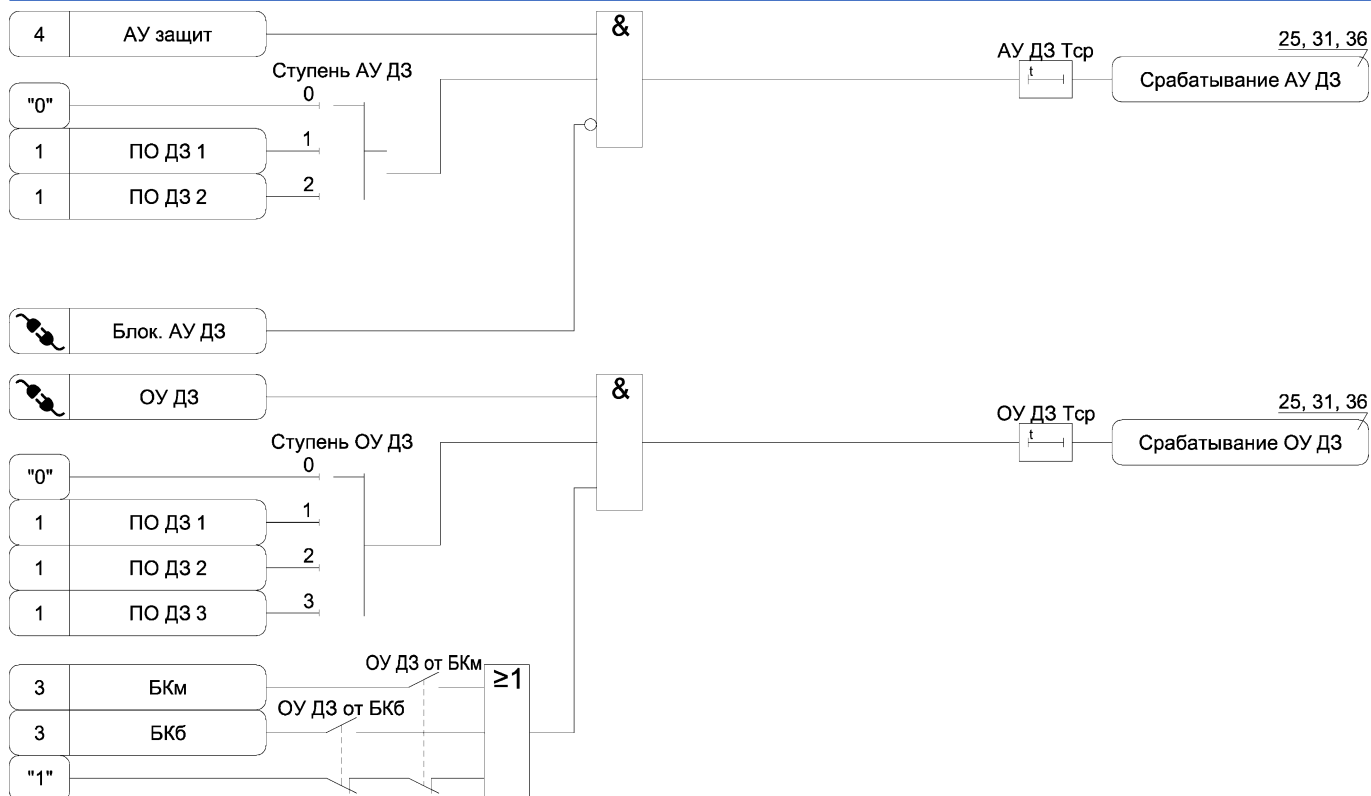
Рисунок А.2 – Функциональная схема алгоритма ускорения ДЗ
