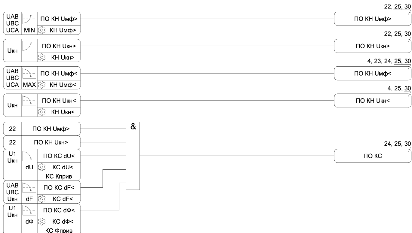
Рисунок А.22 – Функциональная схема алгоритма КН и КС
