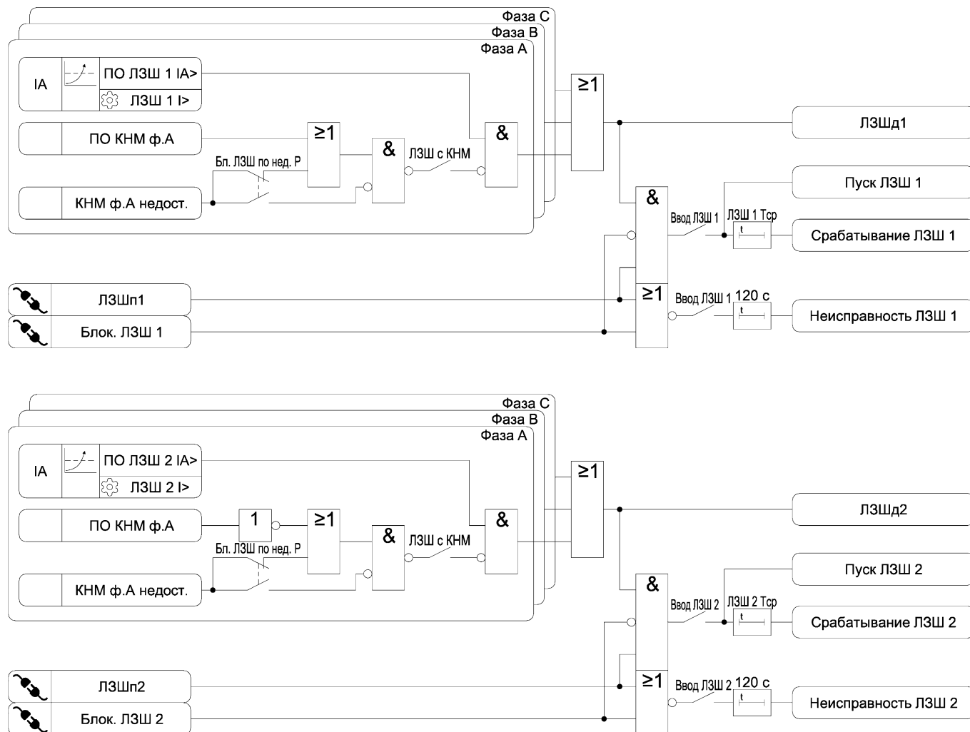
Рисунок 3.16 – Функциональная схема алгоритма ЛЗШ
