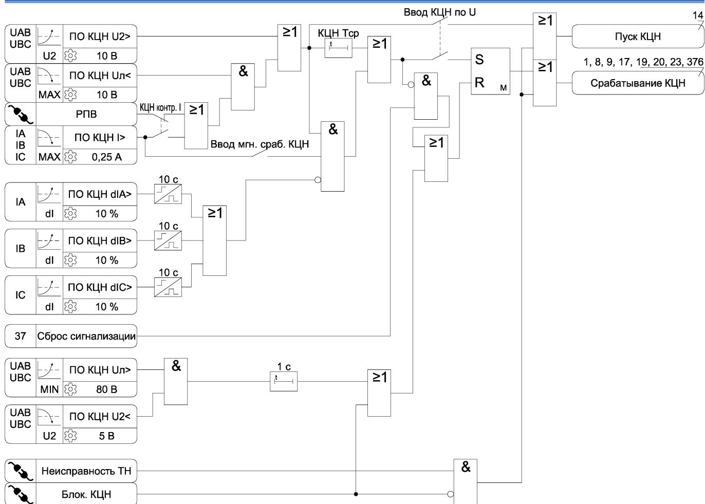
Рисунок А.35 – Функциональная схема алгоритма КЦН
