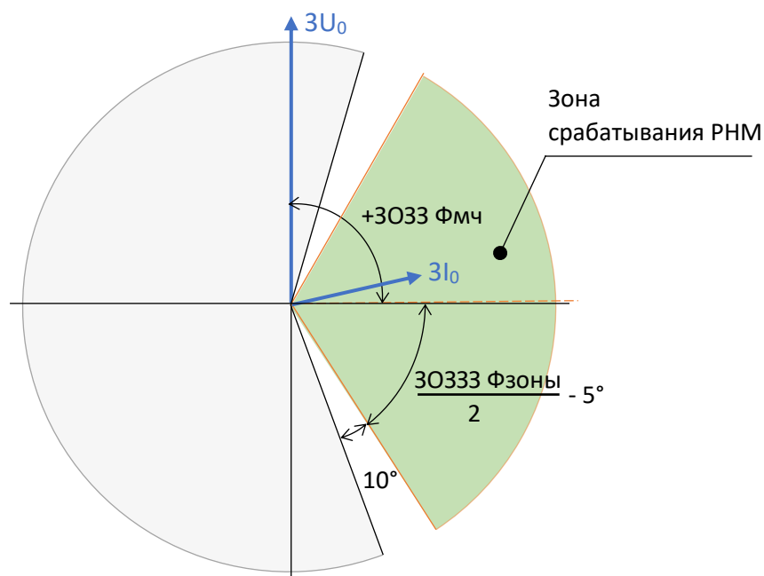
Рисунок 3.19 – Диаграмма срабатывания реле направления мощности нулевой последовательности
