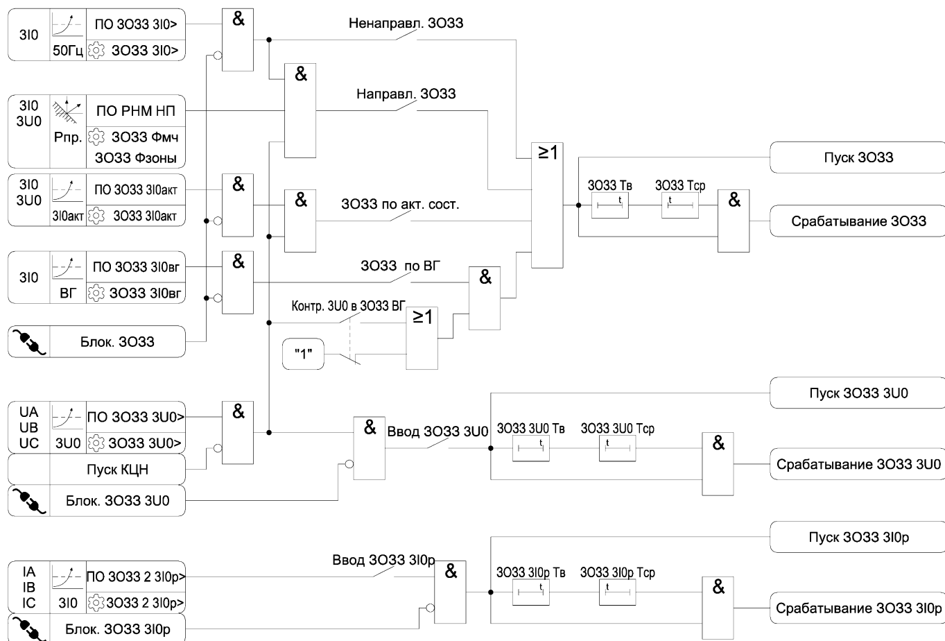
Рисунок 3.18 – Функциональная схема алгоритма ЗОЗЗ
