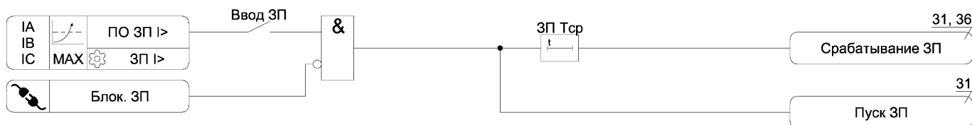
Рисунок А.11 – Функциональная схема алгоритма 3П
