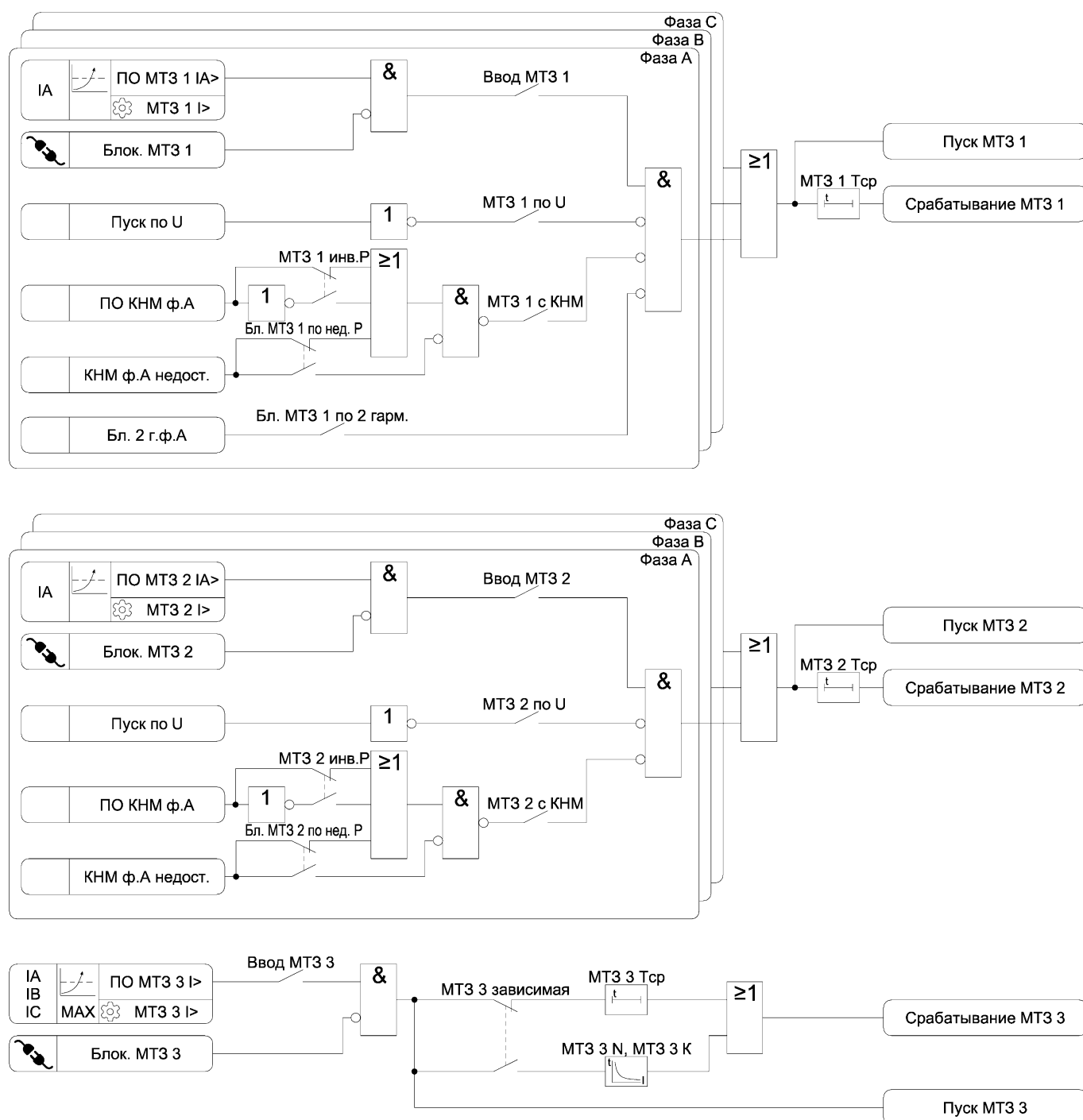
Рисунок 3.9 – Функциональная схема алгоритма МТЗ
