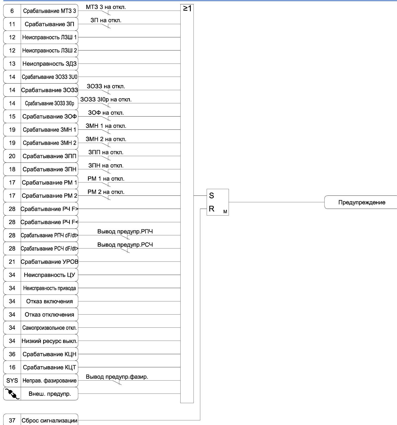
Рисунок А.36 в) – Функциональная схема алгоритма сигнализации
