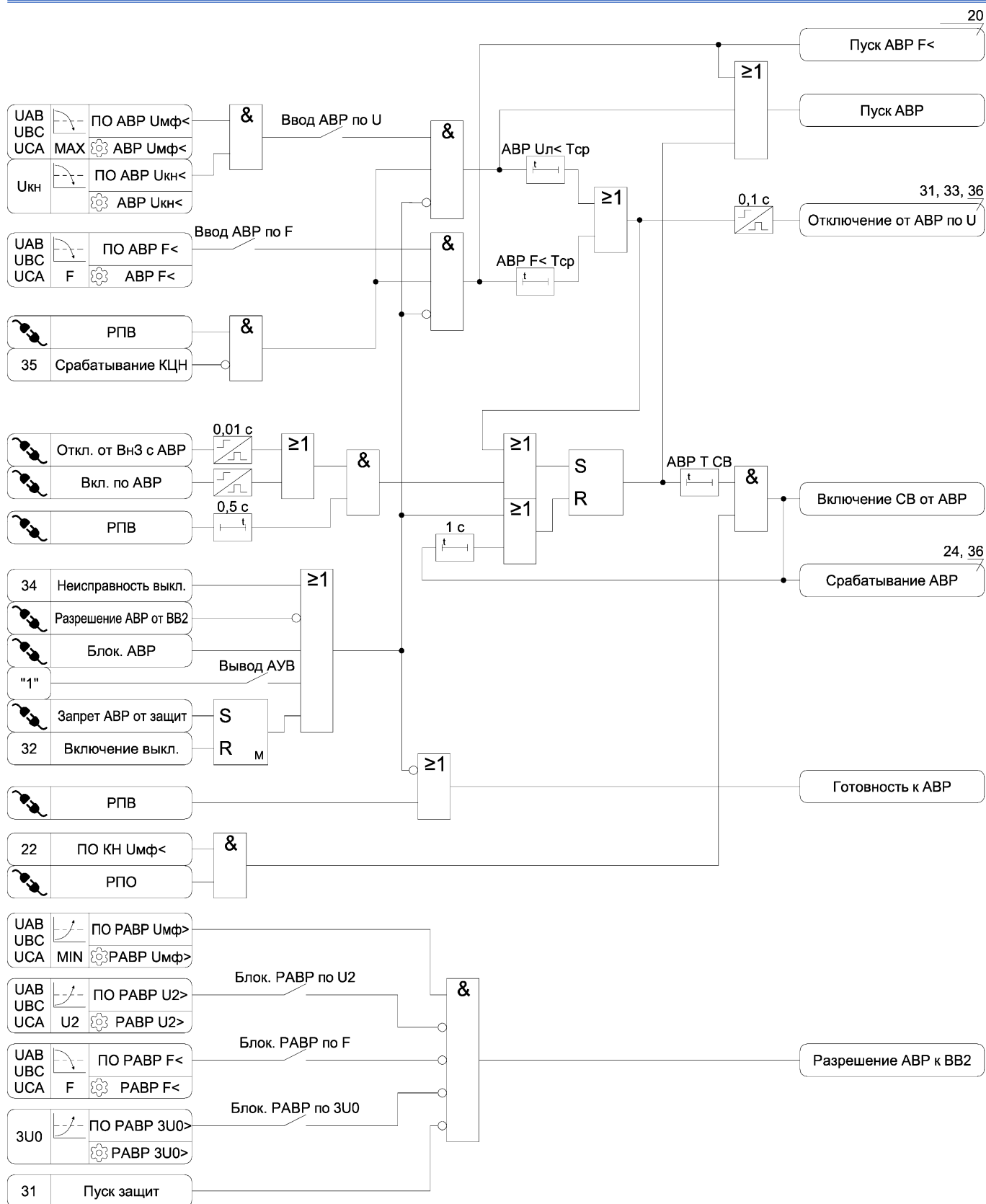
Рисунок А.23 – Функциональная схема алгоритма АВР
