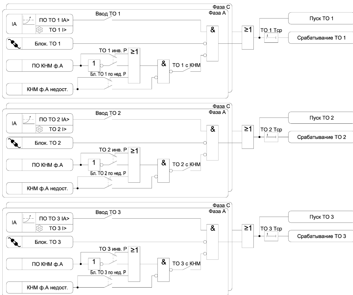
Рисунок 3.1 а) – Функциональная схема алгоритма ТО
