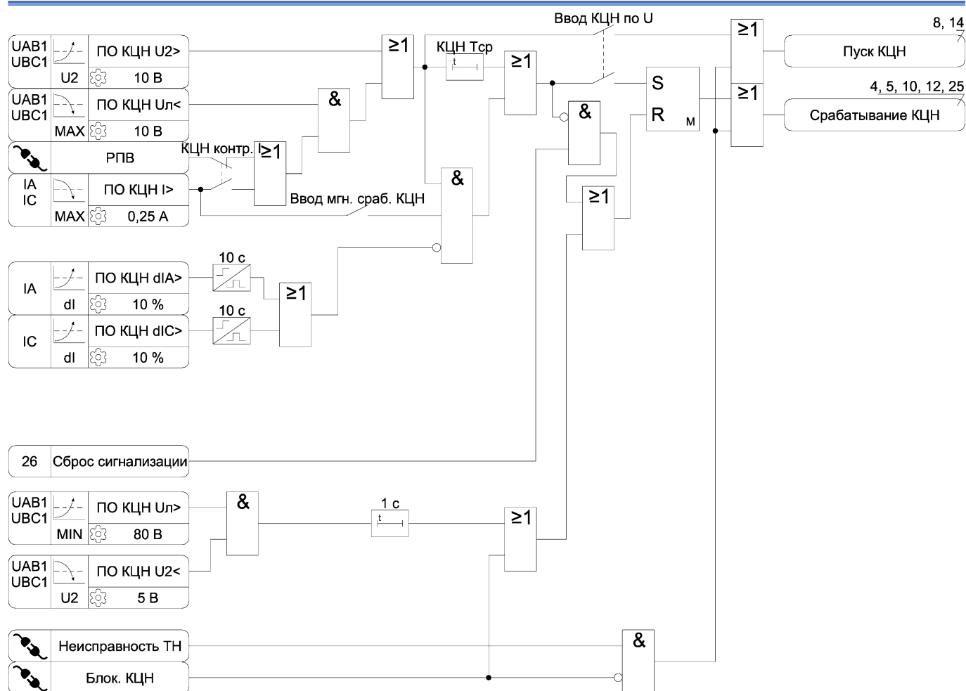
Рисунок А.24 – Функциональная схема алгоритма КЦН
