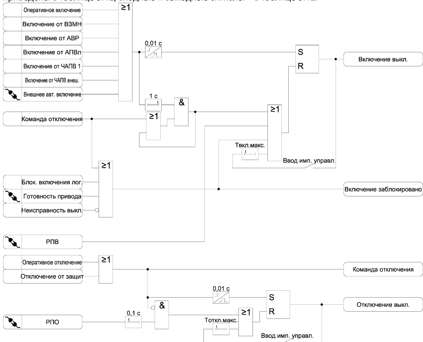
Рисунок 3.24 – Функциональная схема алгоритма управления выключателем
