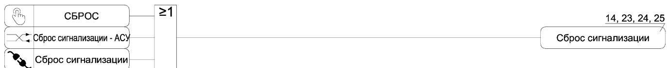
Рисунок А.26 – Функциональная схема алгоритма сброса сигнализации
