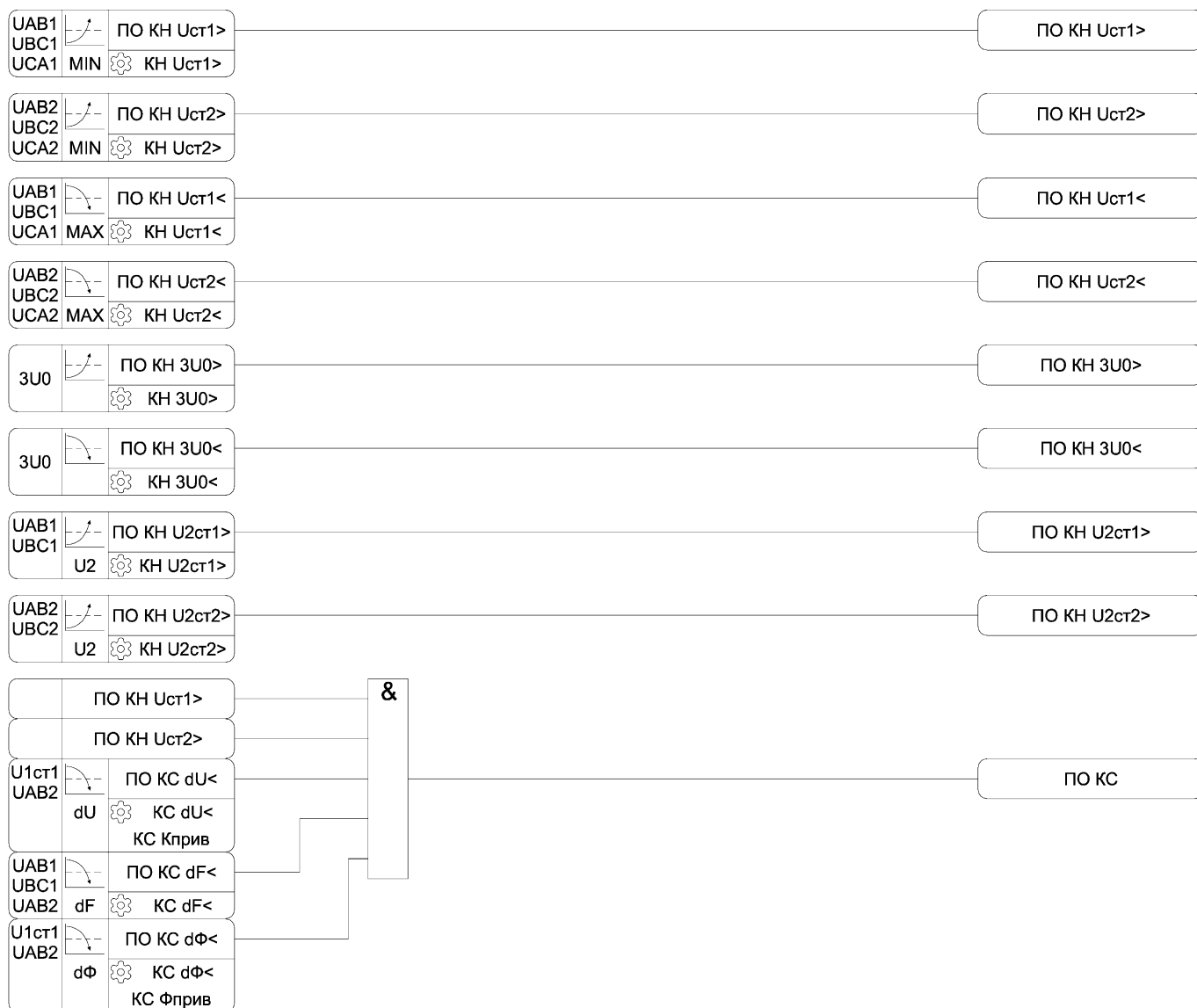
Рисунок 3.15 – Функциональная схема алгоритма КН
