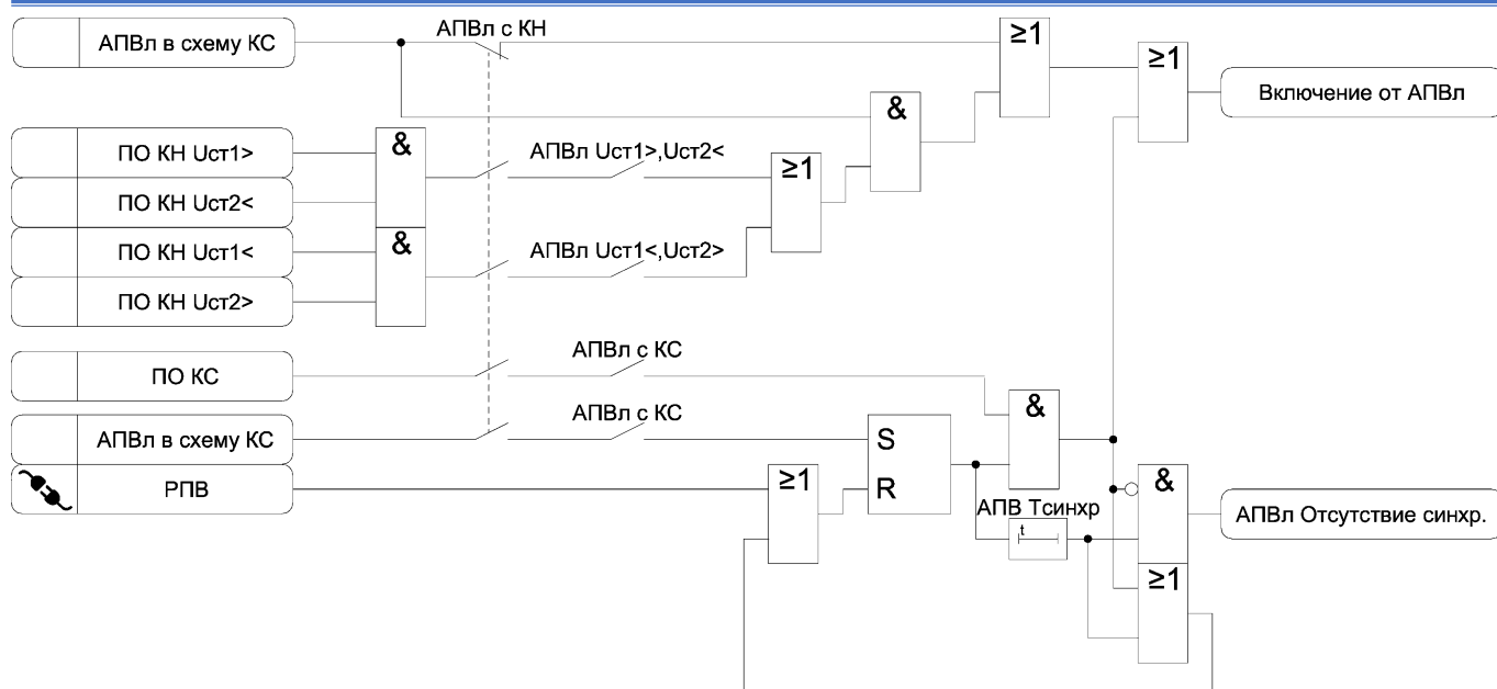
Рисунок 3.17 в) – Функциональная схема алгоритма АПВ
