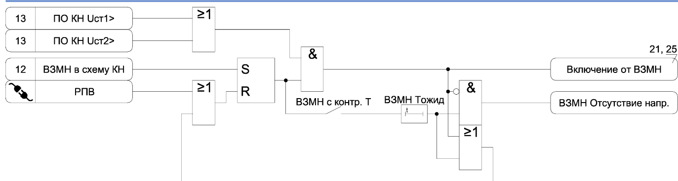
Рисунок А.12 б) – Функциональная схема алгоритма 3МН
