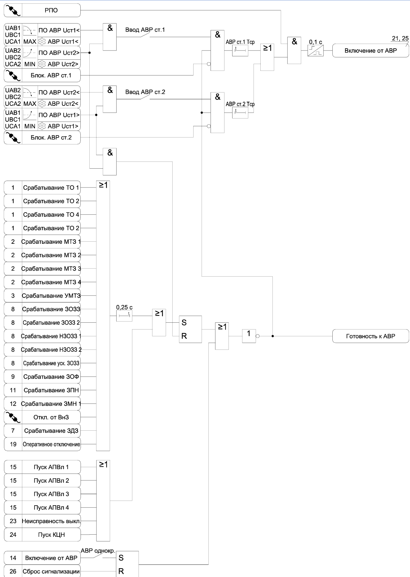
Рисунок А.14 – Функциональная схема алгоритма АВР
