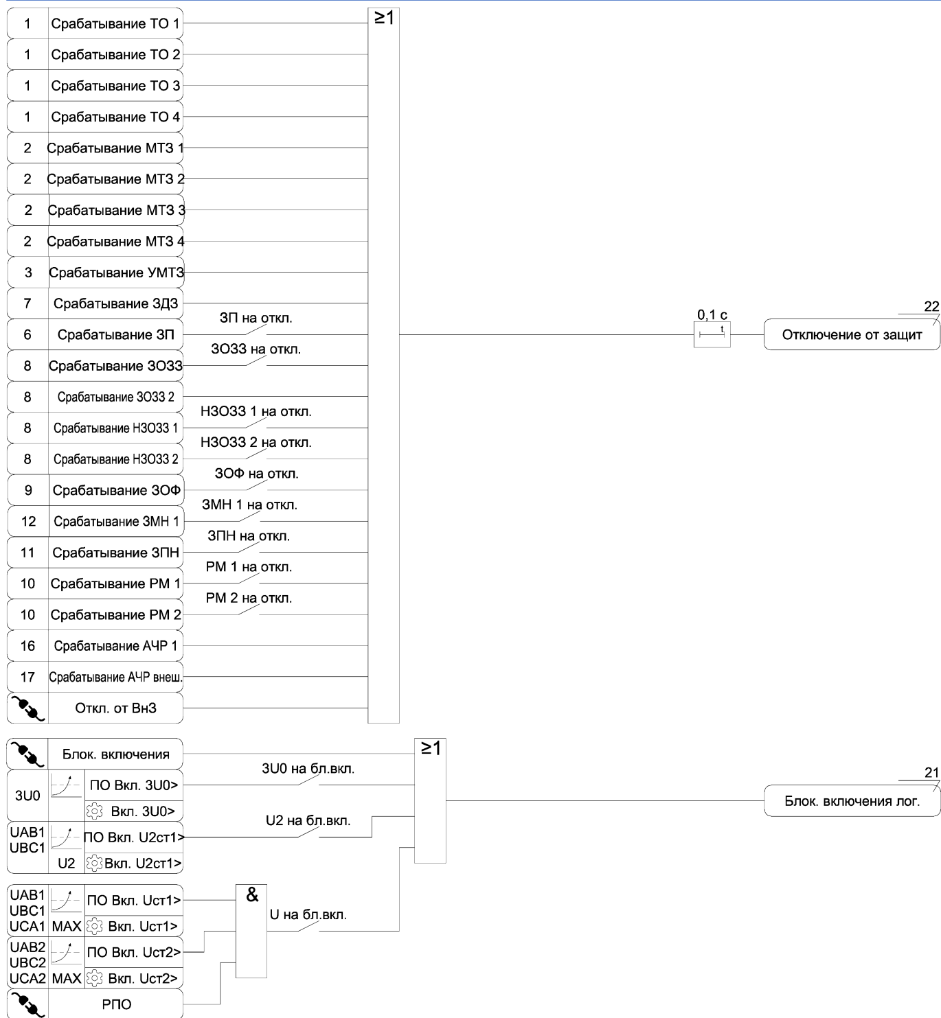
Рисунок А.20 б) – Функциональная схема алгоритма состояния защит
