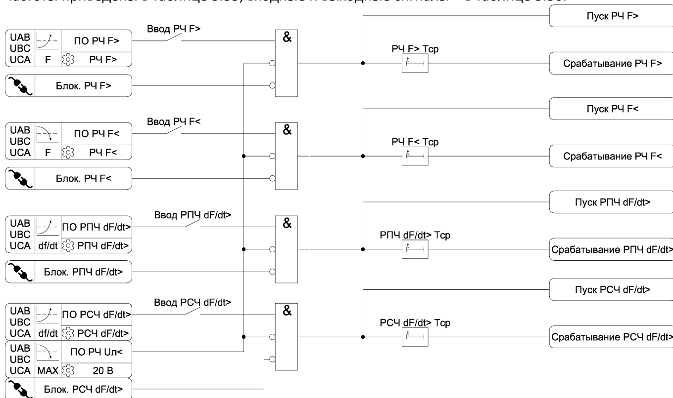
Рисунок 3.20 – Функциональные схемы алгоритмов защиты повышения и снижения частоты
