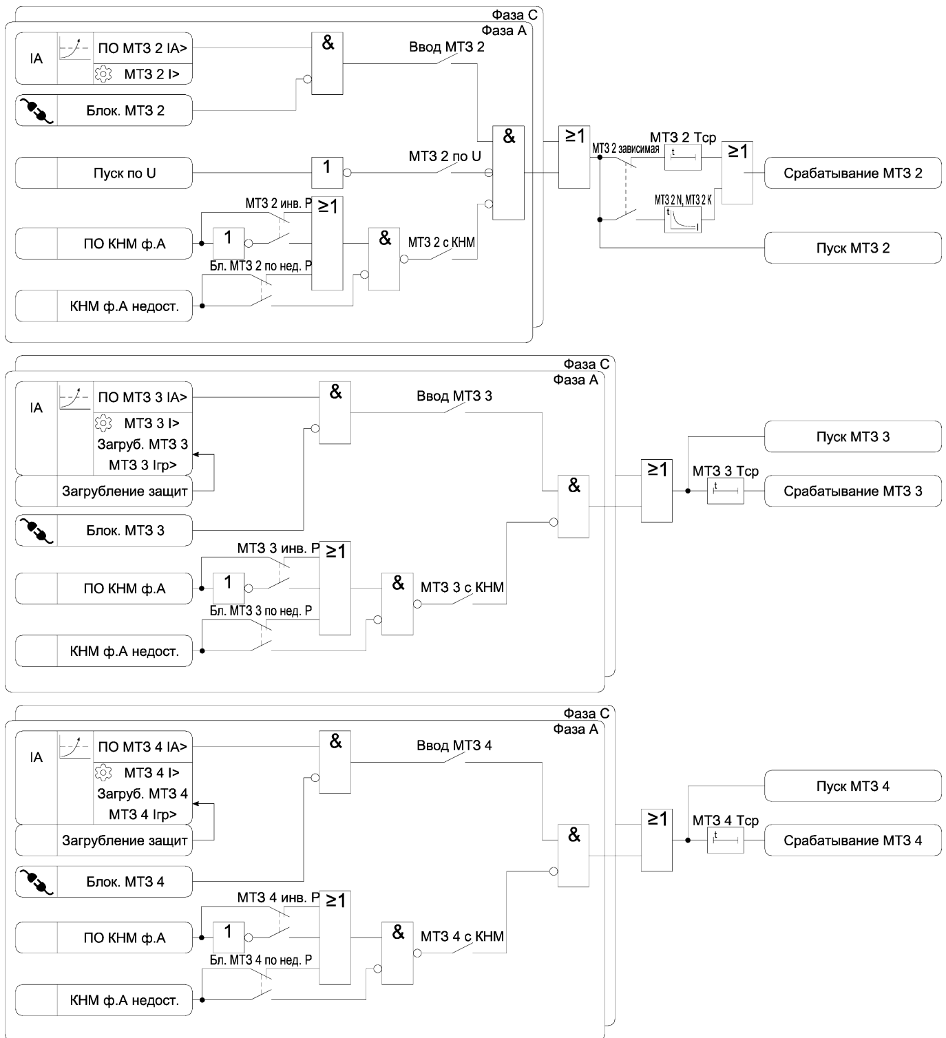
Рисунок 3.2 б) – Функциональная схема алгоритма MT3
