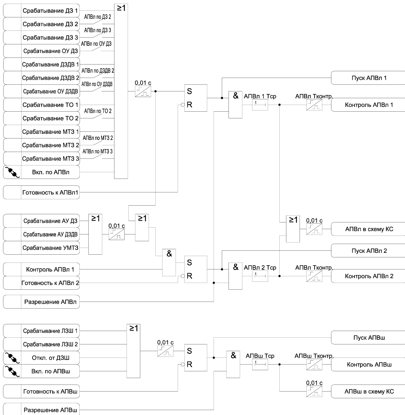
Рисунок 3.35 в) – Функциональная схема алгоритма АПВ
