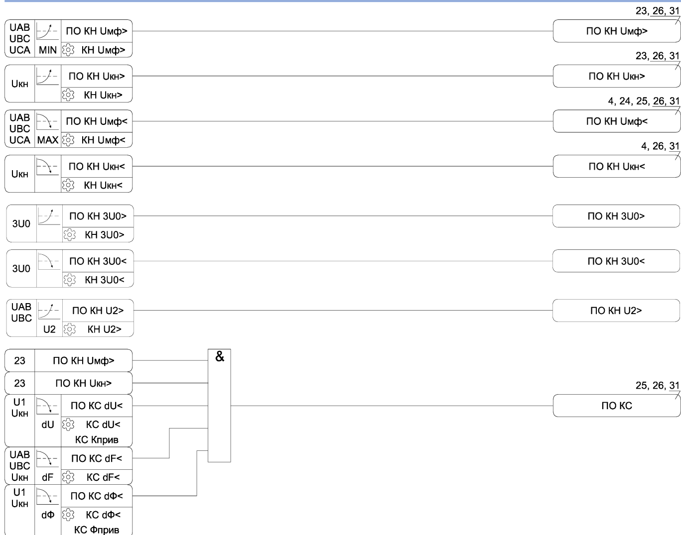
Рисунок А.23 – Функциональная схема алгоритма КН и КС
