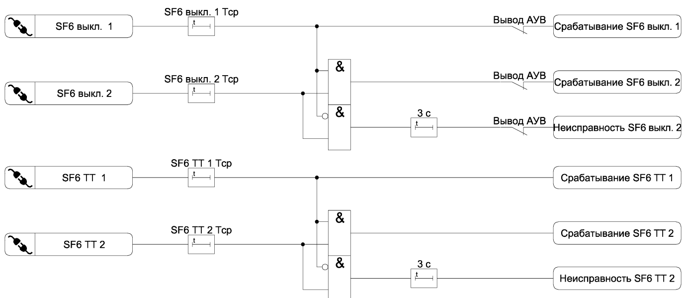
Рисунок 3.39 – Функциональная схема алгоритма защиты от снижения давления элегаза
