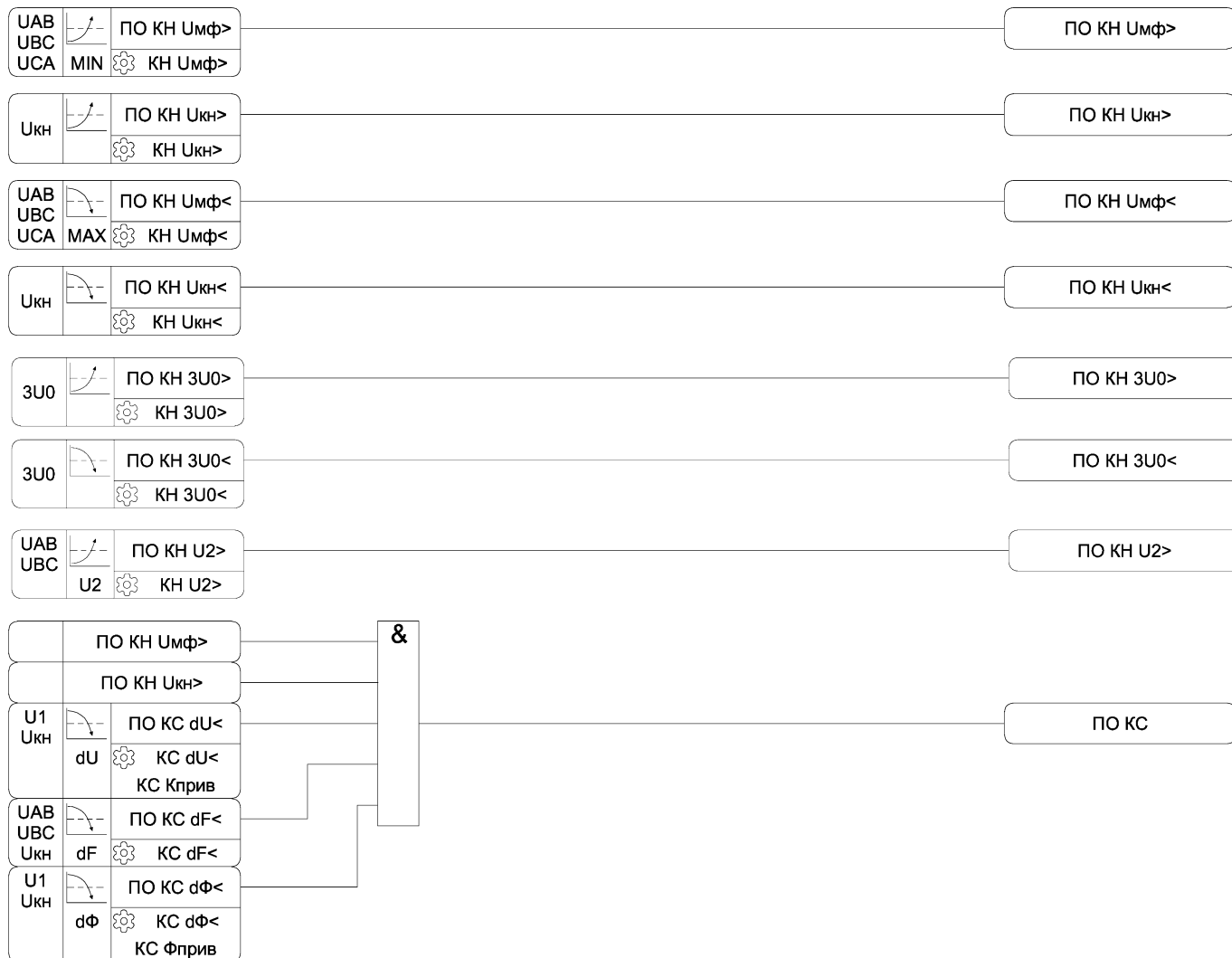
Рисунок 3.30 – Функциональная схема алгоритма КН
