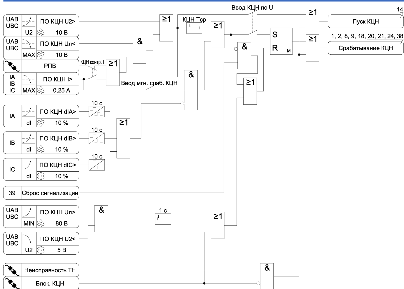
Рисунок А.37 – Функциональная схема алгоритма КЦН
