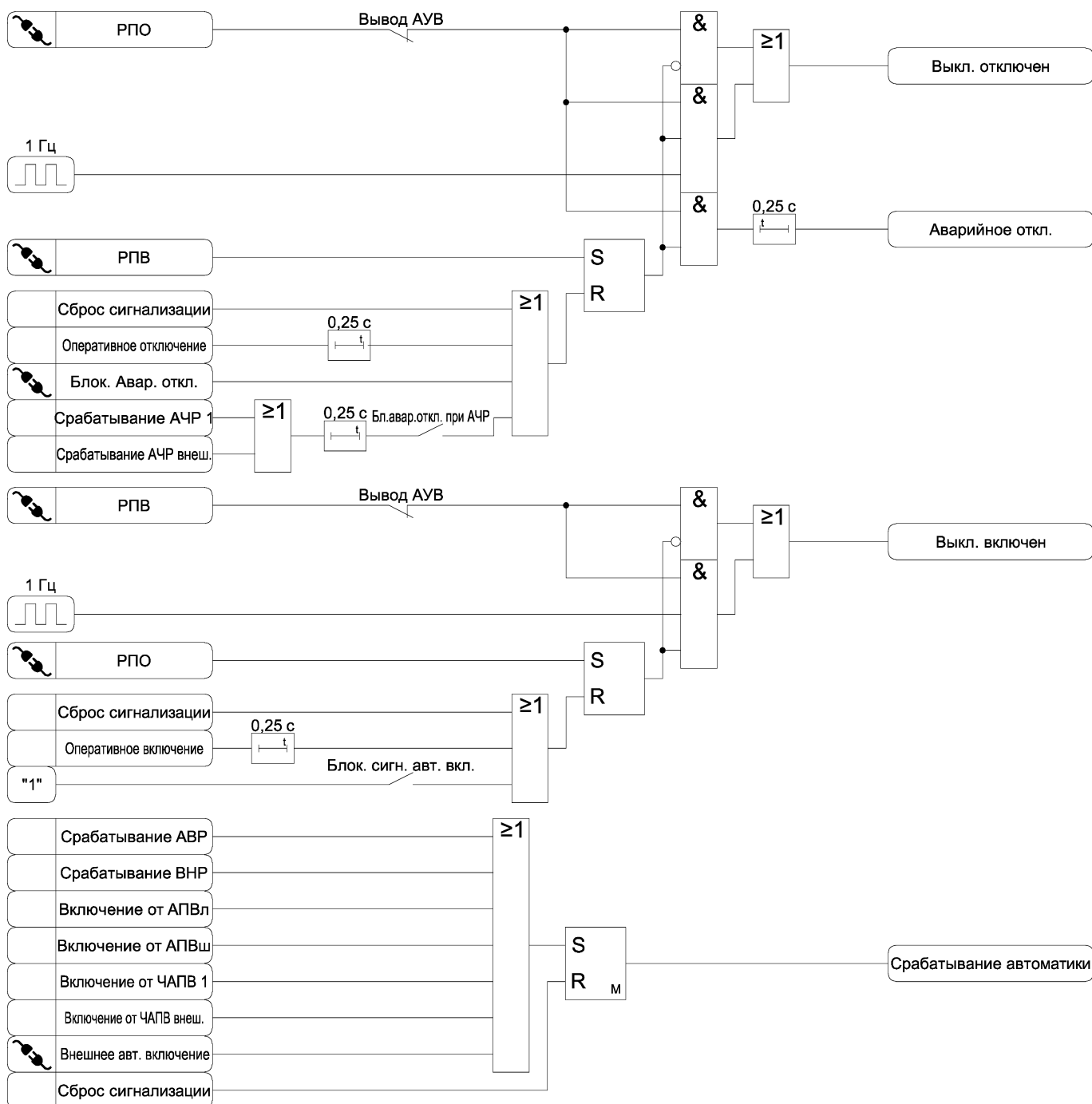
Рисунок 3.47 а) – Функциональная схема алгоритма сигнализации
