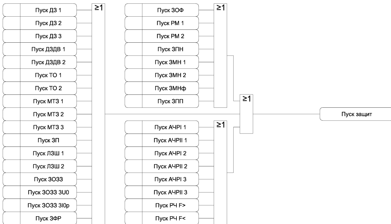
Рисунок 3.42 а) – Функциональная схема алгоритма формирования сигналов состояния защит
