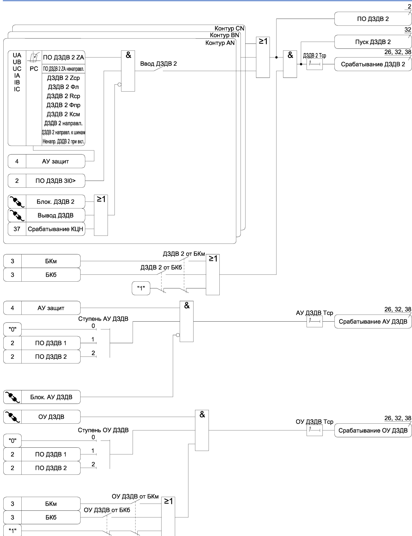
Рисунок А.2 б) – Функциональная схема алгоритма ДЗДВ
