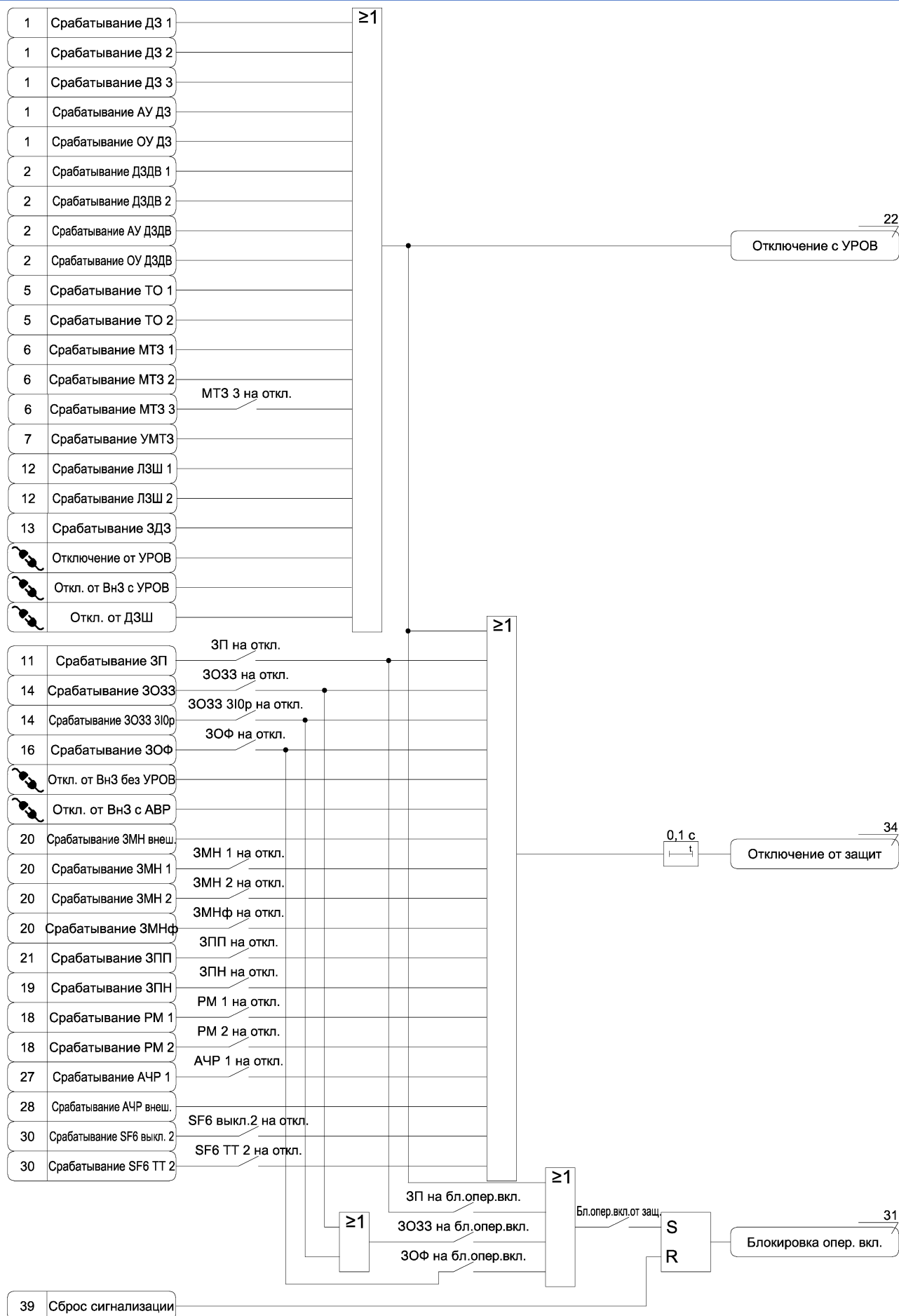
Рисунок А.32 б) – Функциональная схема алгоритма состояния защит
