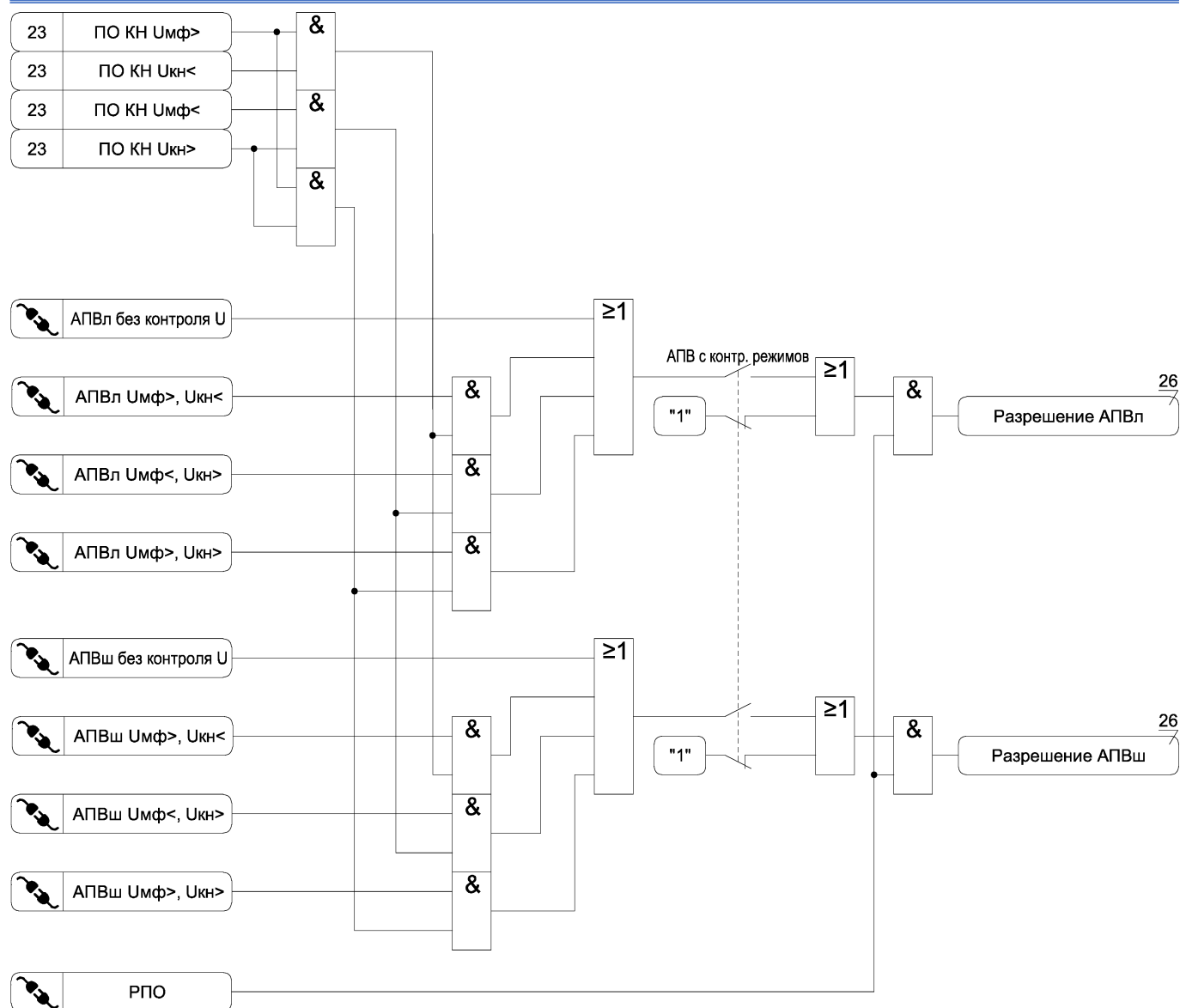
Рисунок А.26 а) – Функциональная схема алгоритма АПУ
