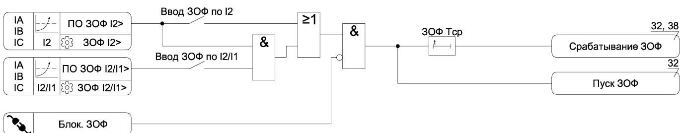
Рисунок А.16 – Функциональная схема алгоритма 30Ф
