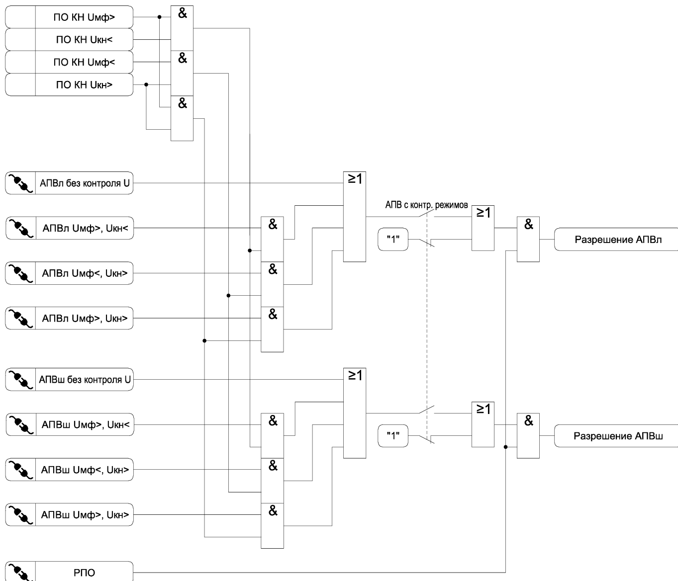
Рисунок 3.35 а) – Функциональная схема алгоритма АПВ
