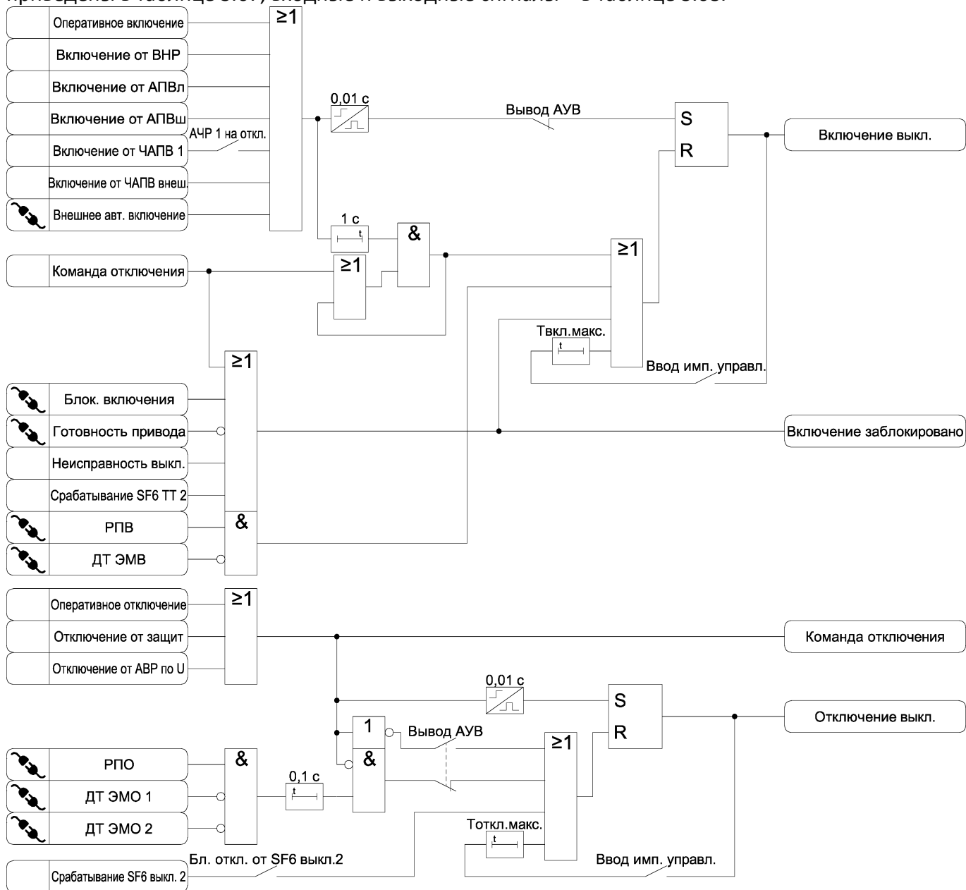
Рисунок 3.43 – Функциональная схема алгоритма управления выключателем
