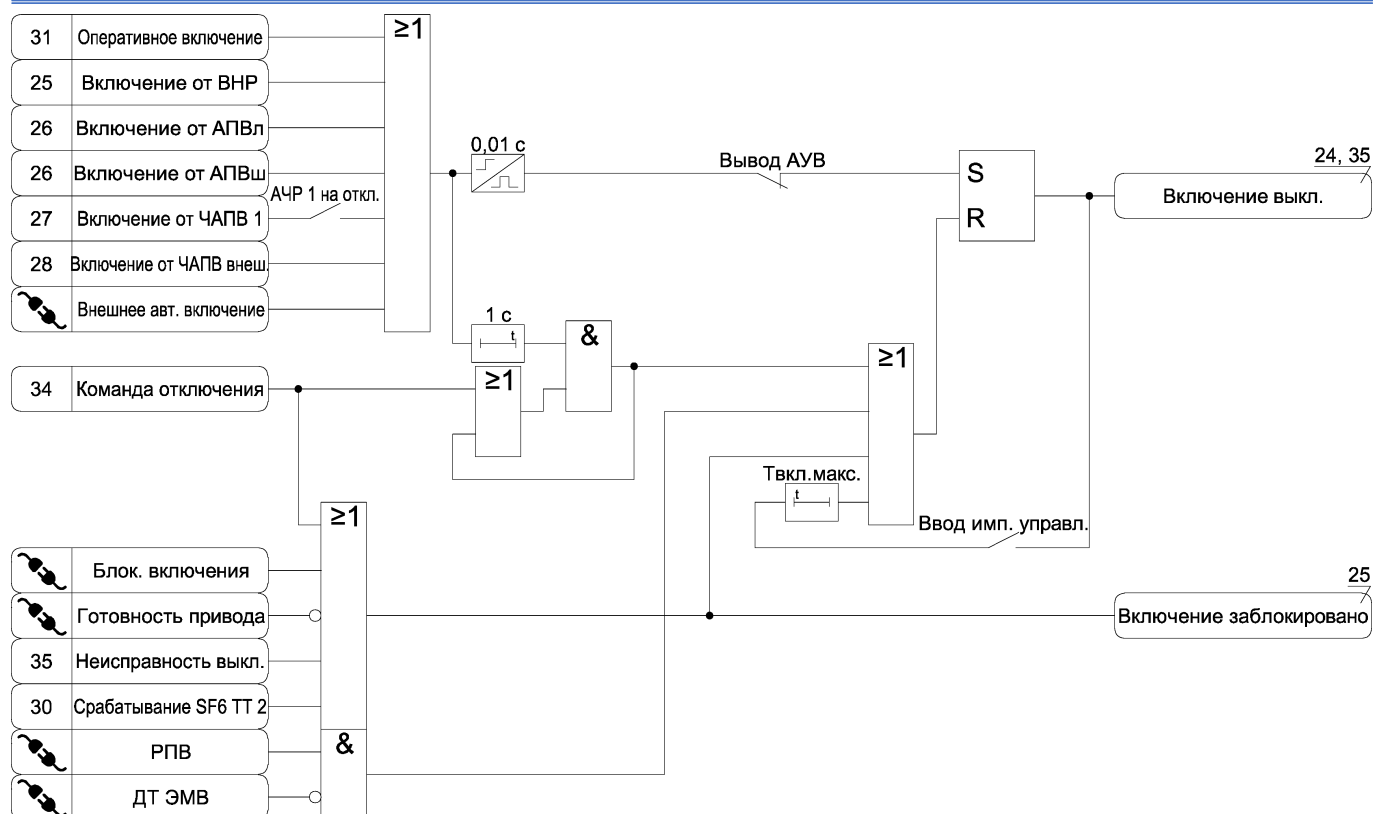
Рисунок А.33 – Функциональная схема алгоритма включения выключателя
