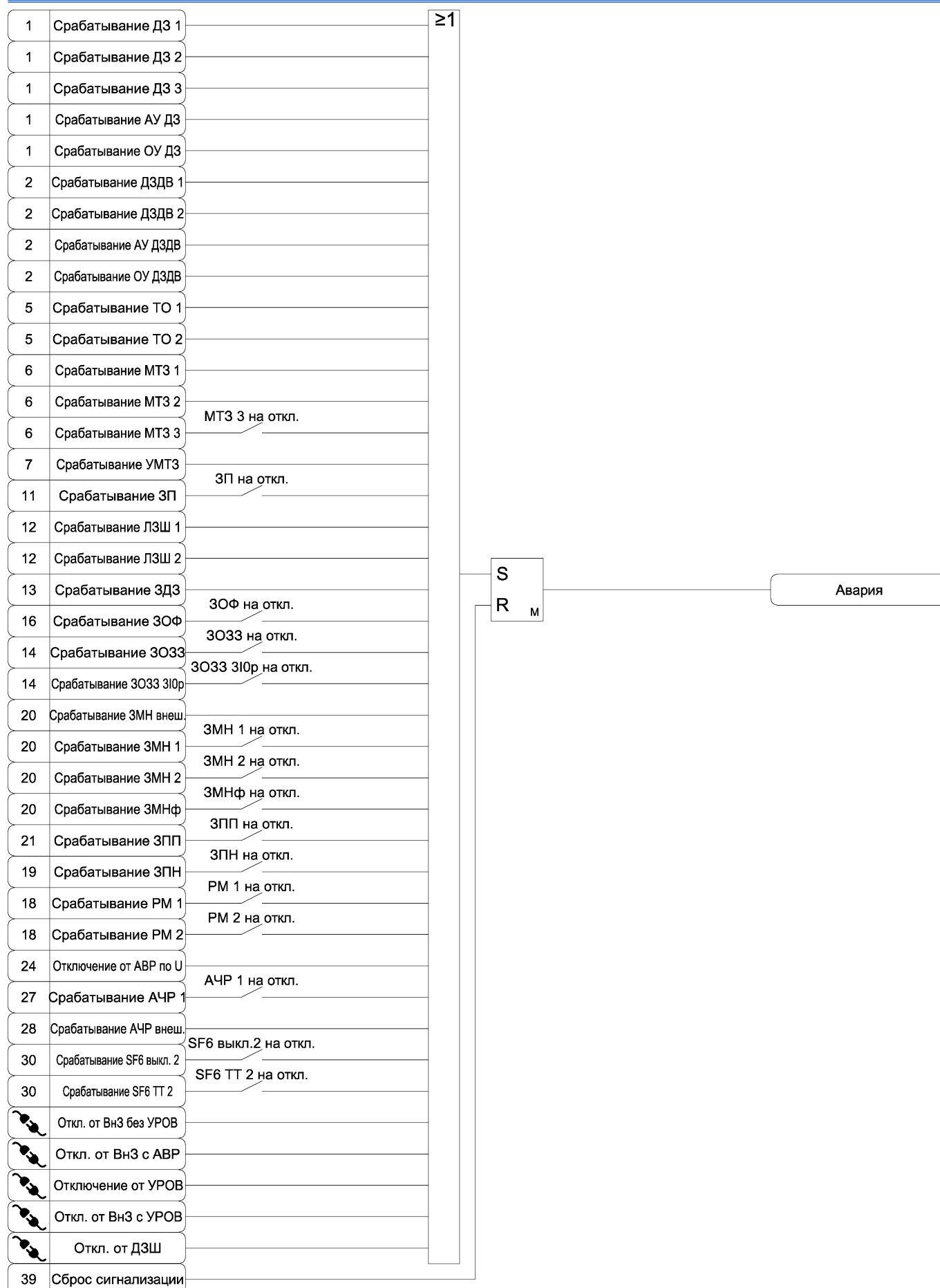
Рисунок А.38 б) – Функциональная схема алгоритма сигнализации
