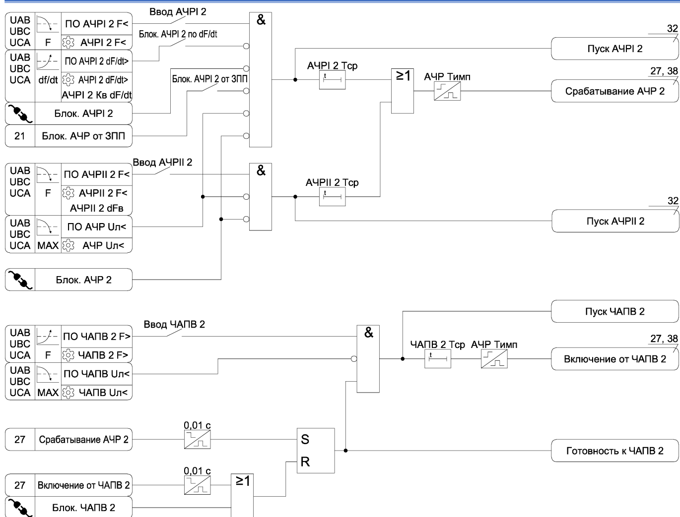
Рисунок А.27 б) – Функциональная схема алгоритма АЧР и ЧАПВ
