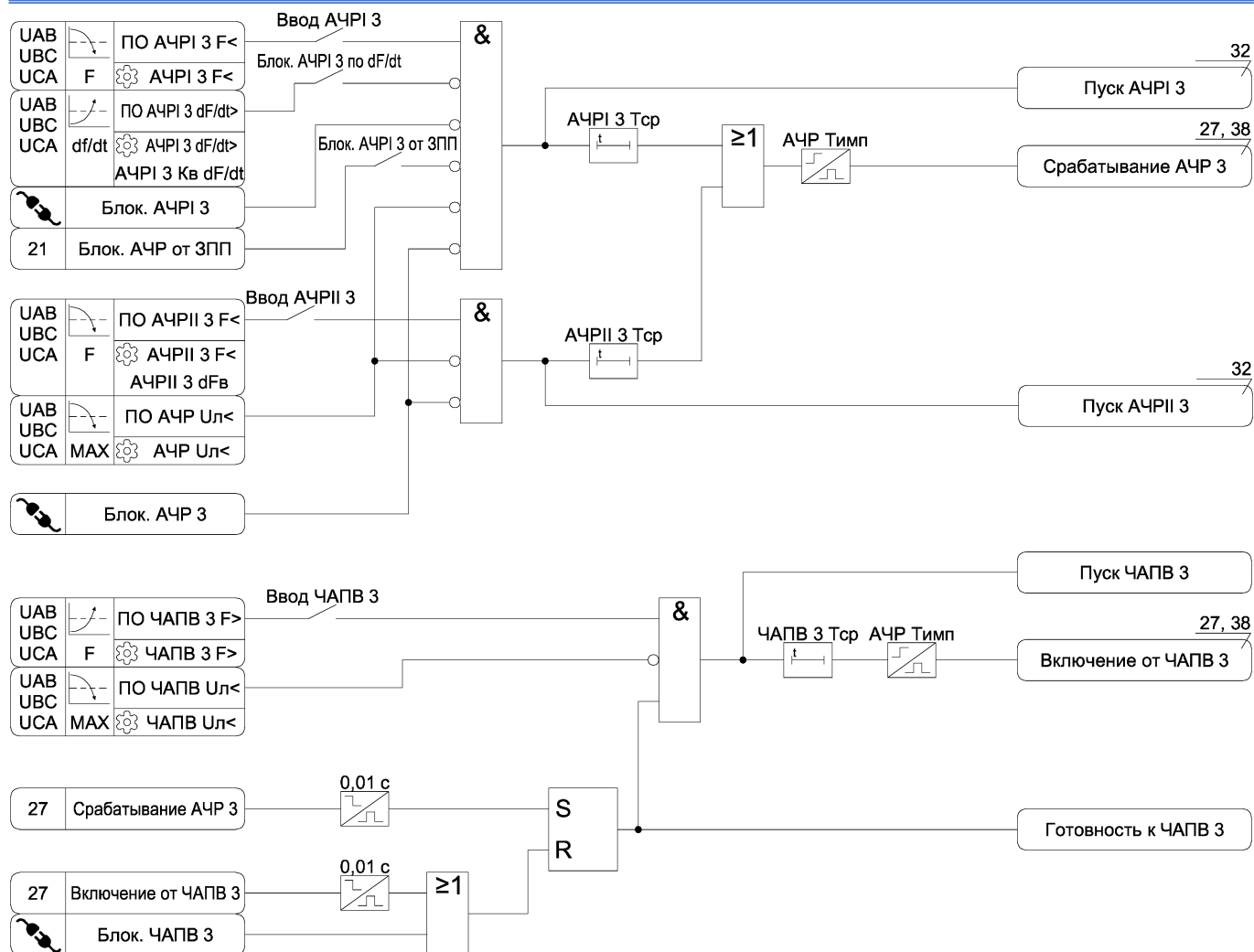
Рисунок А.27 в) – Функциональная схема алгоритма АЧР и АЧРВ
