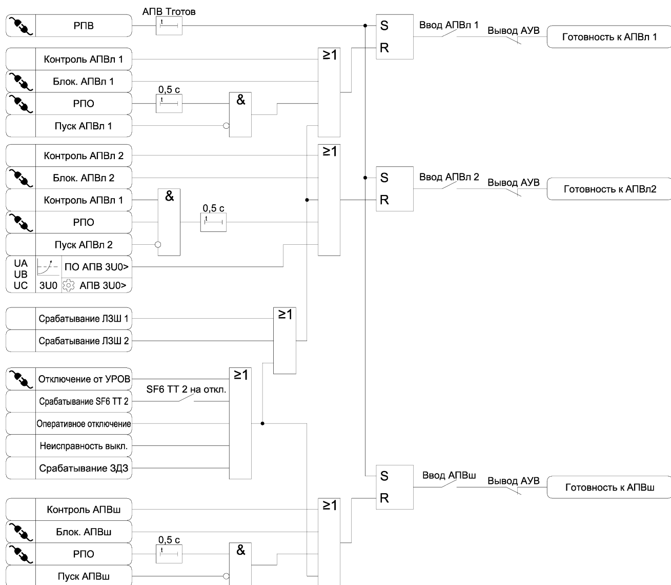
Рисунок 3.35 б) – Функциональная схема алгоритма АПВ
