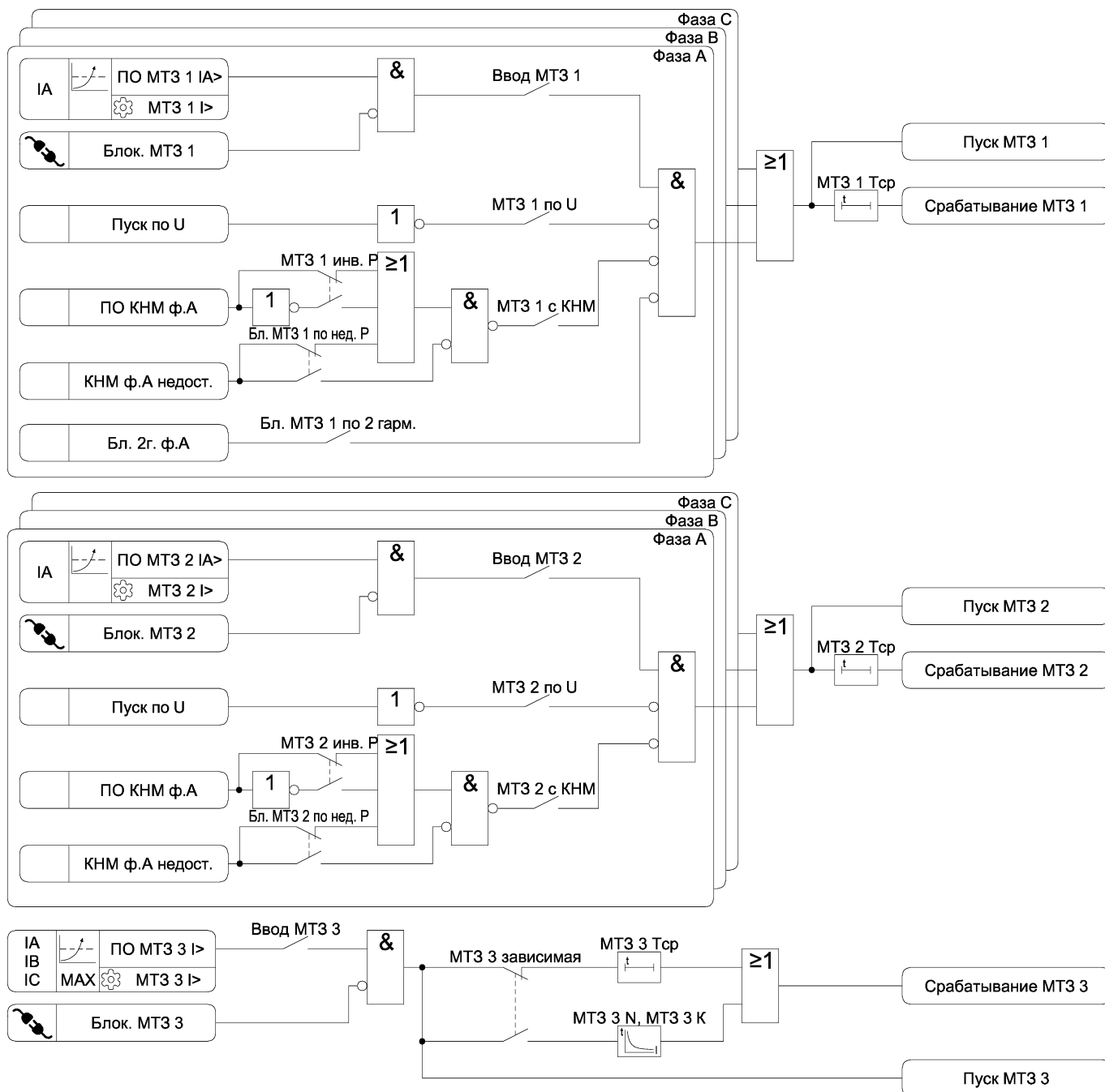
Рисунок 3.9 – Функциональная схема алгоритма МТЗ
