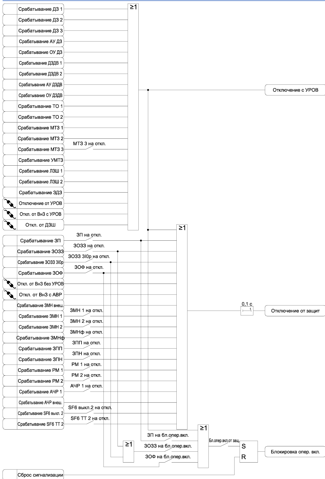
Рисунок 3.42 б) – Функциональная схема алгоритма формирования сигналов состояния защит
