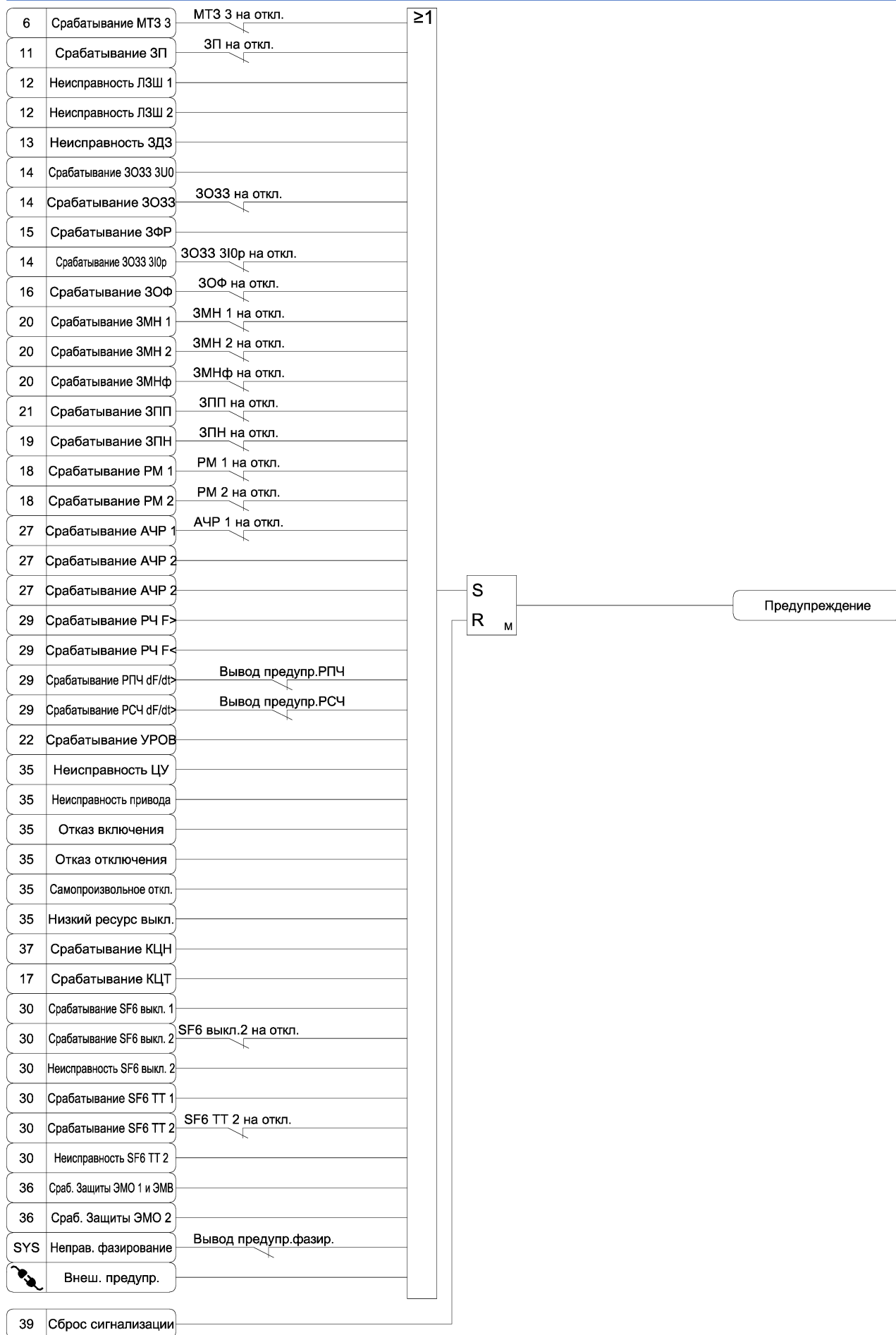
Рисунок А.38 в) – Функциональная схема алгоритма сигнализации
