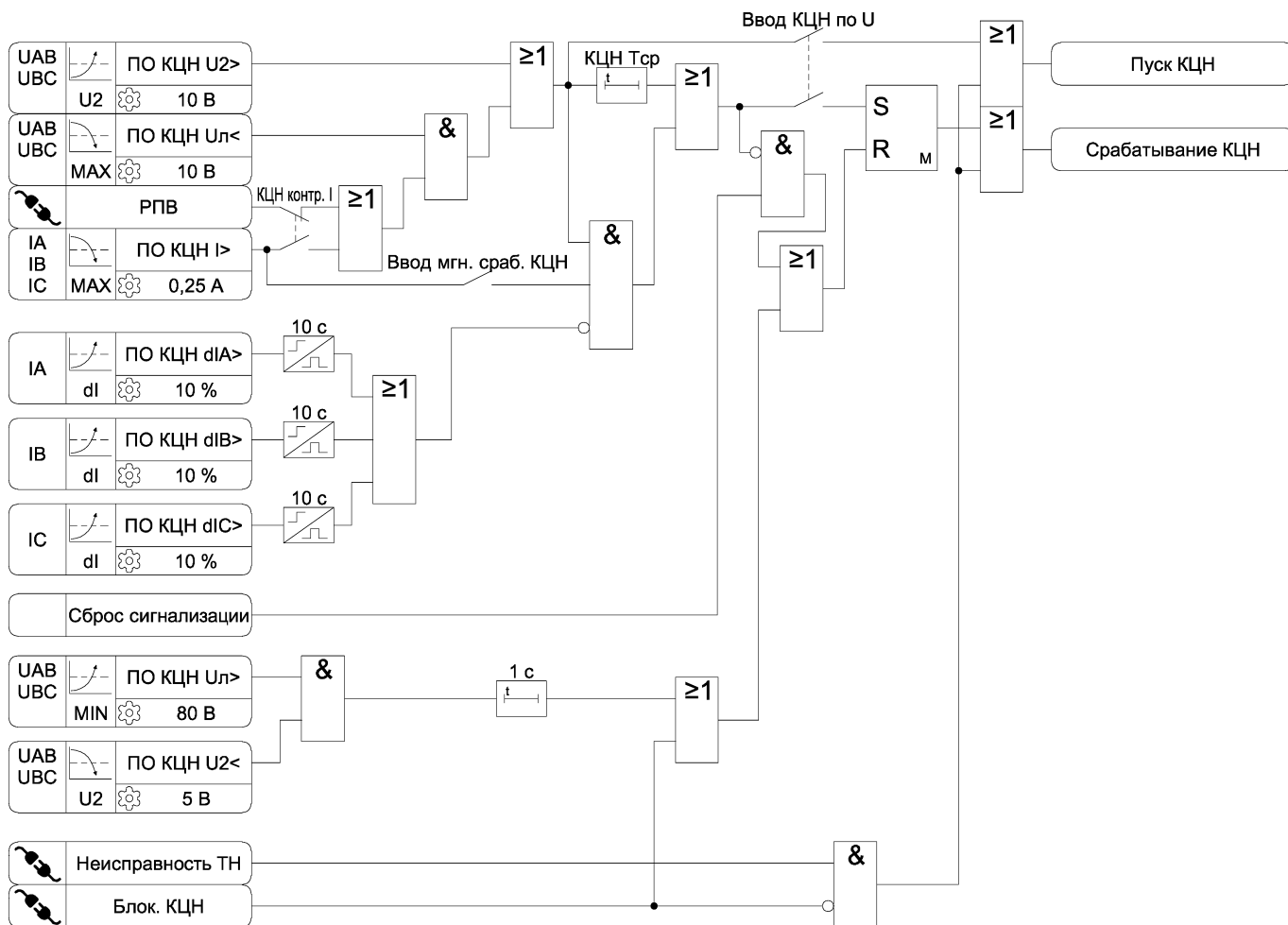
Рисунок 3.46 – Функциональная схема алгоритма КЦН
