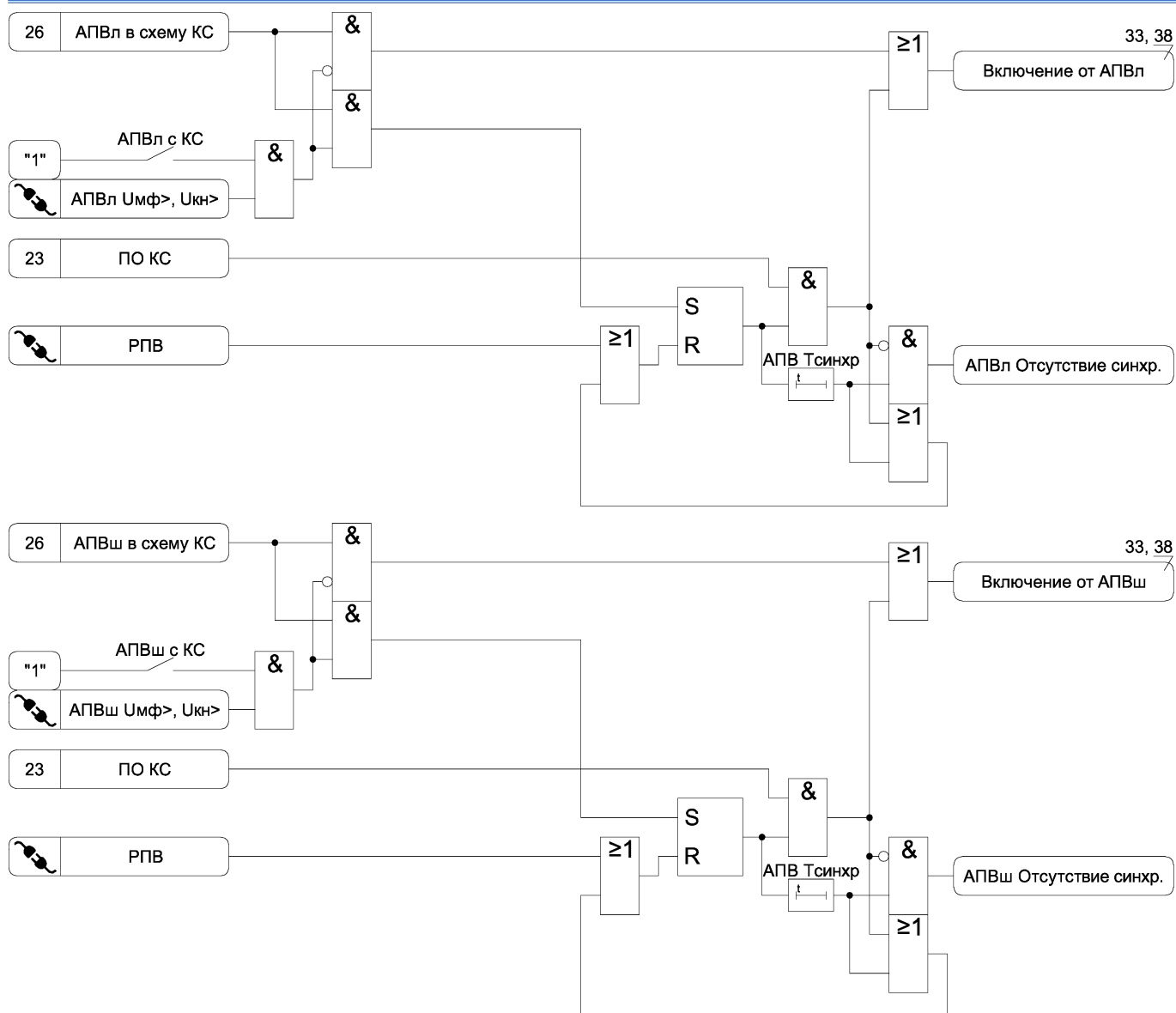
Рисунок А.26 г) – Функциональная схема алгоритма АПВ
