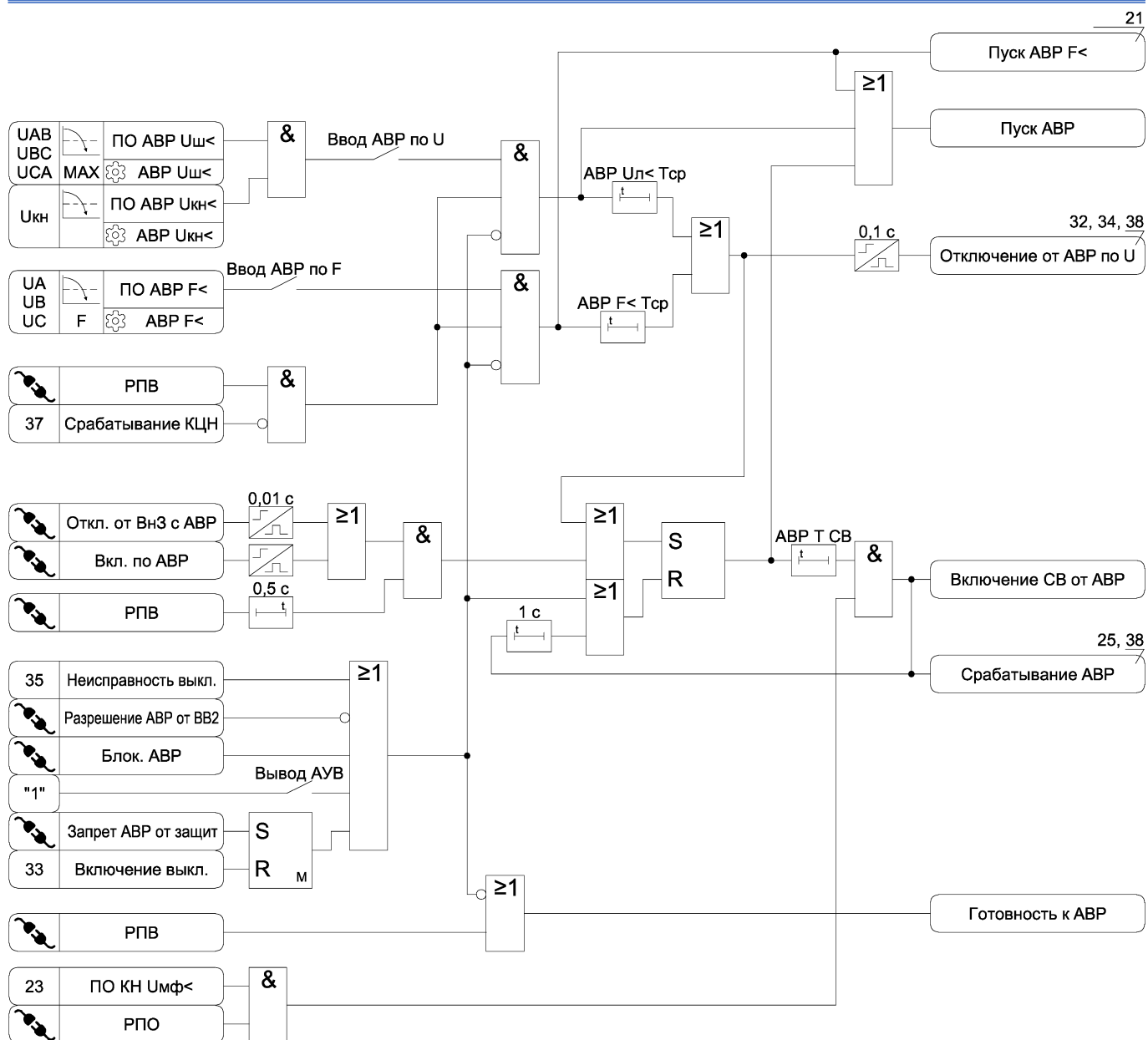
Рисунок А.24 – Функциональная схема алгоритма АВР
