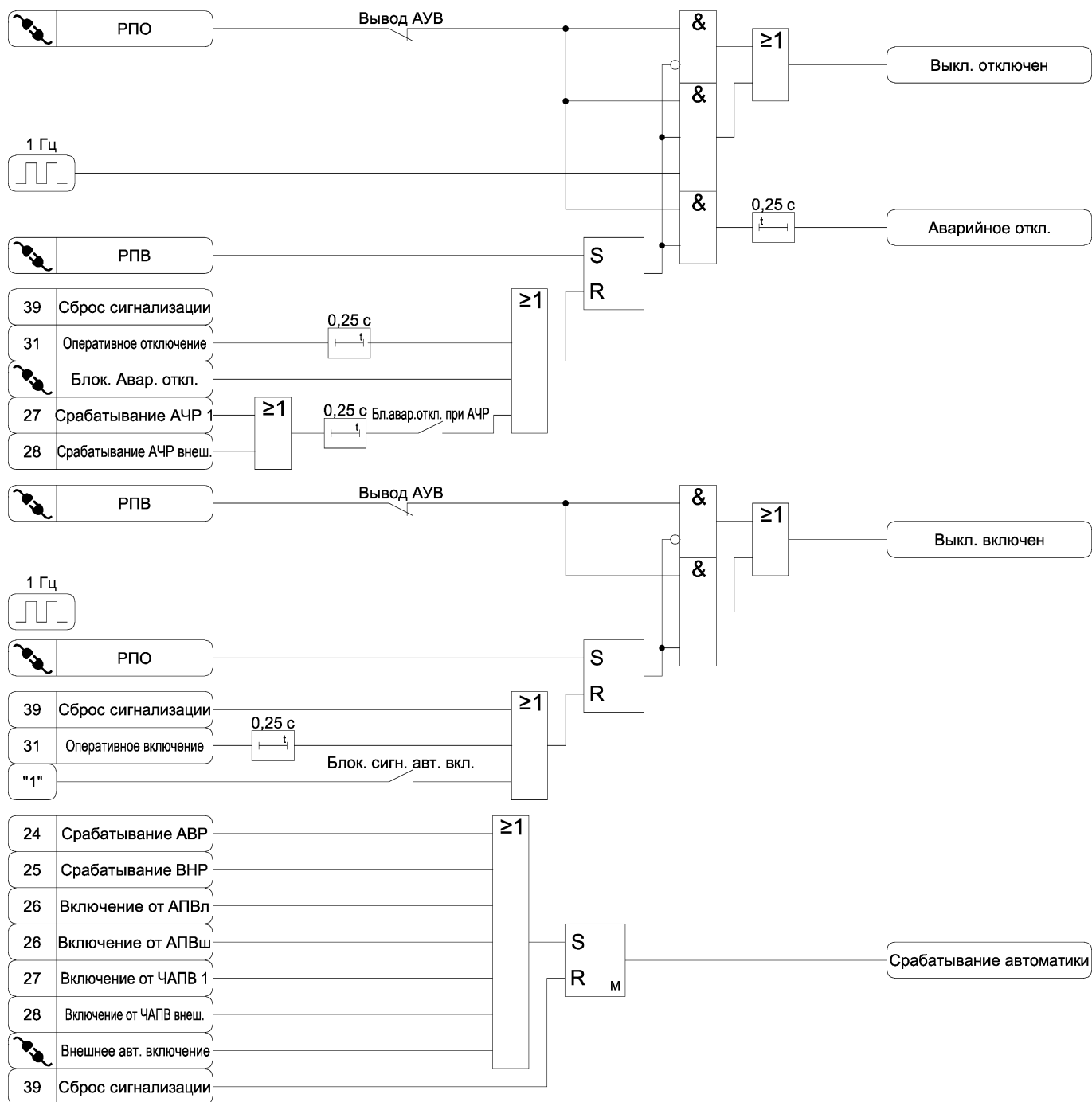
Рисунок А.38 а) – Функциональная схема алгоритма сигнализации
