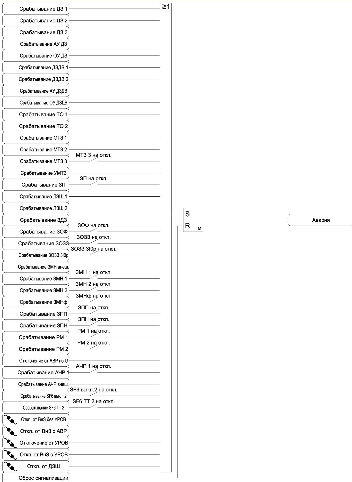
Рисунок 3.47 б) – Функциональная схема алгоритма сигнализации
