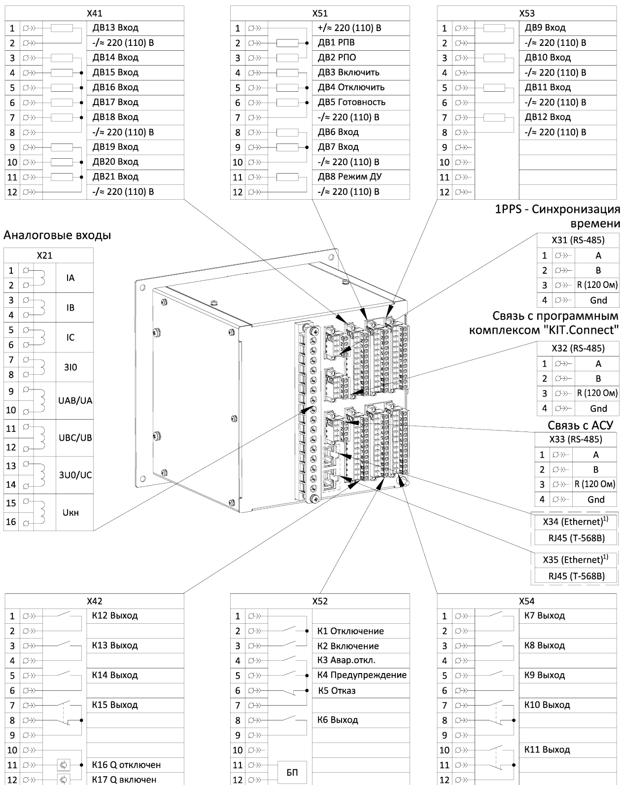
Рисунок 2.1 – Схема подключения устройства
