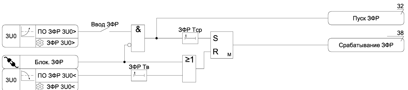
Рисунок А.15 – Функциональная схема алгоритма 3Ф
