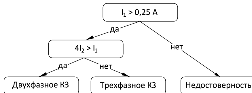
Рисунок 3.49 – Блок-схема определения вида короткого замыкания
