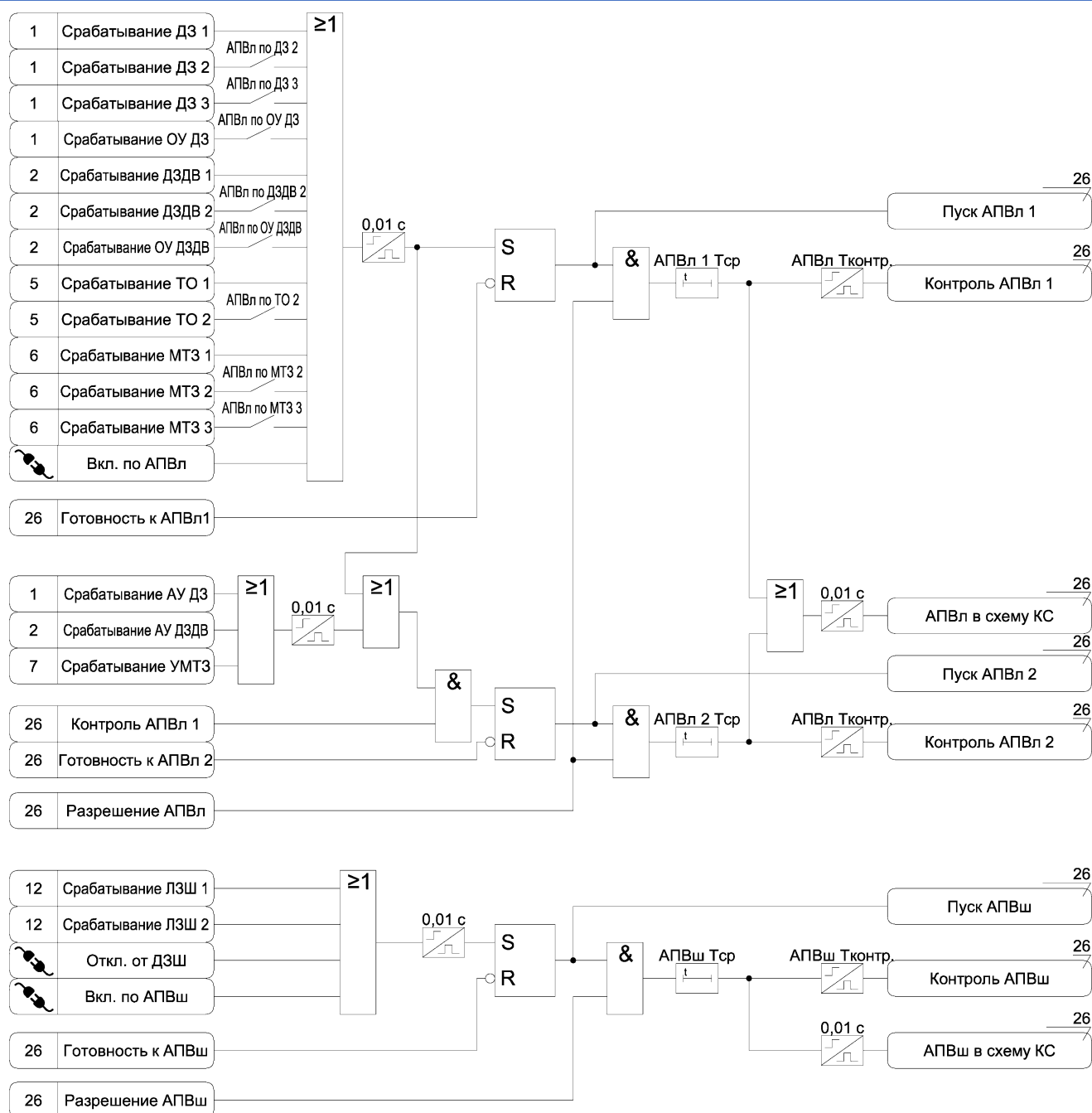
Рисунок А.26 в) – Функциональная схема алгоритма АПВ
