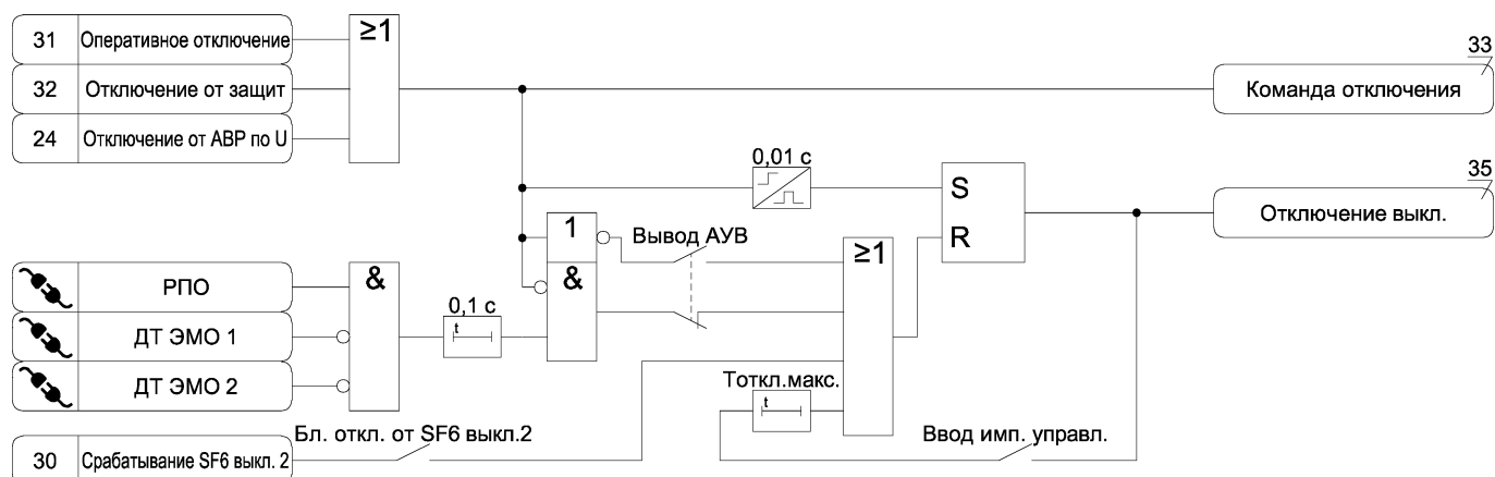
Рисунок А.34 – Функциональная схема алгоритма отключения выключателя
