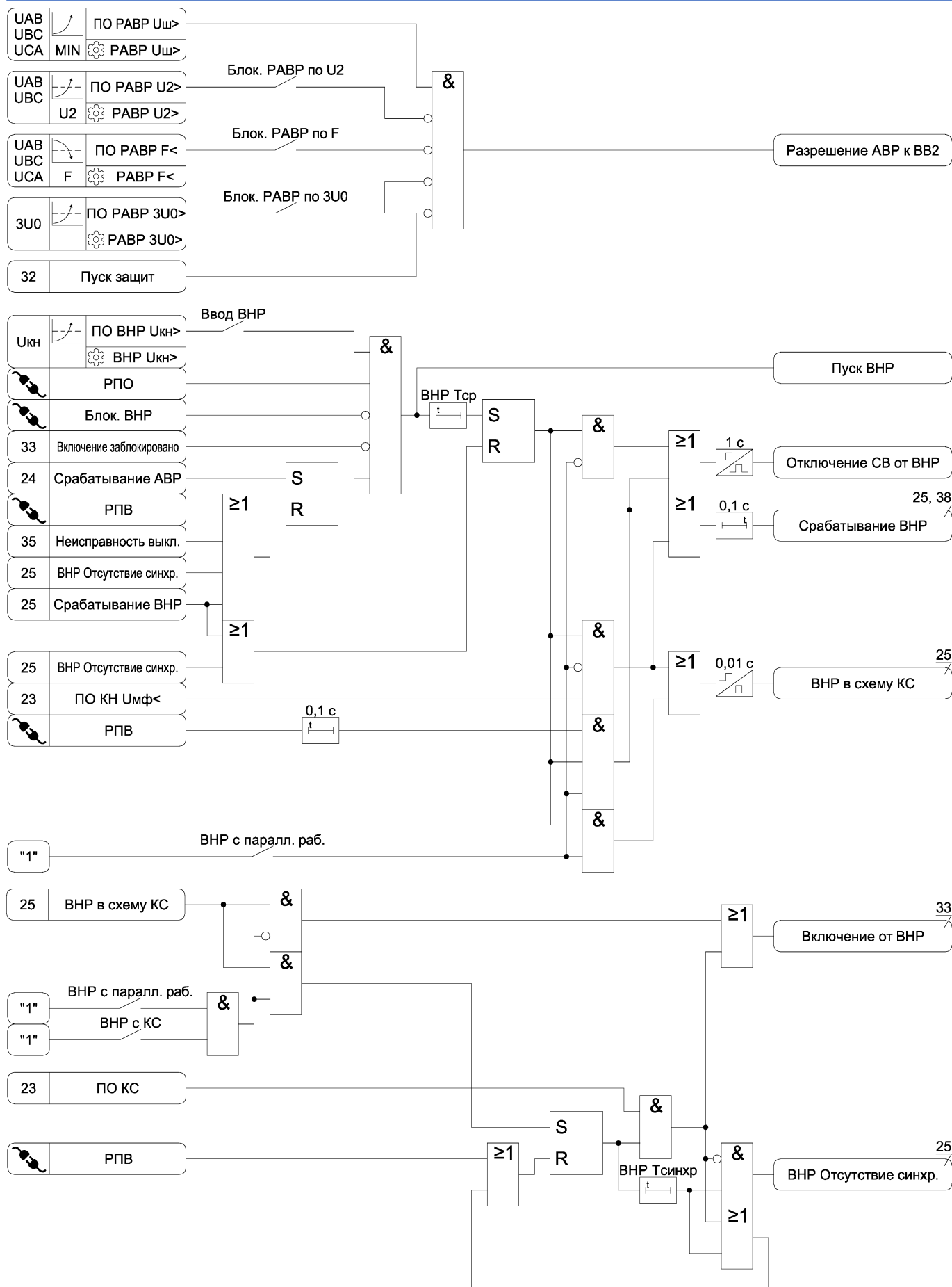
Рисунок А.25 – Функциональная схема алгоритма ВНР
