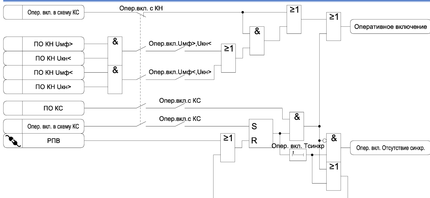
Рисунок 3.40 б) – Функциональная схема алгоритма оперативного управления выключателем
