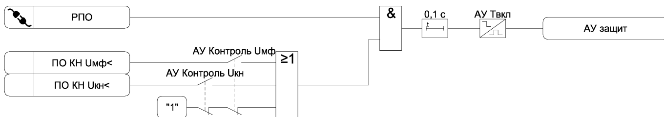
Рисунок 3.7 – Функциональная схема алгоритма автоматического ускорения защит
