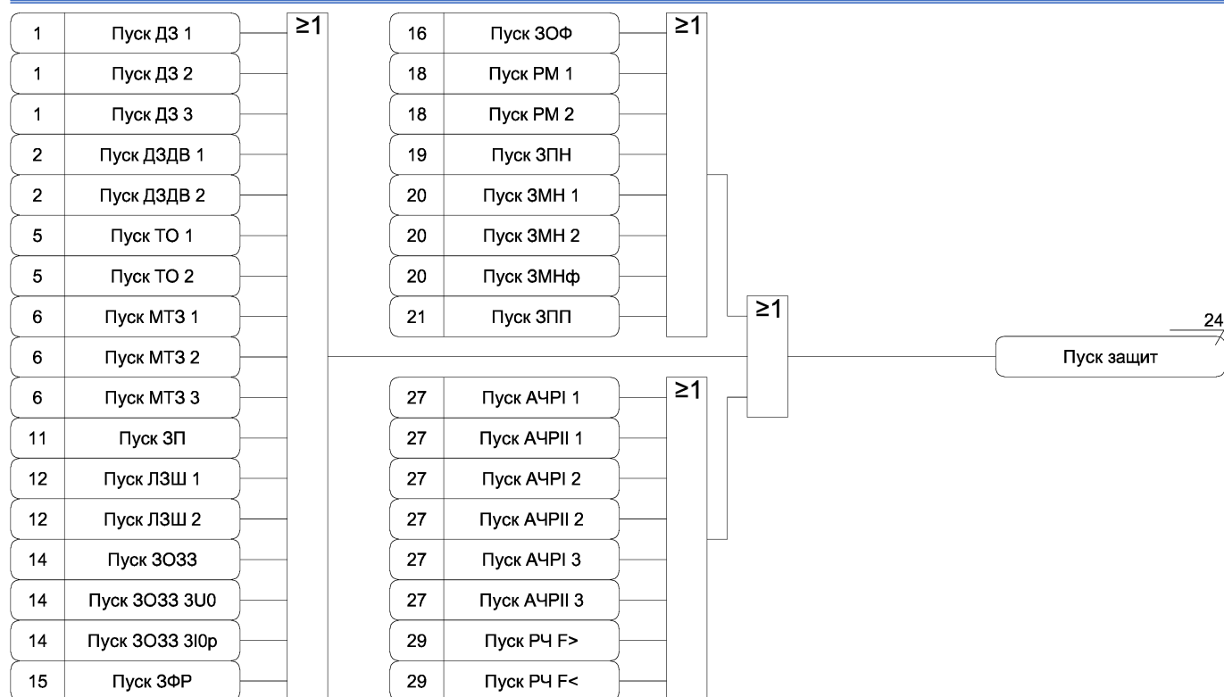
Рисунок А.32 а) – Функциональная схема алгоритма состояния защит
