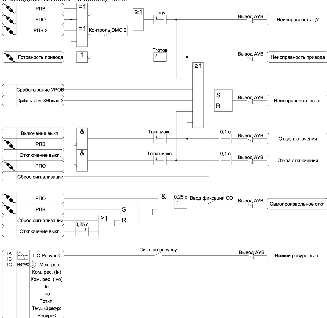
Рисунок 3.44 – Функциональная схема алгоритма диагностики выключателя
