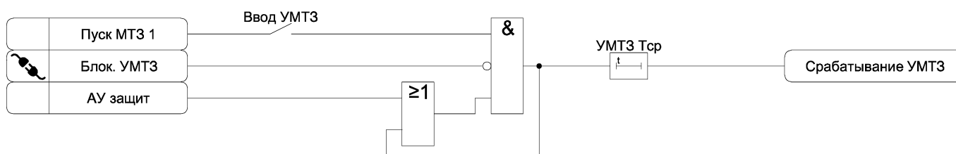
Рисунок 3.10 – Функциональная схема алгоритма УМТЗ
