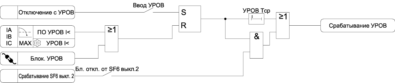
Рисунок 3.29 – Функциональная схема алгоритма УРОВ
