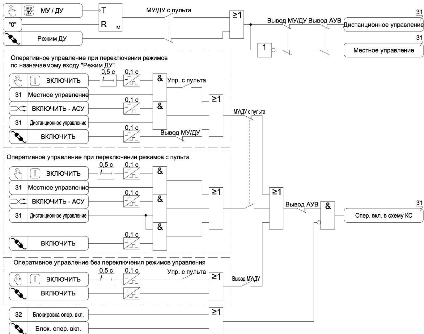
Рисунок А.31 а) – Функциональная схема алгоритма оперативного управления выключателем
