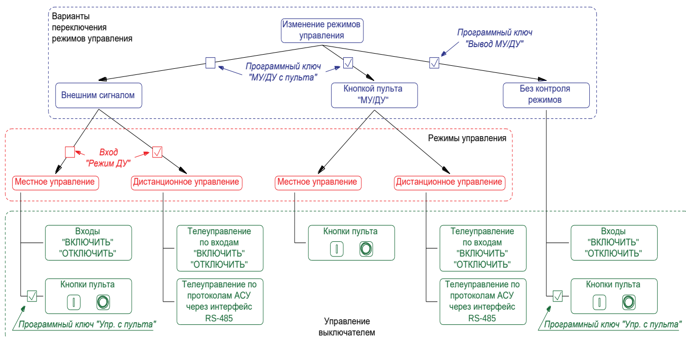
Рисунок 3.41 – Выбор режимов управления
