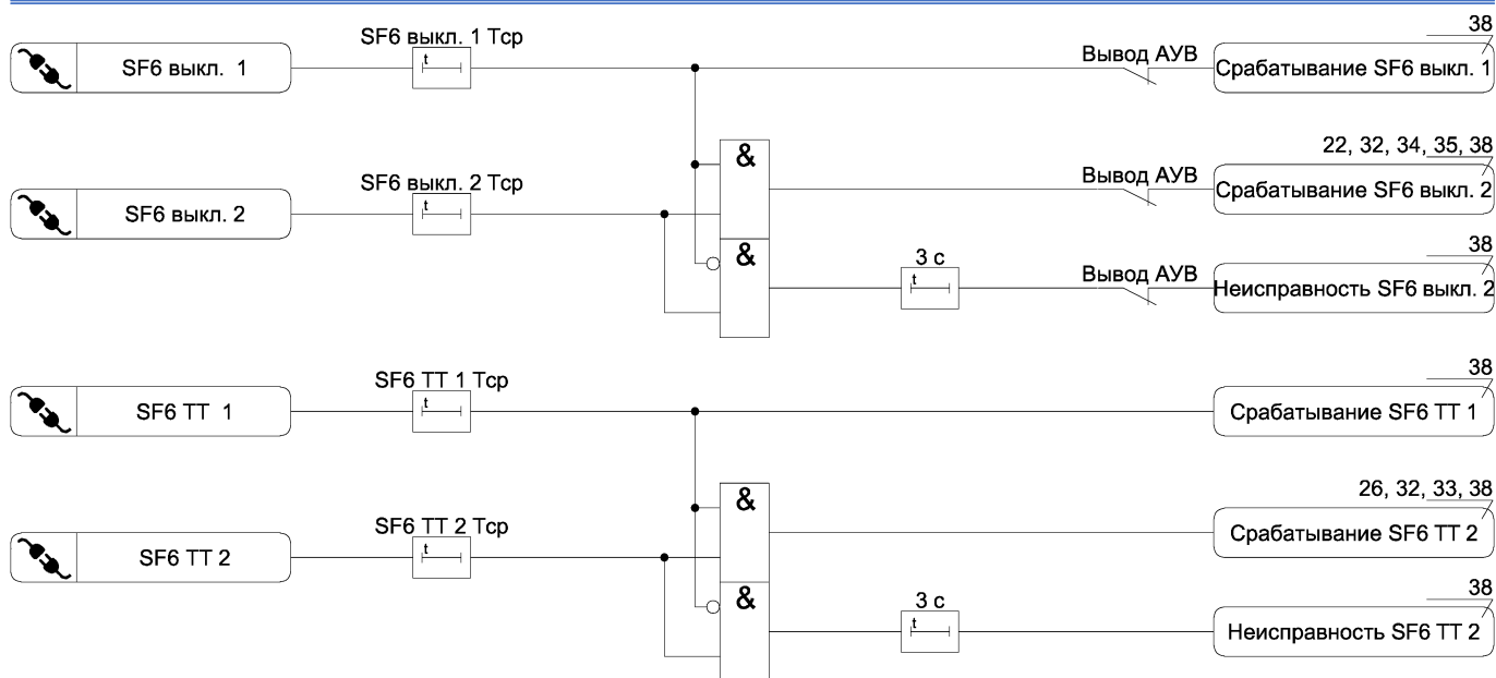
Рисунок А.30 – Функциональная схема алгоритма защиты от снижения давления элегаза
