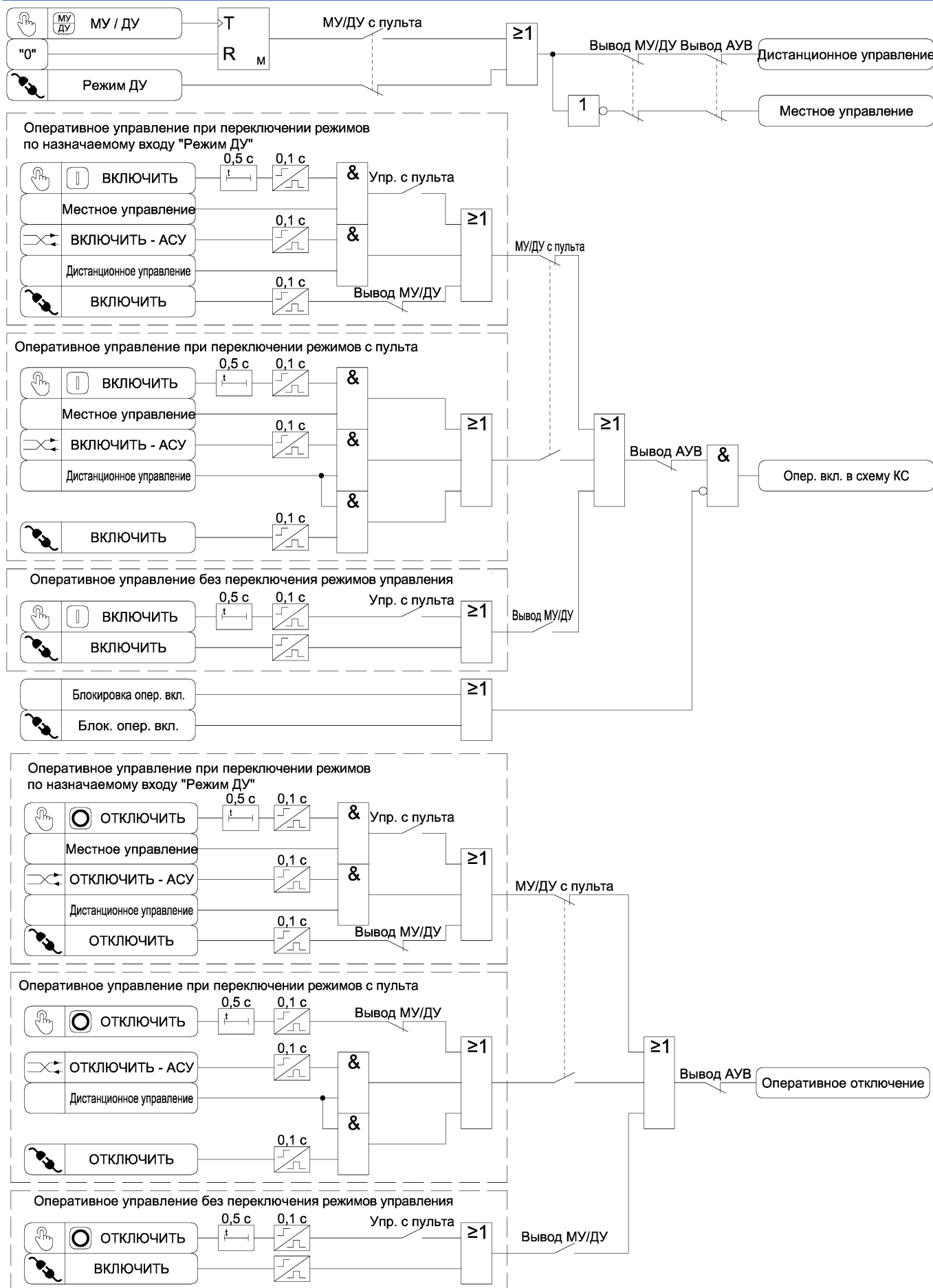
Рисунок 3.40 а) – Функциональная схема алгоритма оперативного управления выключателем
