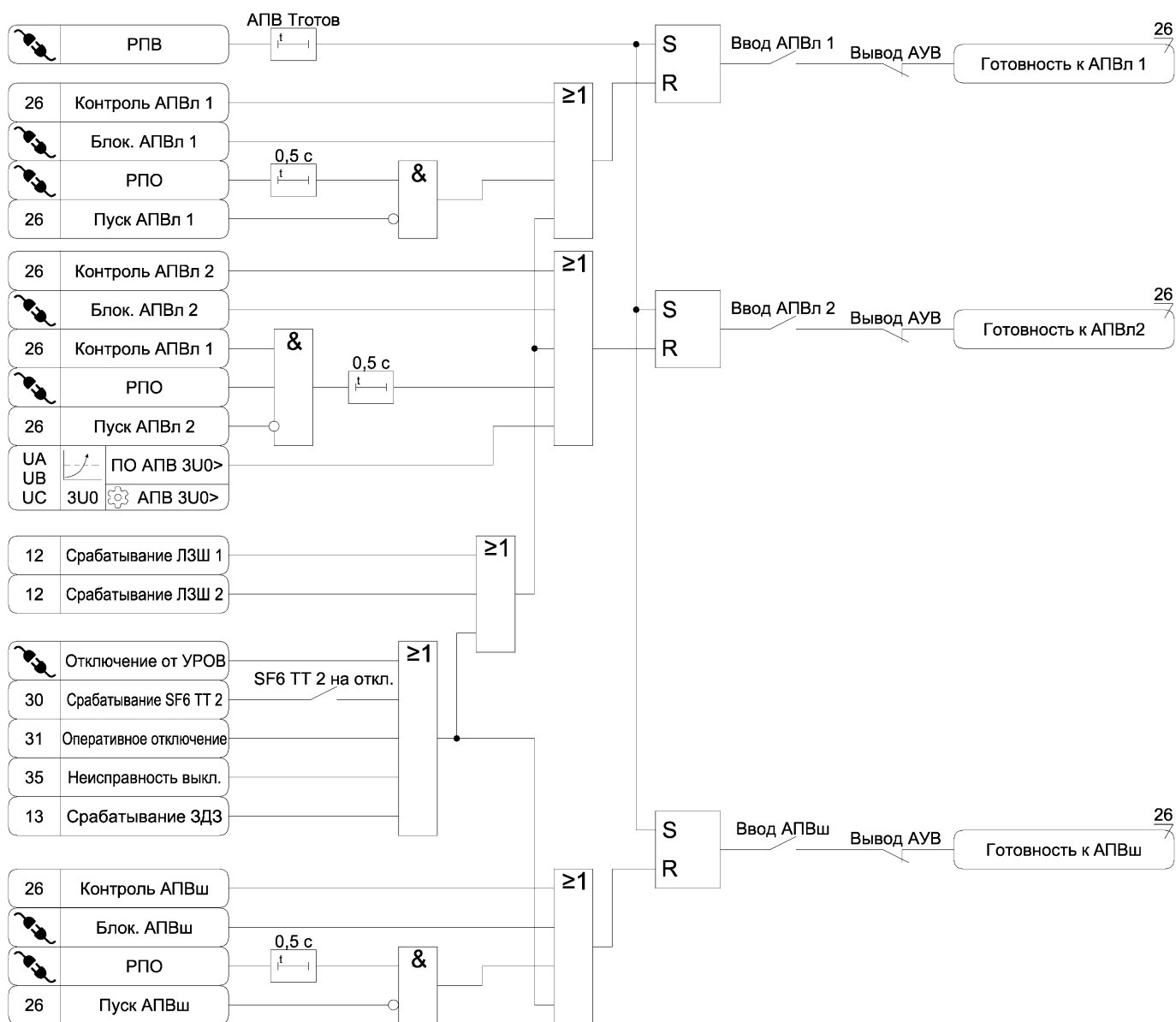
Рисунок А.26 б) – Функциональная схема алгоритма АПУ
