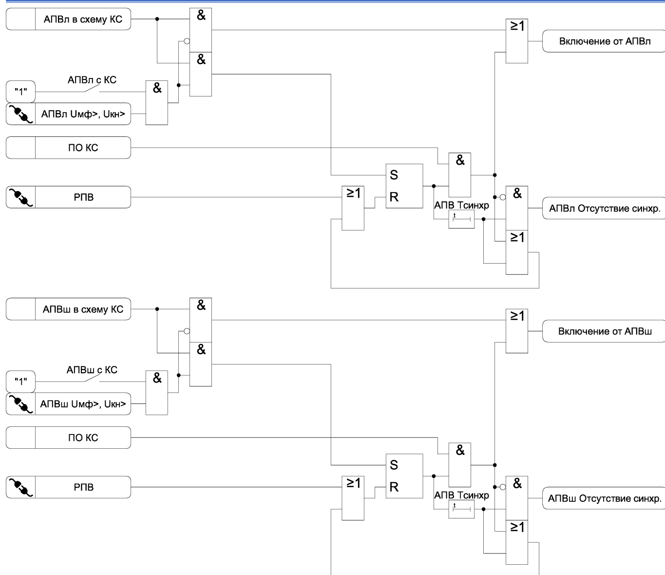
Рисунок 3.35 г) – Функциональная схема алгоритма АПУ
