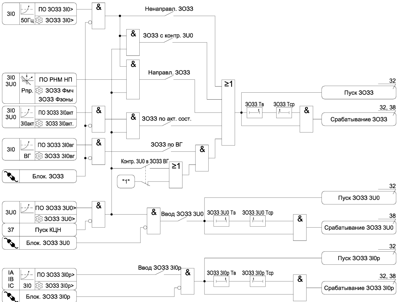
Рисунок А.14 – Функциональная схема алгоритма 3033
