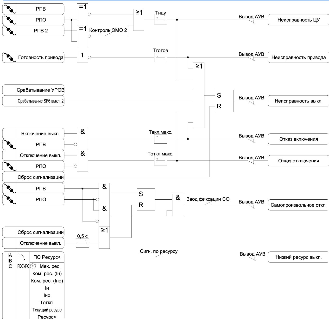
Рисунок 3.16 – Функциональная схема алгоритма диагностики выключателя
