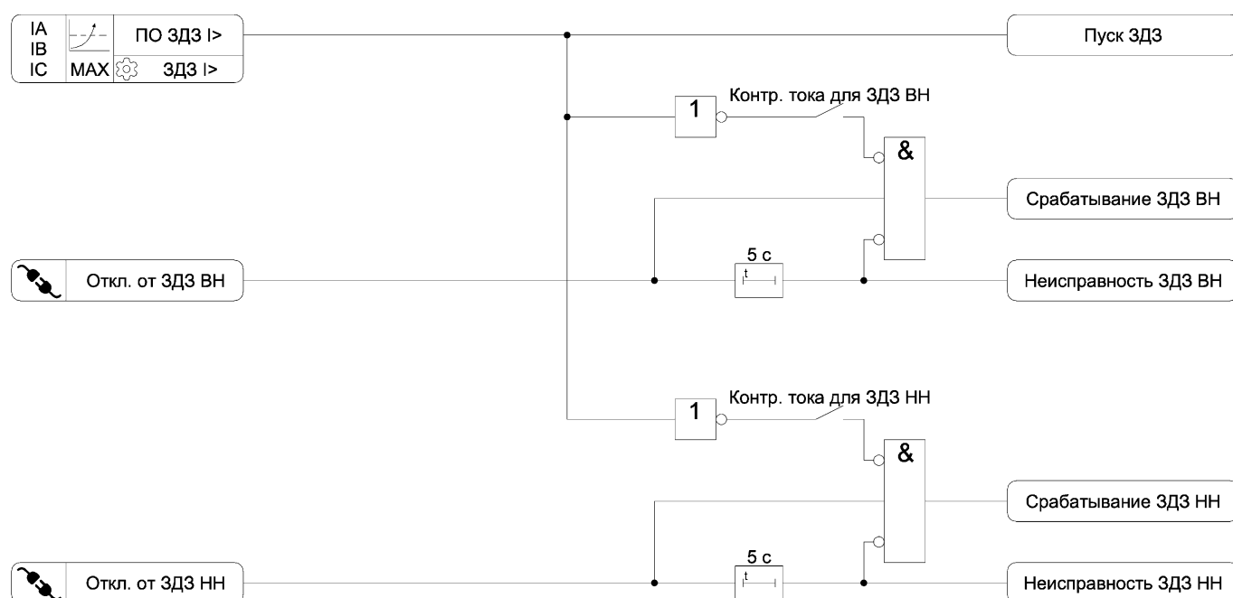
Рисунок 3.6 – Функциональная схема алгоритма ЗДЗ
