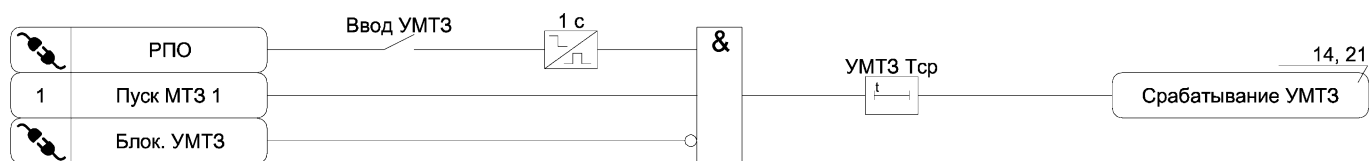
Рисунок А.2 – Функциональная схема алгоритма УМТЗ
