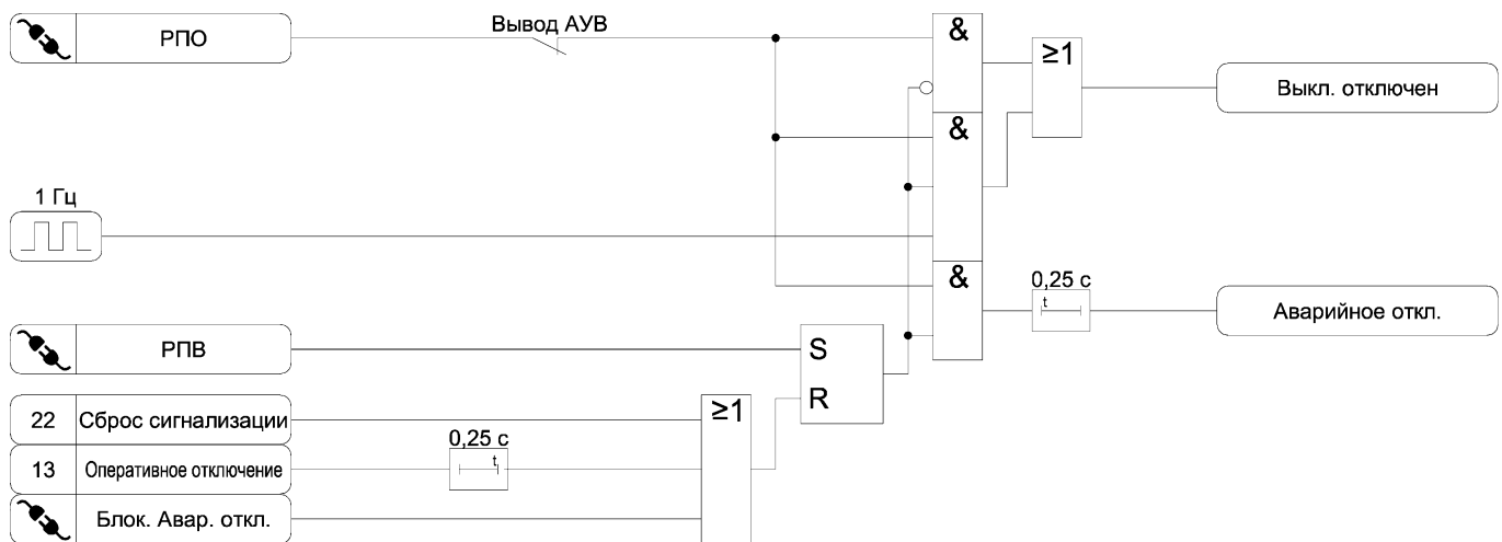
Рисунок А.21 а) – Функциональная схема алгоритма сигнализации
