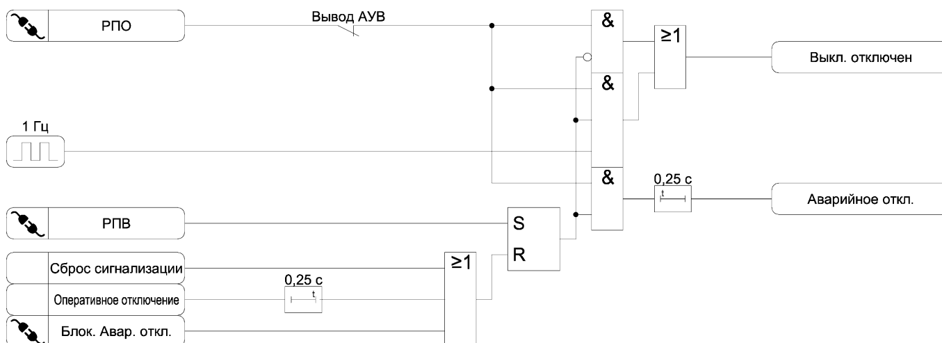
Рисунок 3.20 а)– Функциональная схема алгоритма сигнализации
