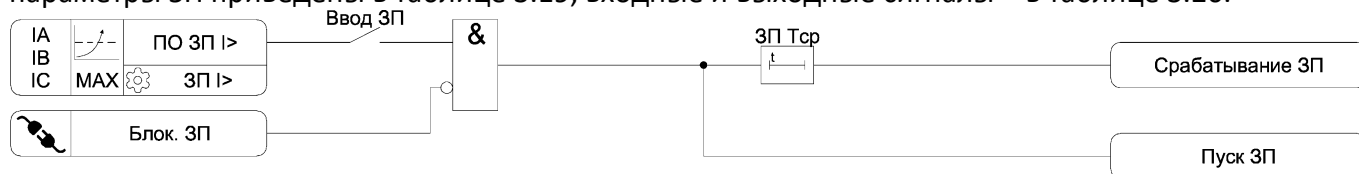
Рисунок 3.11 – Функциональная схема алгоритма ЗП
