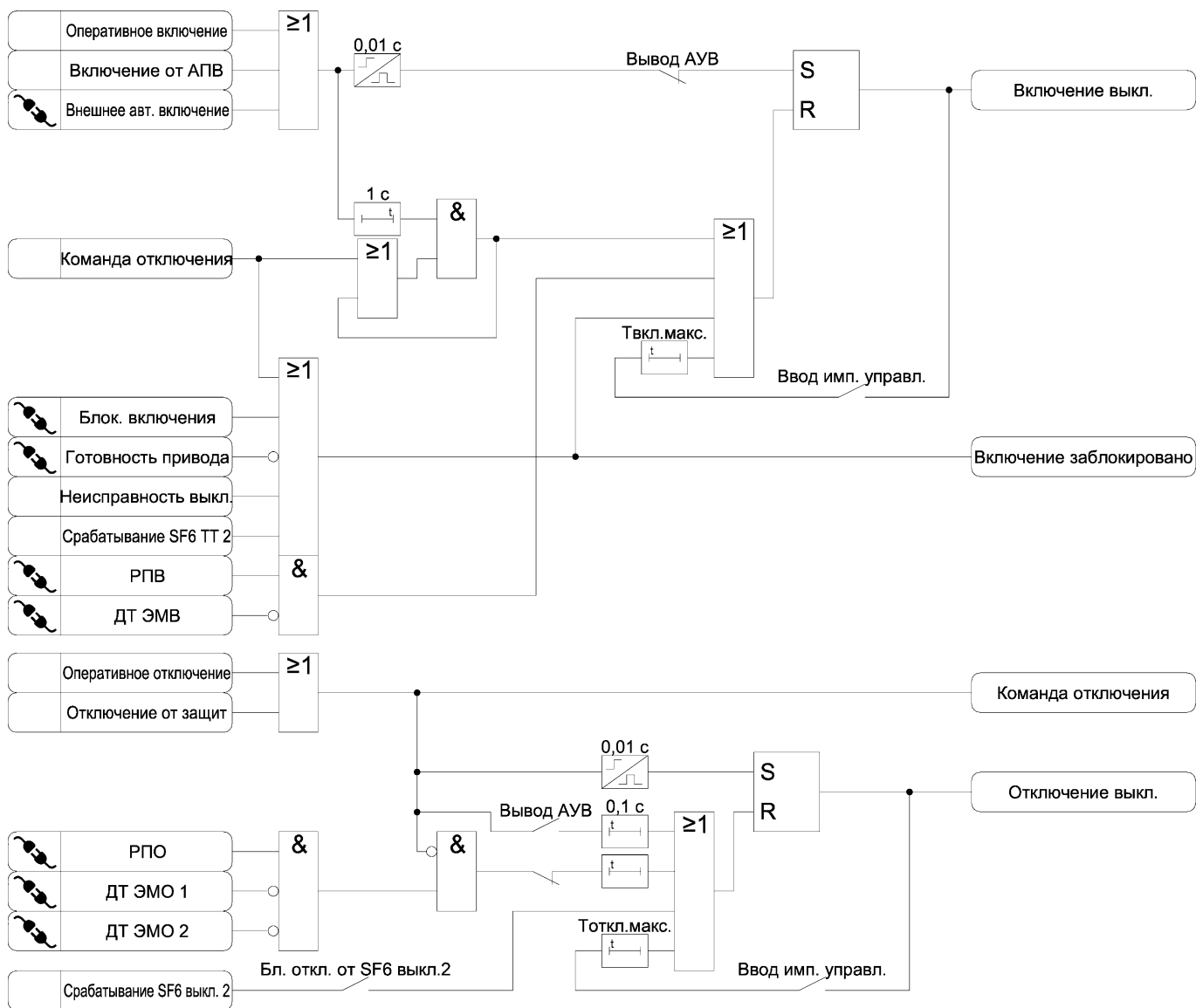
Рисунок 3.15 – Функциональная схема алгоритма управления выключателем
