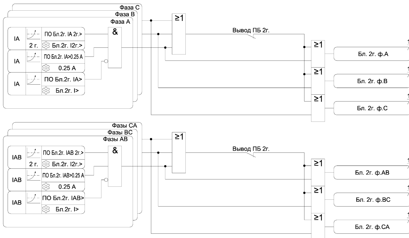
Рисунок А.4 – Функциональная схема алгоритма блокировки по второй гармонике
