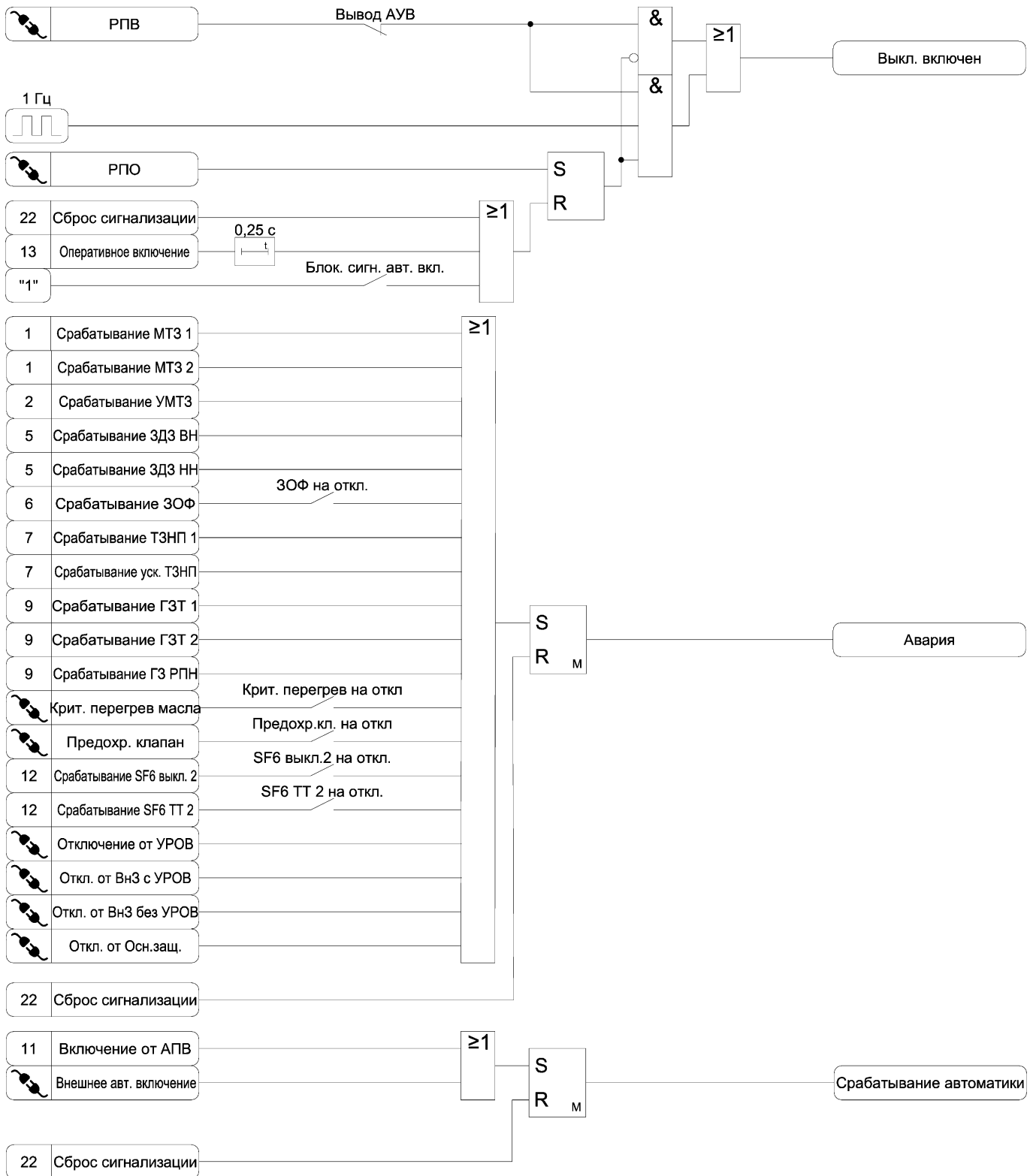
Рисунок А.21 б)– Функциональная схема алгоритма сигнализации
