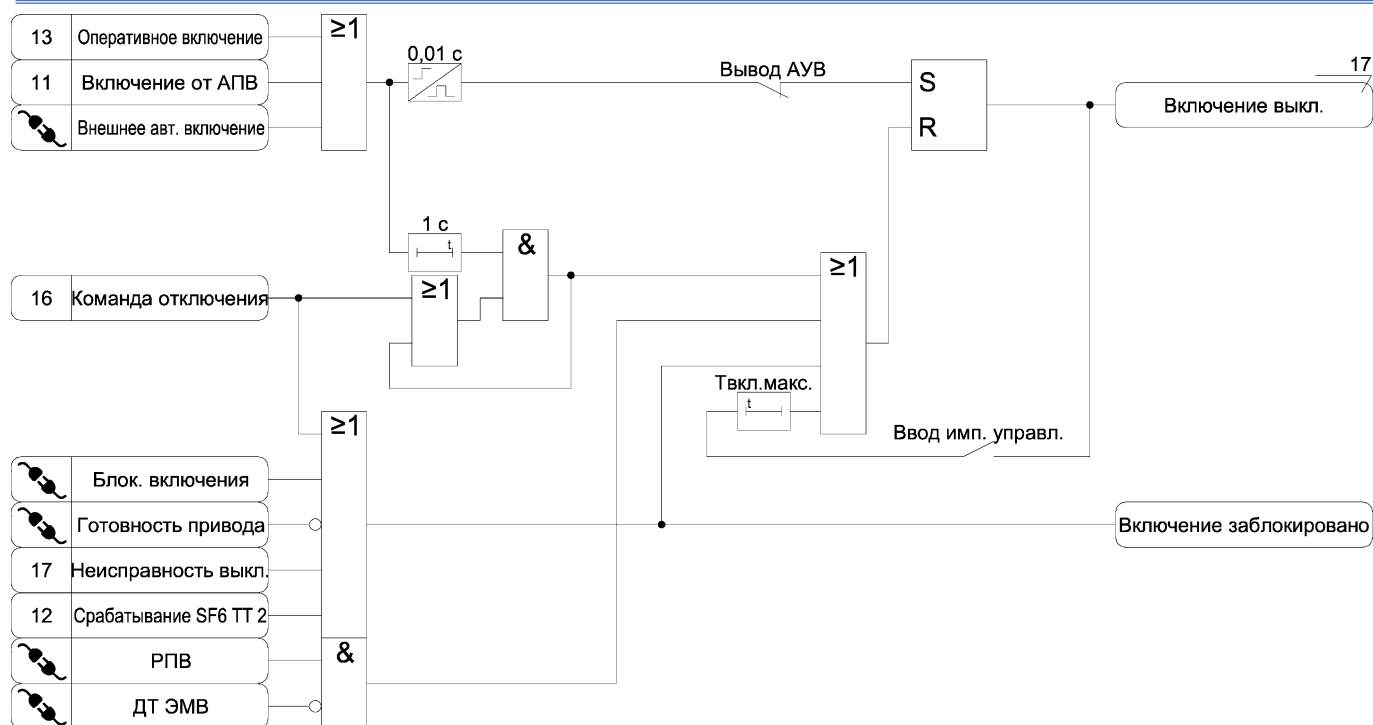
Рисунок А.15 – Функциональная схема алгоритма включения выключателя
