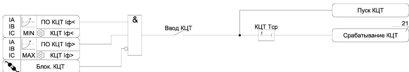
Рисунок А.20 – Функциональная схема алгоритма КЦТ
