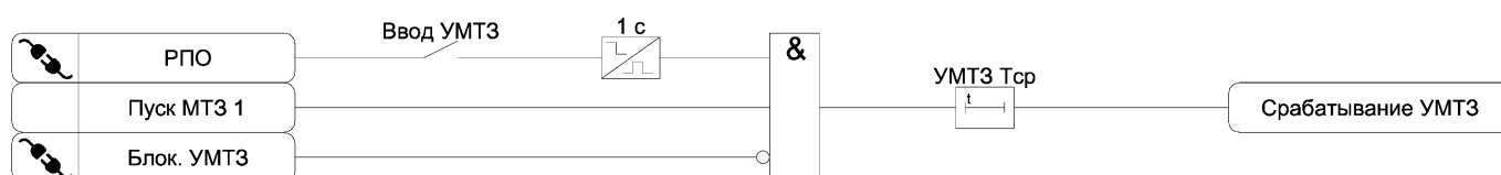
Рисунок 3.2 – Функциональная схема алгоритма УМТЗ
