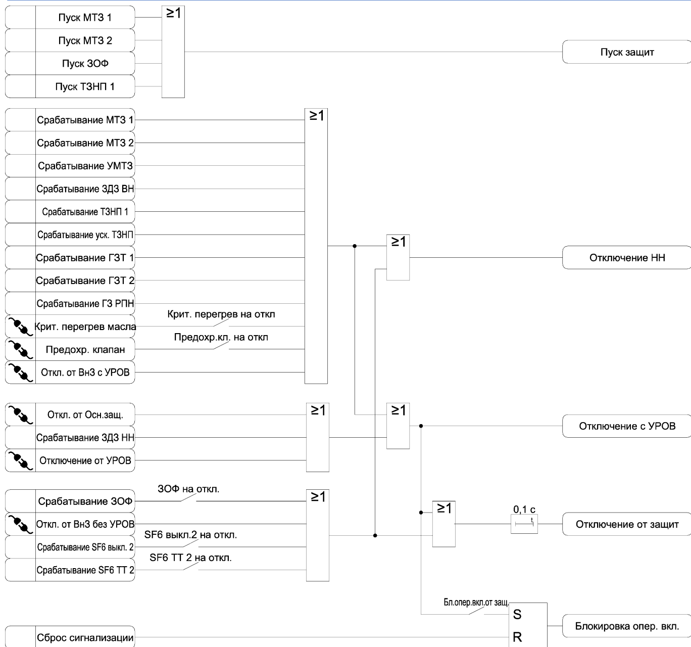
Рисунок 3.14 – Функциональная схема алгоритма формирования сигналов состояния защит
