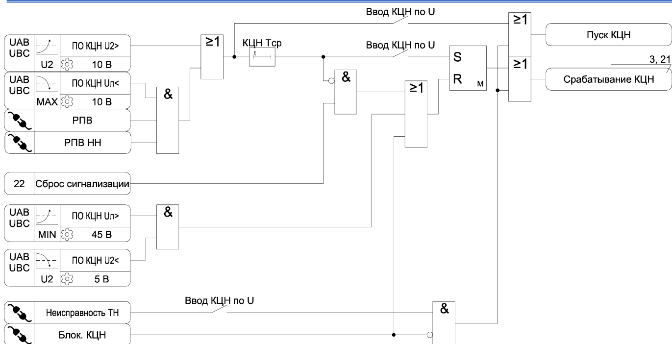
Рисунок А.19 – Функциональная схема алгоритма КЦН
