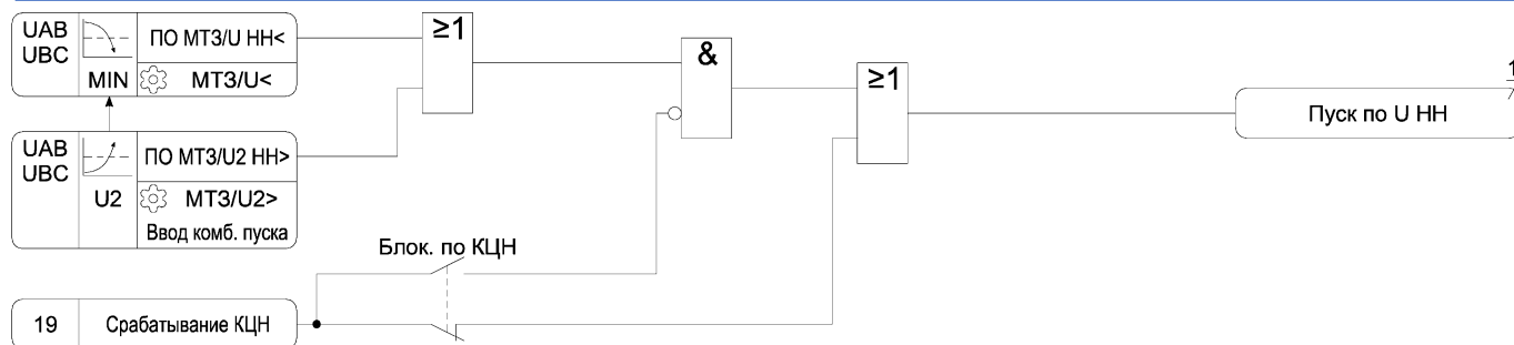
Рисунок А.3 – Функциональная схема алгоритма пуска по напряжению МТЗ
