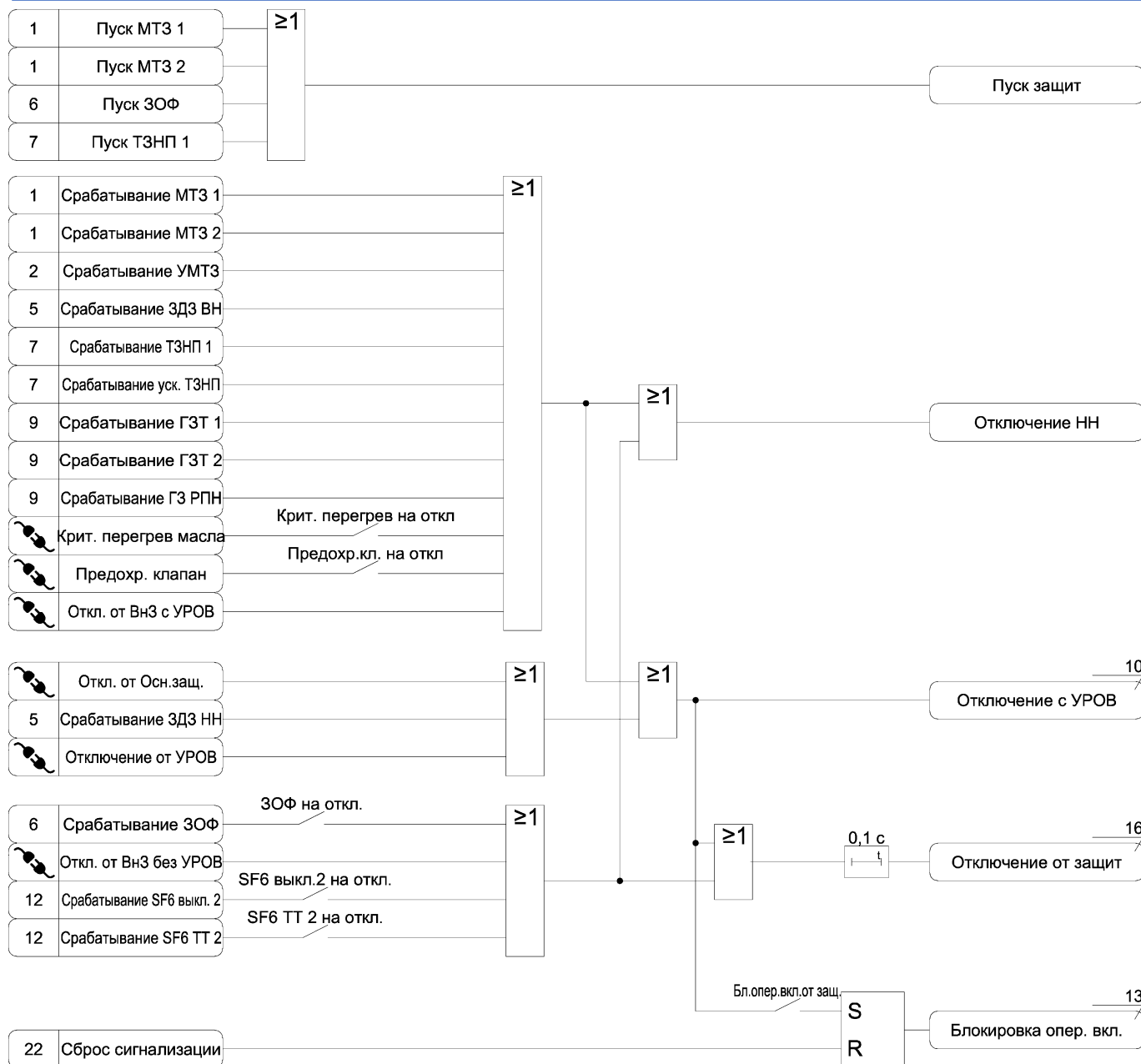
Рисунок А.14 – Функциональная схема алгоритма состояния защит
