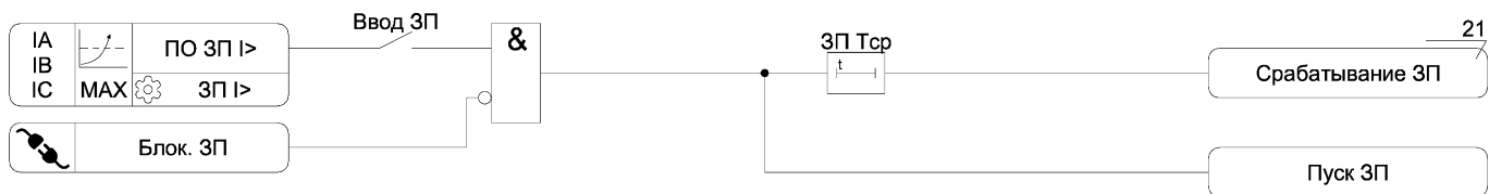
Рисунок А.8– Функциональная схема алгоритма 3П
