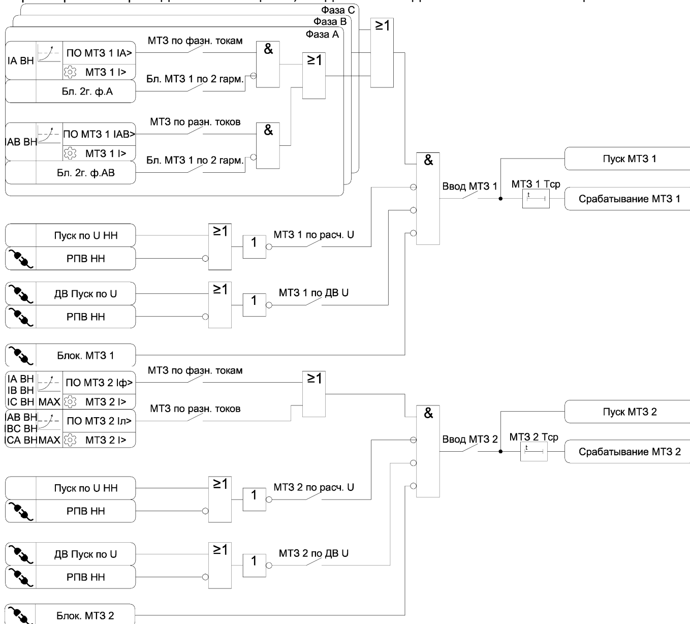
Рисунок 3.1 – Функциональная схема алгоритма МТЗ
