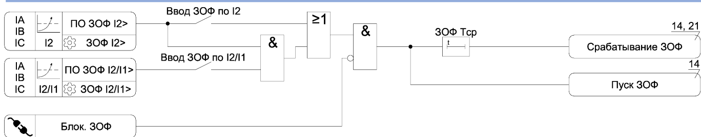
Рисунок А.6– Функциональная схема алгоритма ЗОФ
