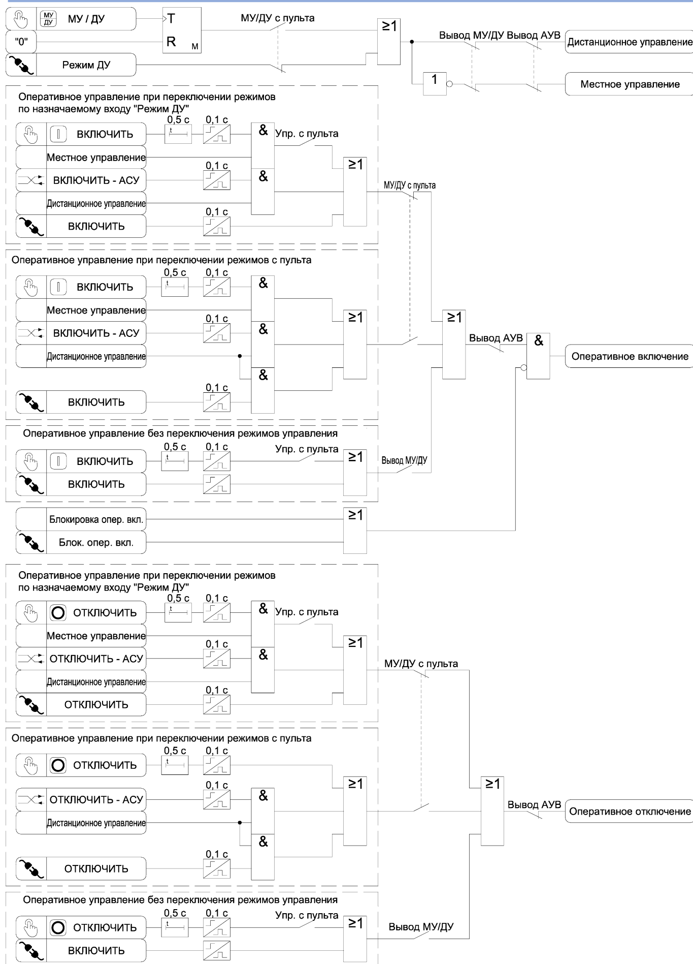
Рисунок 3.12 – Функциональная схема алгоритма оперативного управления выключателем
