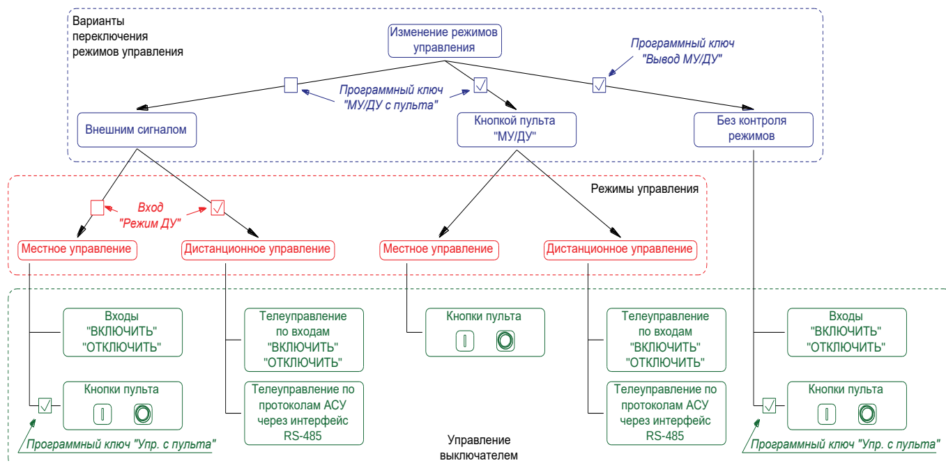
Рисунок 3.13 – Выбор режимов управления
