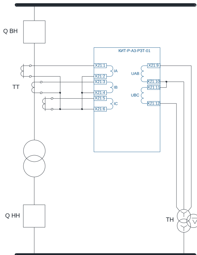
Рисунок 1.1 – Упрощенная схема подключения устройства
