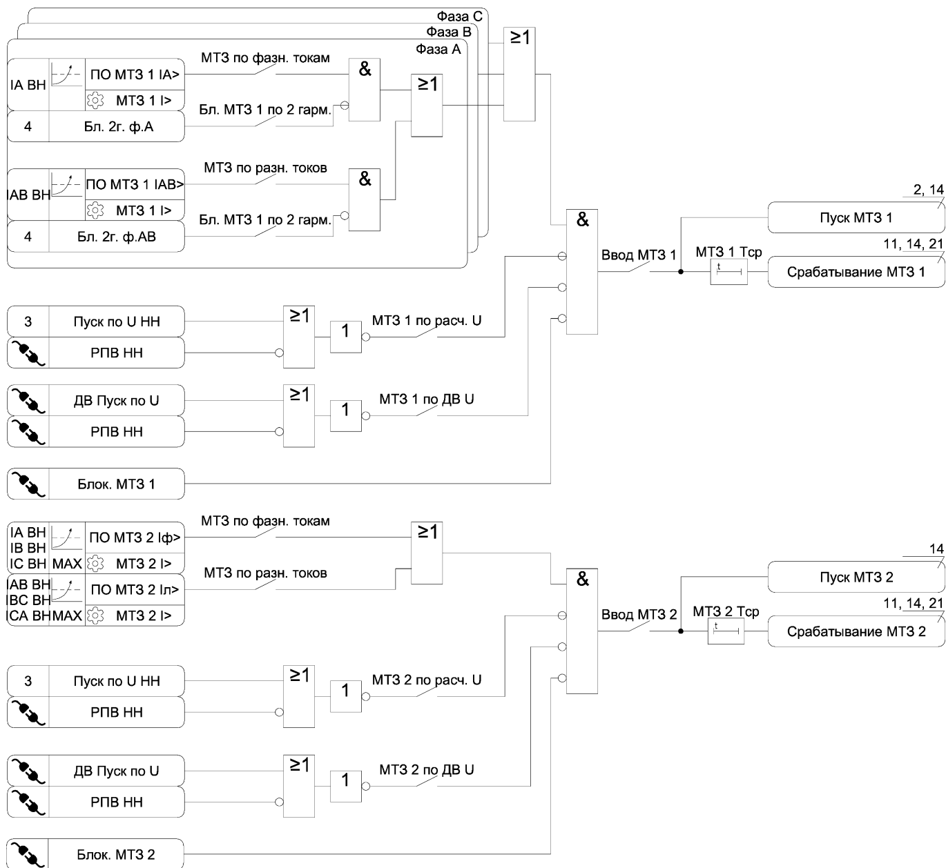
Рисунок А.1 – Функциональная схема алгоритма МТЗ
