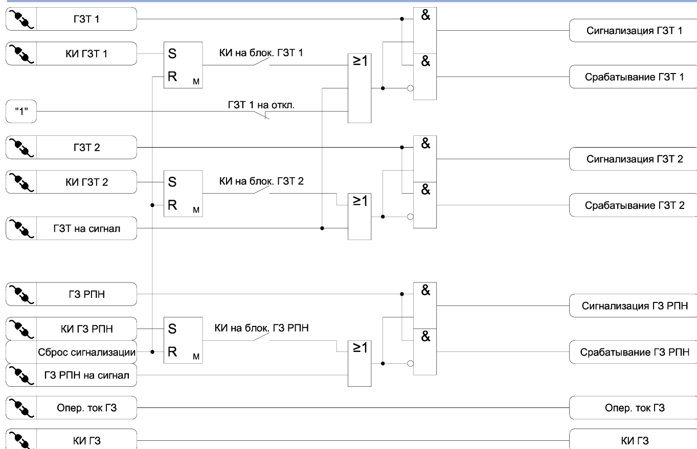
Рисунок 3.8 – Функциональная схема алгоритма ГЗ
