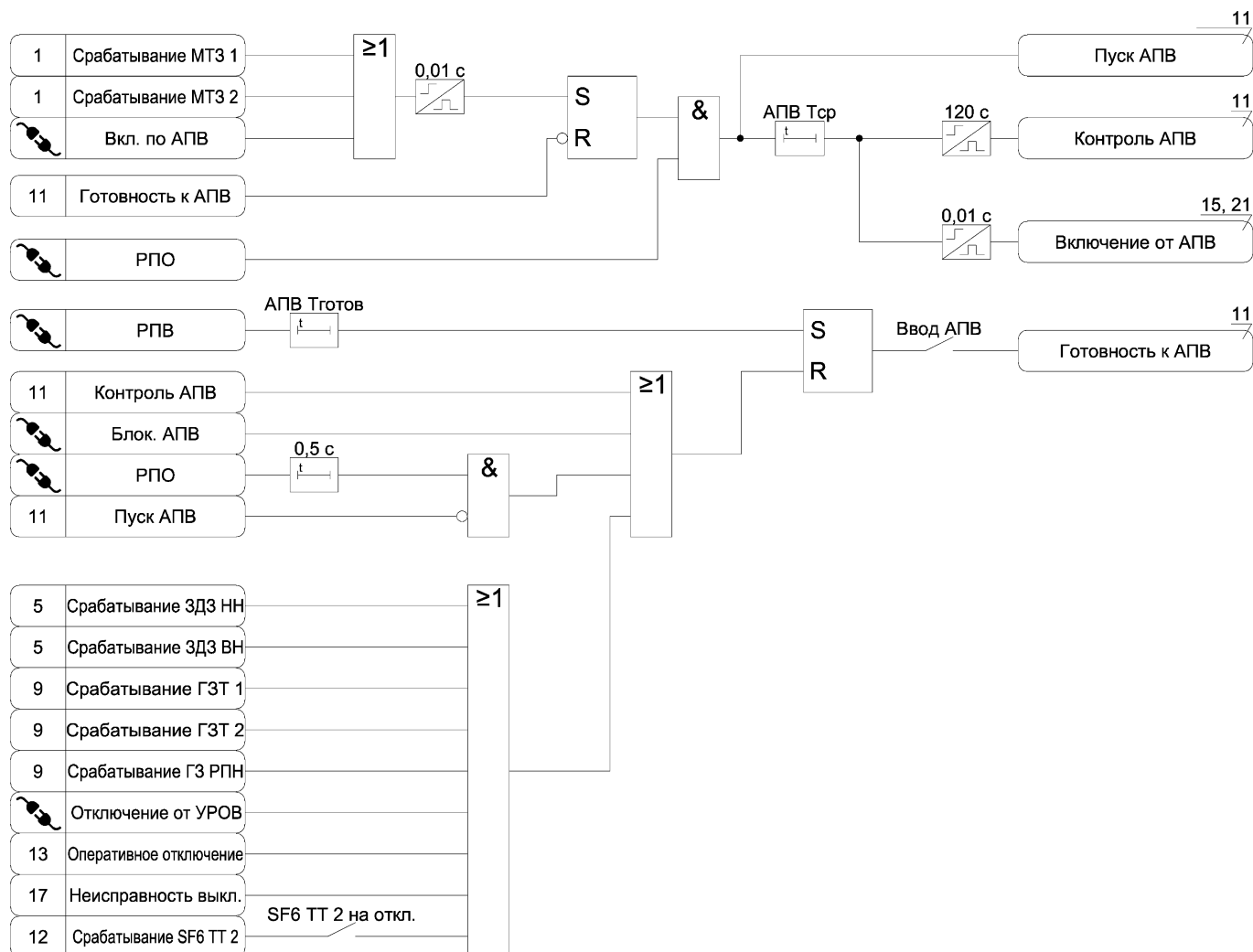
Рисунок А.11 – Функциональная схема алгоритма АПВ
