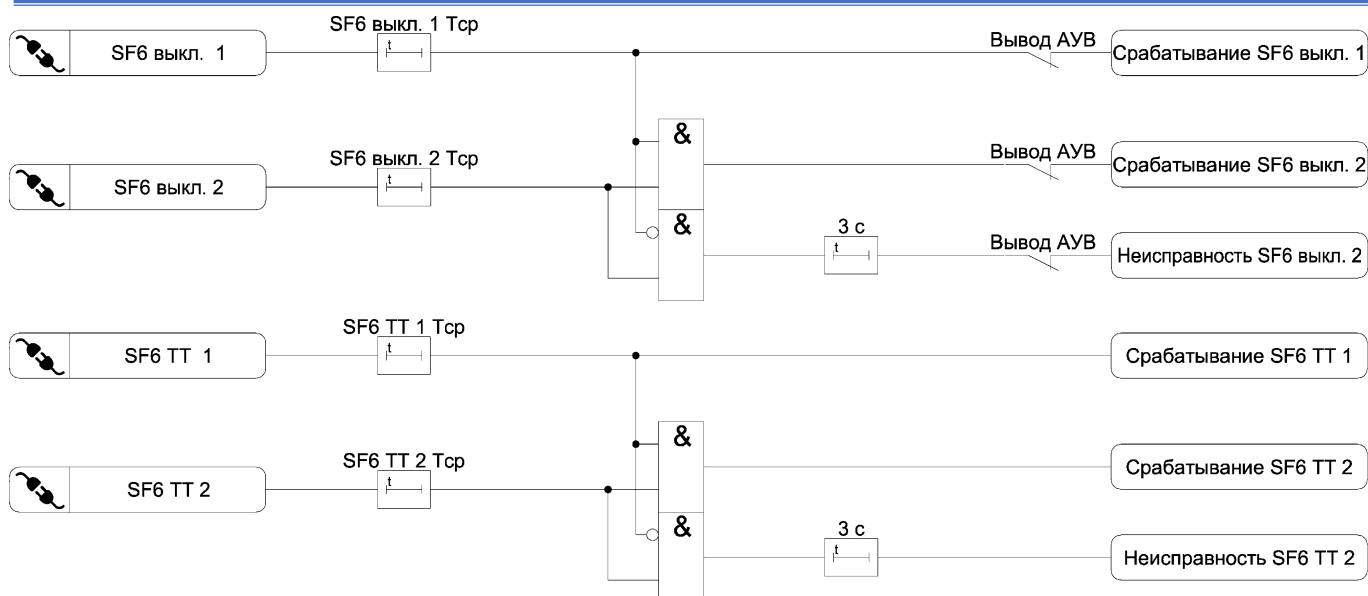
Рисунок 3.11 – Функциональная схема алгоритма защиты от снижения давления элегаза
