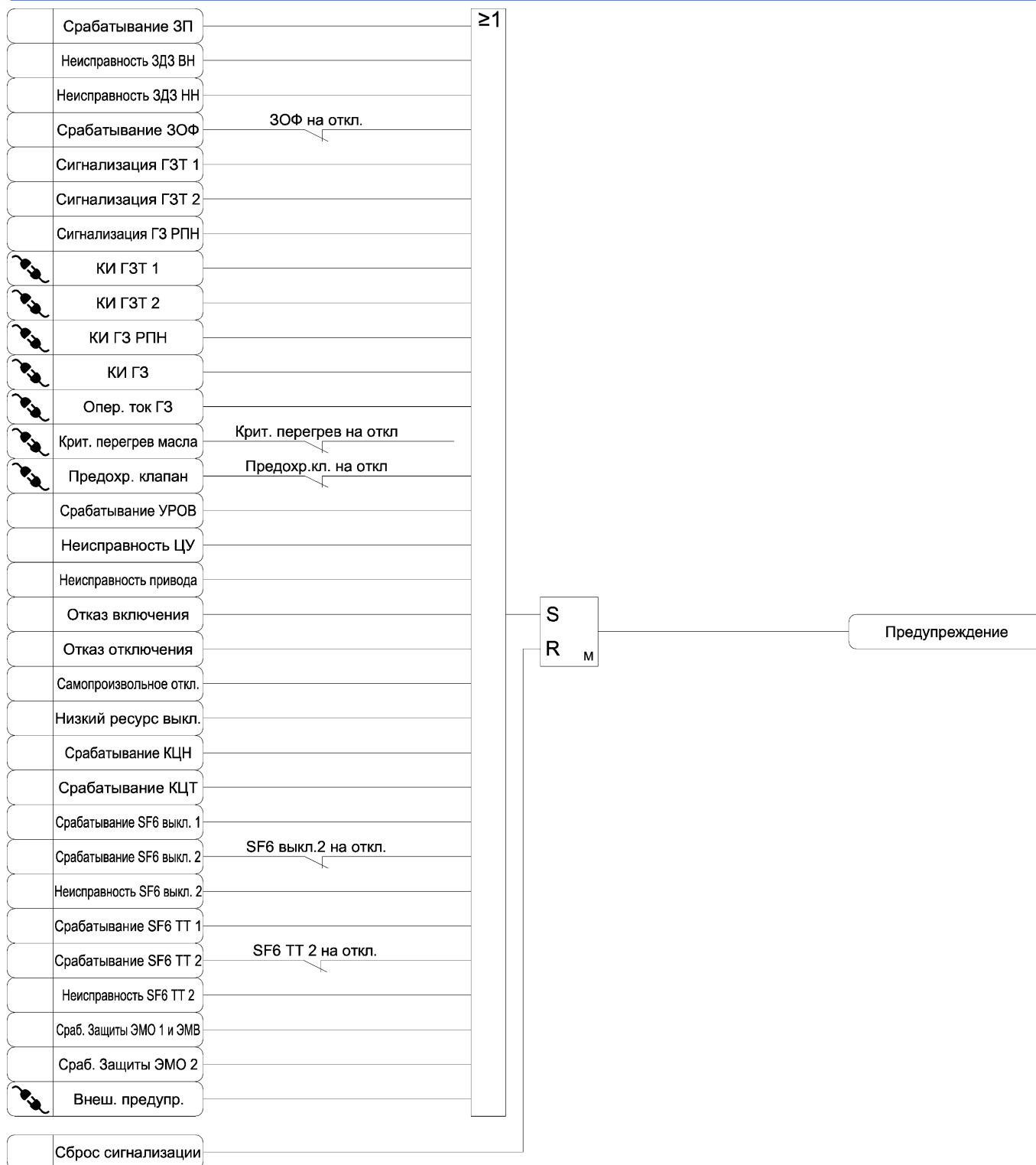
Рисунок 3.20 в) – Функциональная схема алгоритма сигнализации
