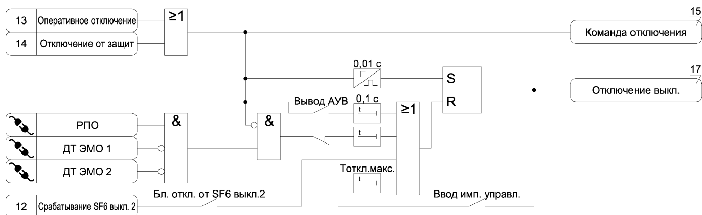
Рисунок А.16 – Функциональная схема алгоритма отключения выключателя
