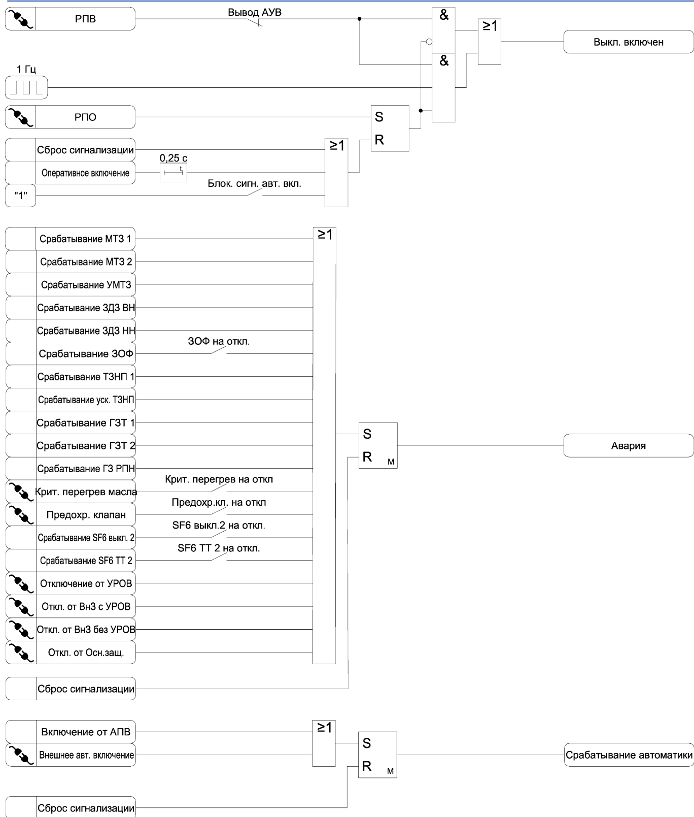
Рисунок 3.20 б) – Функциональная схема алгоритма сигнализации
