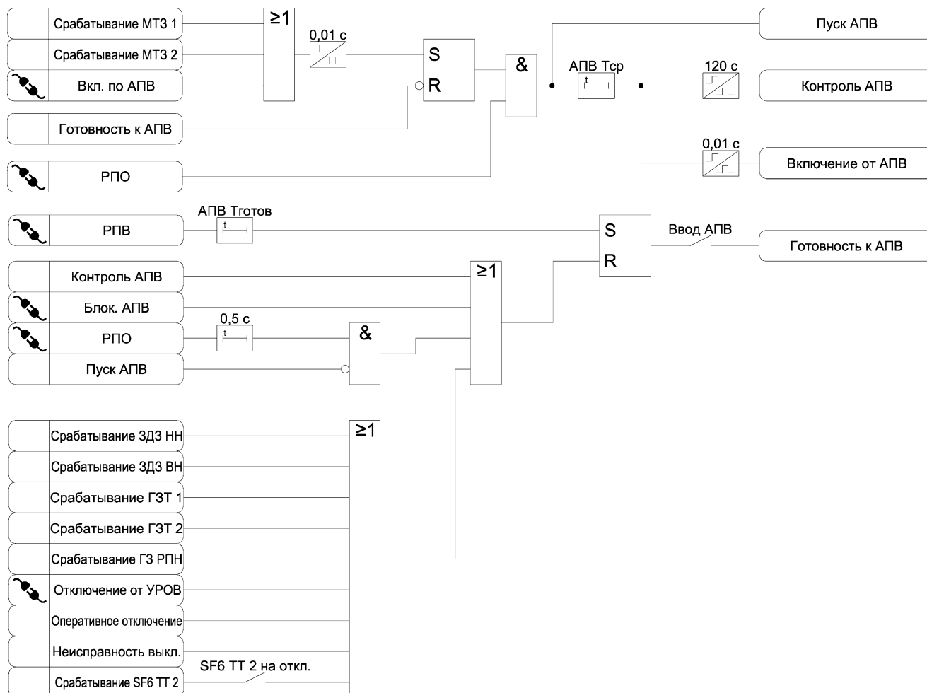
Рисунок 3.10 – Функциональная схема алгоритма АПВ
