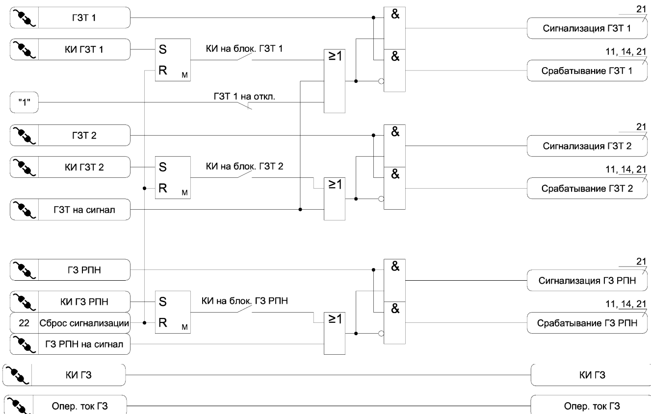
Рисунок А.9– Функциональная схема алгоритма ГЗ
