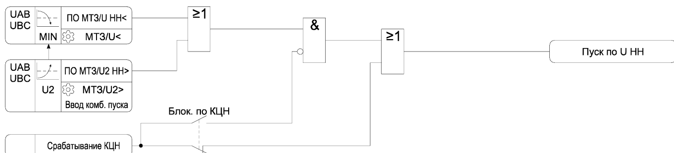
Рисунок 3.3 – Функциональная схема алгоритма МТЗ/У
