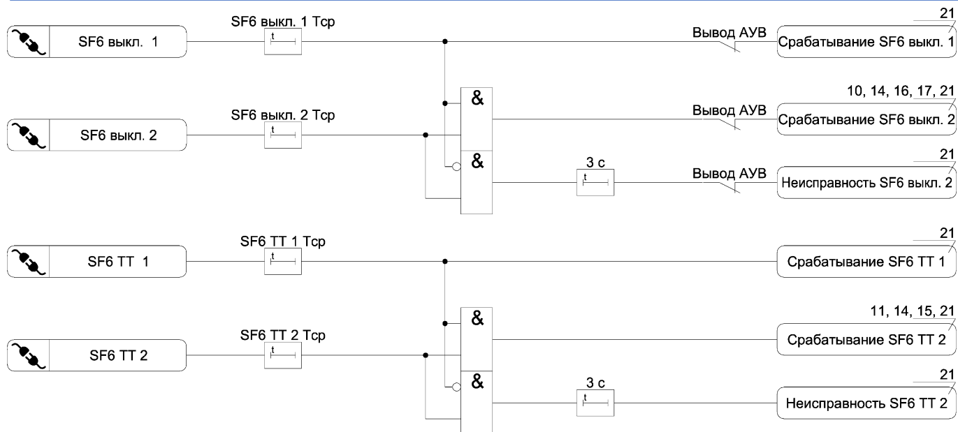
Рисунок А.12 – Функциональная схема алгоритма защиты от снижения давления элегаза
