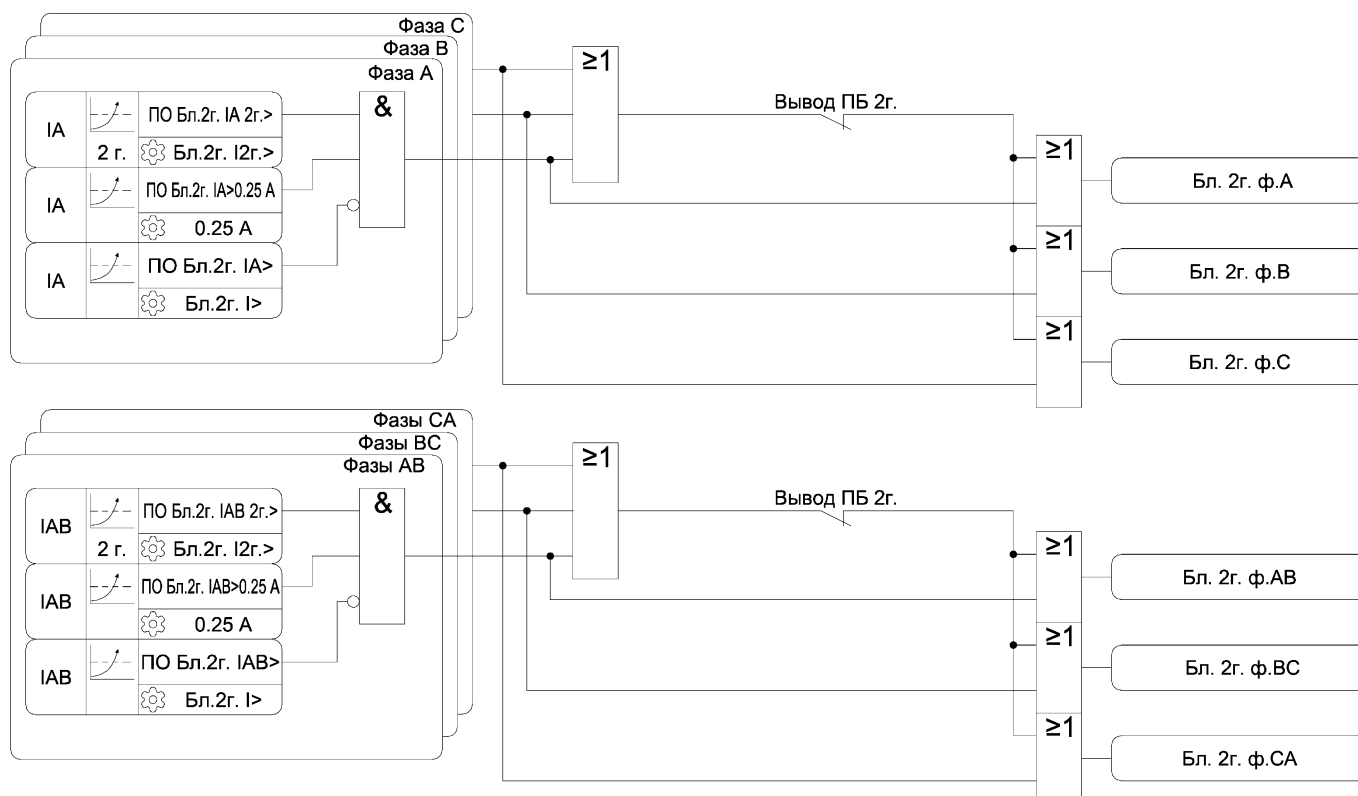
Рисунок 3.4 – Функциональная схема алгоритма МТЗ/У
