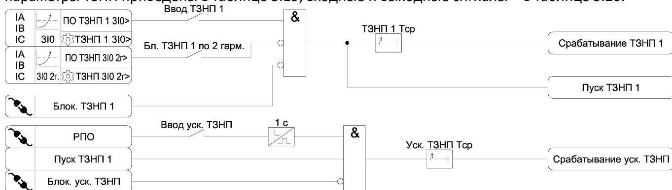
Рисунок 3.11 – Функциональная схема алгоритма ТЗНП
