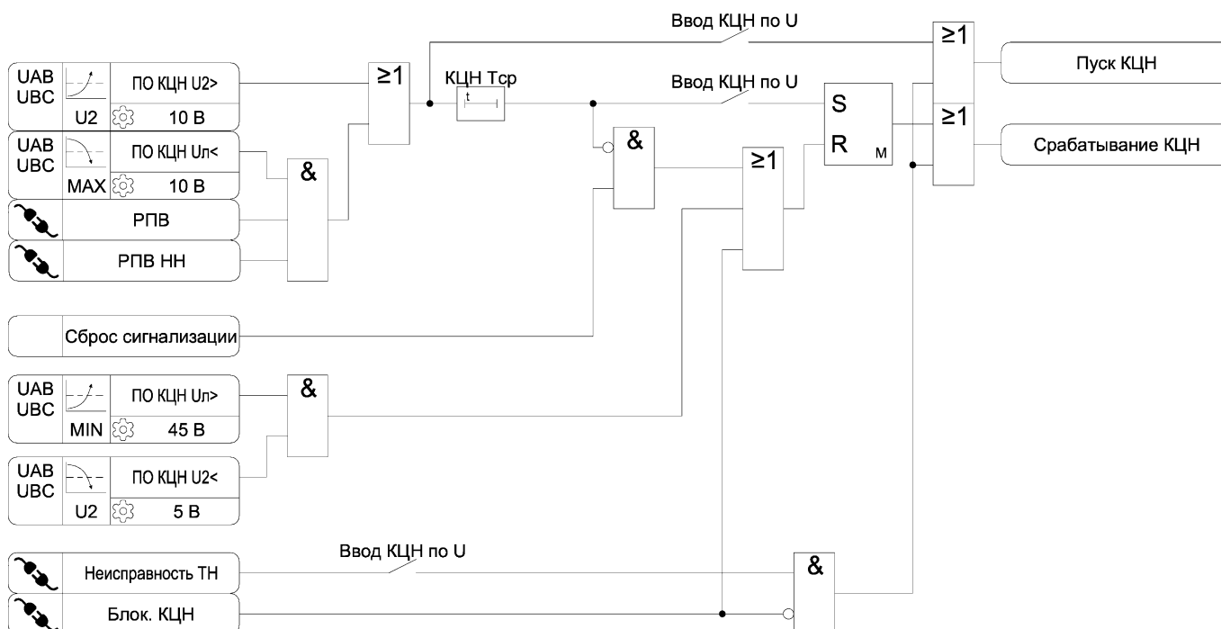
Рисунок 3.18 – Функциональная схема алгоритма КЦН
