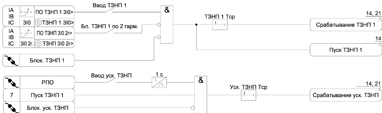
Рисунок А.7– Функциональная схема алгоритма ТЗНП
