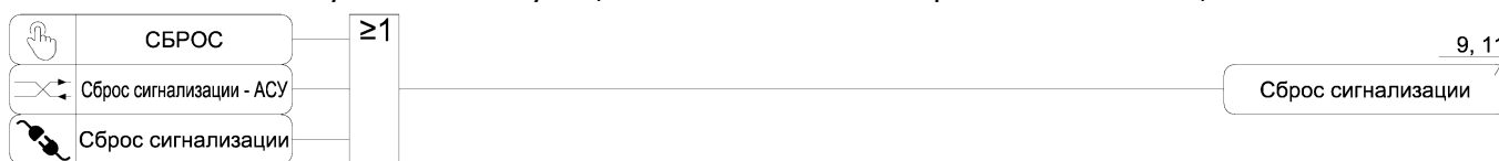
Рисунок А.12 – Функциональная схема алгоритма сброса сигнализации
