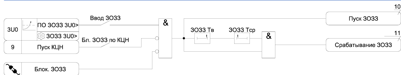
Рисунок А.5 – Функциональная схема алгоритма 3O33
