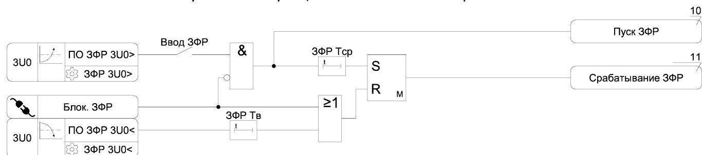
Рисунок А.6 – Функциональная схема алгоритма 3ФР
