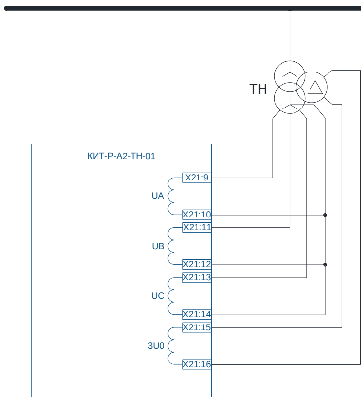
Рисунок 1.1 – Подключение устройства
