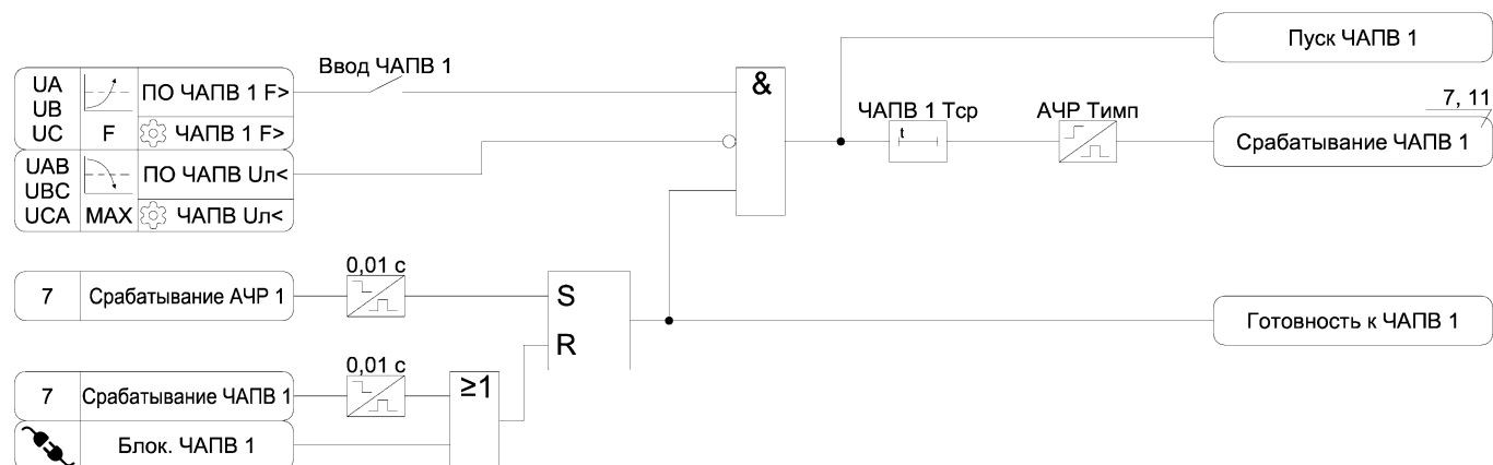
Рисунок А.7 – Функциональные схемы алгоритмов АЧР и АЧПВ
