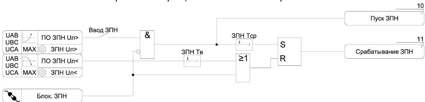
Рисунок А.2 – Функциональная схема алгоритма ЗПН
