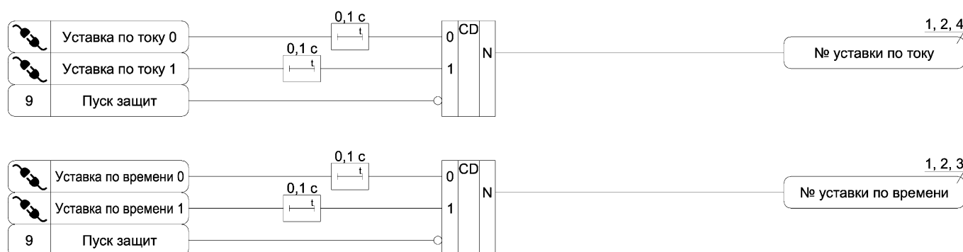
Рисунок А.11 – Функциональная схема алгоритма выбора уставок
