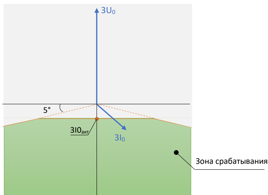
Рисунок 3.14 – Диаграмма срабатывания реле активного тока нулевой последовательности
