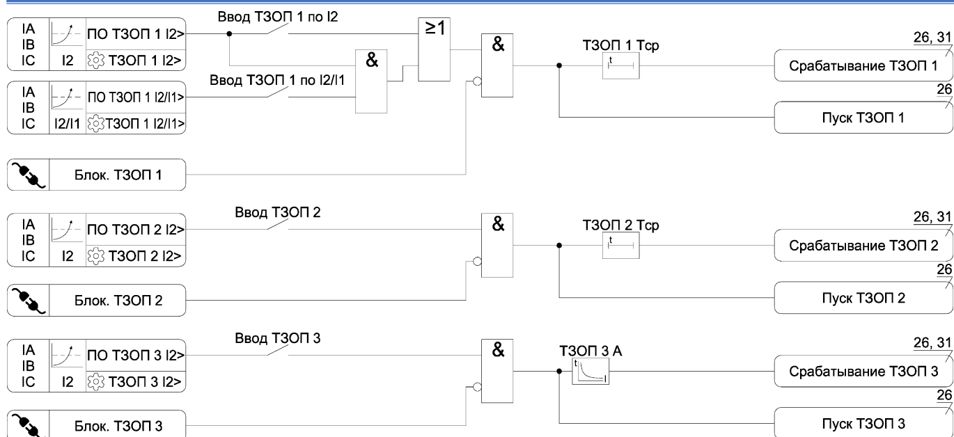
Рисунок А.8 а) – Функциональная схема алгоритма ТЗОП
