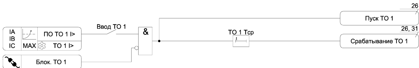
Рисунок А.1 – Функциональная схема алгоритма ТО
