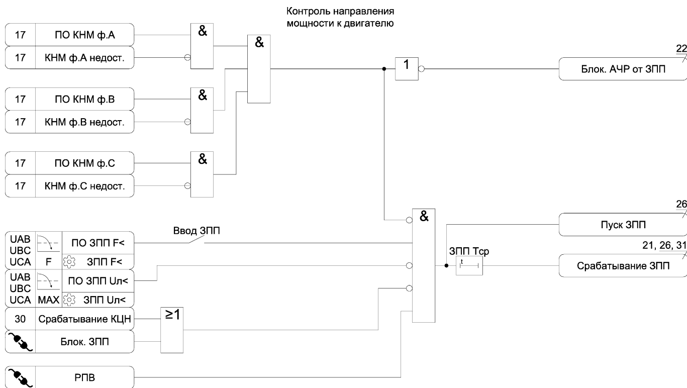
Рисунок А.18 – Функциональная схема алгоритма ЗПП
