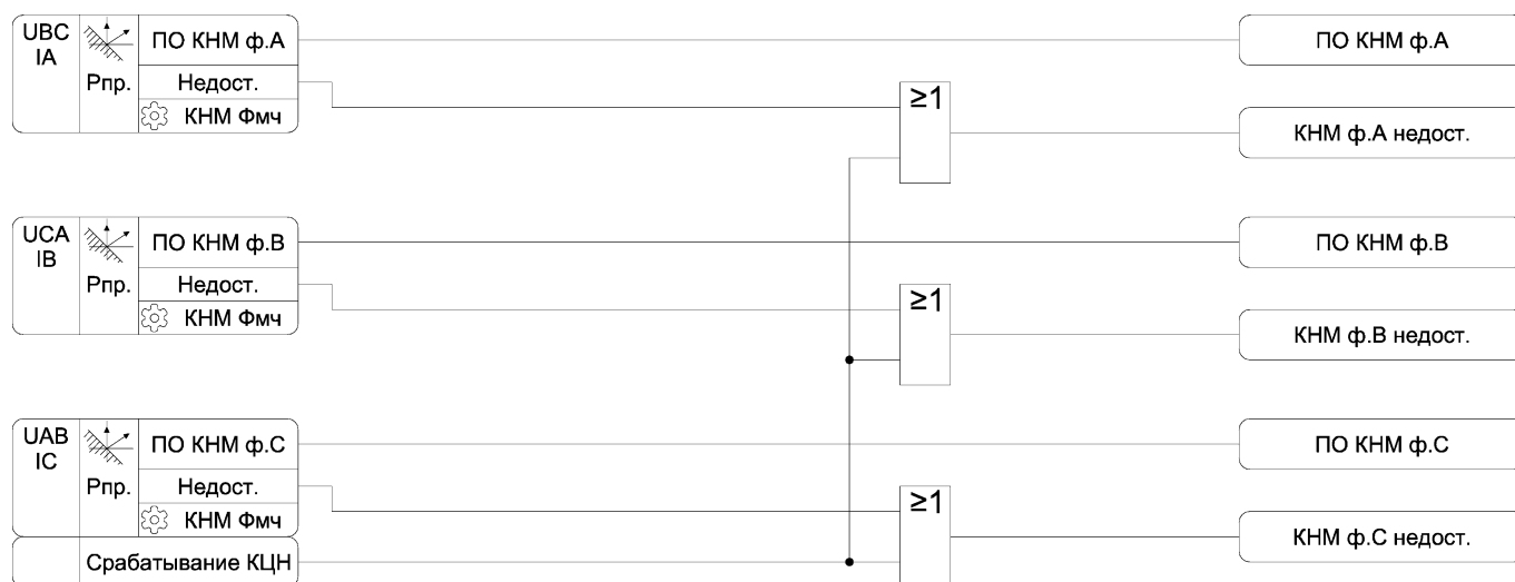
Рисунок 3.23 – Функциональная схема алгоритма КНМ
