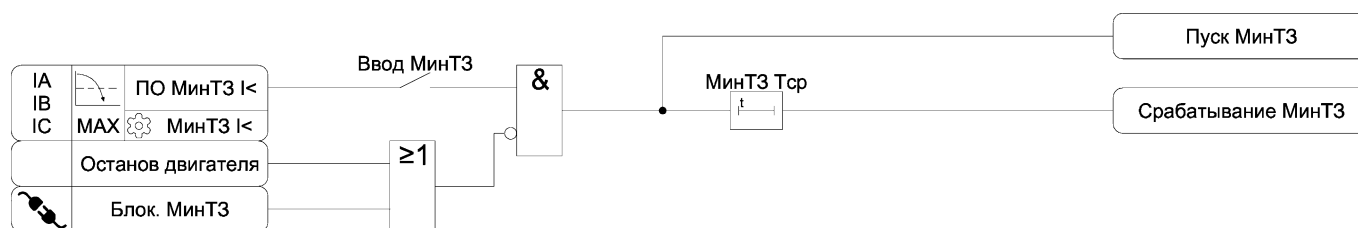
Рисунок 3.10 – Функциональная схема алгоритма МинТЗ
