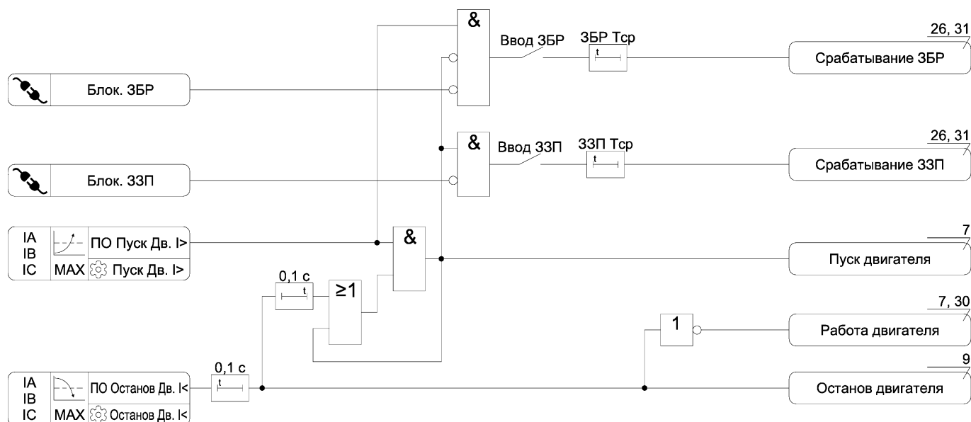
Рисунок А.6 – Функциональная схема алгоритма 33П и 3БП
