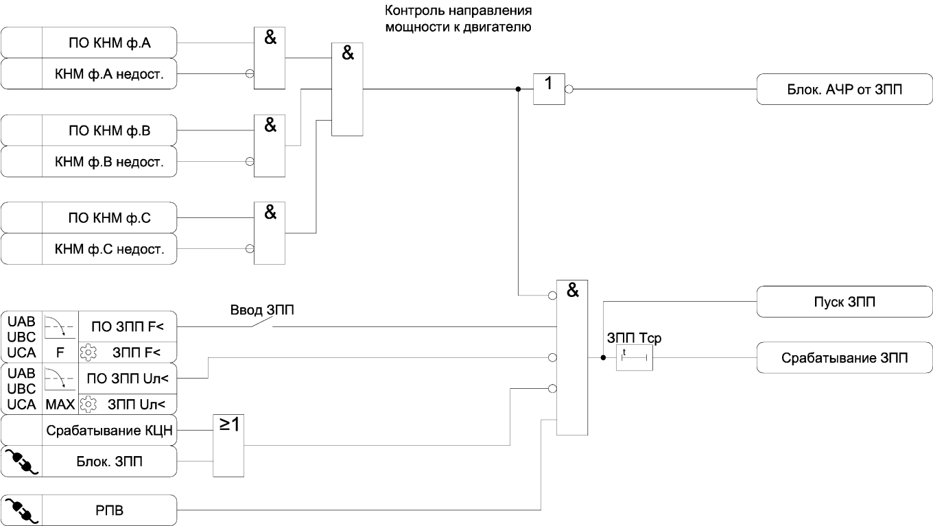
Рисунок 3.25 – Функциональная схема алгоритма ЗПП
