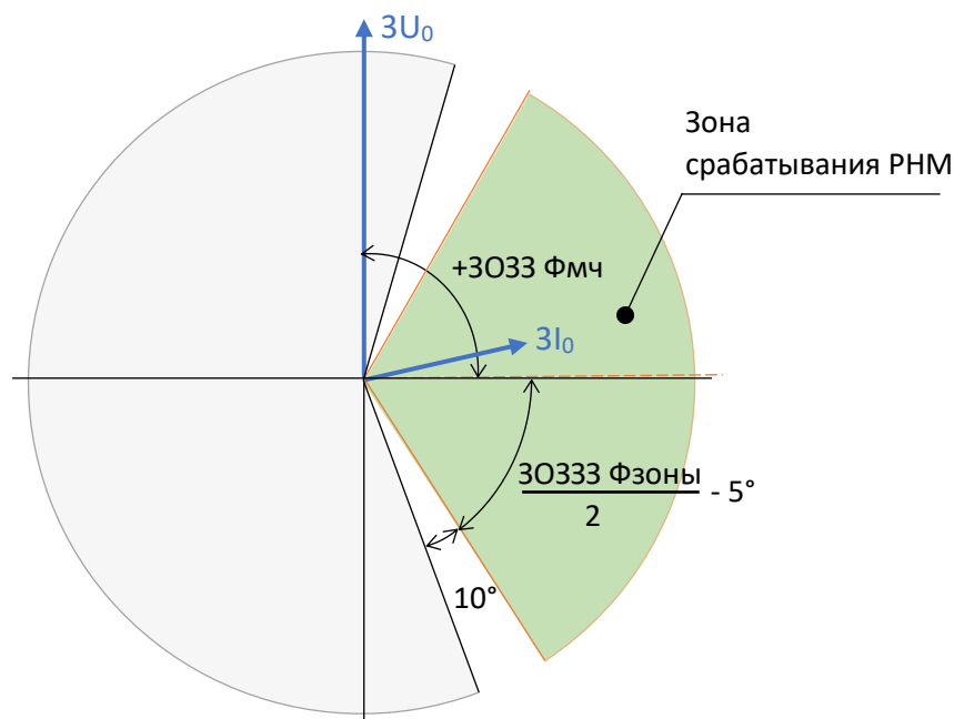
Рисунок 3.13 – Диаграмма срабатывания реле направления мощности нулевой последовательности
