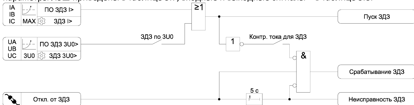
Рисунок 3.4 – Функциональная схема алгоритма ЗДЗ
