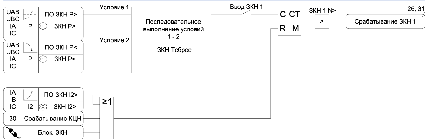
Рисунок А.19 – Функциональная схема алгоритма ЗКН
