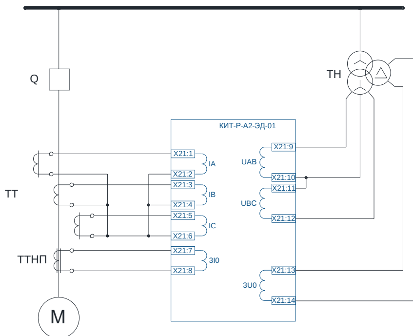
а) схема с тремя ТТ
