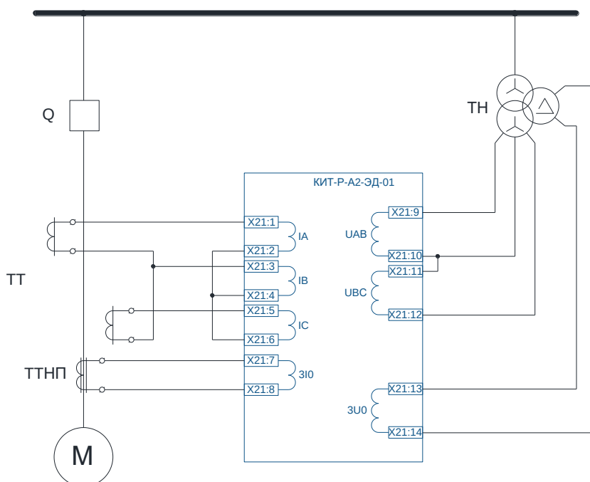
б) схема с двумя ТТ
