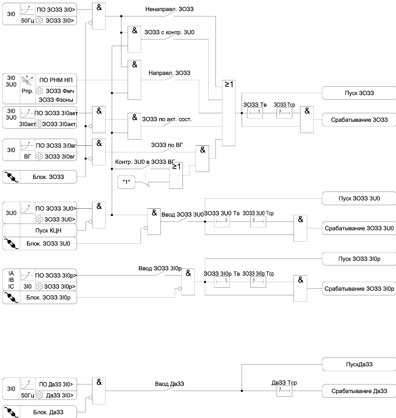
Рисунок 3.12 – Функциональная схема алгоритма ЗОЗЗ
