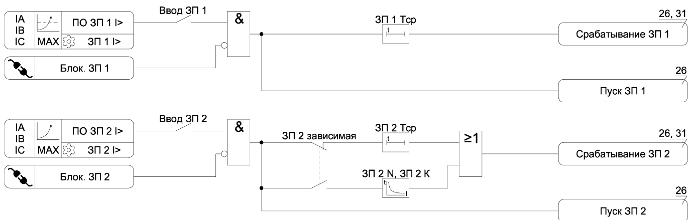
Рисунок А.4 – Функциональная схема алгоритма ЗП
