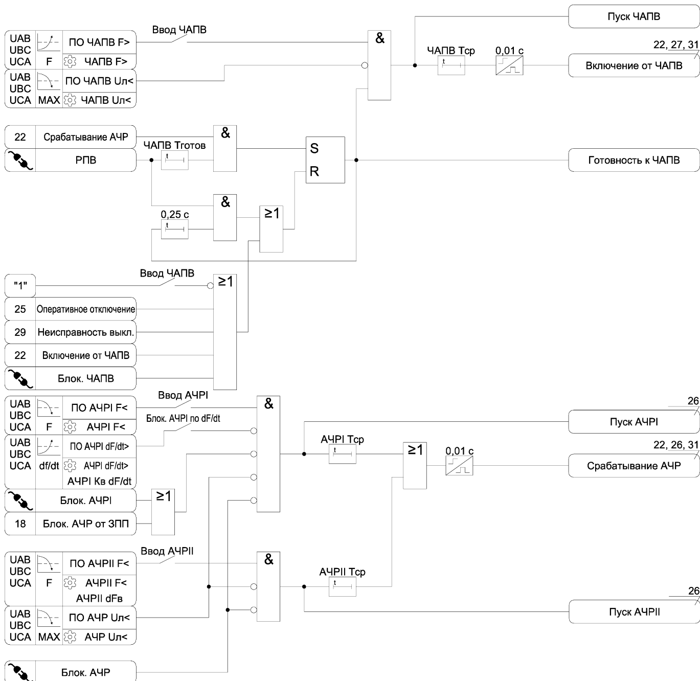
Рисунок А.22 – Функциональная схема алгоритма АЧР и ЧАПВ
