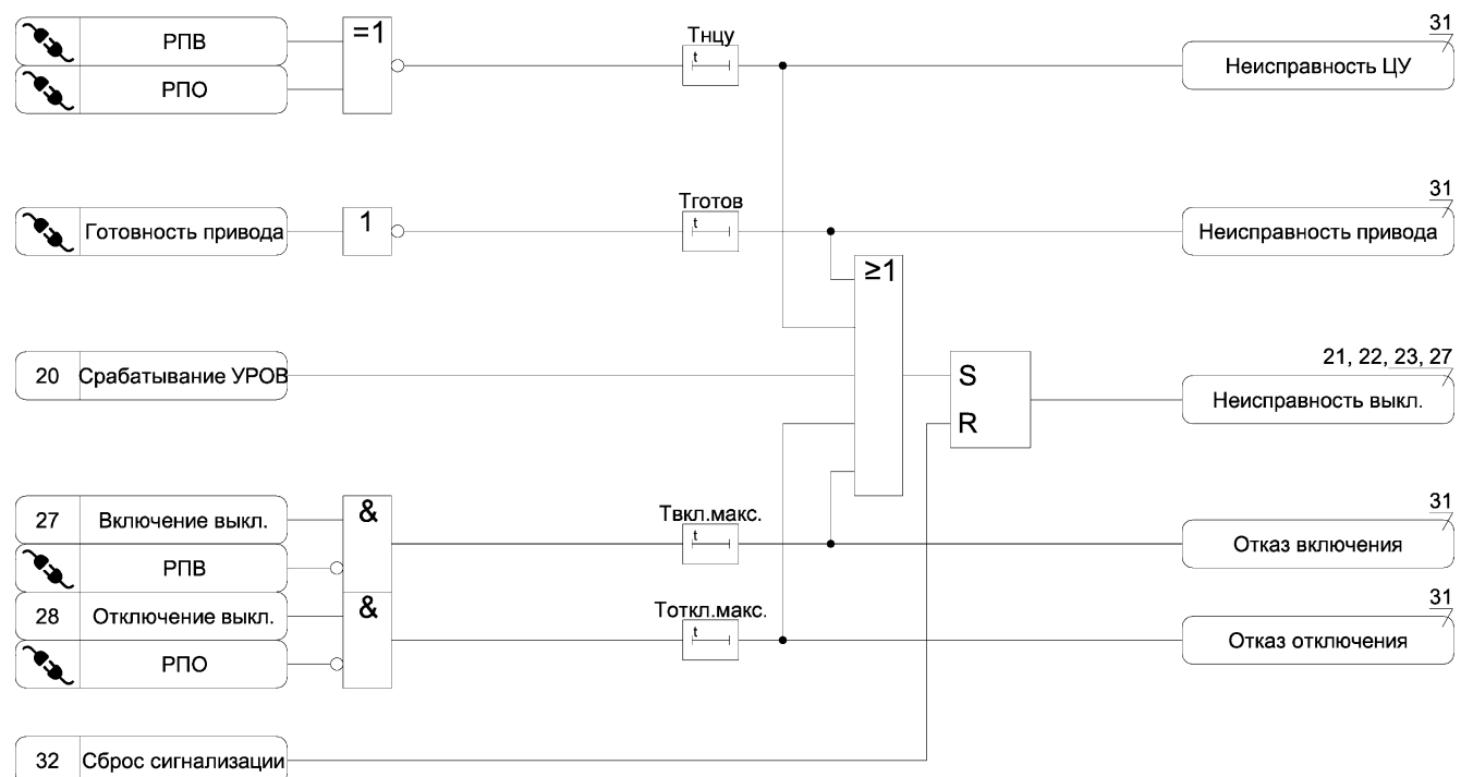
Рисунок А.29 а) – Функциональная схема алгоритма диагностики выключателя
