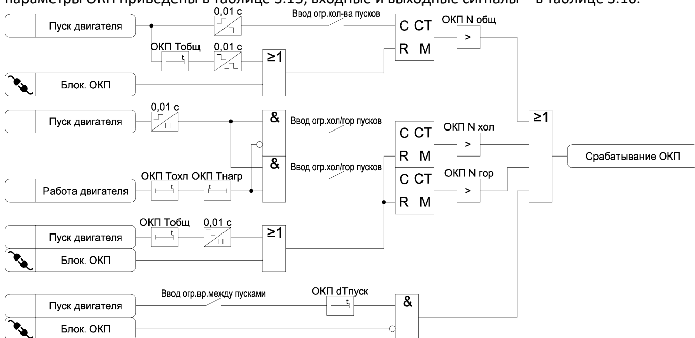
Рисунок 3.8 – Функциональная схема алгоритма ОКП
