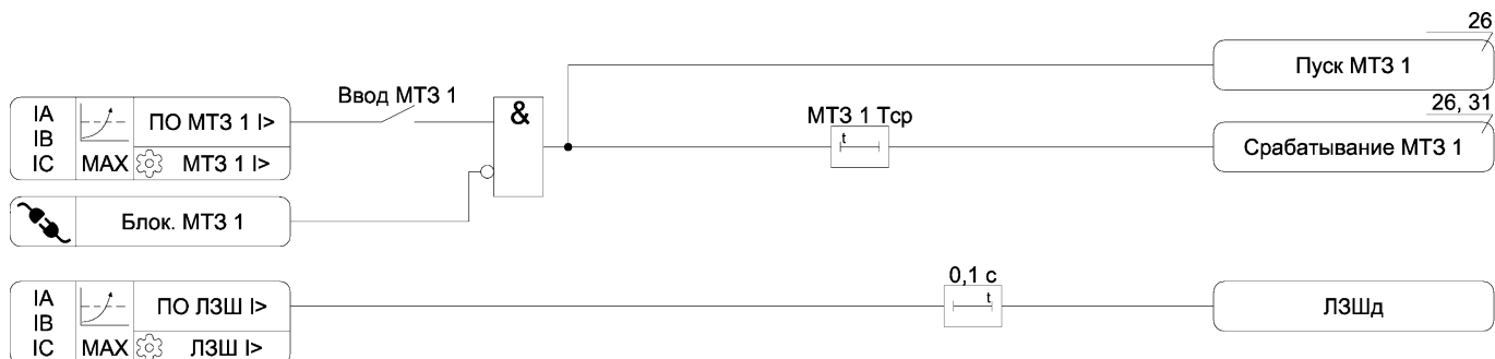
Рисунок А.2 – Функциональная схема алгоритма МТЗ и ЛЗШ
