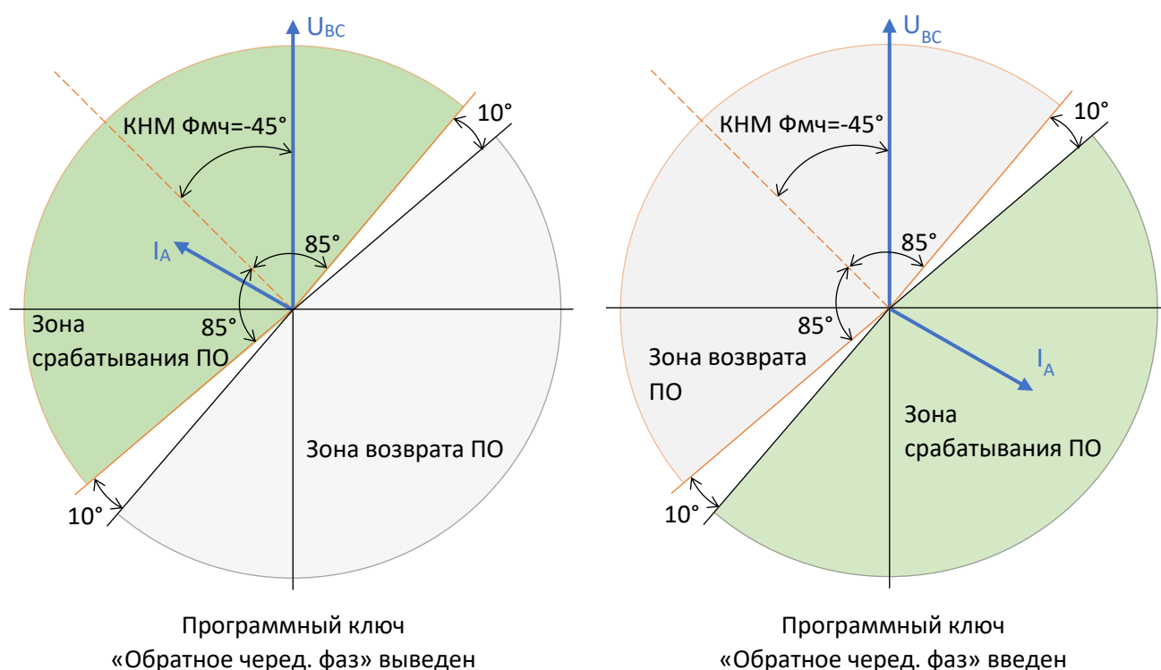
Рисунок 3.24 – Диаграмма срабатывания пускового органа функции КНМ
