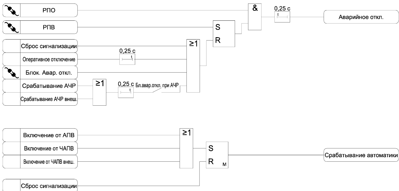
Рисунок 3.39 а) – Функциональная схема алгоритма сигнализации
