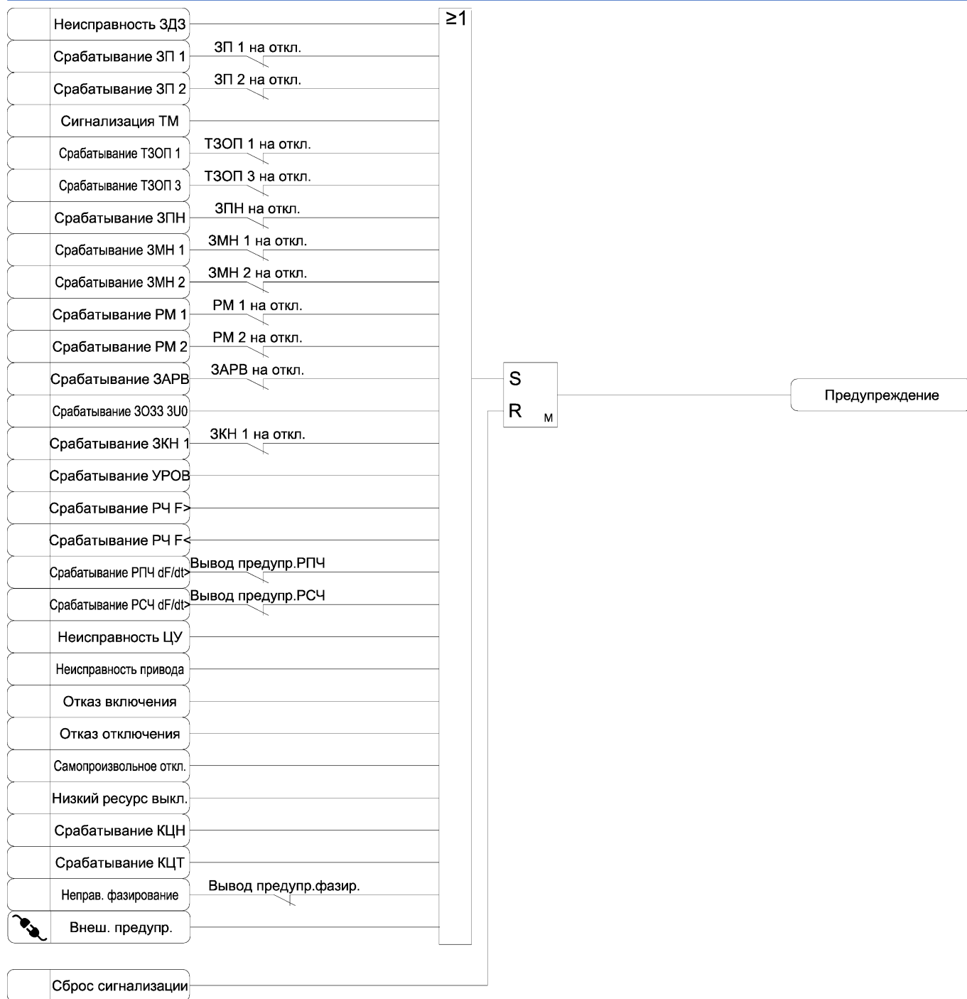
Рисунок 3.39 в) – Функциональная схема алгоритма сигнализации
