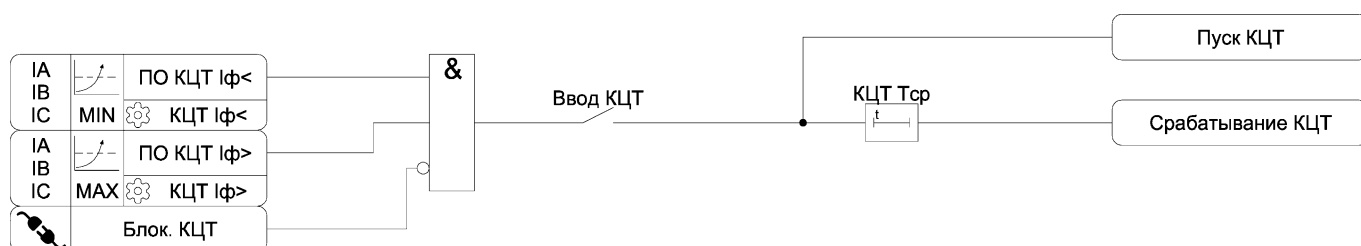
Рисунок 3.11 – Функциональная схема алгоритма КЦТ
