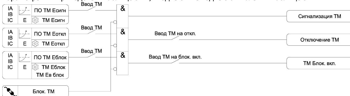
Рисунок 3.6 – Функциональная схема алгоритма ТМ
