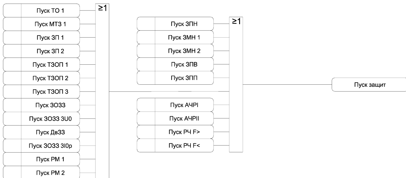
Рисунок 3.35 а) – Функциональная схема алгоритма формирования сигналов состояния защит
