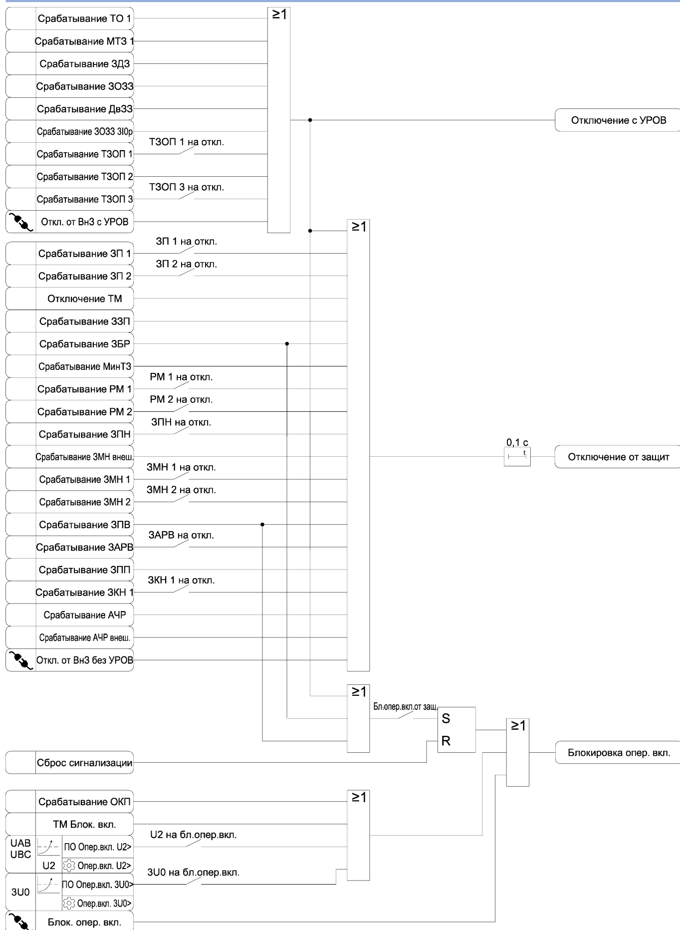
Рисунок 3.35 б) – Функциональная схема алгоритма формирования сигналов состояния защит
