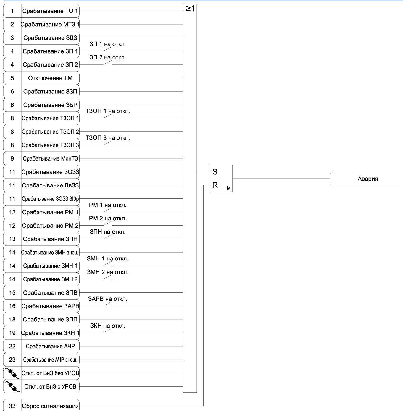
Рисунок А.31 б) – Функциональная схема алгоритма сигнализации
