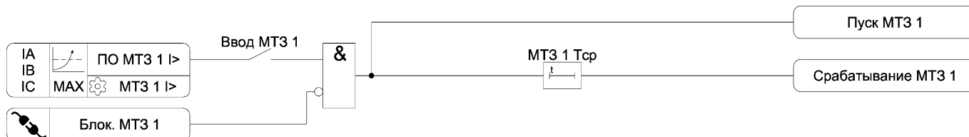
Рисунок 3.2 – Функциональная схема алгоритма МТЗ
