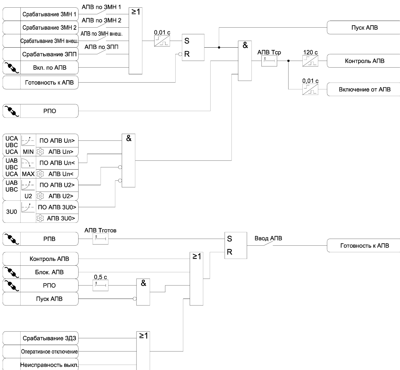
Рисунок 3.29 – Функциональная схема алгоритма АПВ
