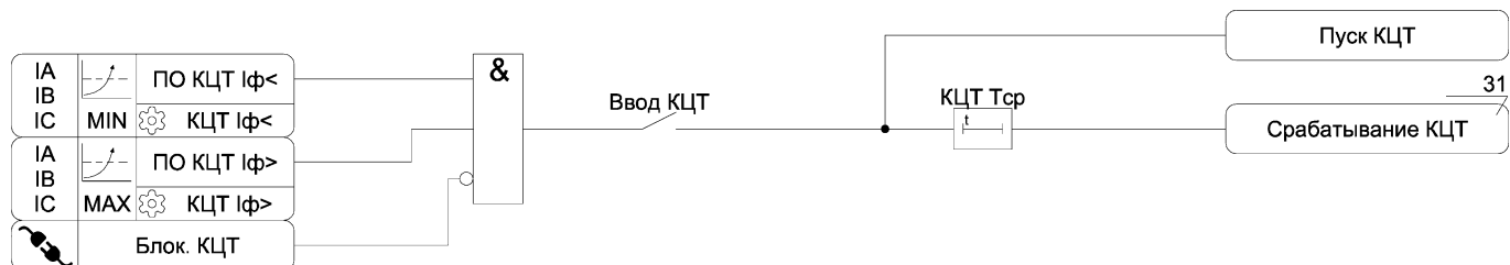
Рисунок А.10 – Функциональная схема алгоритма КЦТ
