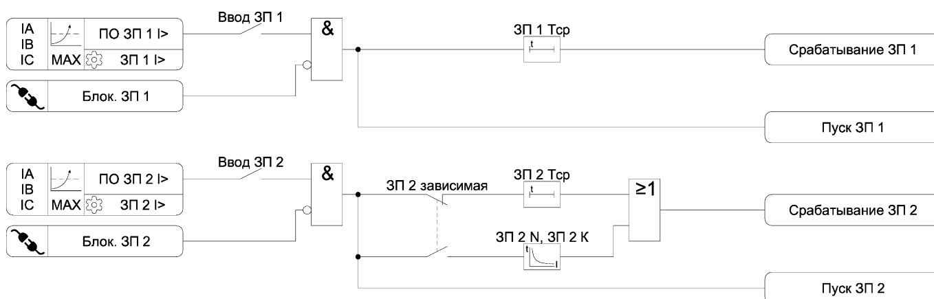
Рисунок 3.5 – Функциональная схема алгоритма ЗП
