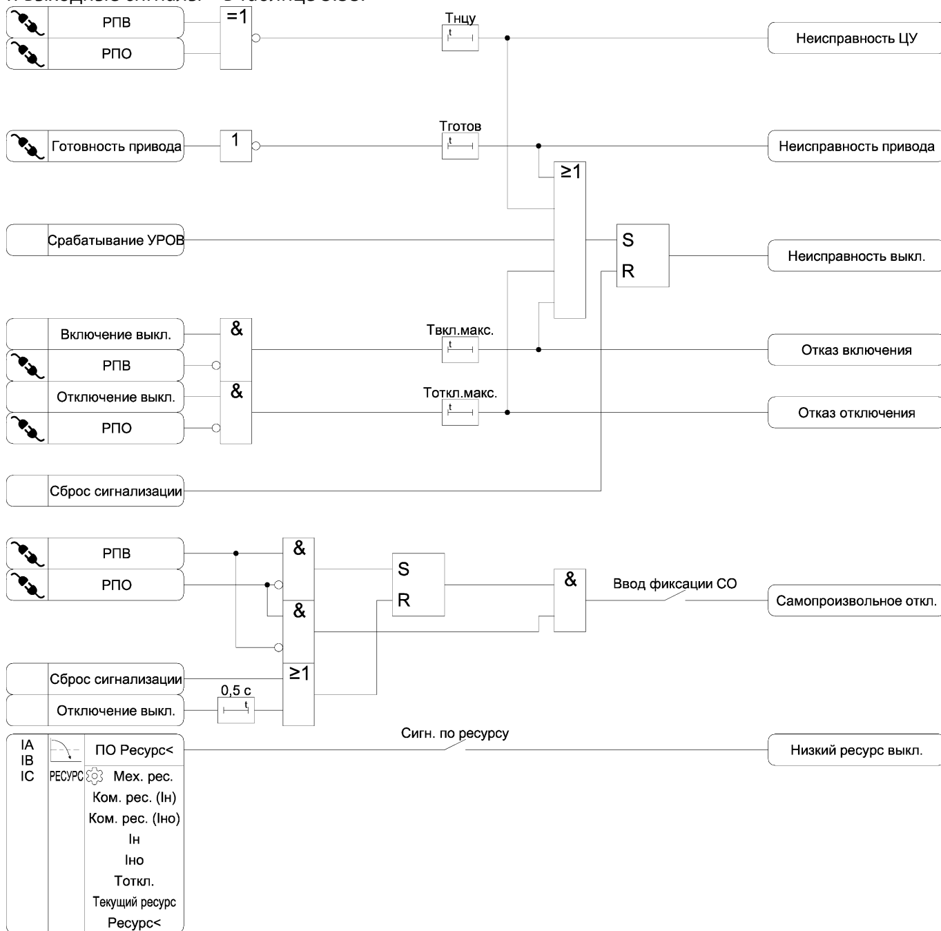
Рисунок 3.37 – Функциональная схема алгоритма диагностики выключателя
