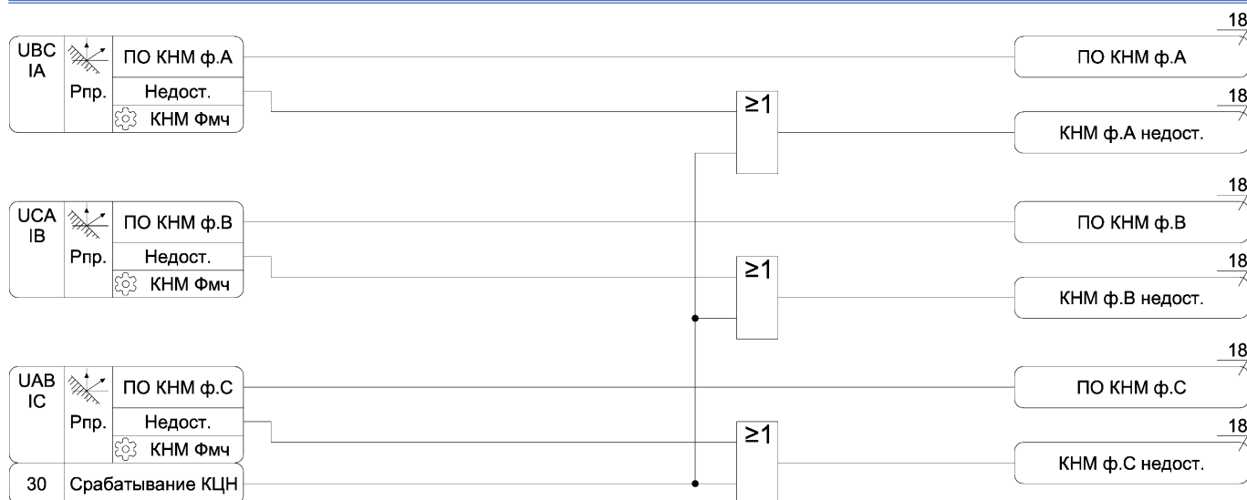
Рисунок А.17 – Функциональная схема алгоритма КНМ
