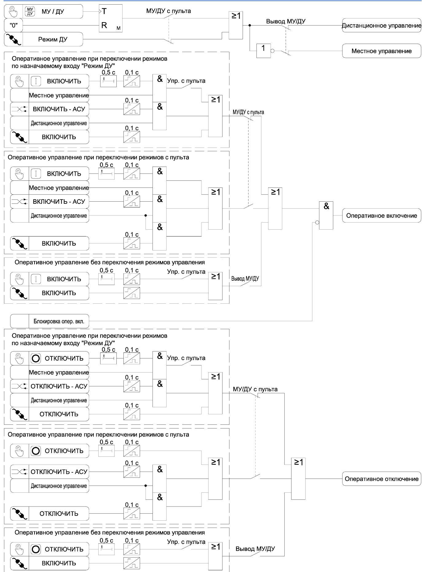
Рисунок 3.33 – Функциональная схема алгоритма оперативного управления выключателем
