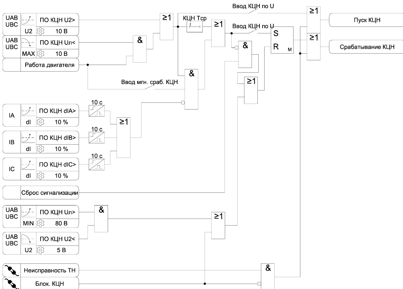
Рисунок 3.38 – Функциональная схема алгоритма КЦН
