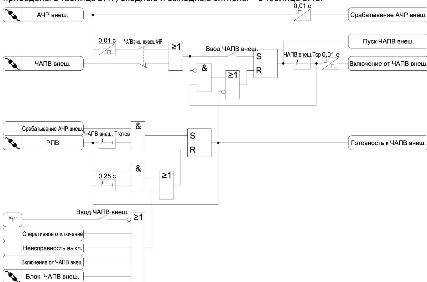
Рисунок 3.31 – Функциональные схемы алгоритмов АЧР и ЧАПВ от внешнего устройства
