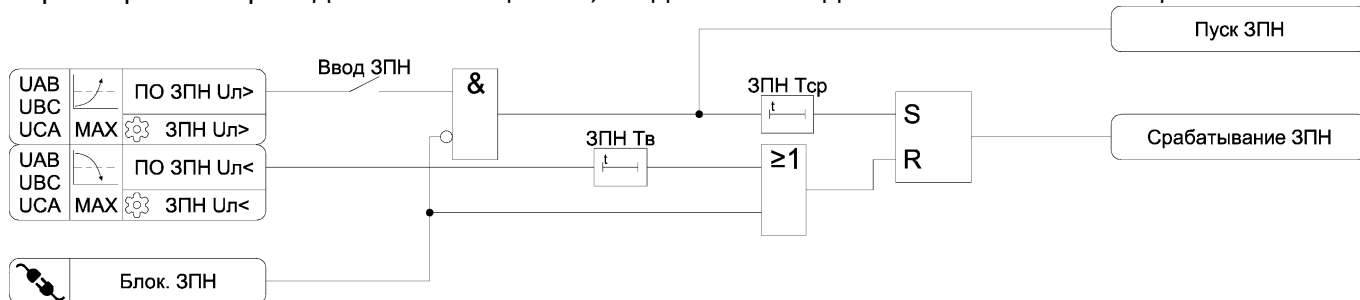
Рисунок 3.17 – Функциональная схема алгоритма ЗПН
