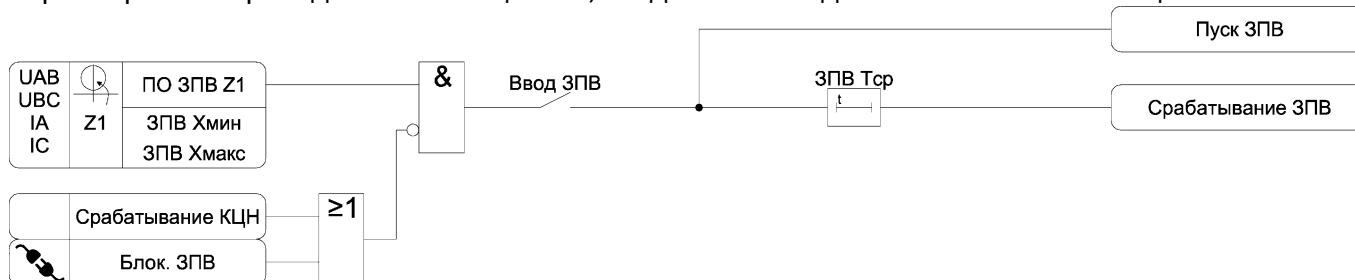
Рисунок 3.19 – Функциональная схема алгоритма ЗПВ
