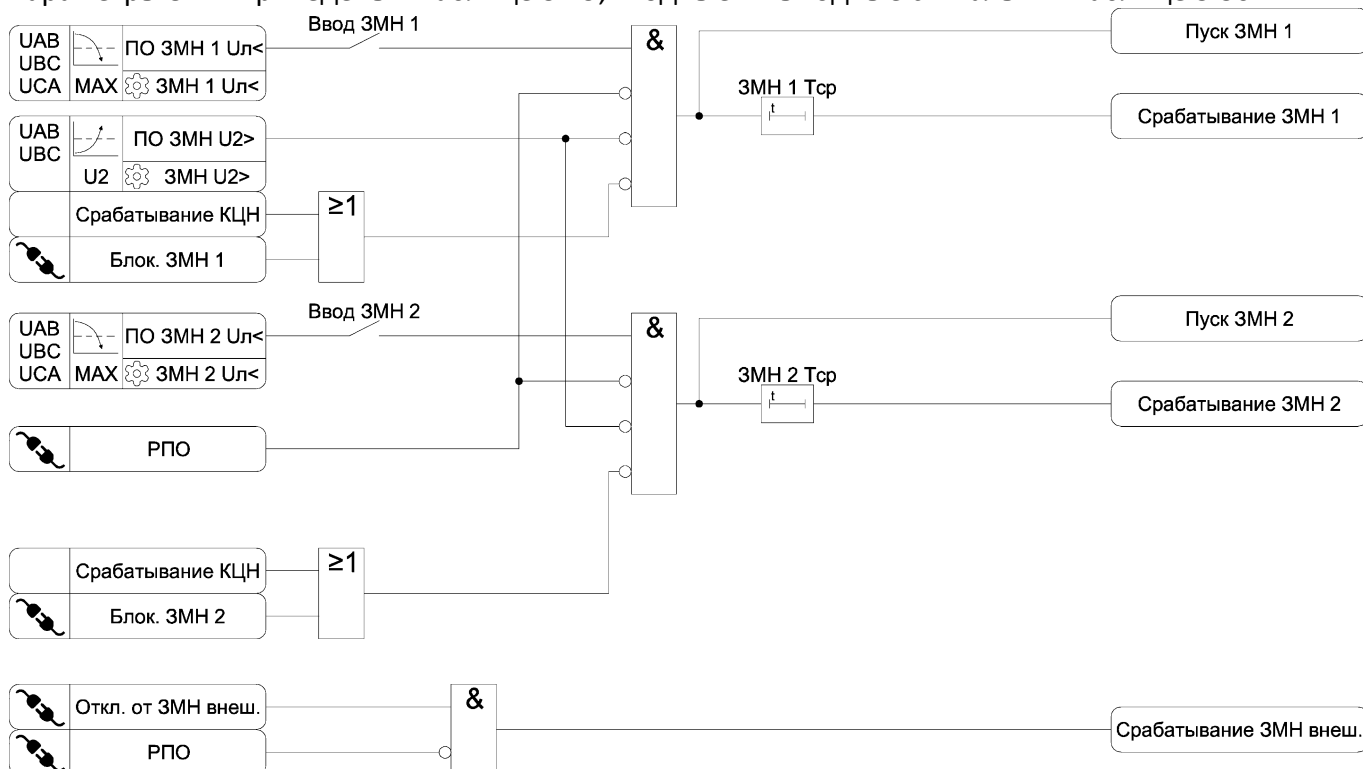
Рисунок 3.18 – Функциональная схема алгоритма ЗМН
