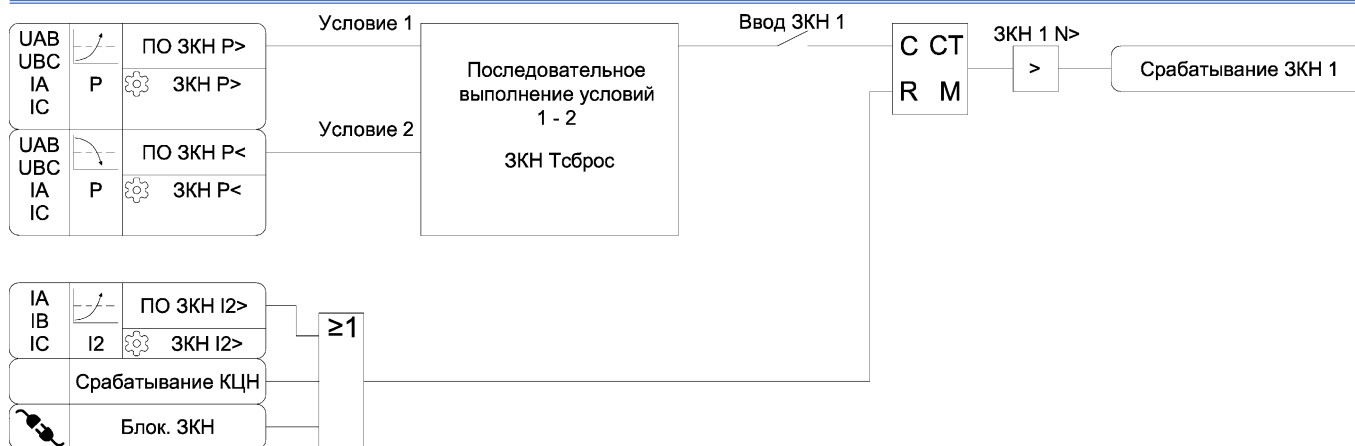
Рисунок 3.26 – Функциональная схема алгоритма ЗКН
