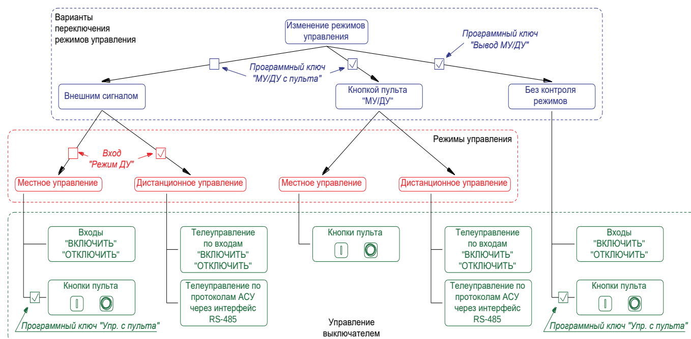
Рисунок 3.34 – Выбор режимов управления
