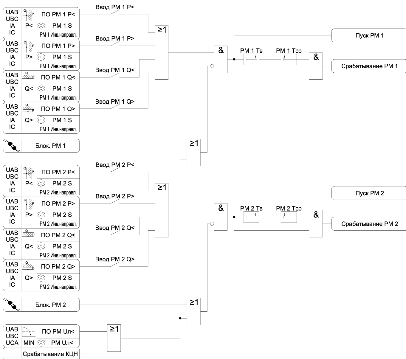
Рисунок 3.15 – Функциональная схема алгоритма защиты по направлению мощности
