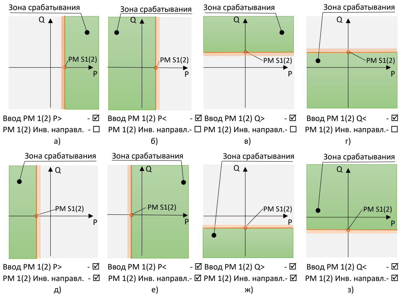
Рисунок 3.16 – Диаграмма срабатывания реле активного тока нулевой последовательности
