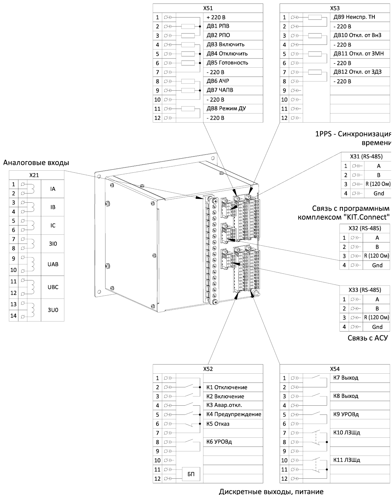
Рисунок 2.1 – Схема подключения устройства
