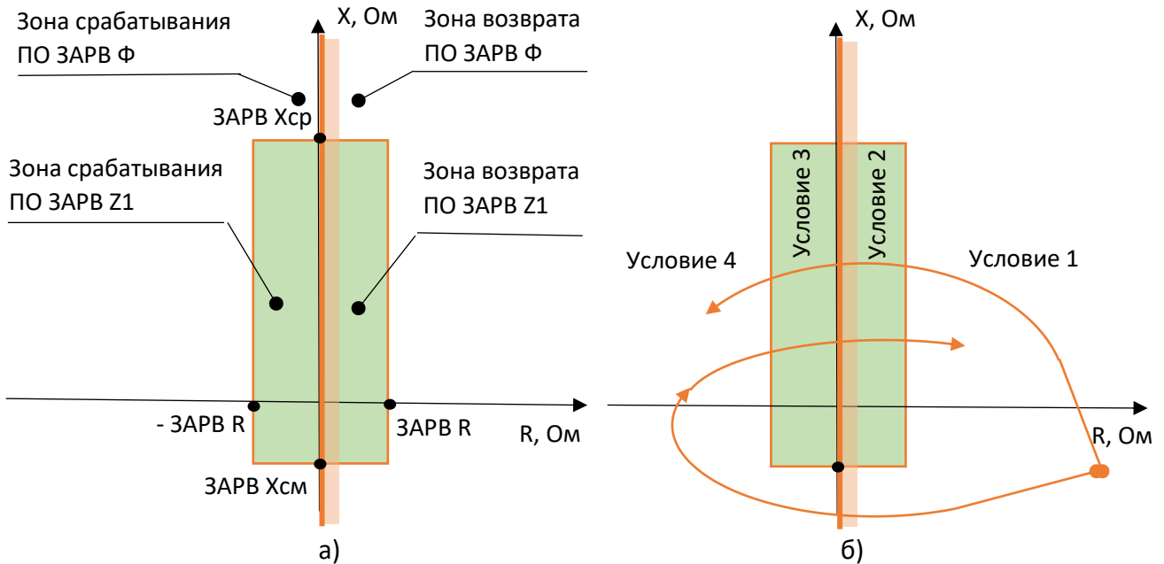
Рисунок 3.22 Характеристика срабатывания ЗАРВ (а) и годограф сопротивления при асинхронном ходе (б)
