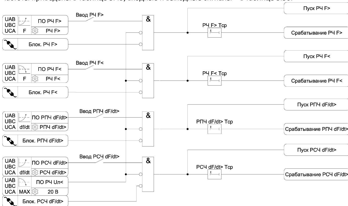
Рисунок 3.32 – Функциональные схемы алгоритмов защиты повышения и снижения частоты
