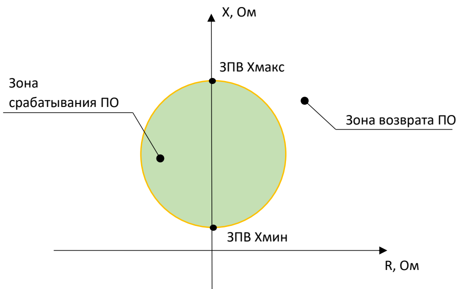
Рисунок 3.20 Характеристика срабатывания ЗПВ
