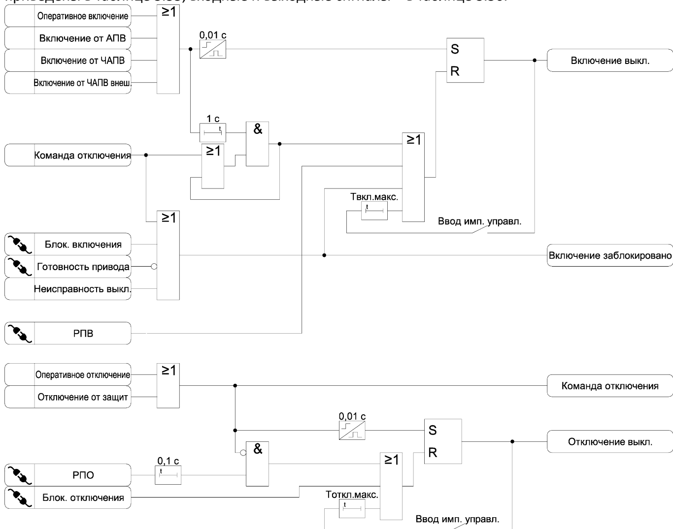
Рисунок 3.36 – Функциональная схема алгоритма управления выключателем
