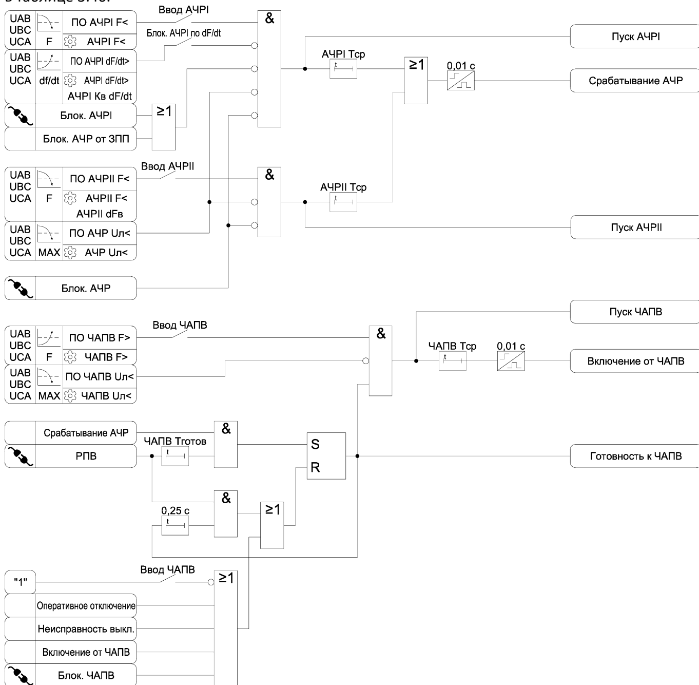
Рисунок 3.30 – Функциональные схемы алгоритмов АЧР и ЧАПВ
