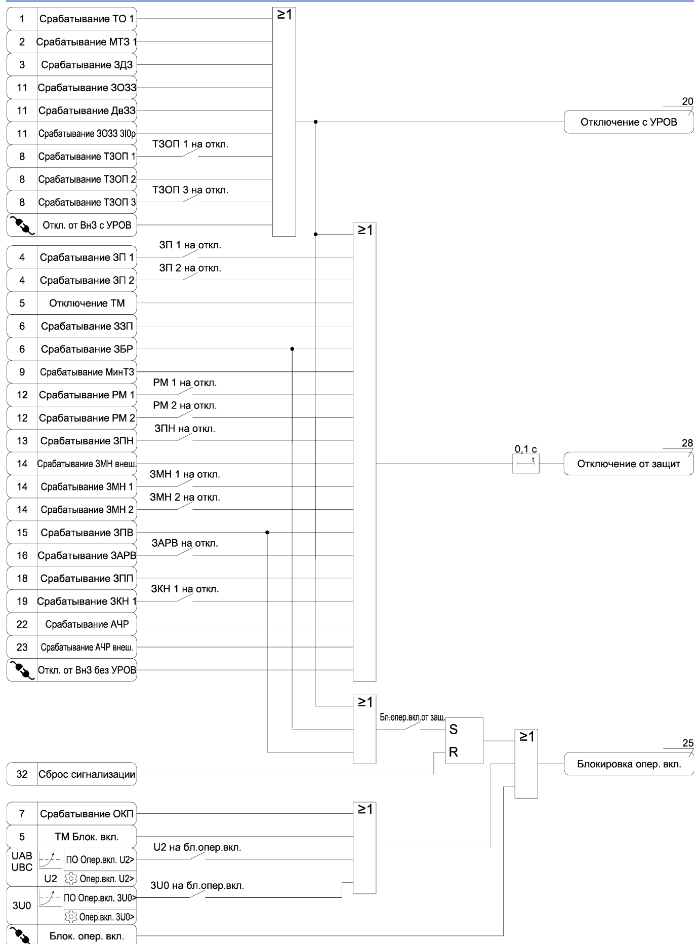
Рисунок А.26 б)– Функциональная схема алгоритма состояния защит
