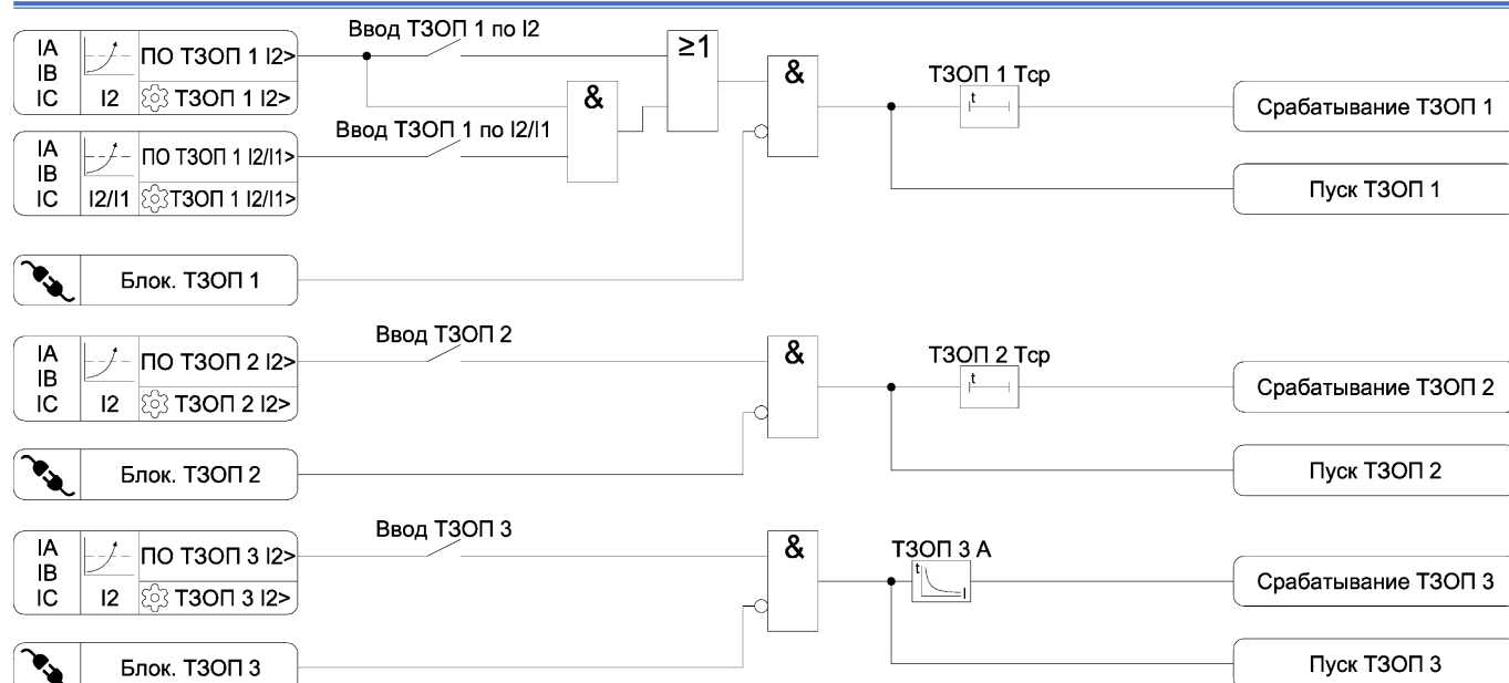
Рисунок 3.9 – Функциональная схема алгоритма ТЗОП
