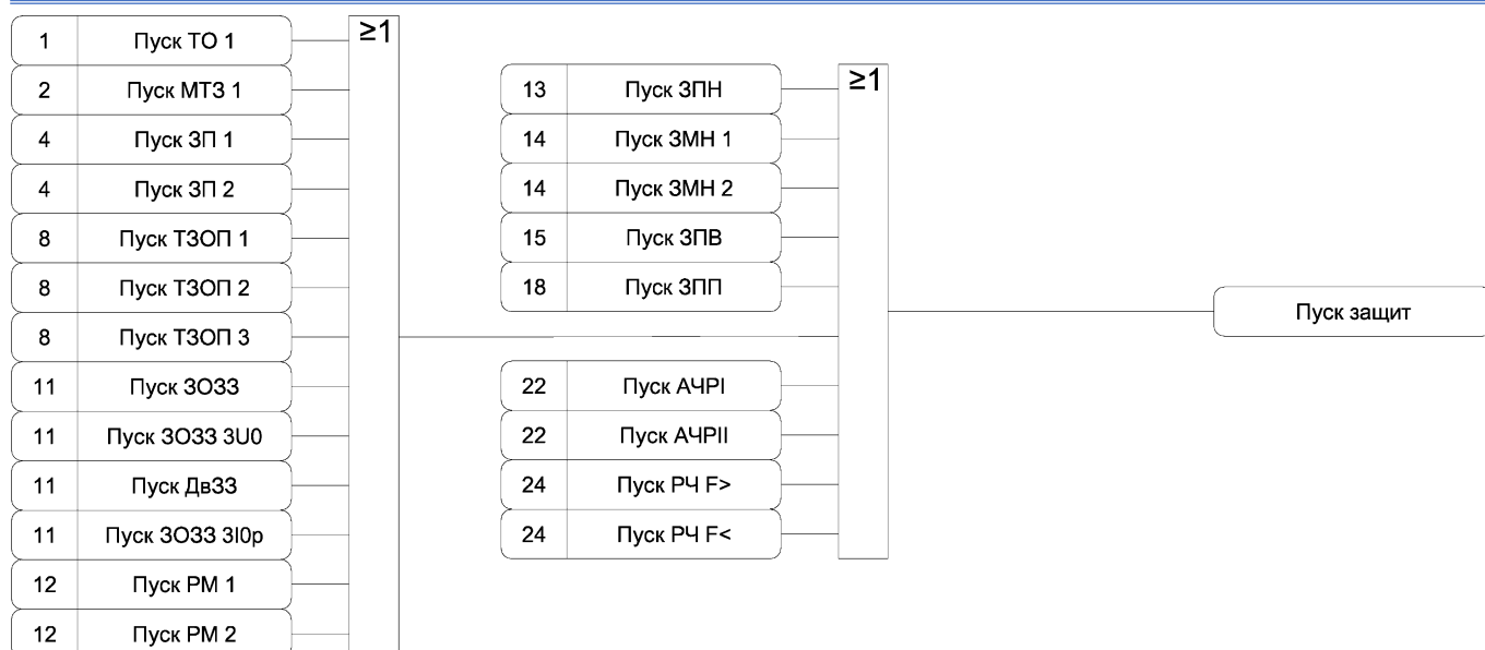
Рисунок А.26 а)– Функциональная схема алгоритма состояния защит
