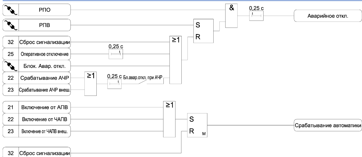
Рисунок А.31 а) – Функциональная схема алгоритма сигнализации
