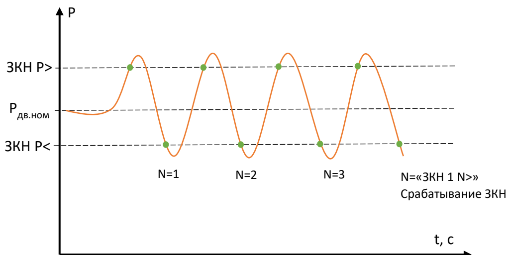
Рисунок 3.27 Временная диаграмма работы 3KH
