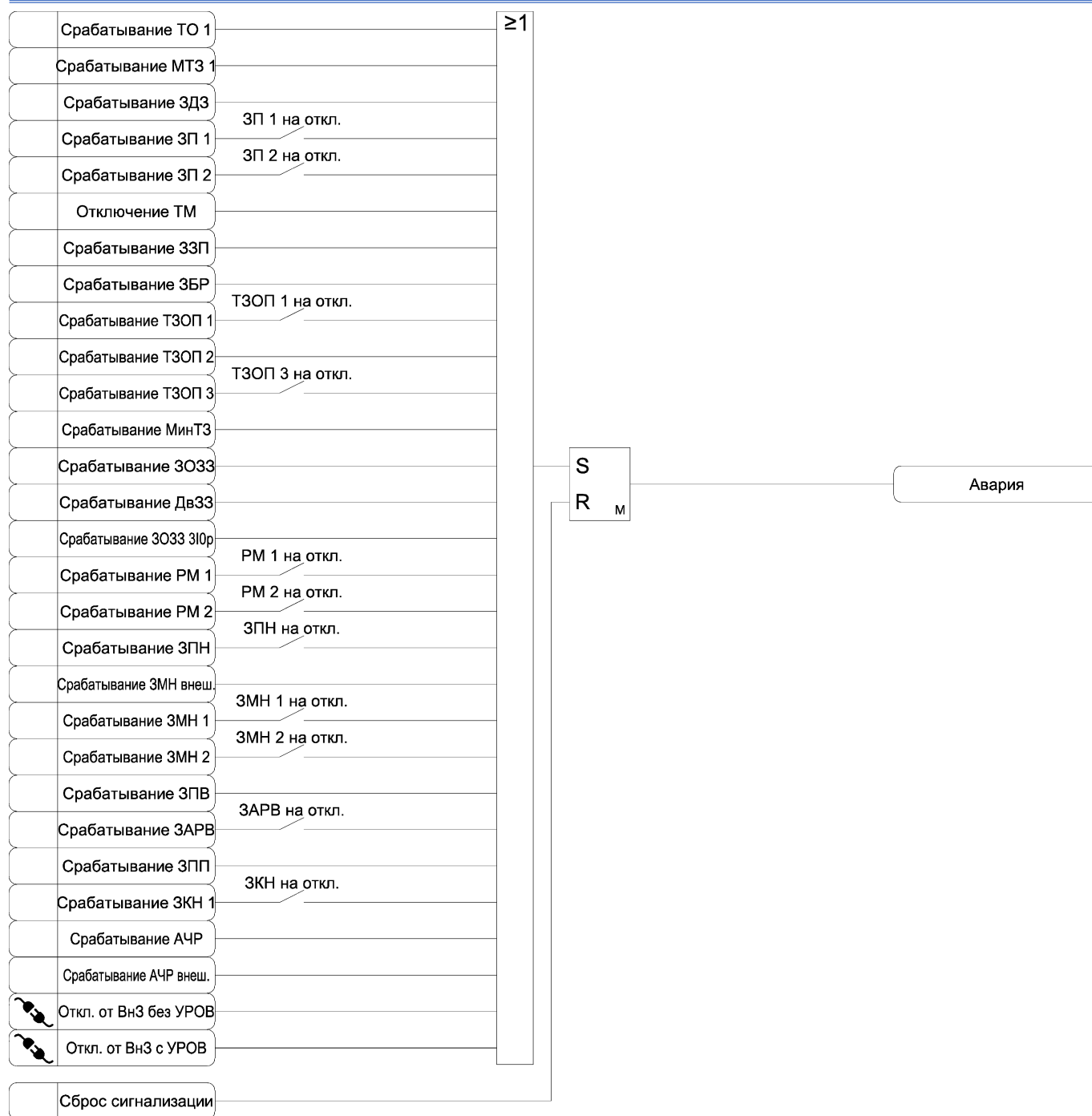
Рисунок 3.39 б) – Функциональная схема алгоритма сигнализации
