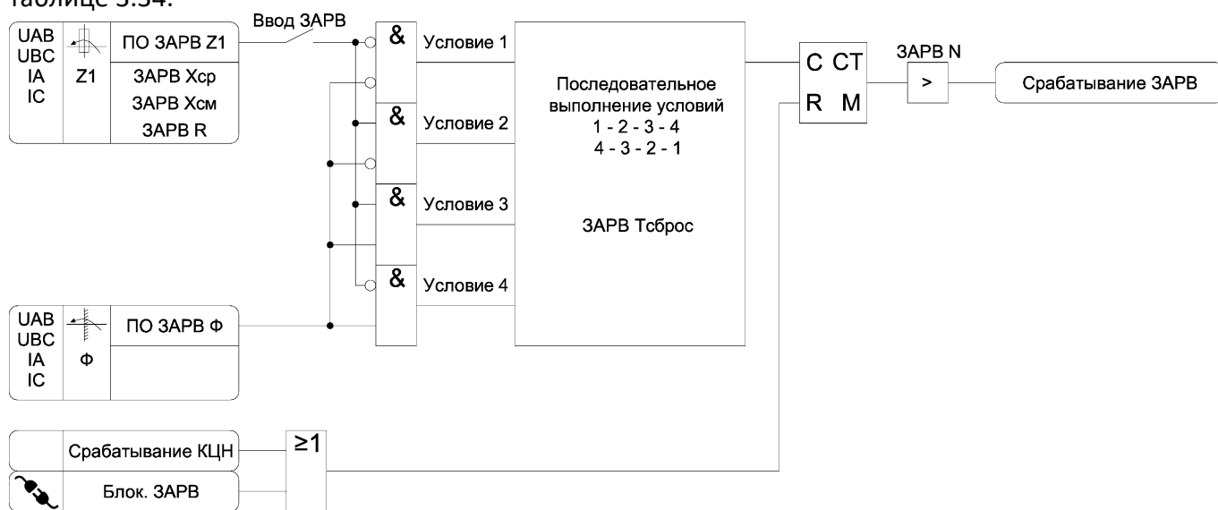
Рисунок 3.21 – Функциональная схема алгоритма ЗАРВ
