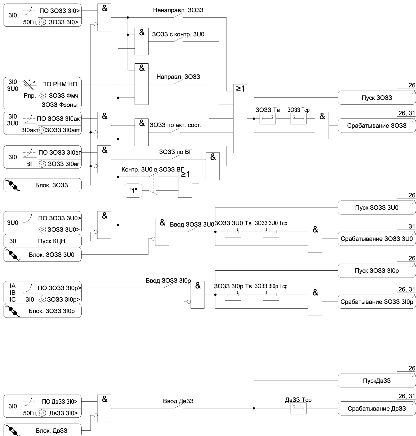
Рисунок А.11 – Функциональная схема алгоритма 3033
