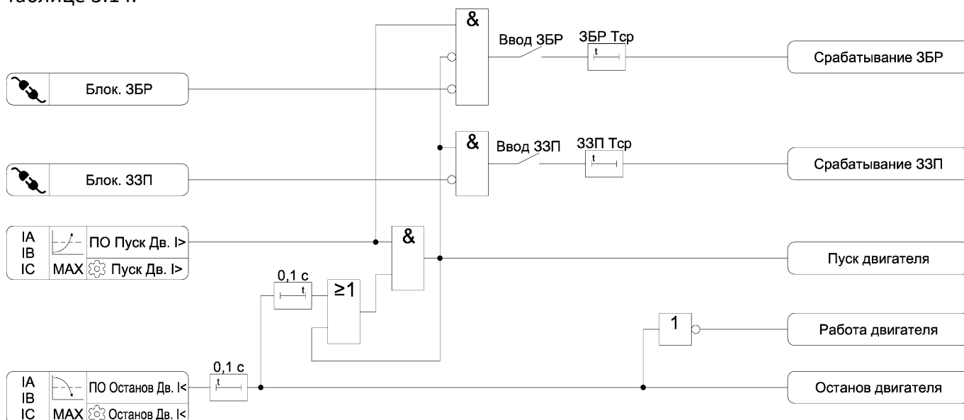
Рисунок 3.7 – Функциональная схема алгоритма ЗЗП и ЗБР
