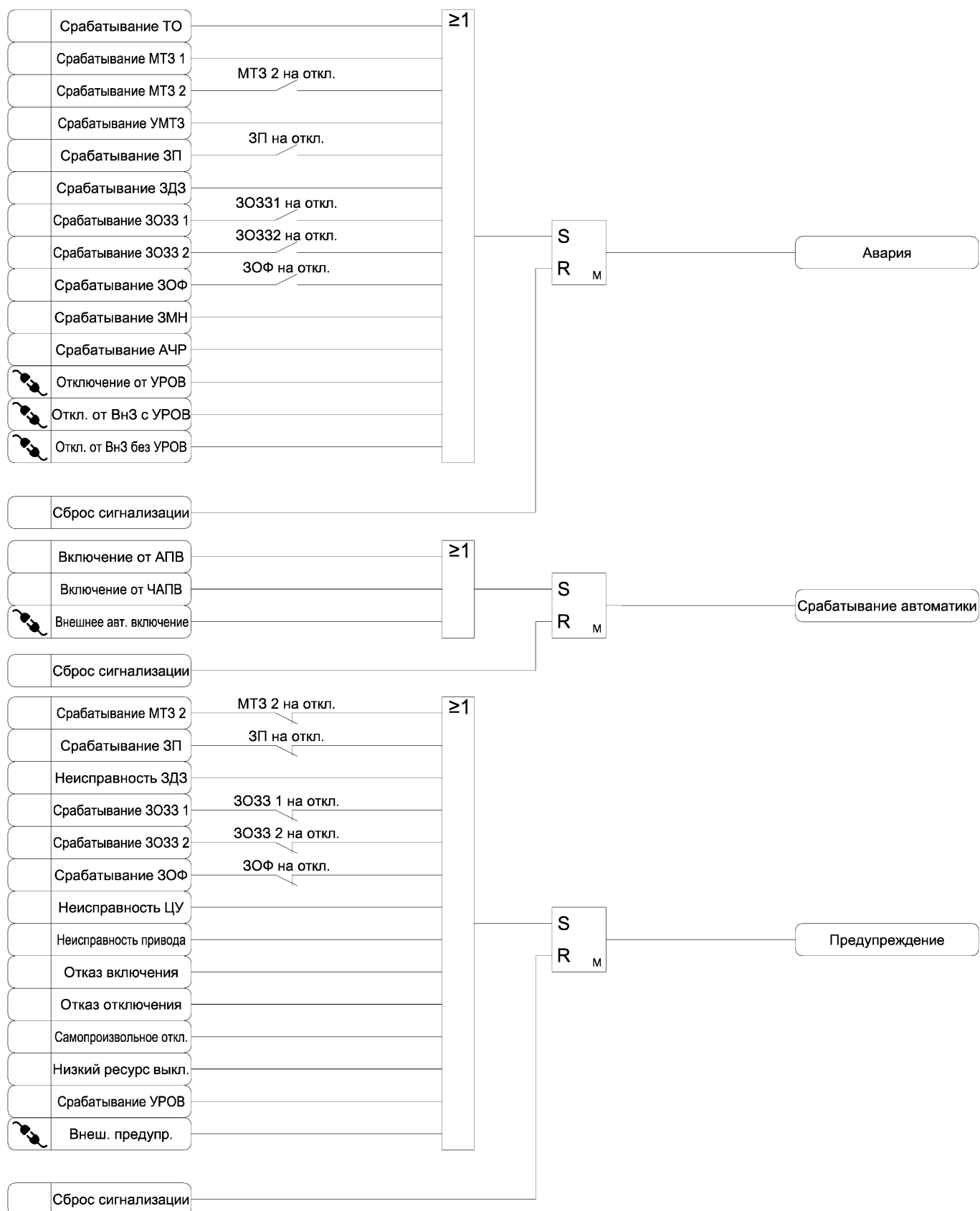
Рисунок 3.18 б)– Функциональная схема алгоритма сигнализации
