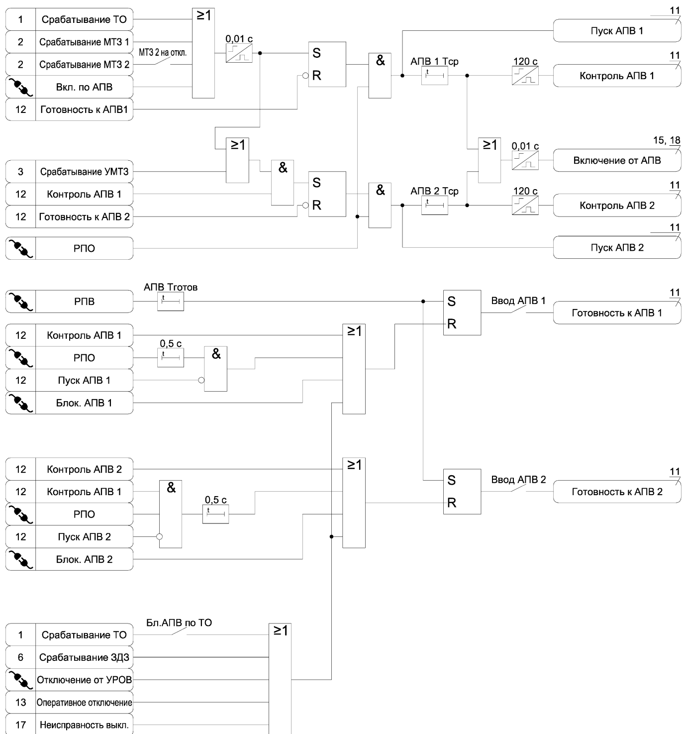
Рисунок А.12 – Функциональная схема алгоритма АПВ
