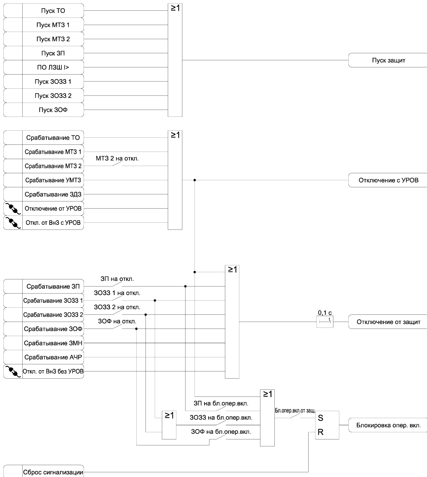
Рисунок 3.15 – Функциональная схема алгоритма формирования сигналов состояния защит
