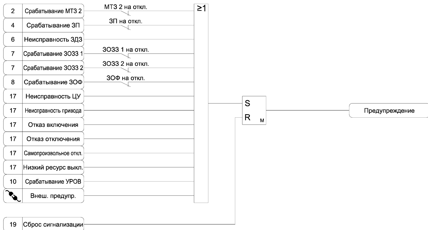
Рисунок А.18 б) – Функциональная схема алгоритма сигнализации
