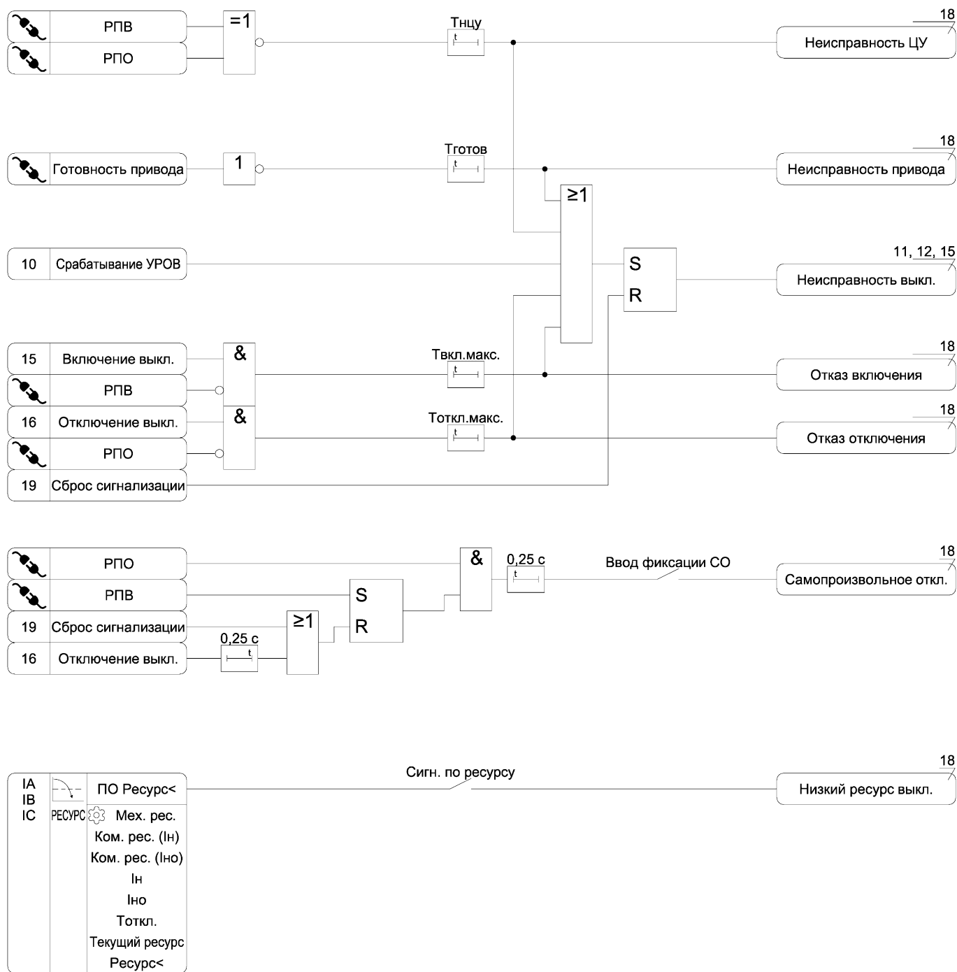
Рисунок А.17 – Функциональная схема алгоритма диагностики выключателя
