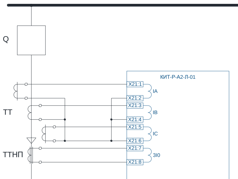
а) схема с тремя ТТ
