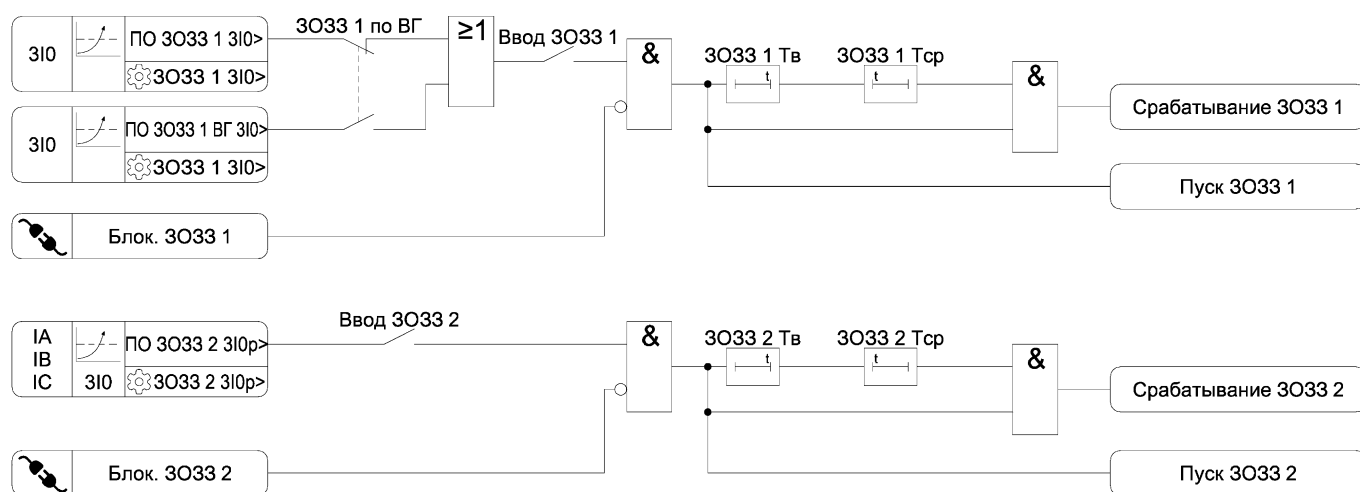
Рисунок 3.7 – Функциональная схема алгоритма ЗОЗЗ
