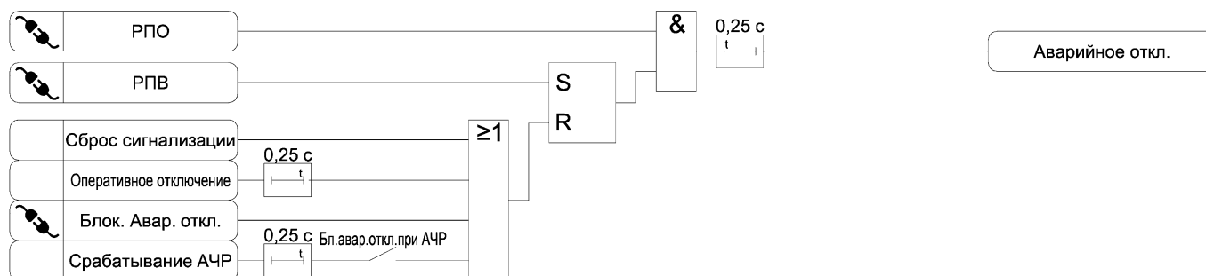
Рисунок 3.18 а) – Функциональная схема алгоритма сигнализации
