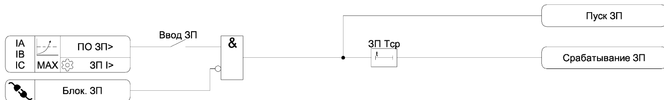
Рисунок 3.4 – Функциональная схема алгоритма ЗП
