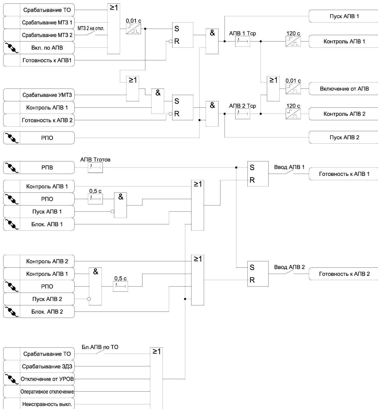
Рисунок 3.12 – Функциональная схема алгоритма АПВ
