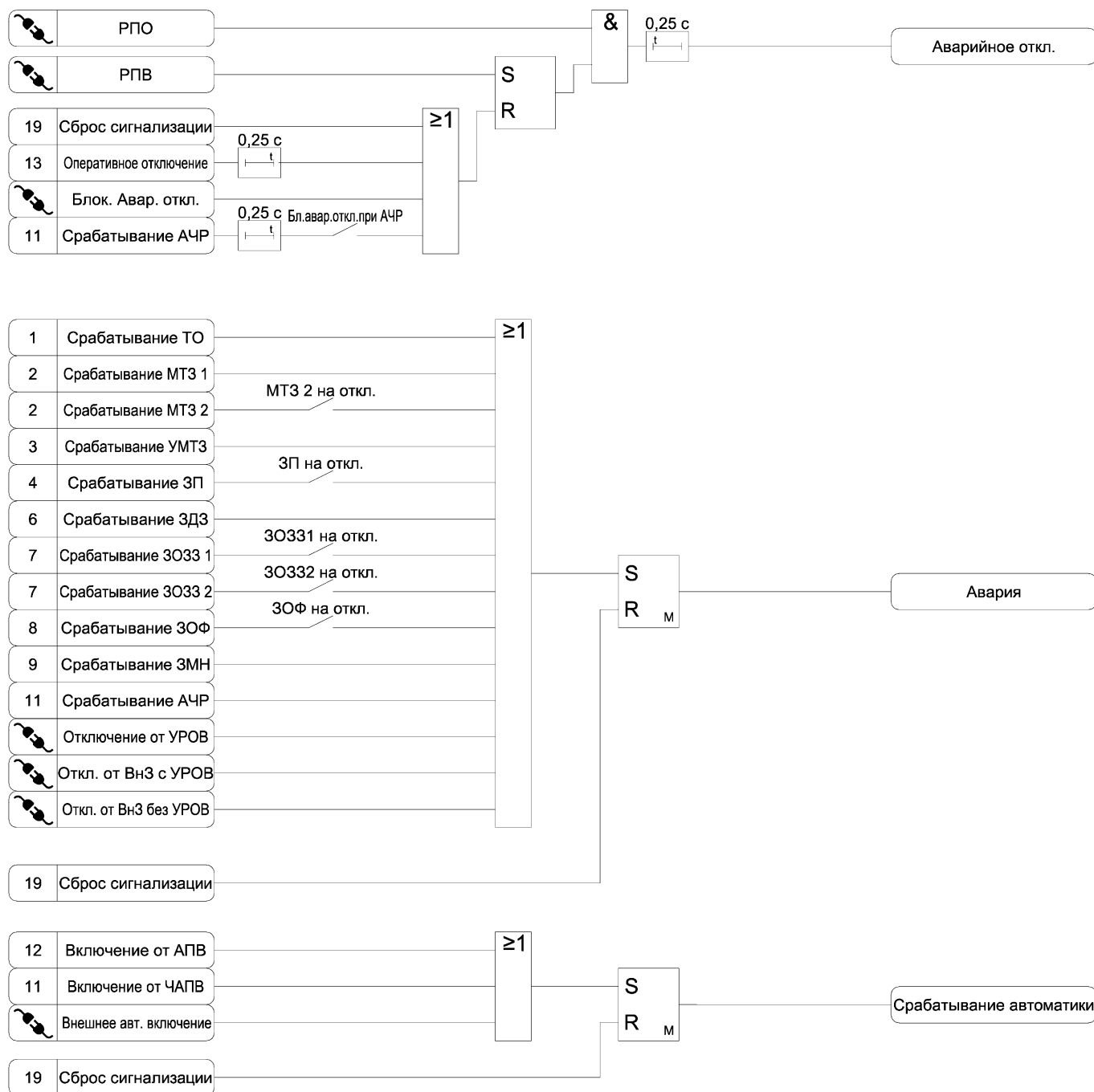
Рисунок А.18 а) – Функциональная схема алгоритма сигнализации
