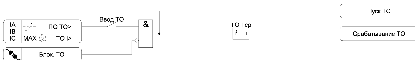
Рисунок 3.1 – Функциональная схема алгоритма ТО
