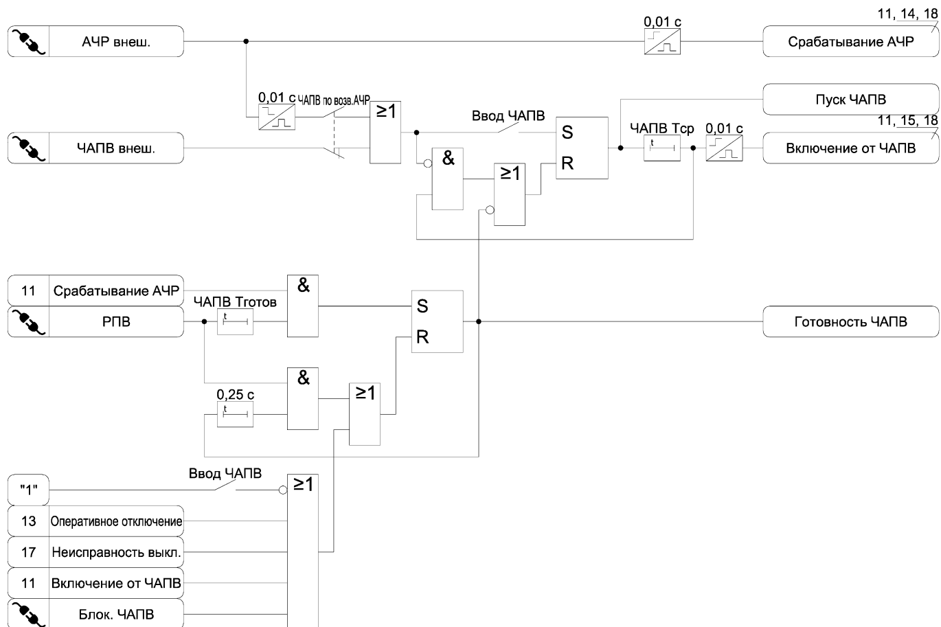
Рисунок А.11 – Функциональные схемы алгоритмов АЧР и ЧАПВ
