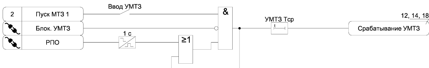
Рисунок А.3 – Функциональная схема алгоритма УМТЗ
