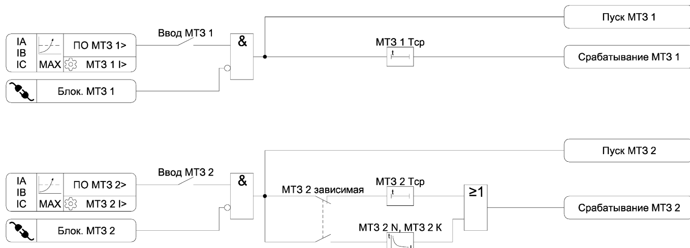
Рисунок 3.2 – Функциональная схема алгоритма МТЗ
