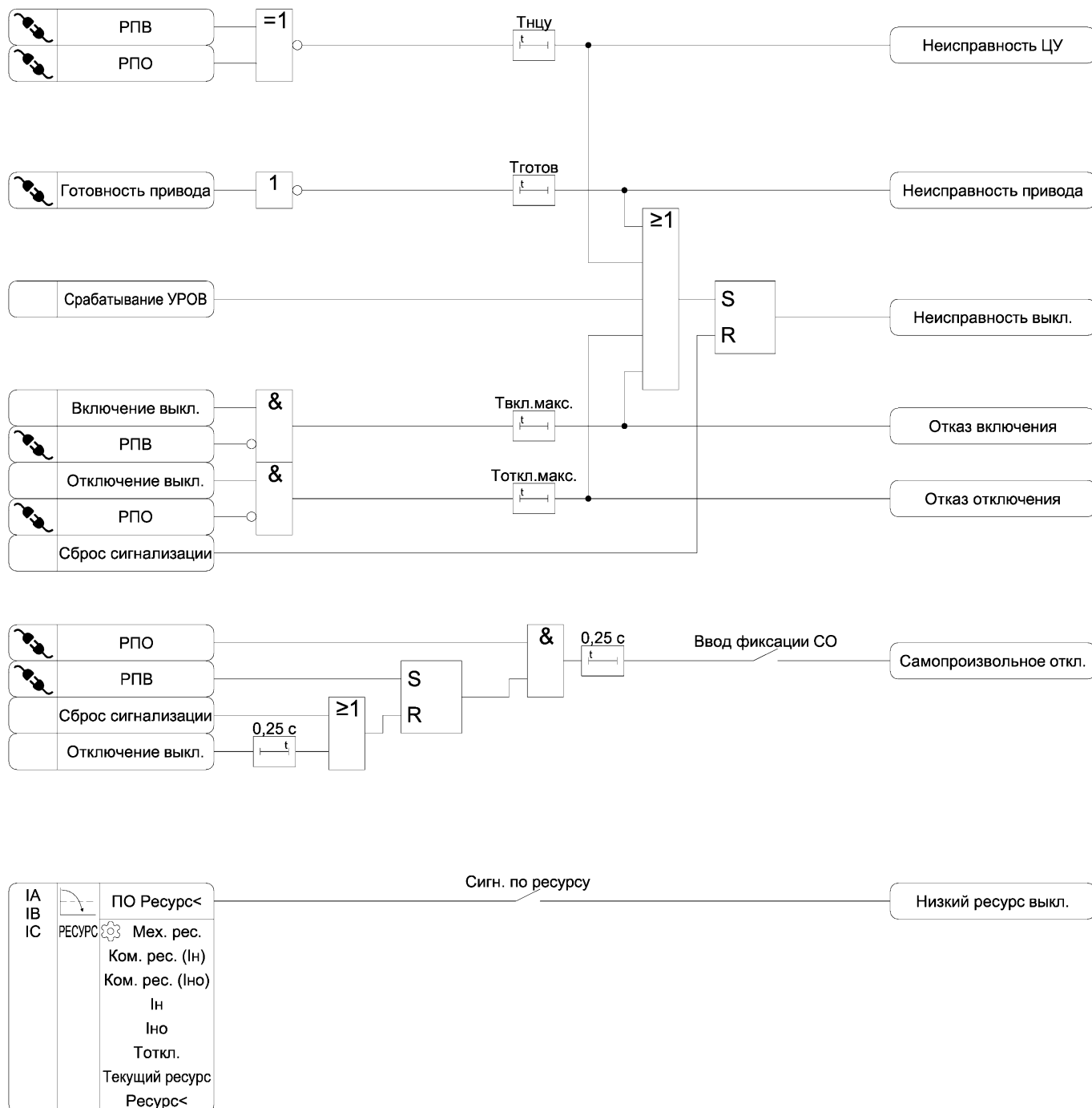
Рисунок 3.17 – Функциональная схема алгоритма диагностики выключателя
