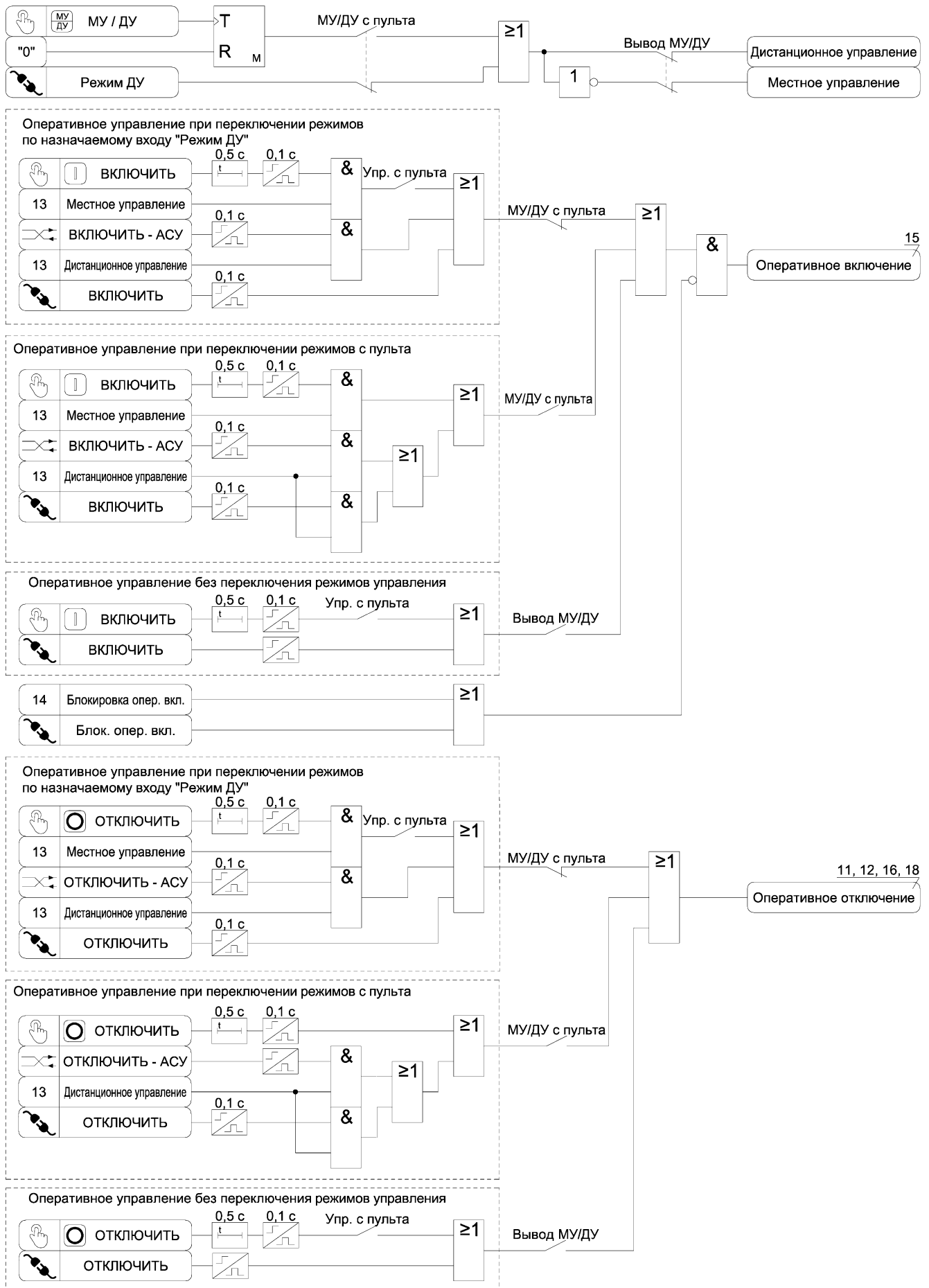
Рисунок А.13 – Функциональная схема алгоритма оперативного управления выключателем
