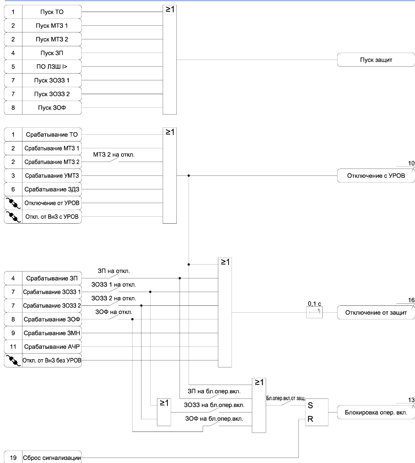
Рисунок А.14 – Функциональная схема алгоритма состояния защит
