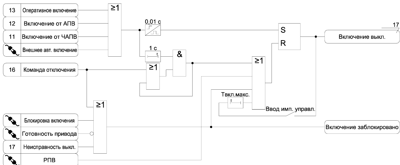
Рисунок А.15 – Функциональная схема алгоритма включения выключателя
