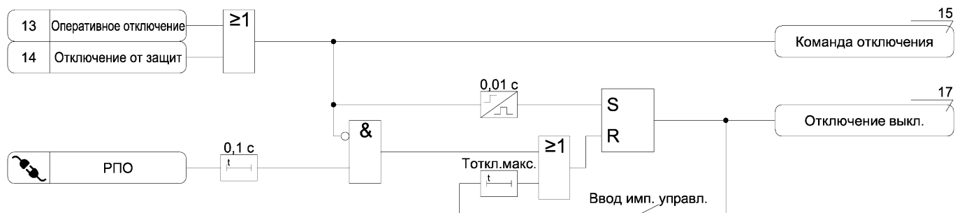
Рисунок А.16 – Функциональная схема алгоритма отключения выключателя
