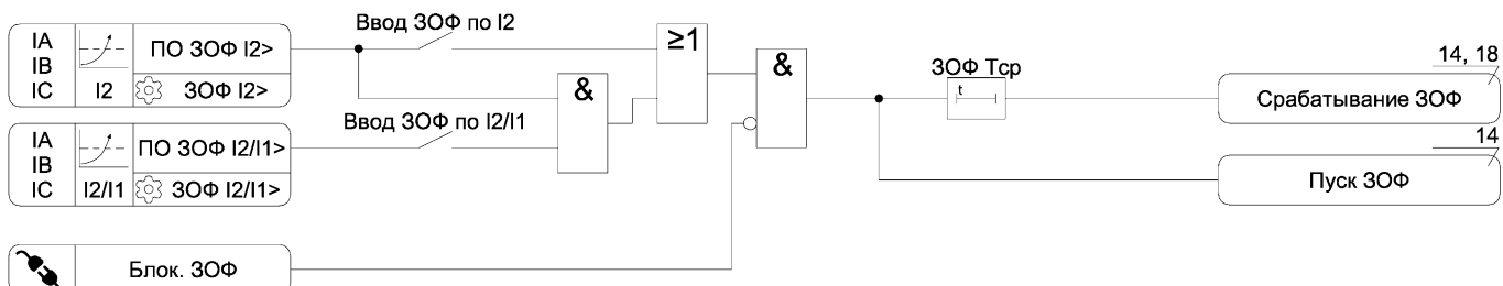
Рисунок А.8 – Функциональная схема алгоритма ZOФ
