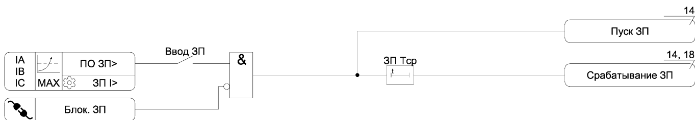
Рисунок А.4 – Функциональная схема алгоритма ЗП
