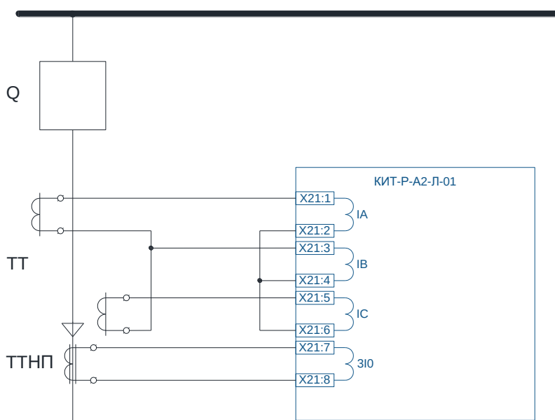
б) схема с двумя ТТ
