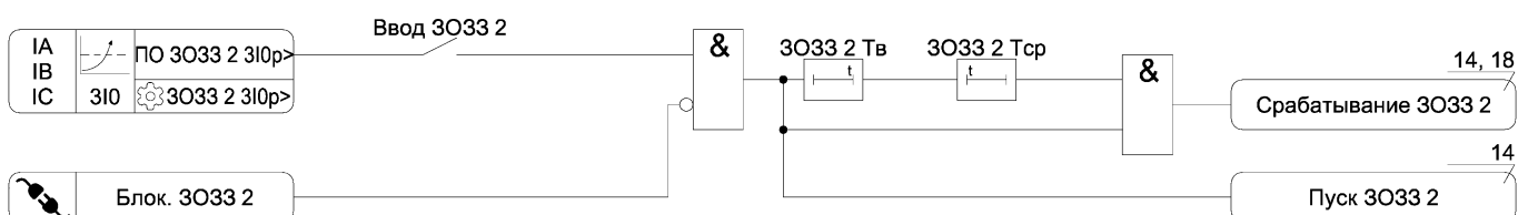
Рисунок А.7 – Функциональная схема алгоритма ZO33
