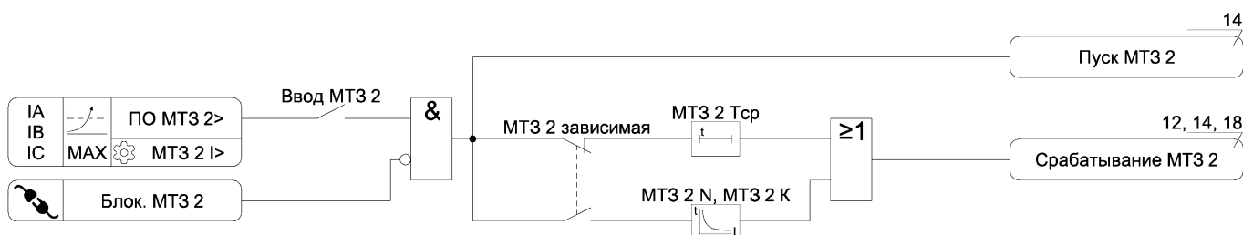
Рисунок А.2 – Функциональная схема алгоритма МТЗ
