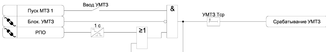
Рисунок 3.3 – Функциональная схема алгоритма УМТЗ
