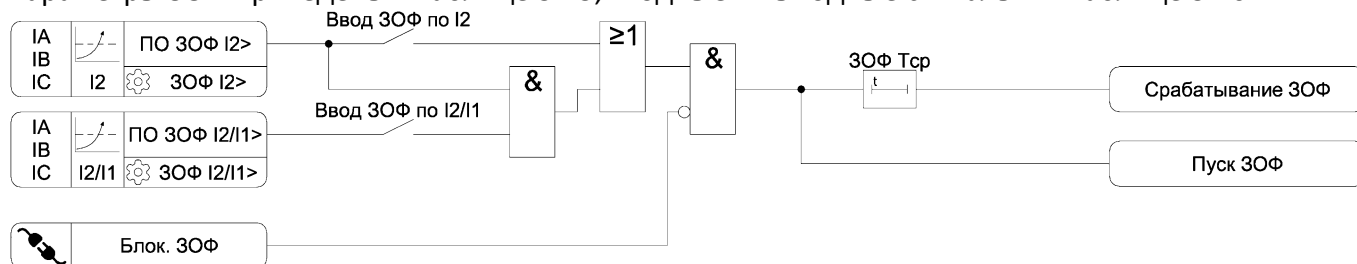
Рисунок 3.8 – Функциональная схема алгоритма ЗОФ
