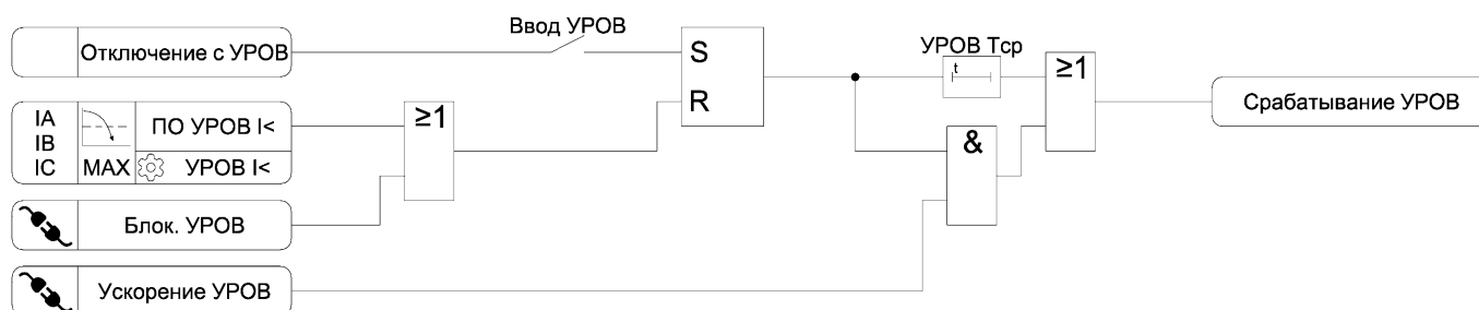
Рисунок 3.10 – Функциональная схема алгоритма УРОВ
