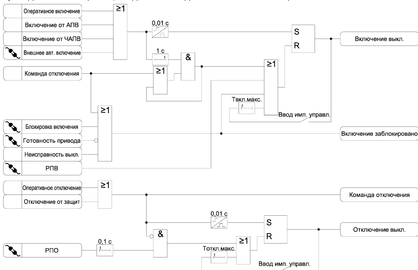
Рисунок 3.16 – Функциональная схема алгоритма управления выключателем
