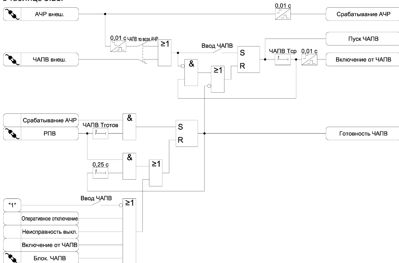
Рисунок 3.11 – Функциональные схемы алгоритмов АЧР и ЧАПВ
