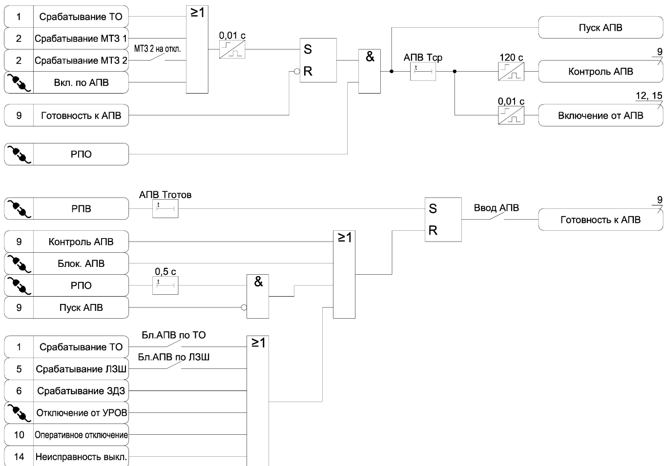
Рисунок А.9 – Функциональная схема алгоритма АПВ
