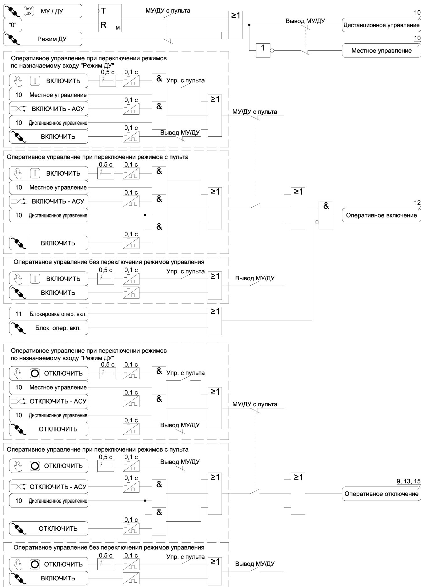
Рисунок А.10 – Функциональная схема алгоритма оперативного управления выключателем
