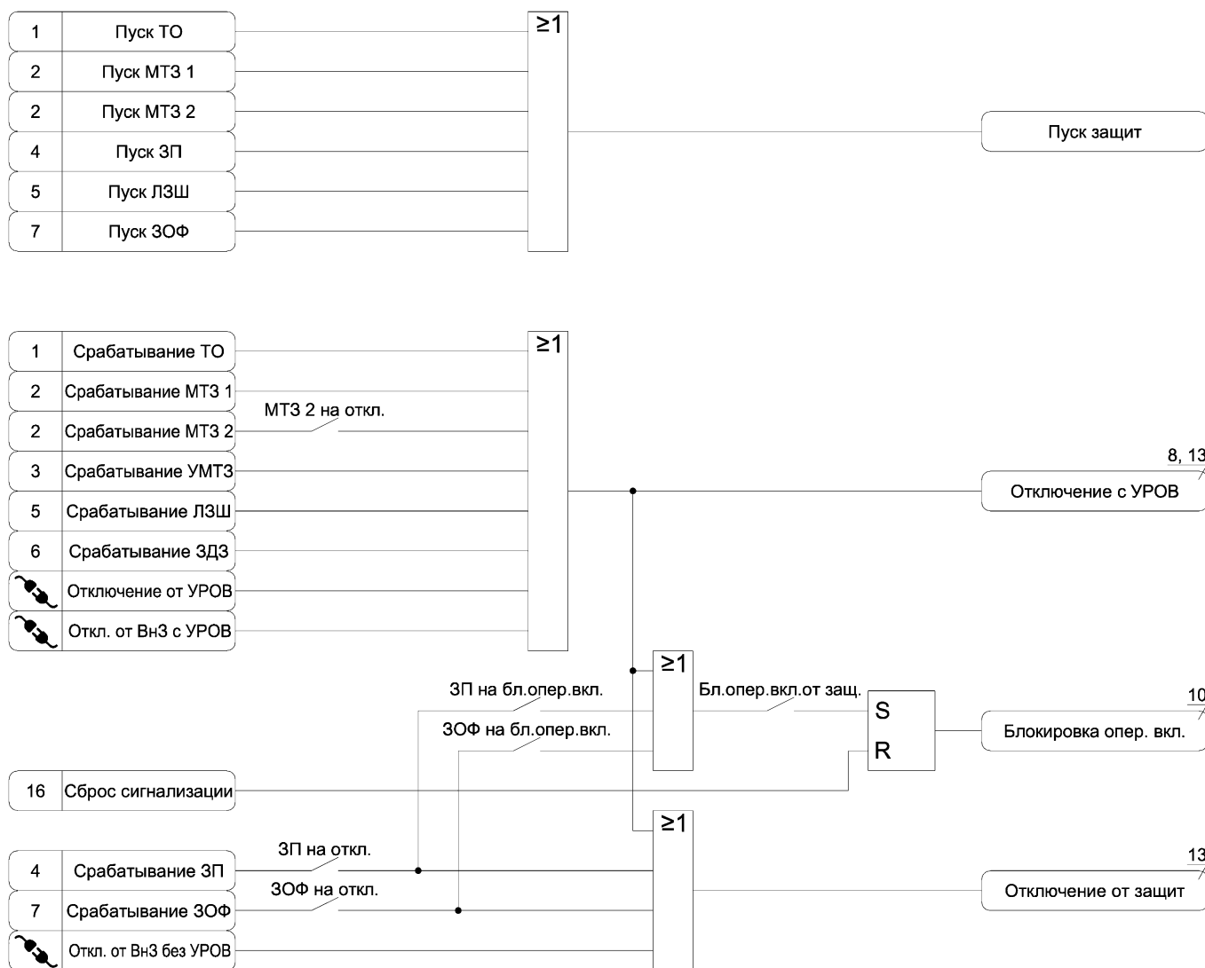
Рисунок А.11 – Функциональная схема алгоритма состояния защит
