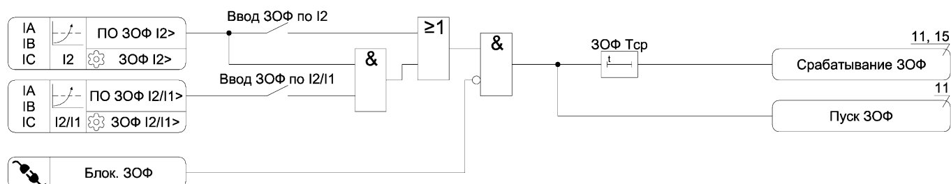
Рисунок А.7 – Функциональная схема алгоритма ЗОФ
