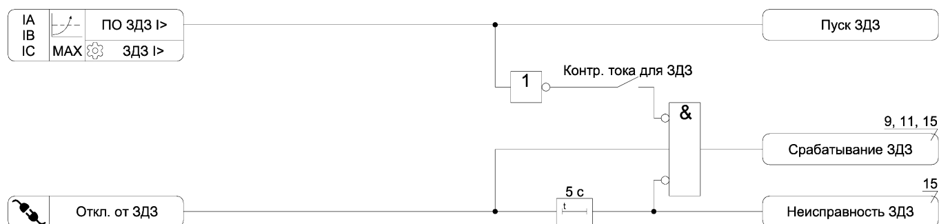
Рисунок А.6 – Функциональная схема алгоритма ЗДЗ
