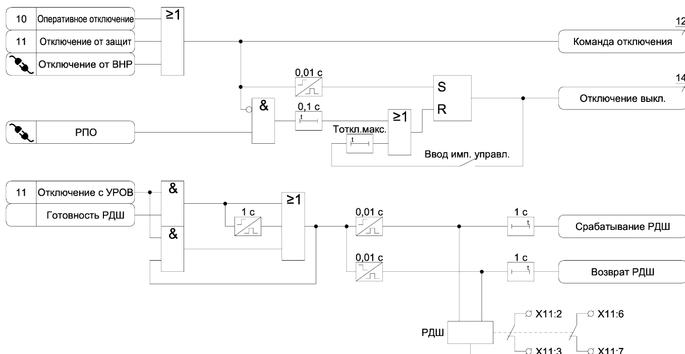
Рисунок А.13 – Функциональная схема алгоритма отключения выключателя
