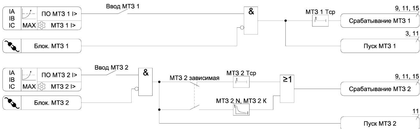
Рисунок А.2 – Функциональная схема алгоритма МТЗ
