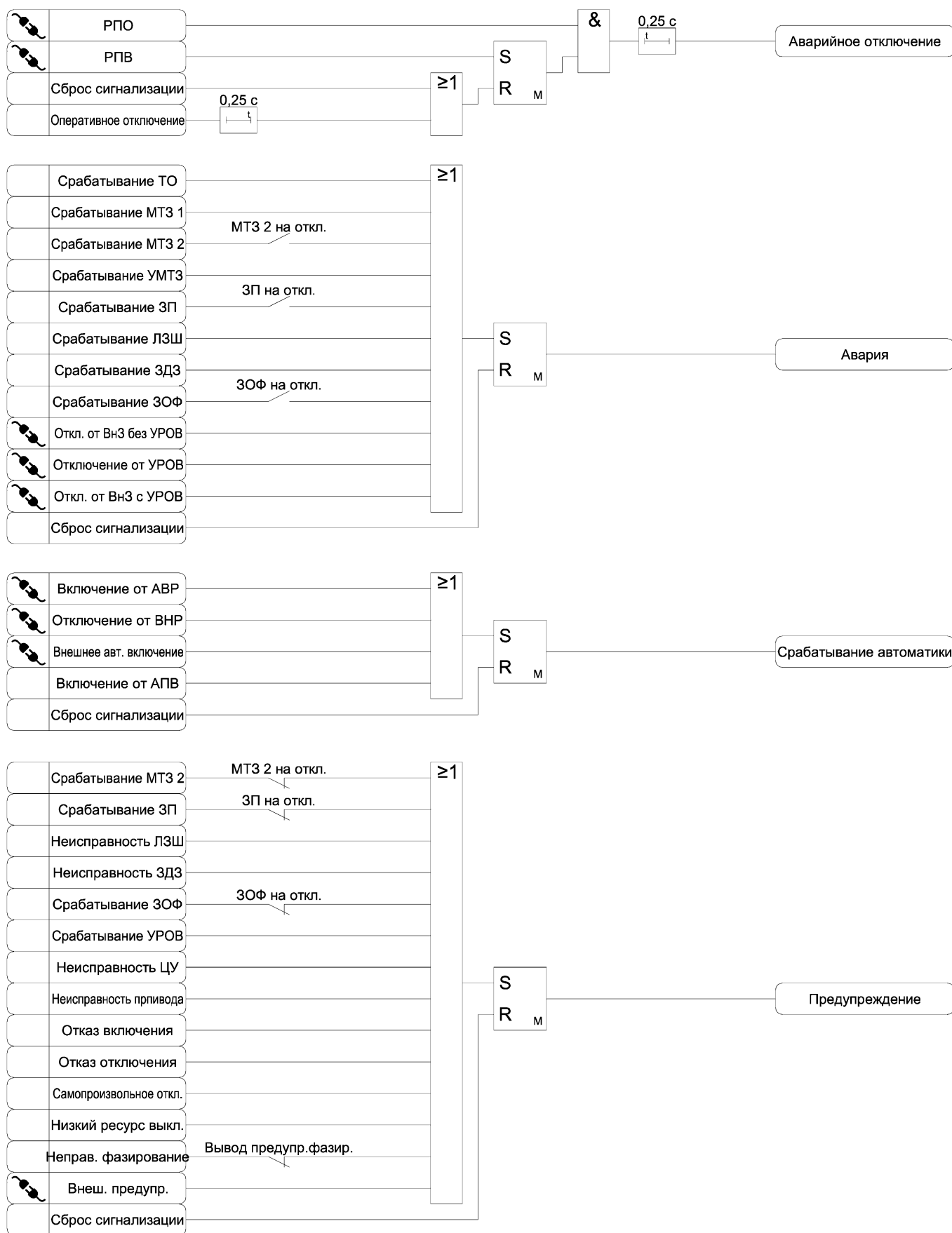
Рисунок 3.15 – Функциональная схема алгоритма сигнализации
