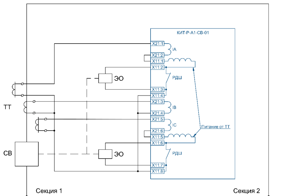
а) схема с тремя ТТ
