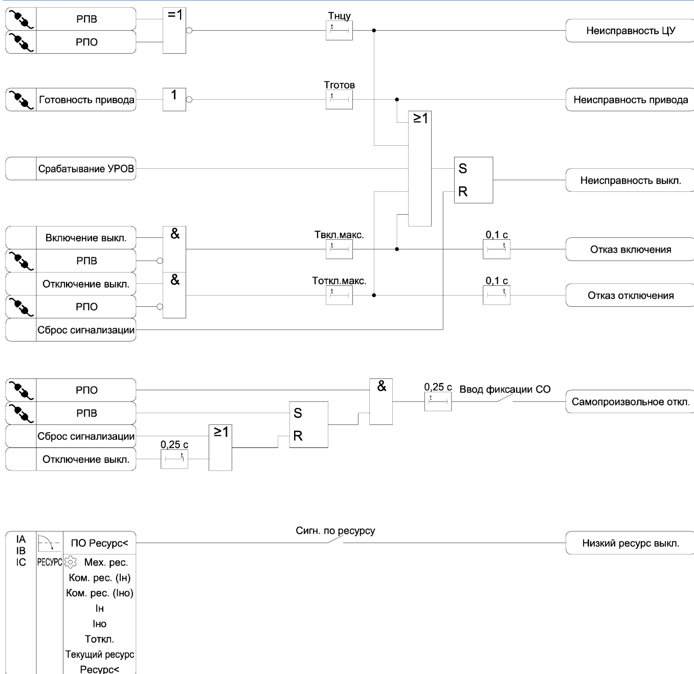
Рисунок 3.14 – Функциональная схема алгоритма диагностики выключателя
