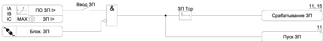
Рисунок А.4 – Функциональная схема алгоритма ЗП
