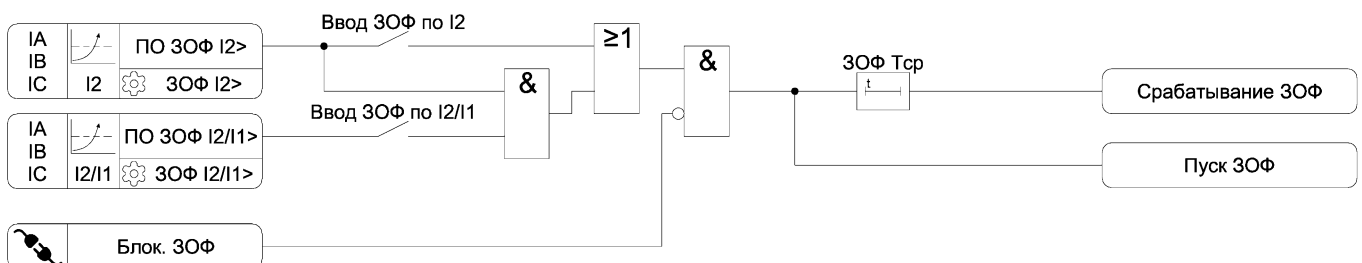
Рисунок 3.7 – Функциональная схема алгоритма ЗОФ
