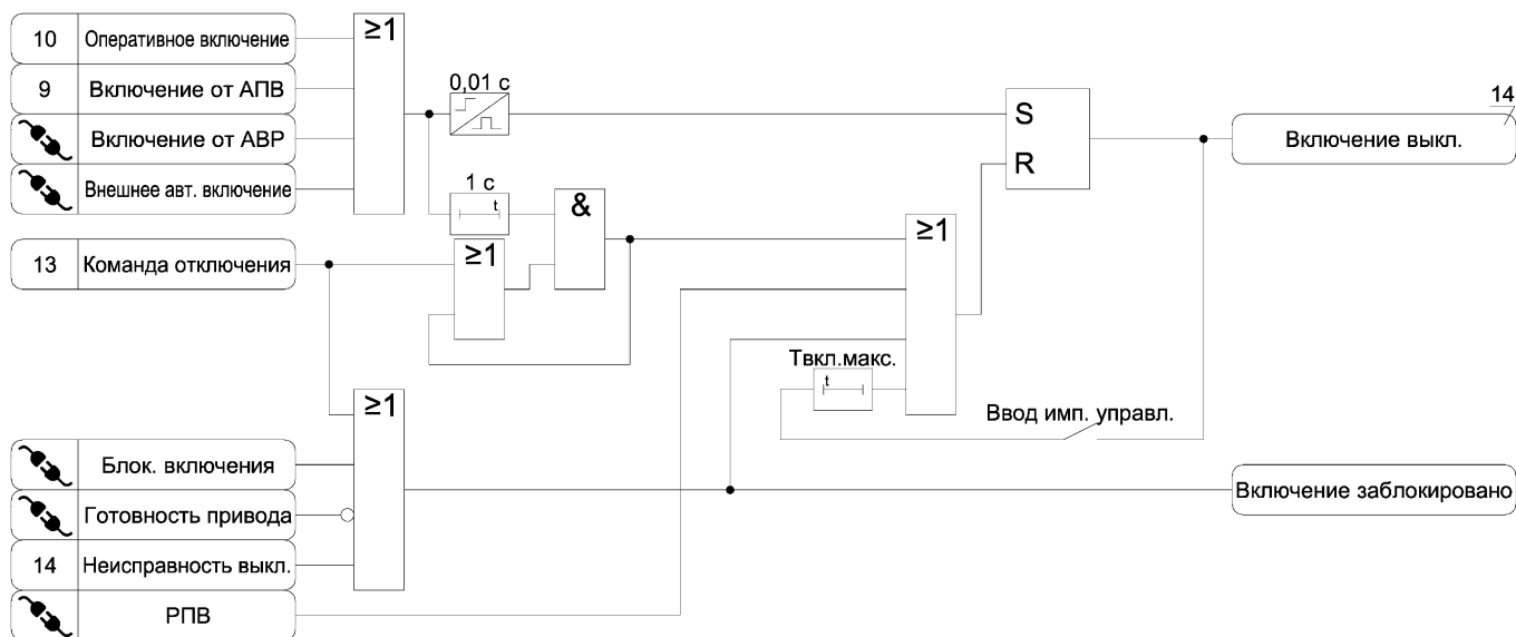
Рисунок А.12 – Функциональная схема алгоритма включения выключателя
