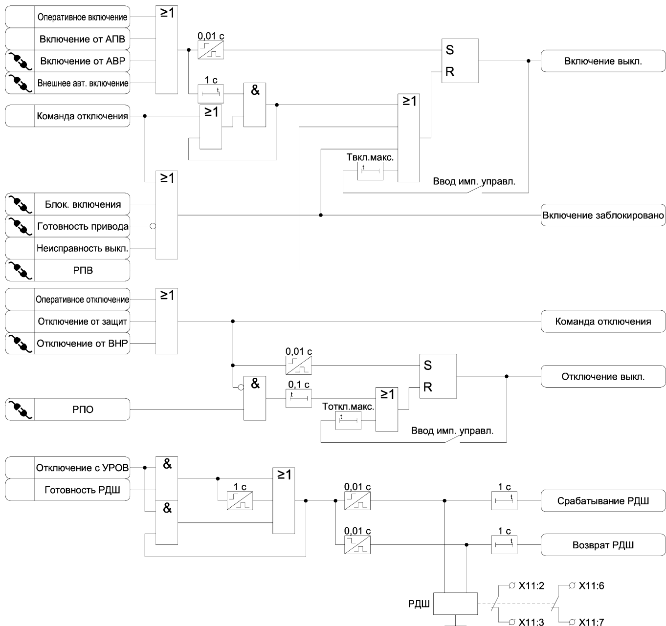
Рисунок 3.13 – Функциональная схема алгоритма управления выключателем
