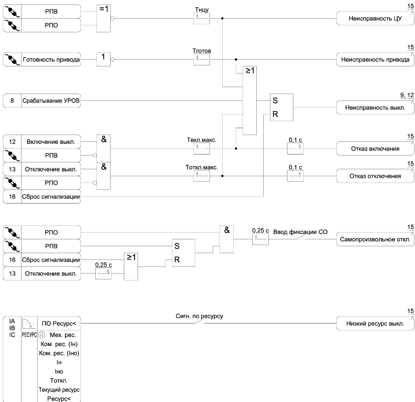
Рисунок А.14 – Функциональная схема алгоритма диагностики выключателя
