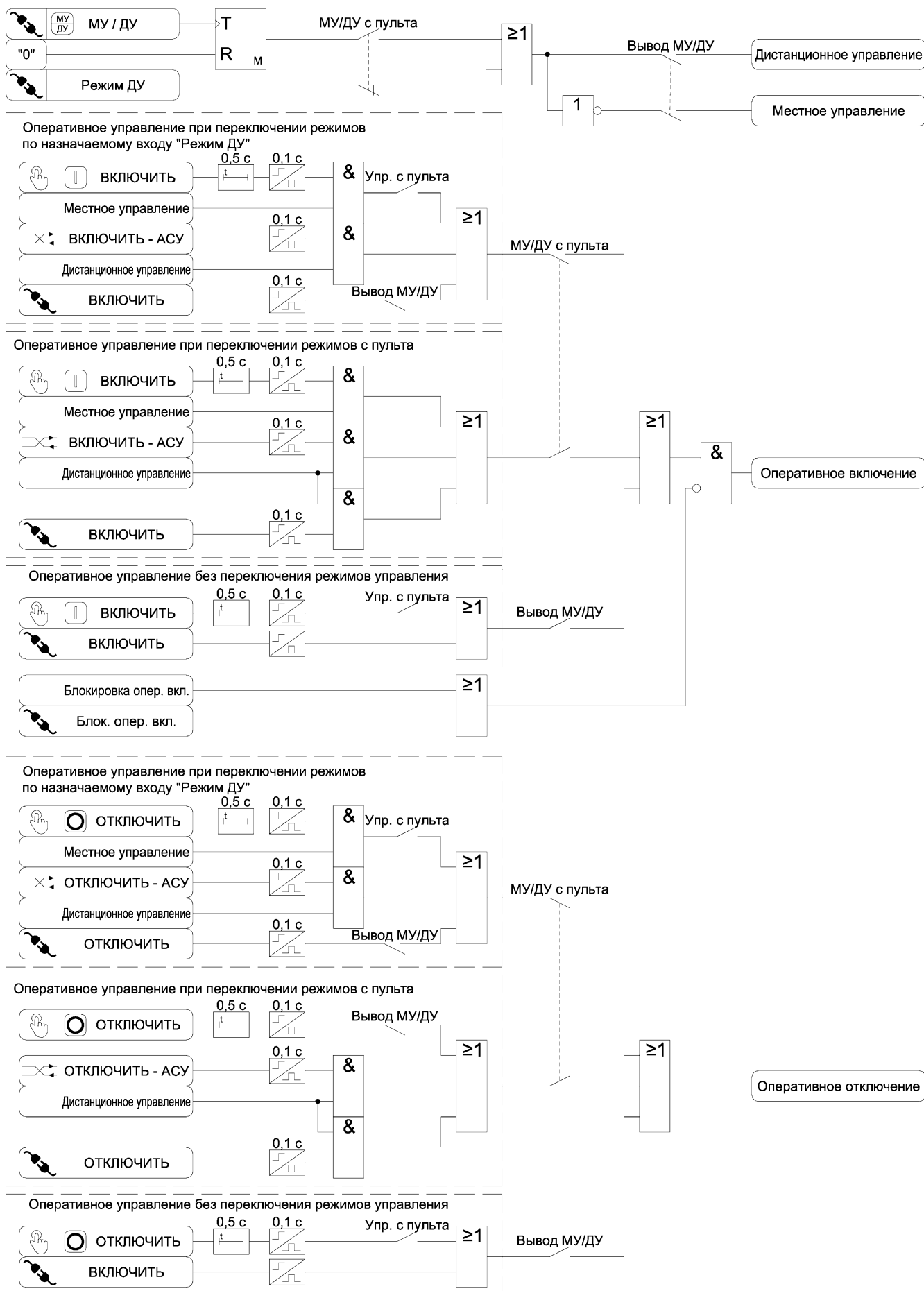
Рисунок 3.10 – Функциональная схема алгоритма оперативного управления выключателем
