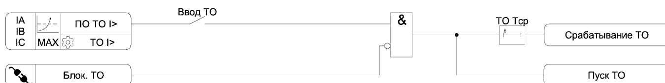
Рисунок 3.1 – Функциональная схема алгоритма ТО
