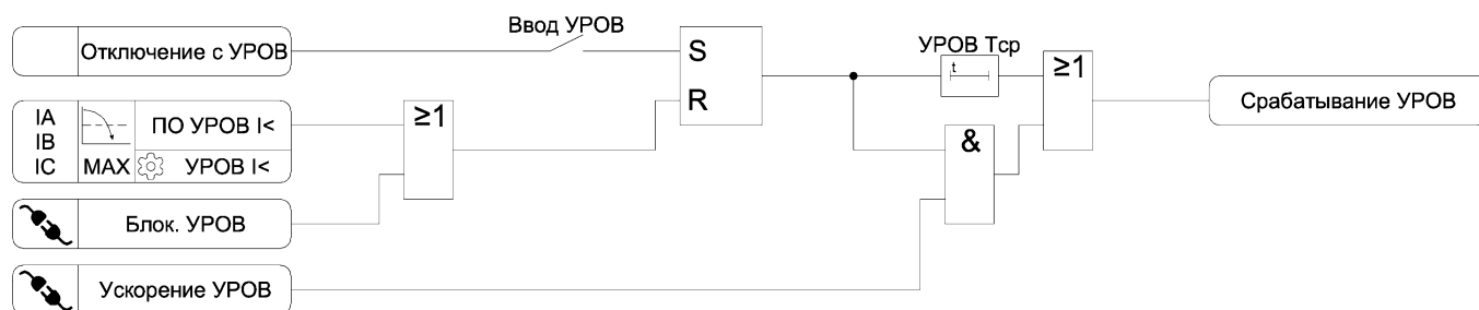
Рисунок 3.8 – Функциональная схема алгоритма УРОВ
