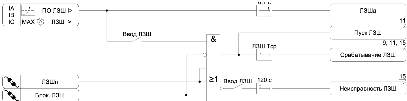
Рисунок А.5 – Функциональная схема алгоритма ЛЗШ
