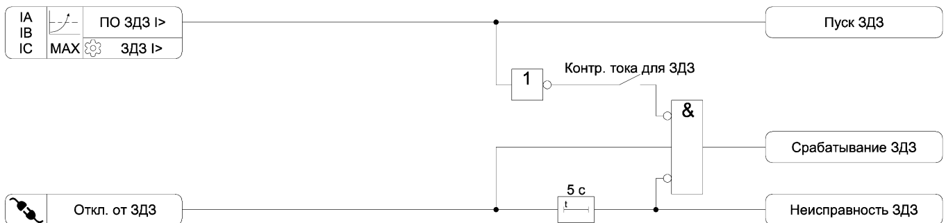
Рисунок 3.6 – Функциональная схема алгоритма ЗДЗ
