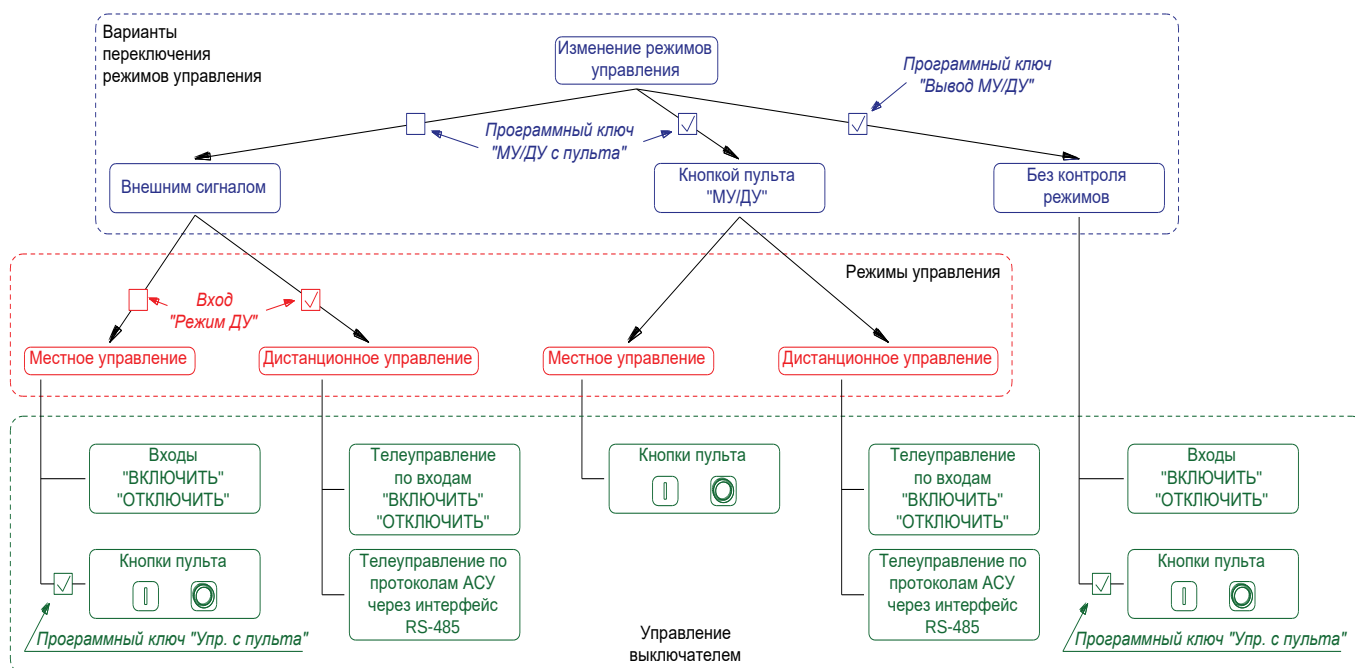
Рисунок 3.11 – Выбор режимов управления
