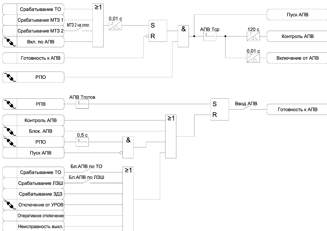
Рисунок 3.9 – Функциональная схема алгоритма АПВ
