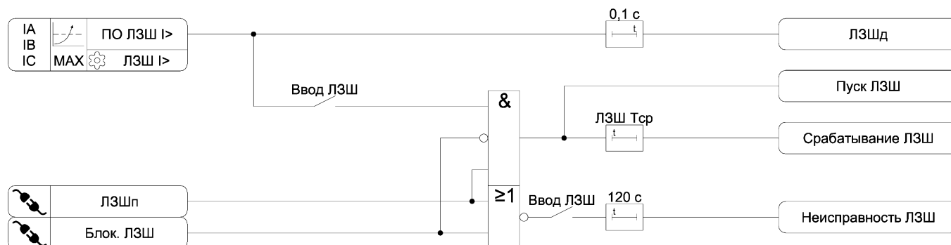
Рисунок 3.5 – Функциональная схема алгоритма ЛЗШ
