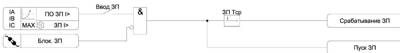
Рисунок 3.4 – Функциональная схема алгоритма ЗП
