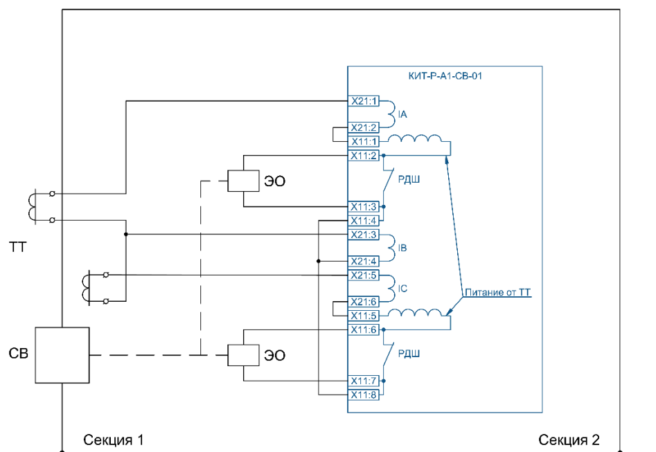
б) схема с двумя ТТ
