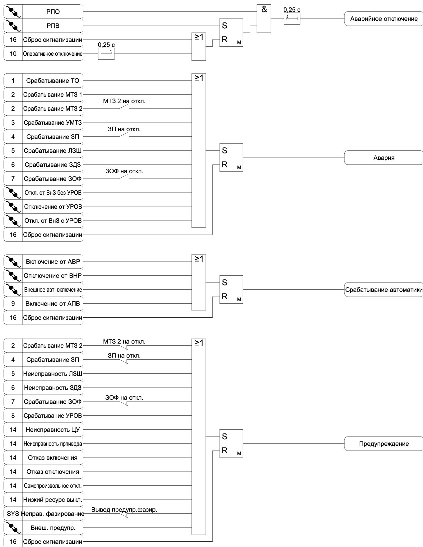
Рисунок А.15 – Функциональная схема алгоритма сигнализации
