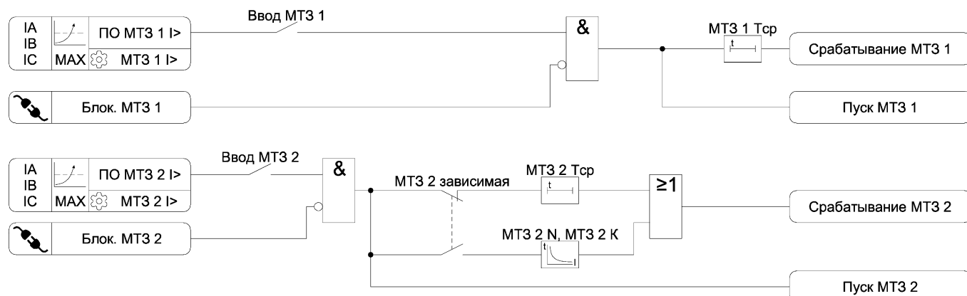
Рисунок 3.2 – Функциональная схема алгоритма МТЗ
